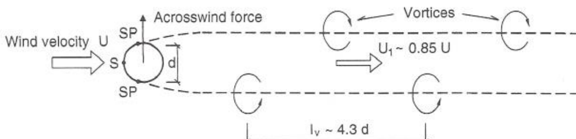
Figura 2.11 Desprendimiento alternado de vórtices. Recuperado de: https://bit.ly/2VdqU8w el 25 de febrero, 2019.
