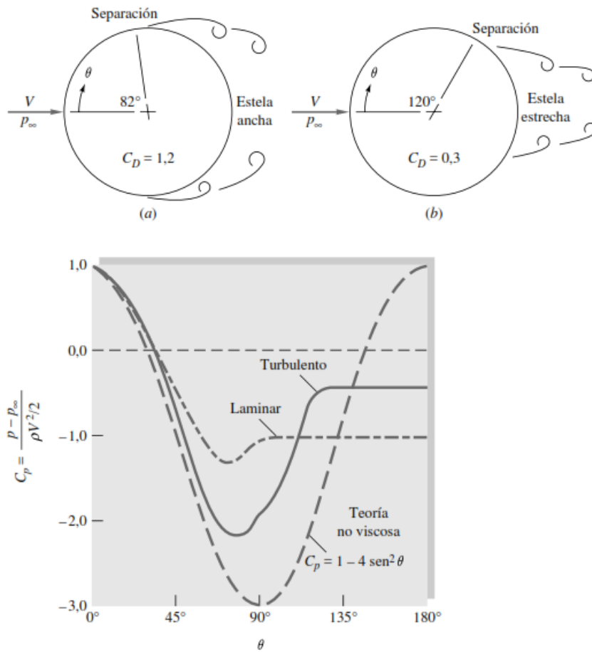
Figura 2.7 Comportamiento de un flujo alrededor de un tubo de sección circular. Recuperado de: Mecánica de fluidos , F. White. sexta edición
