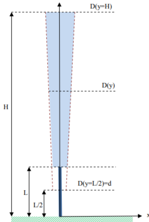
Figura 3.7 Modelo geométrico.
