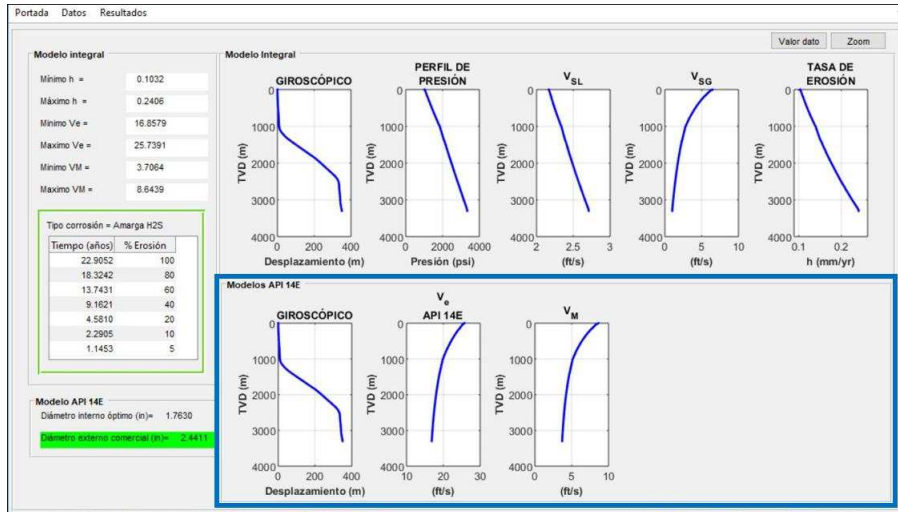
Figura 6.16: Gráficas de norma API 14E.
