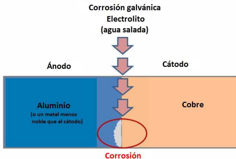
Figura 2.4: Corrosión galvánica [21].
