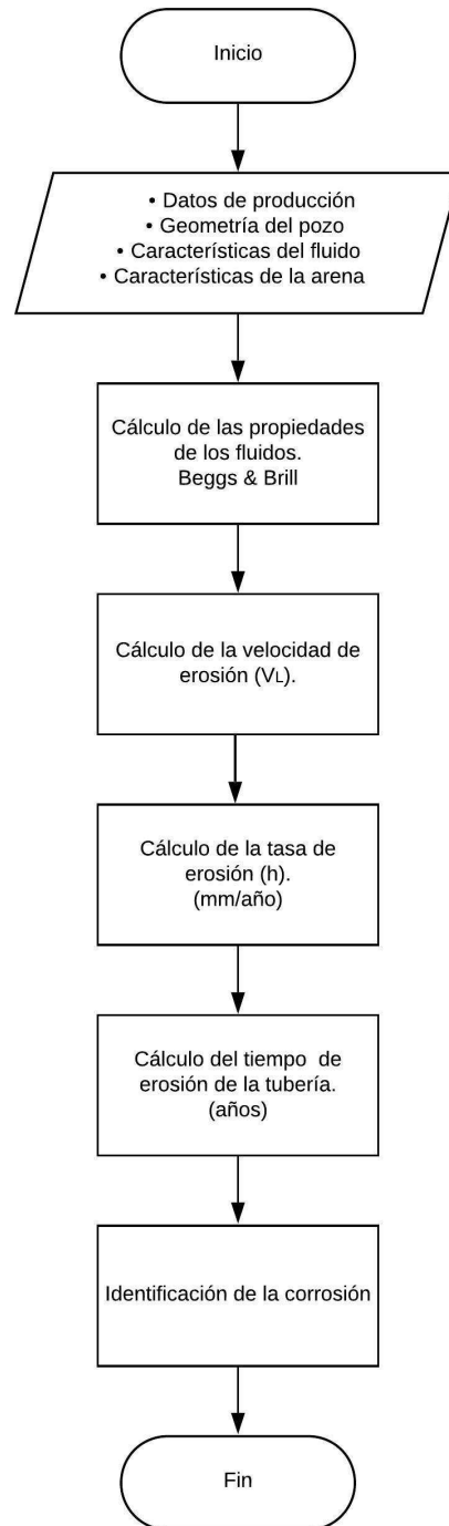
Figura 4.2: Diagrama de flujo de modelo de erosión - corrosión.
