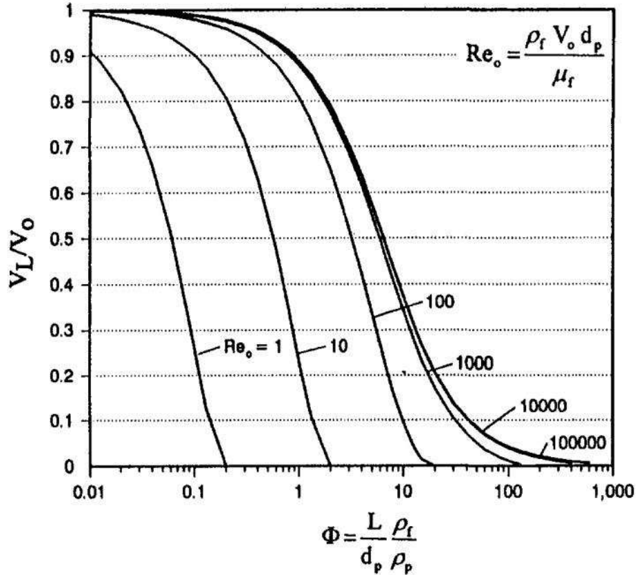
Figura 3.2: Gráfica para obtener la velocidad de impacto de la partícula, Shirazi, McLaury y Shadeley (1995) [31].
