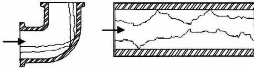
Figura 3.1: Colisión directa y aleatoria en codos y tuberías, Ahlert (1994)[30].
