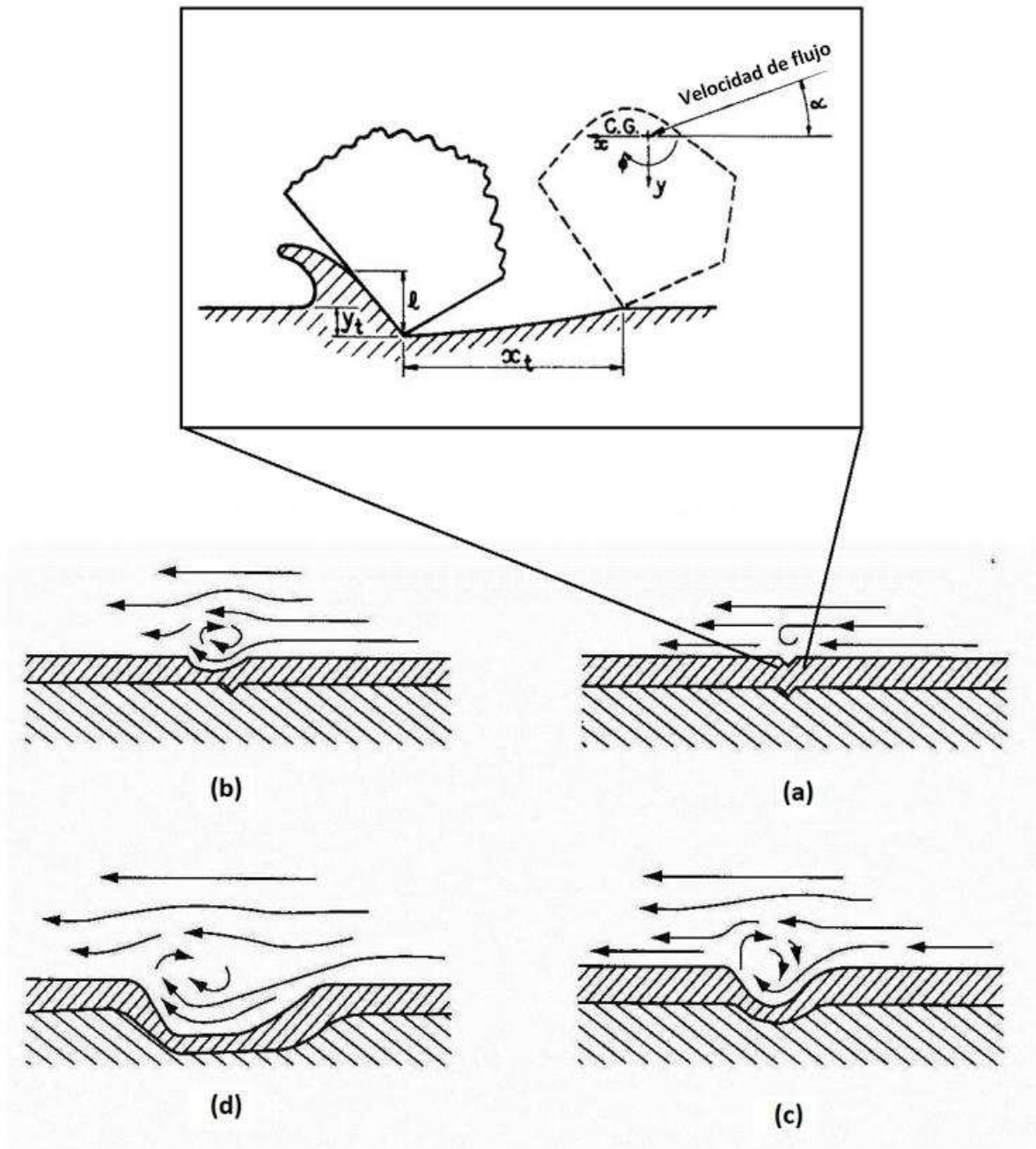
Figura 4.1: Imagen idealizada de grano abrasivo golpeando una superficie y eliminando material [28].
