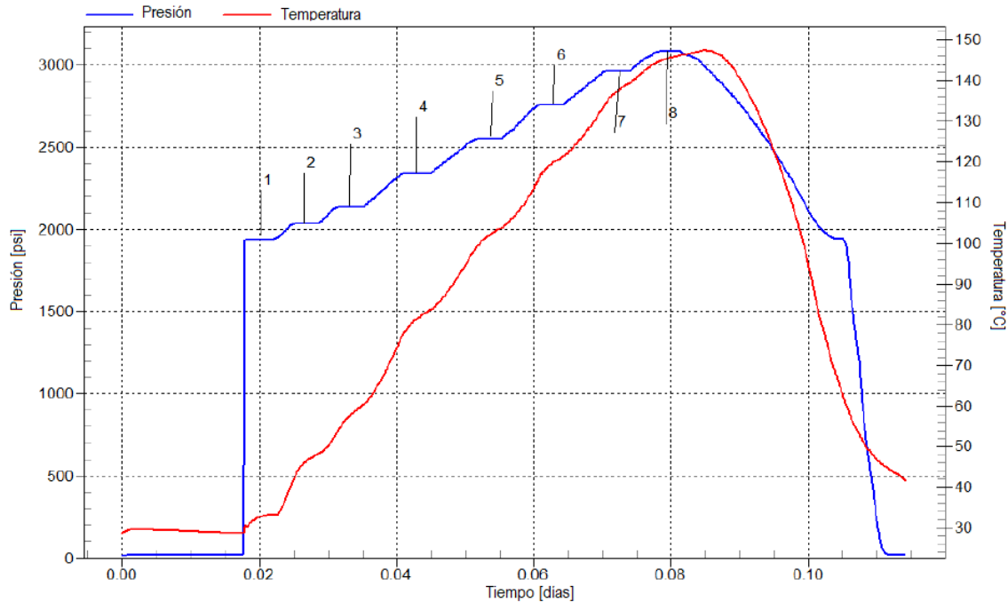
Fig. II.3.2.1.1 Gráfico representante de presión contra tiempo contra temperatura en un RPF, (MSSM).
