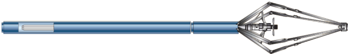
Fig. I.3.1.1 Medidor de flujo con molinete, ( Principles of production logging, Schlumberger ).
