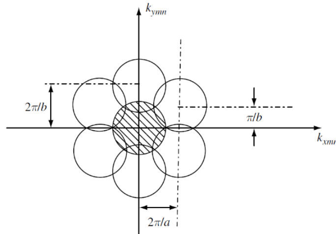
Figura 3.13: modos Floquet en una malla triangular equilateral.
