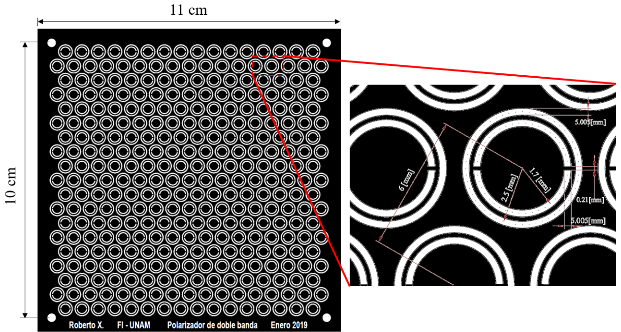
Figura 4.1: Mascara para la SSF del polarizador de doble banda.
