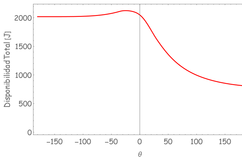
Figura 5.14. Variación de la disponibilidad total.
