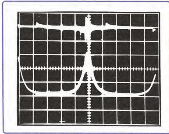
Figura 2.11. Diagrama P-t de un motor de combustión interna [20].
