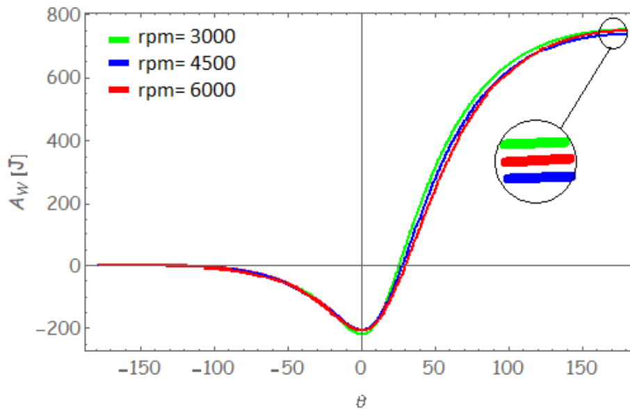
Figura 5.28. Disponibilidad por transferencia de trabajo.
