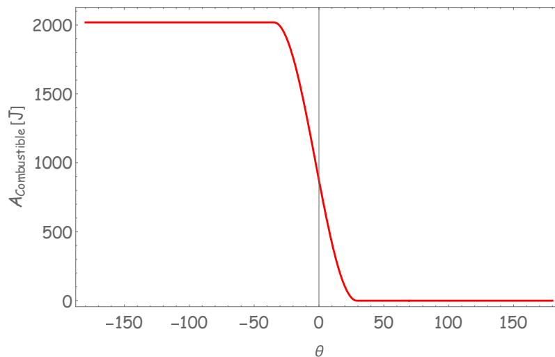
Figura 5.12. Variación de la disponibilidad del combustible.
