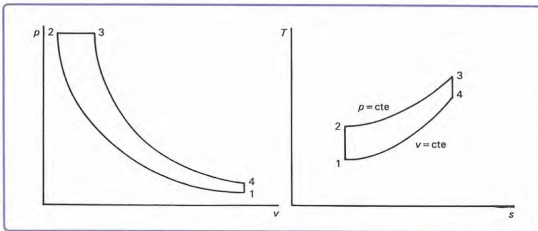
Figura 2.12. Diagrama pv y Ts para el ciclo Diesel [20].
