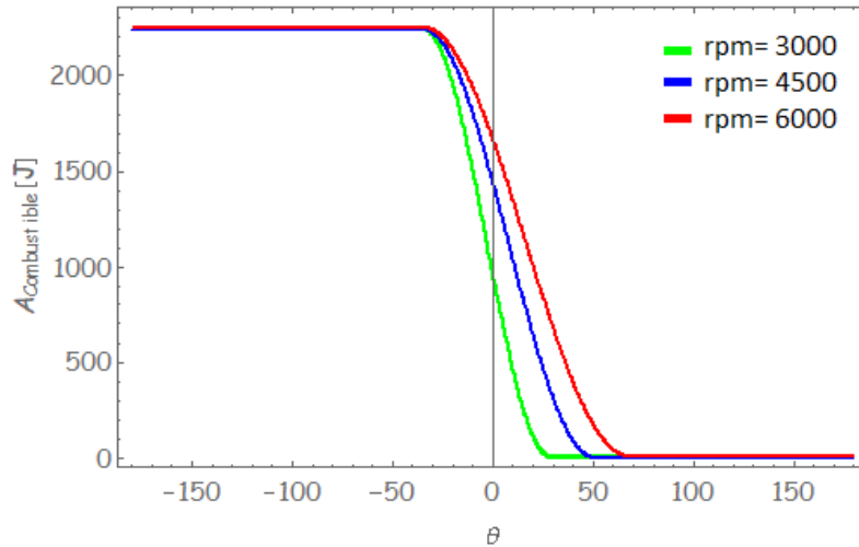
Figura 5.27. Disponibilidad del combustible con el ángulo del cigüeñal.
