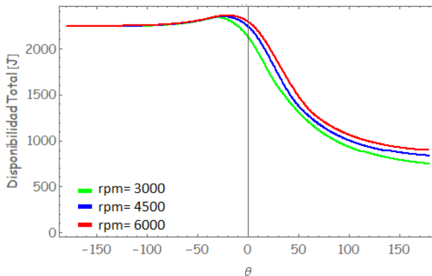
Figura 5.31. Disponibilidad total del sistema.
