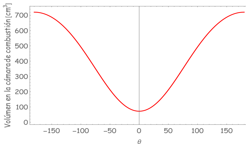
Figura 5.1. Variación del volumen con el ángulo del cigüeñal.
