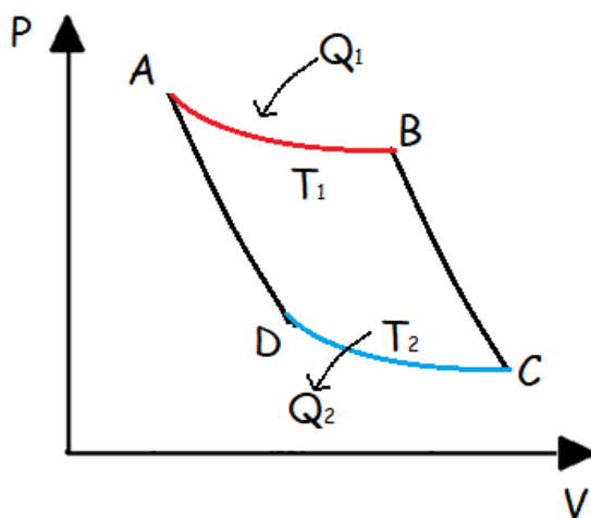
Figura 2.3. Ciclo de Carnot.
