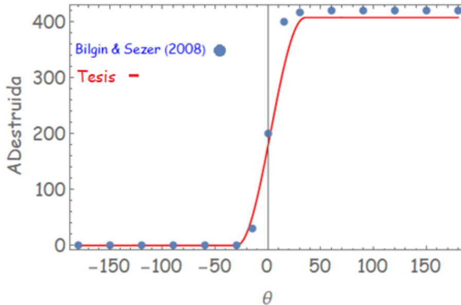
Figura 4.7 Comparación de las irreversibilidades que se generan en la cámara de combustión.
