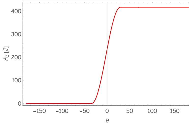
Figura 5.13. Variación de las irreversibilidades.
