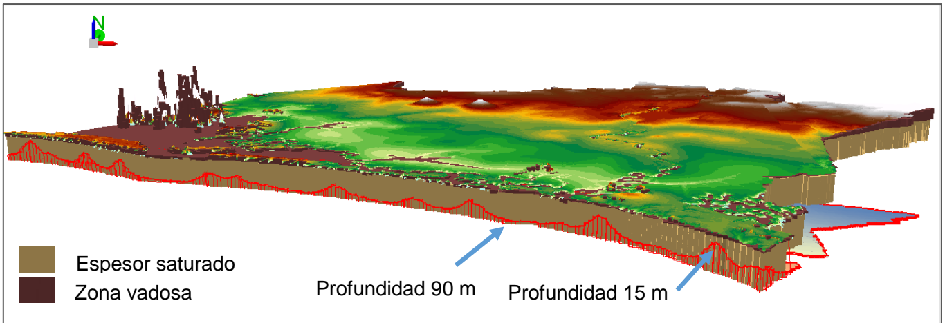
Figura 6.16. Intersección de la línea de intrusión con el acuífero a lo largo de la línea de costa.
