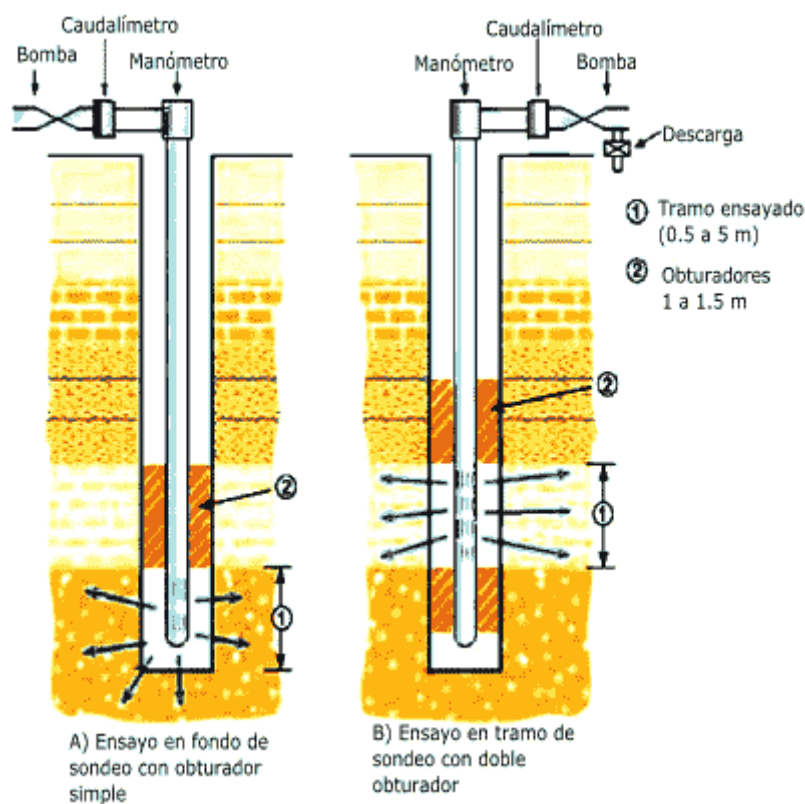
Figura 10. Obturadores para Pruebas Lugeón. El obturador simple es muy similar al empleado para inyección de lechada cemento-agua-bentonita. (Maldonado, 2018)
