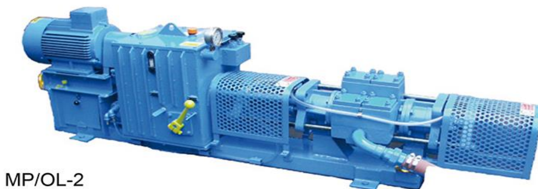
Figura 8. Bomba de inyección Clivio. (Tecopsa, s.f.)
