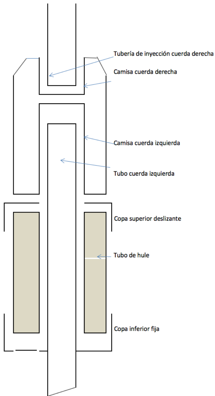
Figura 7. Corte longitudinal del obturador
