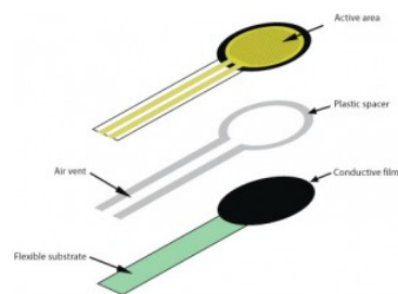
(b) Capas de un sensor resistivo FSR.
