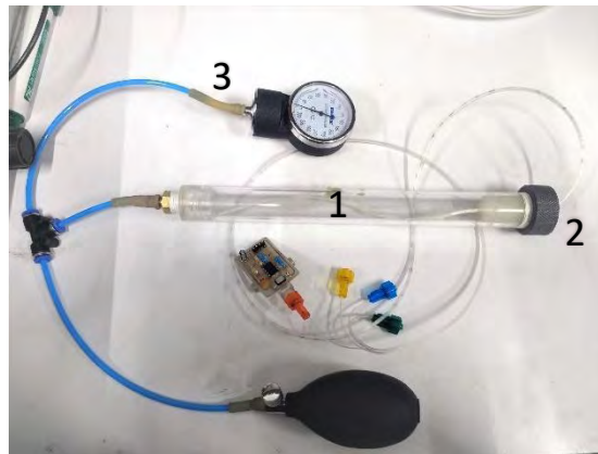
Figura 37. Cámara de presurización para pruebas
