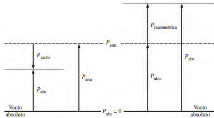
Figura 16. Presiones absoluta, de vacío y manométrica [18]
