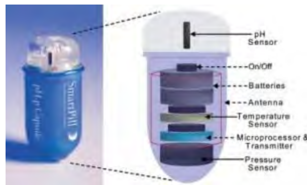
Figura 28. SmartPill [25].
