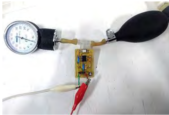
Figura 34. Configuración para pruebas del sensor de presión
