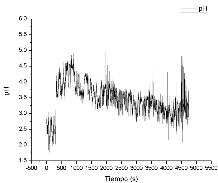
Figura 55. Datos de pH registrados durante las pruebas de variación con ácido clorhídrico
