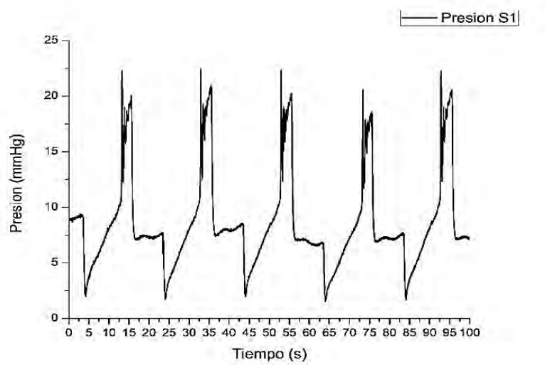
Figura 53. Patrón de presión entregado por el sensor de presión S1 durante pruebas
