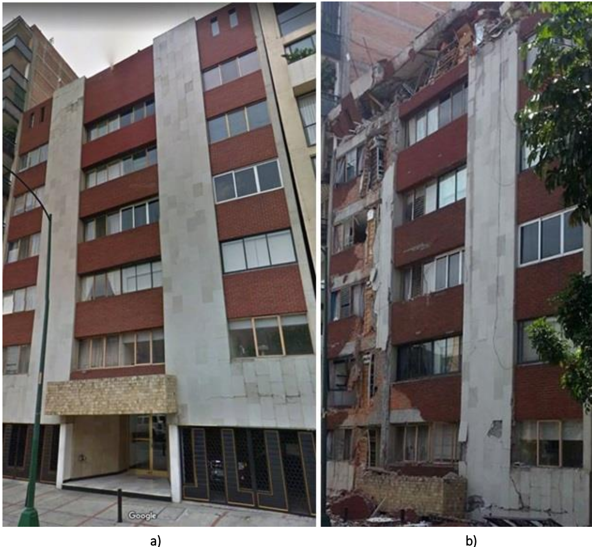
Figura A. 16 Edificio en Patricio Sanz y Xola Brujas: a) antes del evento sísmico y b) después del evento sísmico de M7.1 ( http://bit.do/d3u65 )
