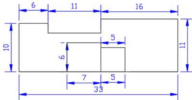
Figura C. 32 Vista en planta del edificio Colapsado en Calle Génova 33 antes del evento sísmico de M7.1
