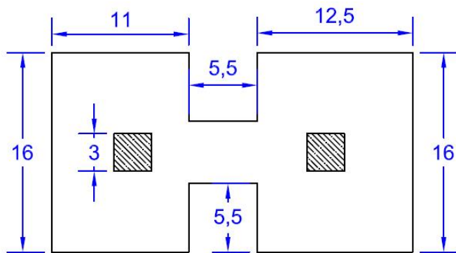
Figura C. 16 Vista en planta del edificio Colapsado en Patricio Sanz y Xola Brujas antes del evento sísmico de M7.1
