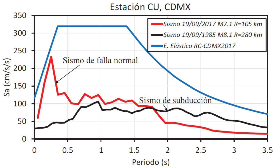
Figura 2.2 Comparación de los espectros de respuesta en terreno firme calculados para los sismos del 19 de septiembre de 2017 (M7.1) y del 19 de septiembre de 1985 (M8.1) y el espectro de diseño elástico que contempla el nuevo reglamento de construcciones de la ciudad de México en la CDMX (IIUNAM 2017)
