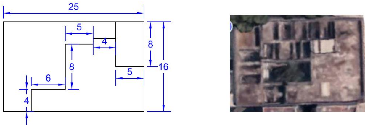
Figura C. 20 Vista en planta del edificio Colapsado en Magnolia esq. Lerdo antes del evento sísmico de M7.1
