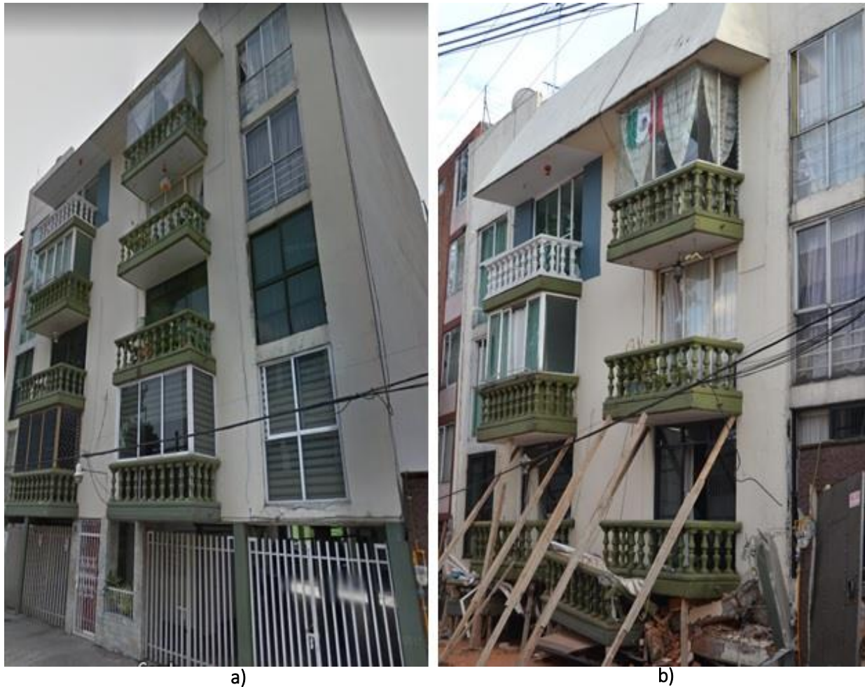
Figura A. 35 Edificio en Balsas No. 18, Miravalle: a) antes del evento sísmico y b) después del evento sísmico de M7 ( http://bit.ly/2nmr5PB )
