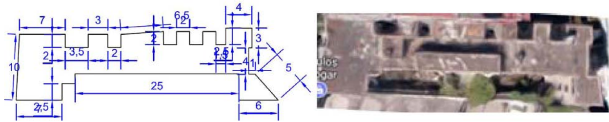
Figura C. 25 Vista en planta del edificio Colapsado en Ámsterdam 25 antes del evento sísmico de M7.1
