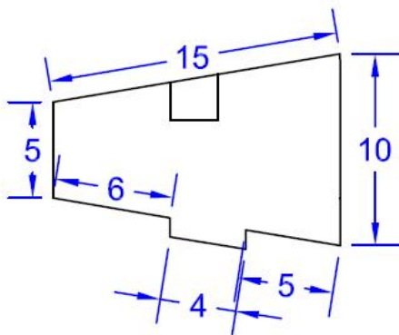
Figura C. 18 Vista en planta del edificio Colapsado en Niños Héroes 173, esquina Galicia antes del evento sísmico de M7.1
