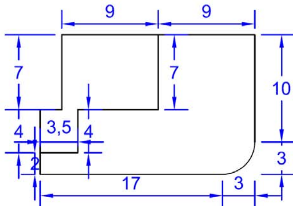
Figura C. 31 Vista en planta del edificio Colapsado en Av. México antes del evento sísmico de M7.1
