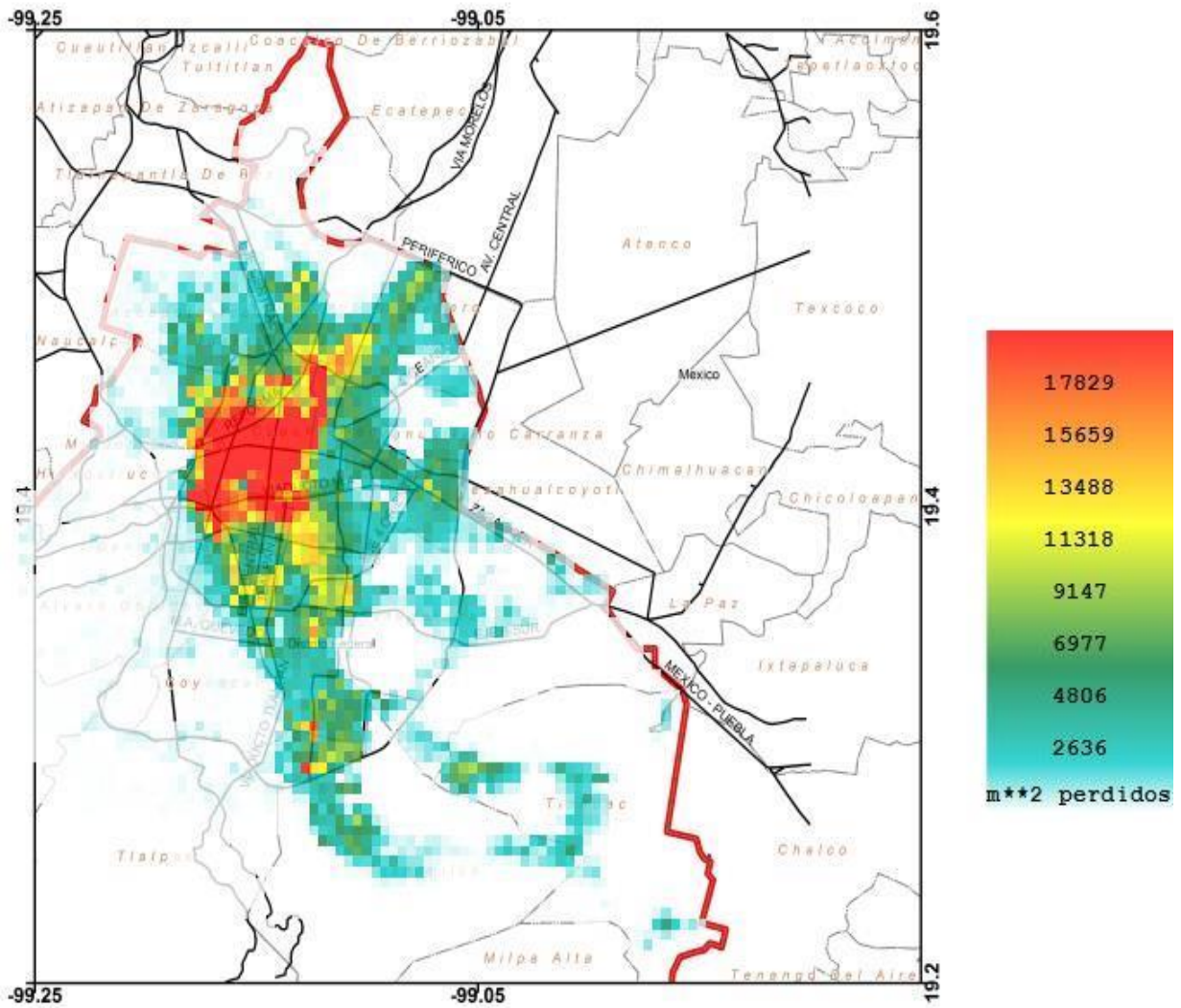
Figura 4.1 Estimación de daños en construcciones después del evento sísmico del 19/9/2017 de M7.1 (IIUNAM 2017)
