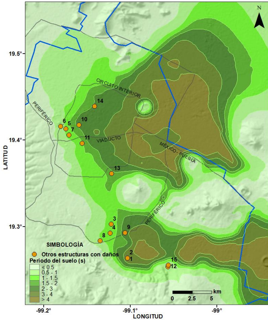
Figura 3.2 Estructuras con daños y periodos de suelo en la CDMX 2017
