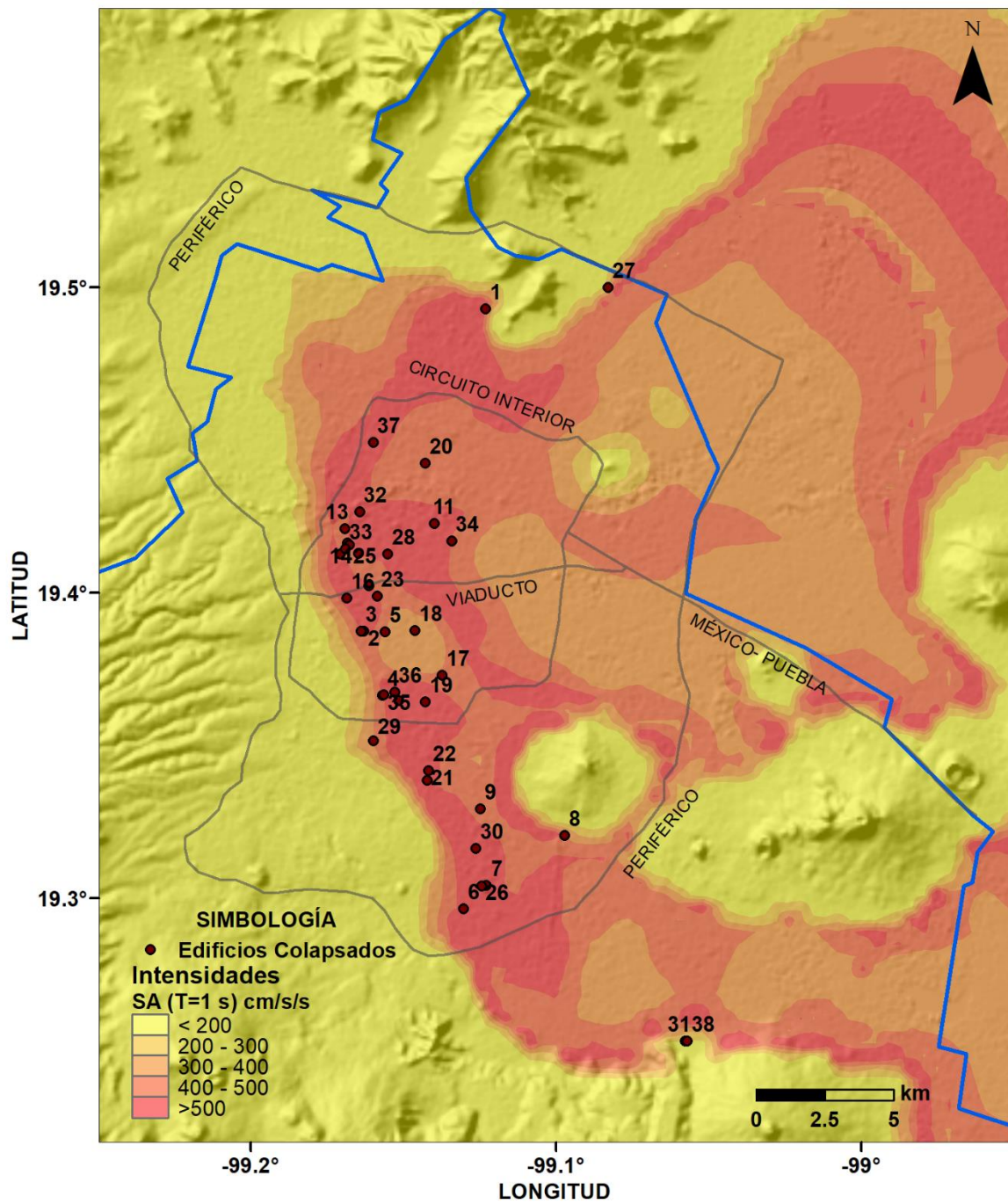
Figura 3.4 Construcciones colapsadas y distribución de las intensidades sísmicas asociadas a un periodo estructural de T=1s en la CDMX
