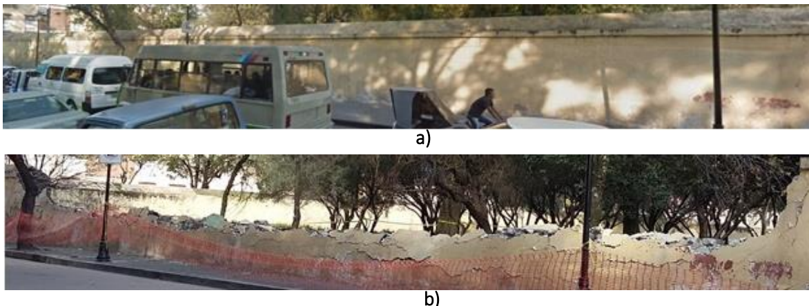
Figura B. 2 Barda de la iglesia de San Bernardino de Siena en Lirio Acuático y Av. 16 de septiembre: a) antes del evento sísmico y b) después del evento sísmico de M7.1 (imágenes obtenidas de Google Maps)
