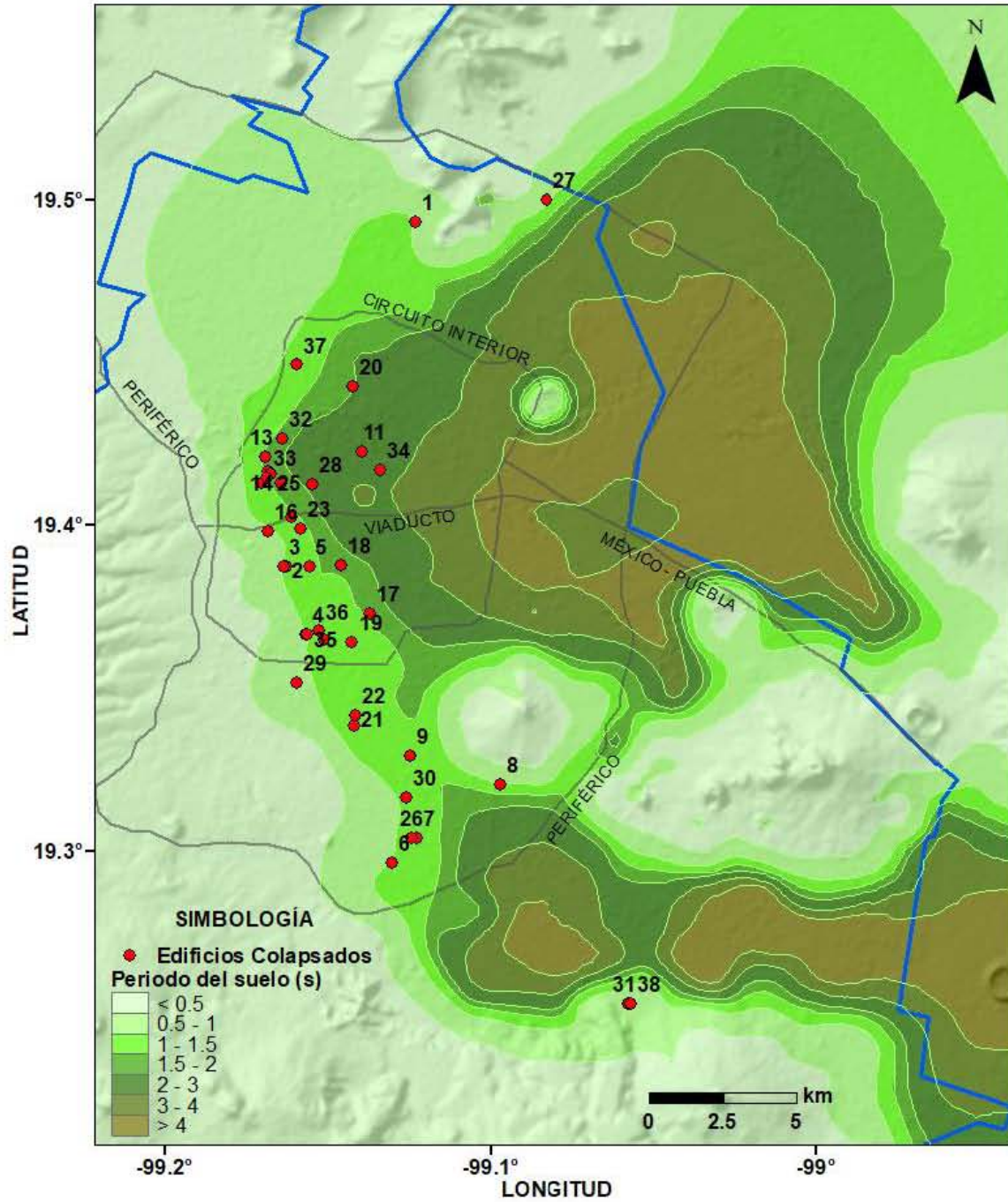
Figura 3.1 Edificios colapsados y periodos de suelo en la CDMX 2017
