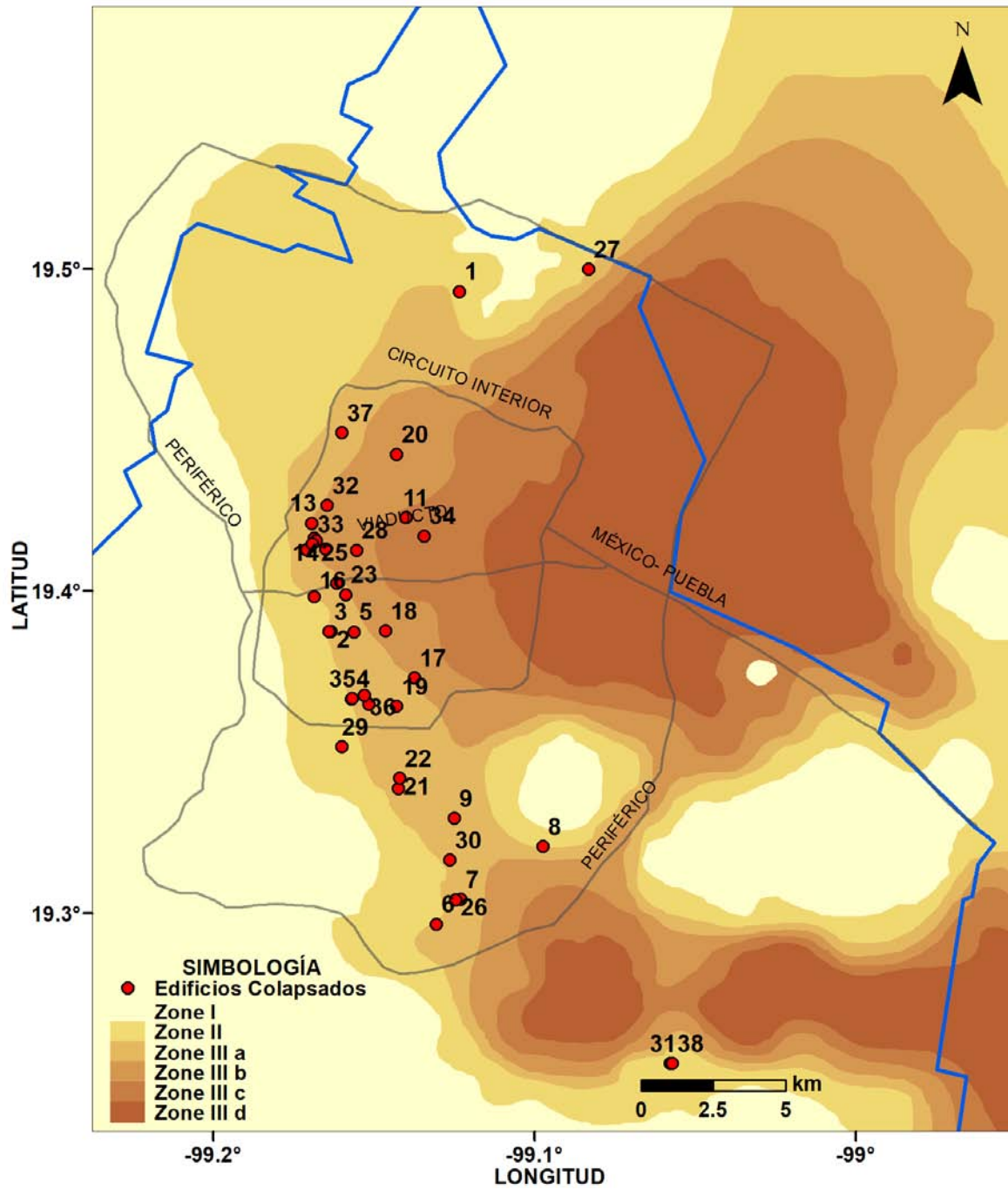
Figura 3.3 Construcciones colapsadas y ubicación de estas acorde a la zona geotécnica en la CDMX
