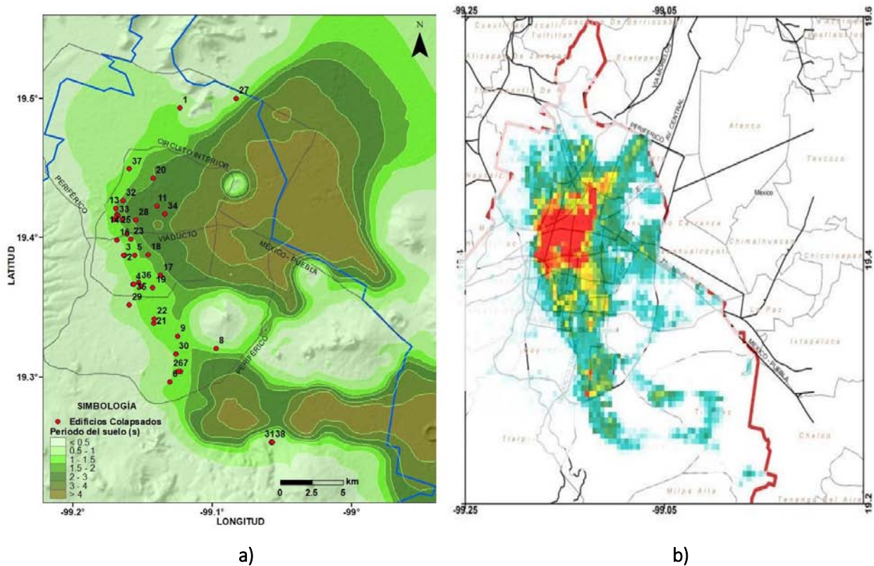
Figura 4.4 Comparación de los mapas de las edificaciones colapsadas tras el evento sísmico de M7.1 el 19/09/2017 en la CDMX: a) Mapa generado con el programa ARGIS 2017 y b) Mapa generado por el sistema de estimación temprana del IIUNAM 2017
