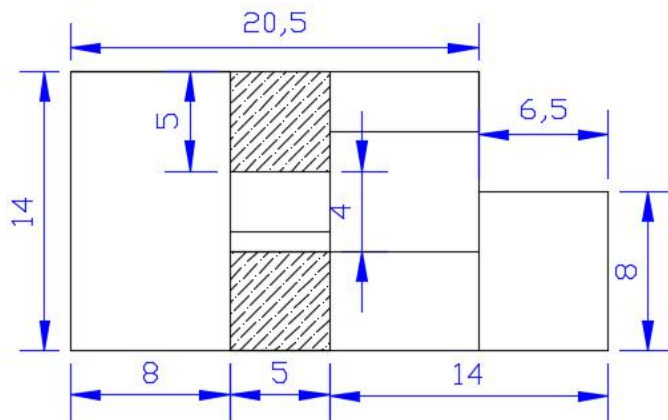
Figura C. 33 Vista en planta del edificio Colapsado en Sonora 149 antes del evento sísmico de M7.1
