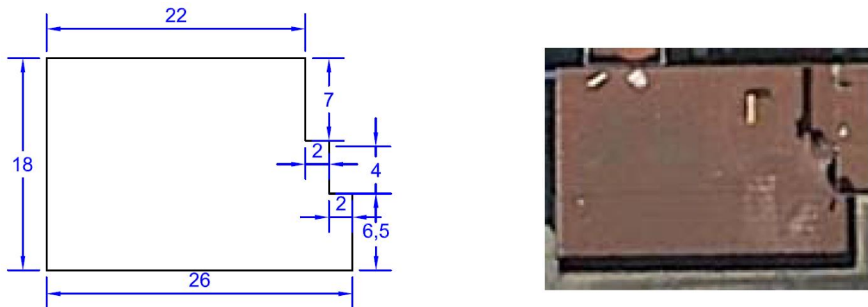
Figura C. 26 Vista en planta del edificio Colapsado en Calzada del Hueso 480 antes del evento sísmico de M7.1
