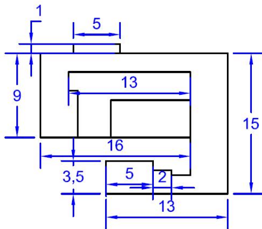
Figura C. 10 Vista en planta del edificio Colapsado en Amsterdam 107 antes del evento sísmico de M7.1
