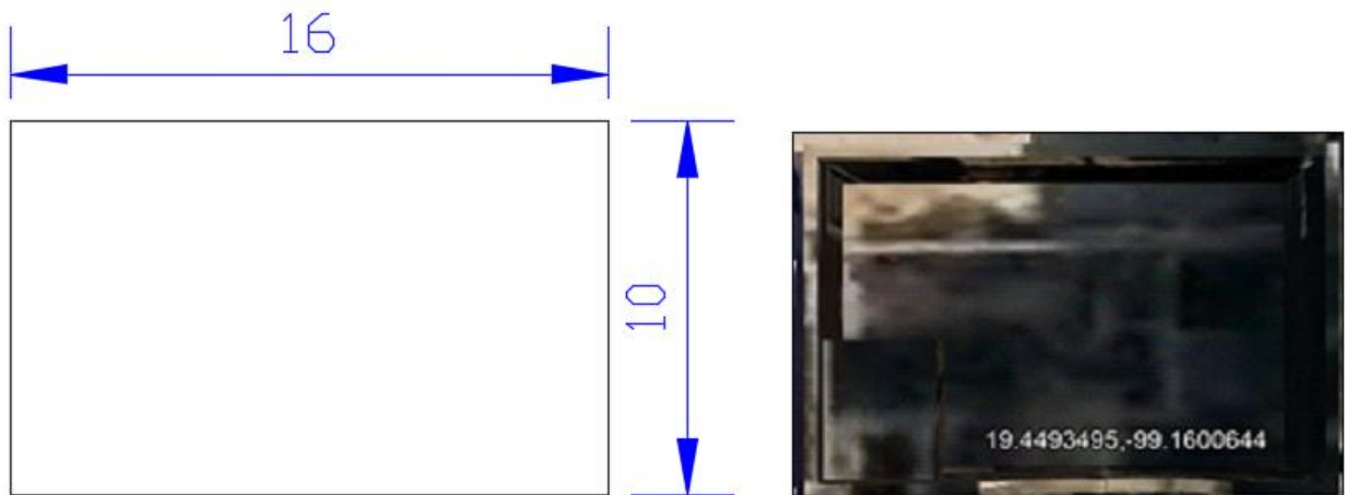
Figura C. 38 Vista en planta del edificio Colapsado en Sabino esquina Diaz Mirón antes del evento sísmico de M7.1
