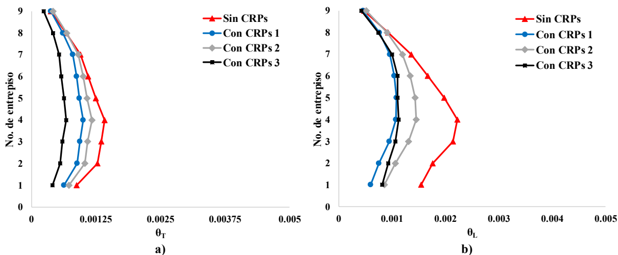
Fig. 4.12 Distorsiones de entrepiso para 0.025 g, registro SXP8509
