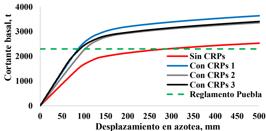
Fig. 4.10 Curva de capacidad en T
