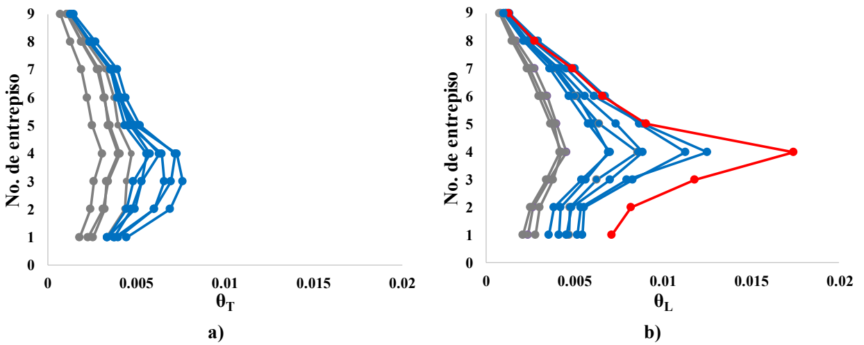
Fig. 3.9 Distorsiones con intensidad de 0.12 g
