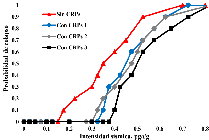
Fig. 4.23 Curvas de probabilidad de colapso
