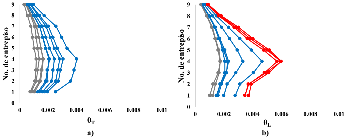
Fig. 3.8 Distorsiones con intensidad de 0.05 g
