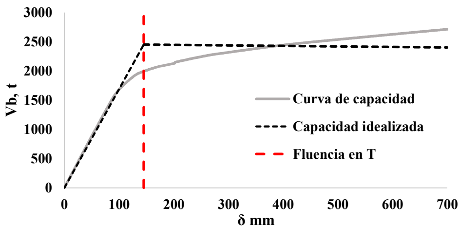
Fig. 4.2 Curva de capacidad en dirección T
