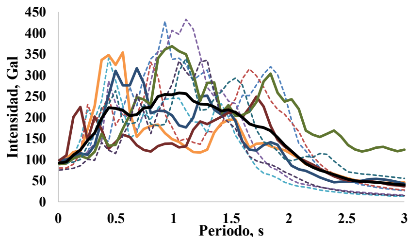
Fig. 3.5 Espectros de respuesta de los sismos utilizados
