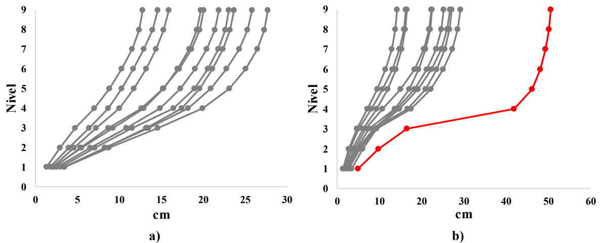
Fig. 3.6 Desplazamientos laterales con intensidad de 0.2 g
