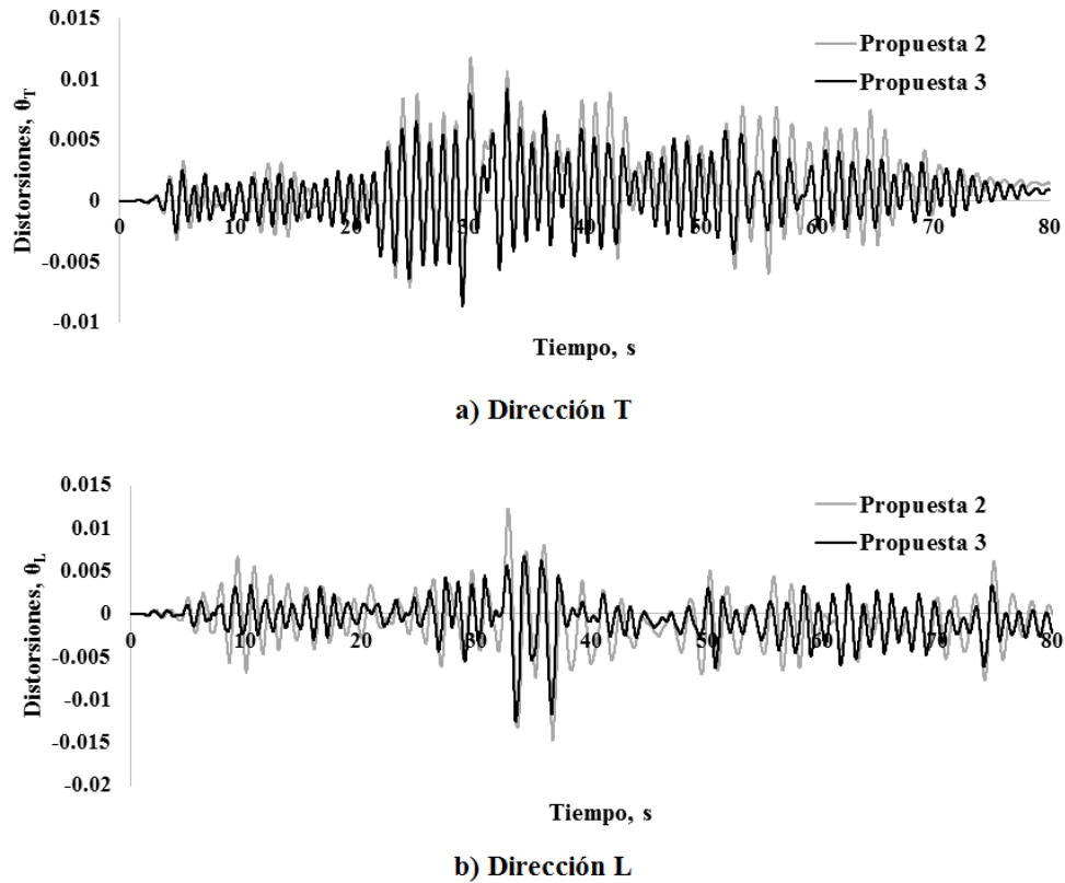
Fig. 4.19 Historia de distorsiones del cuarto entpiso para el registro UC449906
