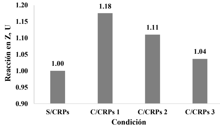
Fig. 4.22 Carga vertical en la cimentación
