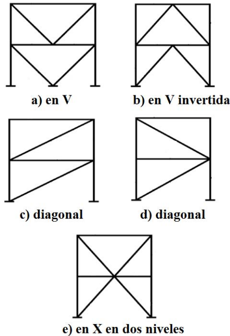
Fig. 2.6 Configuraciones de contraventeos, NTCEM-16
