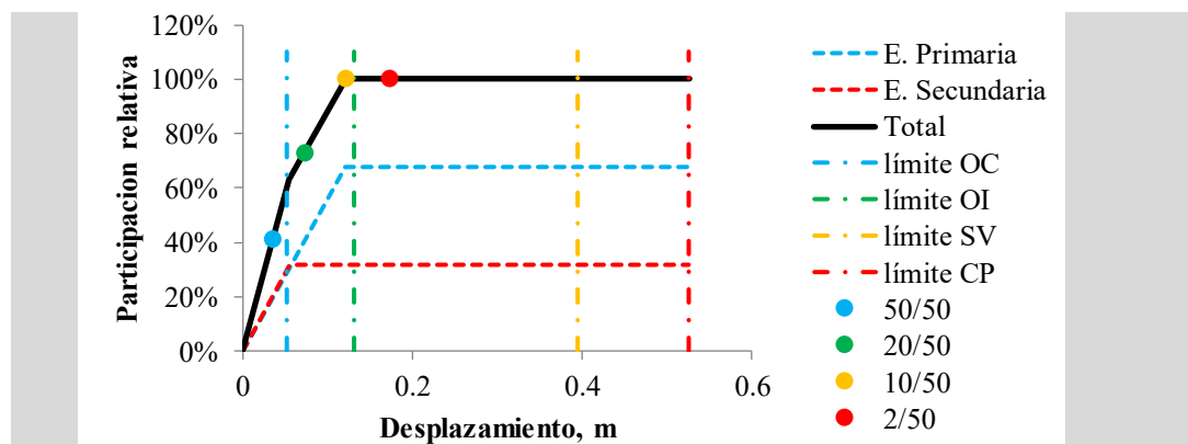
Fig. 4.7 Demanda de desplazamientos del sistema dual en L
