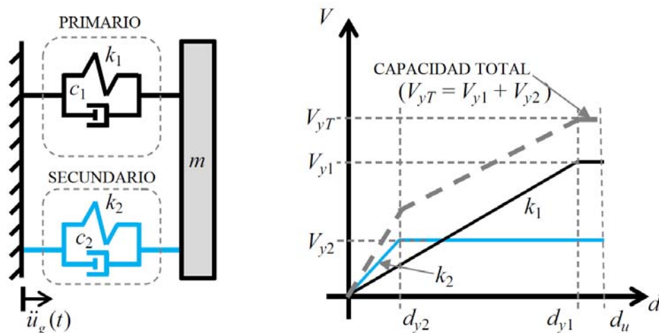
Fig. 2.1 Oscilador dual equivalente a 1GDL y sus curvas de comportamiento, Guerrero et al., 2016.
