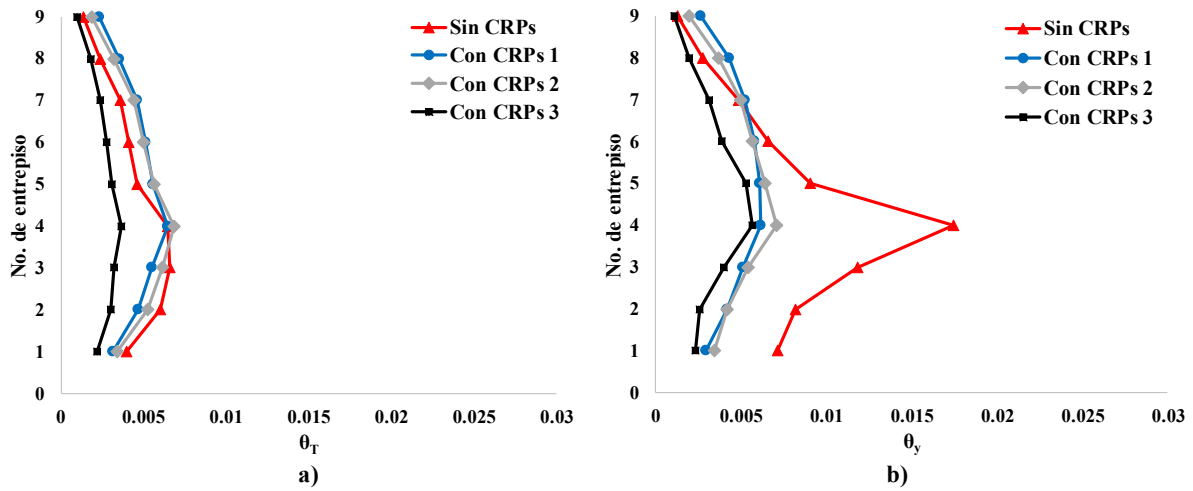
Fig. 4.14 Distorsiones de entrepiso para 0.12 g, registro SXPU8509
