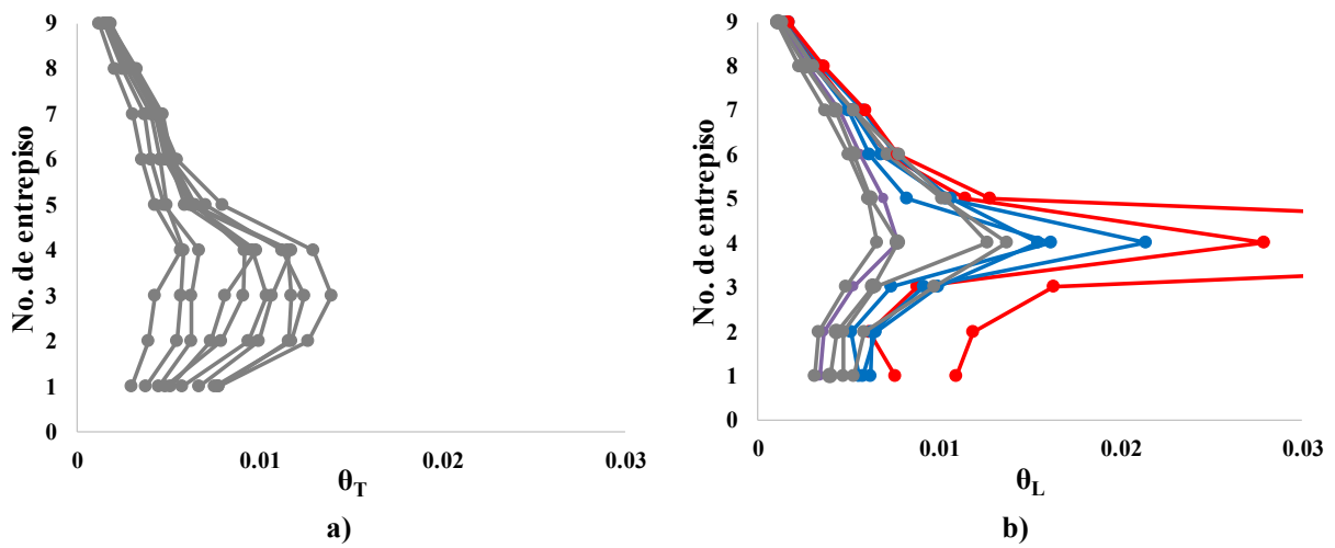
Fig. 3.10 Distorsiones con intensidad de 0.2 g
