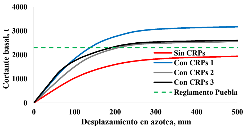
Fig. 4.11 Curva de capacidad en L
