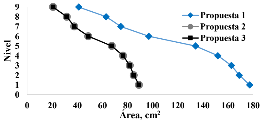
Fig. 4.9 Áreas de acero en L
