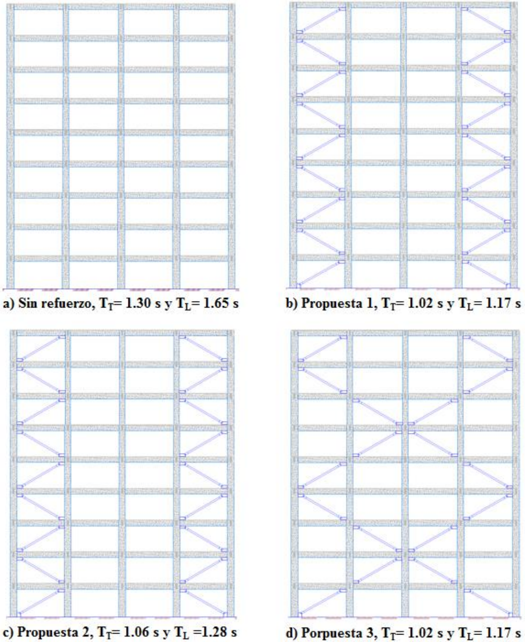
Fig. 4.1 Distribuciones propuestas para los CRPs
