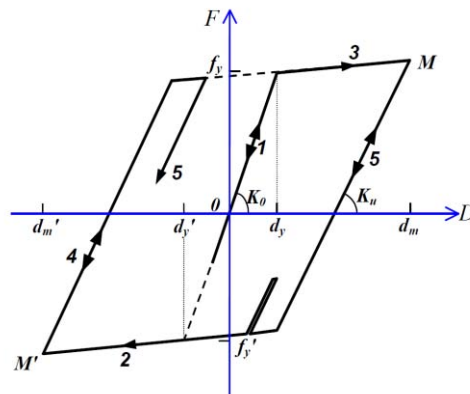
Fig. 3.2 Modelo bilineal degradante
