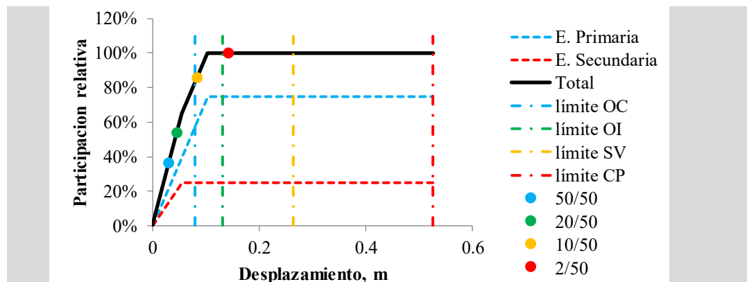
Fig. 4.6 Demanda de desplazamientos del sistema dual en T
