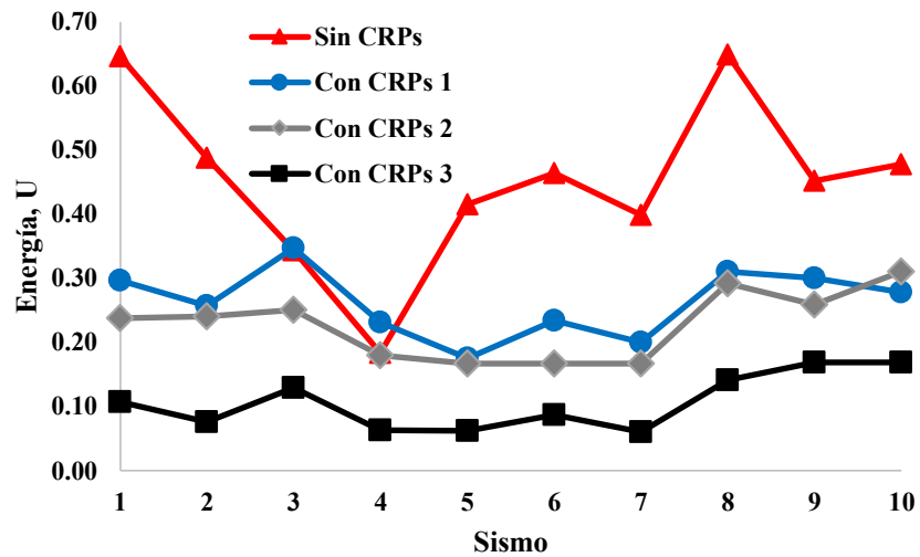
Fig. 4.20 Energía disipada para una intensidad de 0.2g: estructura primaria
