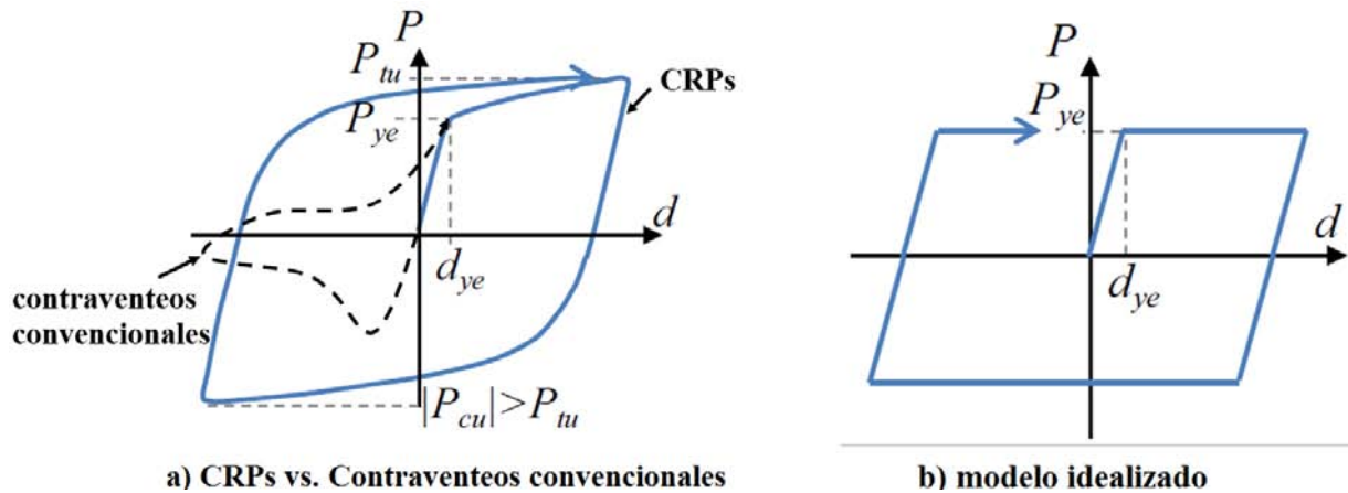
Fig. 2.5 Comportamiento histerético de CRPs.
