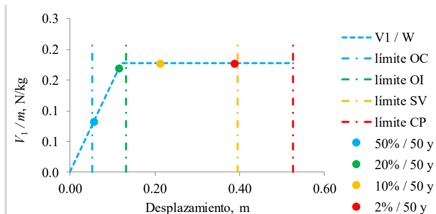
Fig. 4.5 Demanda de desplazamientos del sistema de 1GDL en L
