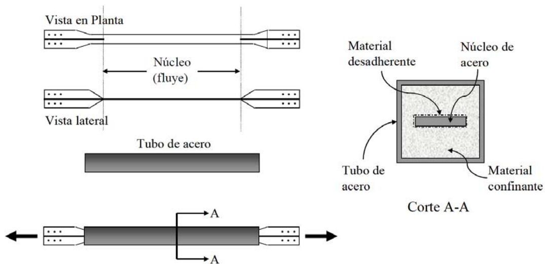
Fig. 2.4 Esquema de los CRPs (Terán y Virto, 2009)
