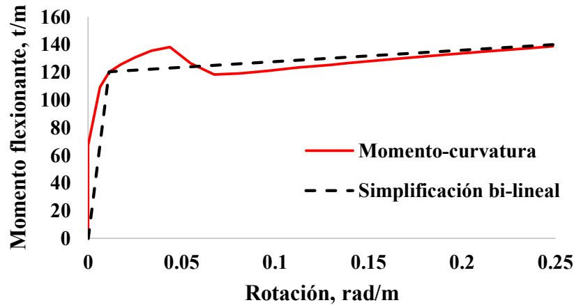
Fig. 3.3 Simplificación de la curva momento-curvatura a una curva bilineal
