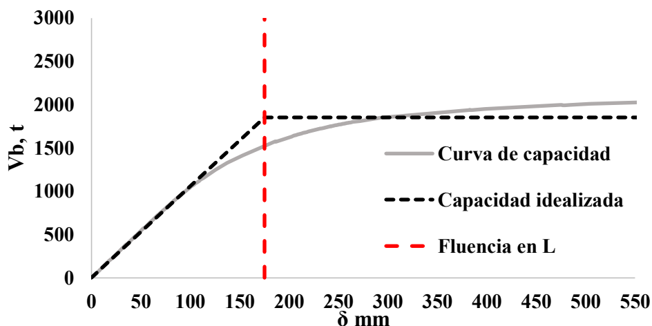
Fig. 4.3 Curva de capacidad en dirección L
