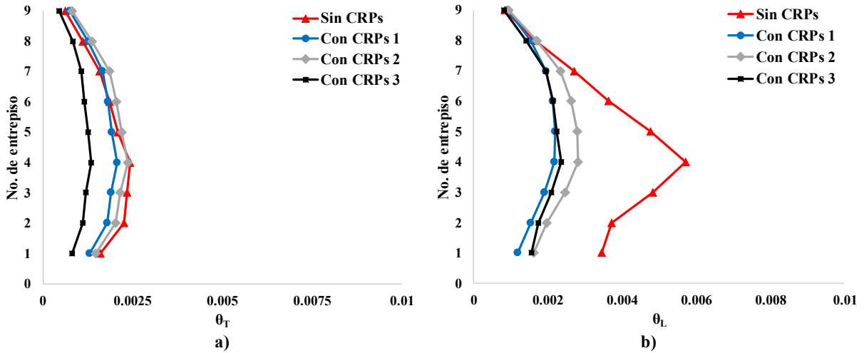
Fig. 4.13 Distorsiones de entrepiso para 0.05 g, registro SXPU8509
