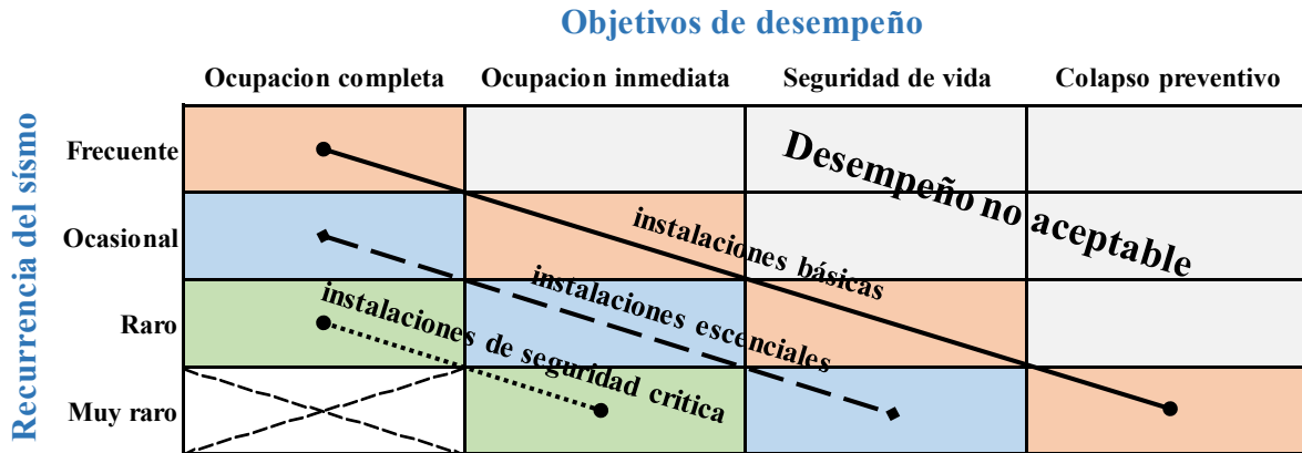
Fig. 2.3 Objetivos de desempeño sísmico (adaptada de Visión 2000, SEAOC, 1995)
