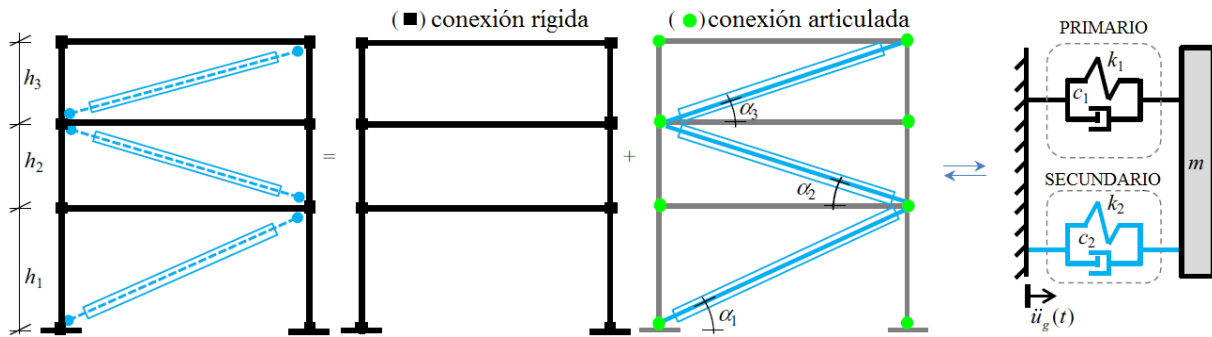
Fig. 2.2 Estructura de MGDL equipada con CRPs representado por un oscilador dual equivalente de 1GDL (Guerrero et al., 2016)
