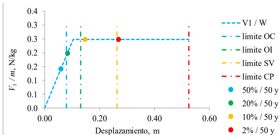
Fig. 4.4 Demanda de desplazamientos del sistema con 1GDL en T
