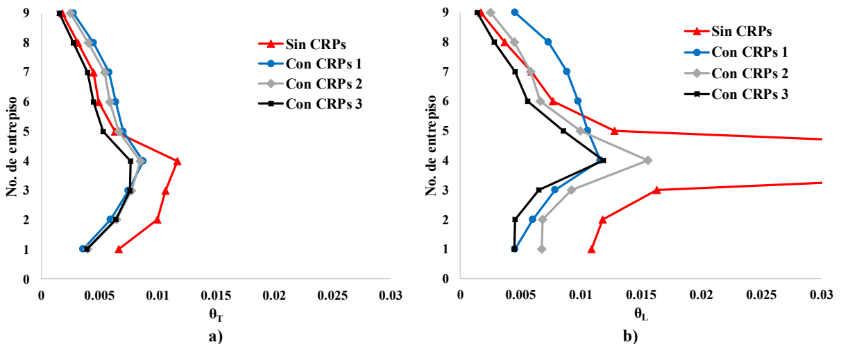
Fig. 4.15 Distorsiones de entrepiso para 0.2 g, registro SXPU8509
