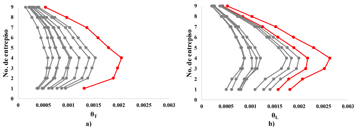
Fig. 3.7 Distorsiones con intensidad de 0.025 g
