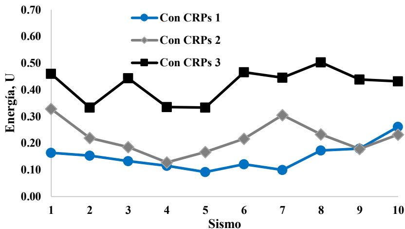
Fig. 4.21 Energía disipada para una intensidad de 0.2g: CRPs
