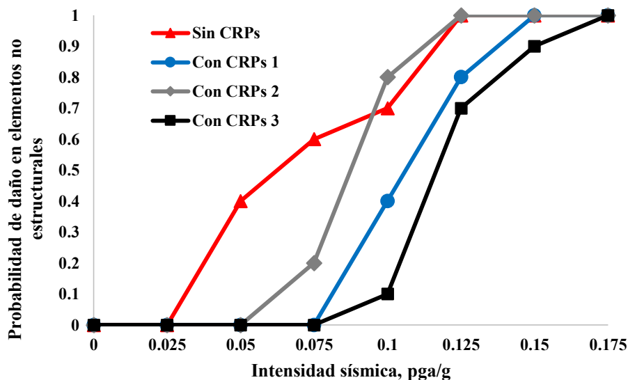
Fig. 4.24 Curva de probabilidad de daño a elementos no estructurales
