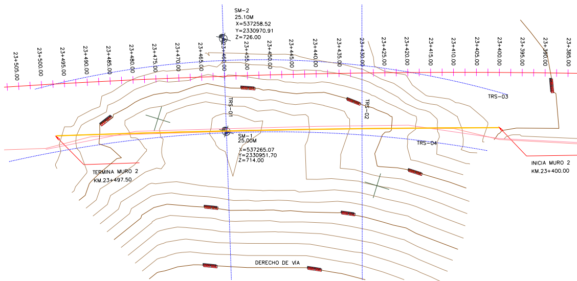
Figura 18. Ubicación de los tendidos de refracción sísmica (TRS)
