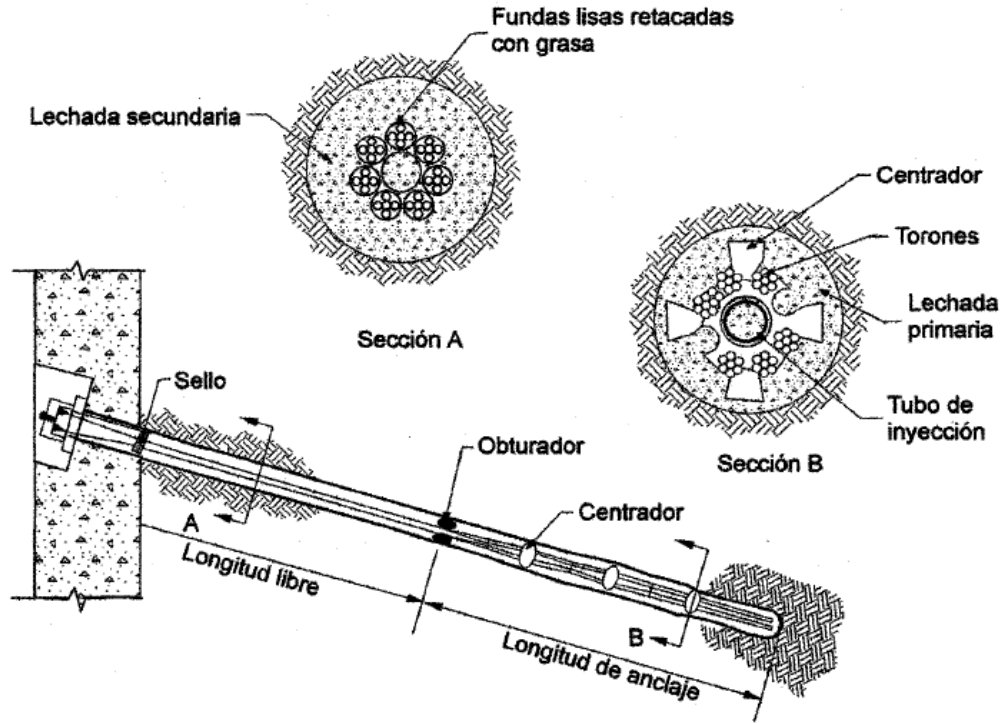
Figura 8. Elementos de protección simple en un ancla. Fuente Ovando y Olgúin (2002).
