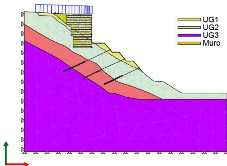
Figura 26. Modelo de elemento finito del talud, condiciones de proyecto.
