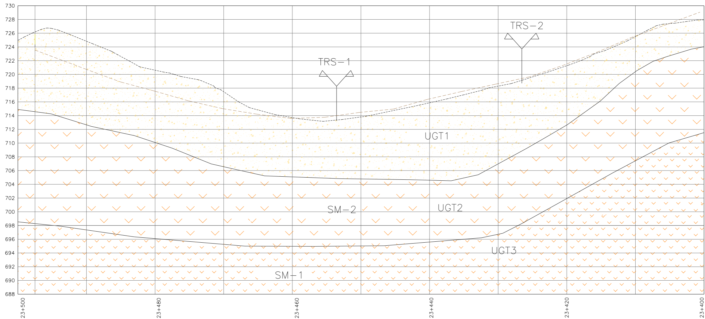
Ubicación de los sondeos mixtos (SM) y los tendidos de refracción sísmica longitudinales (TRS)
