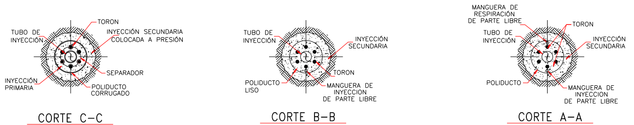
Figura 25. Cortes transversales de las secciones del ancla.
