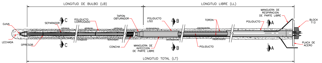
Figura 24. Esquema del ancla a tensión propuesta.
