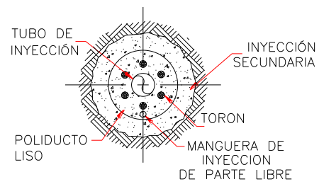
CORTE B-B
