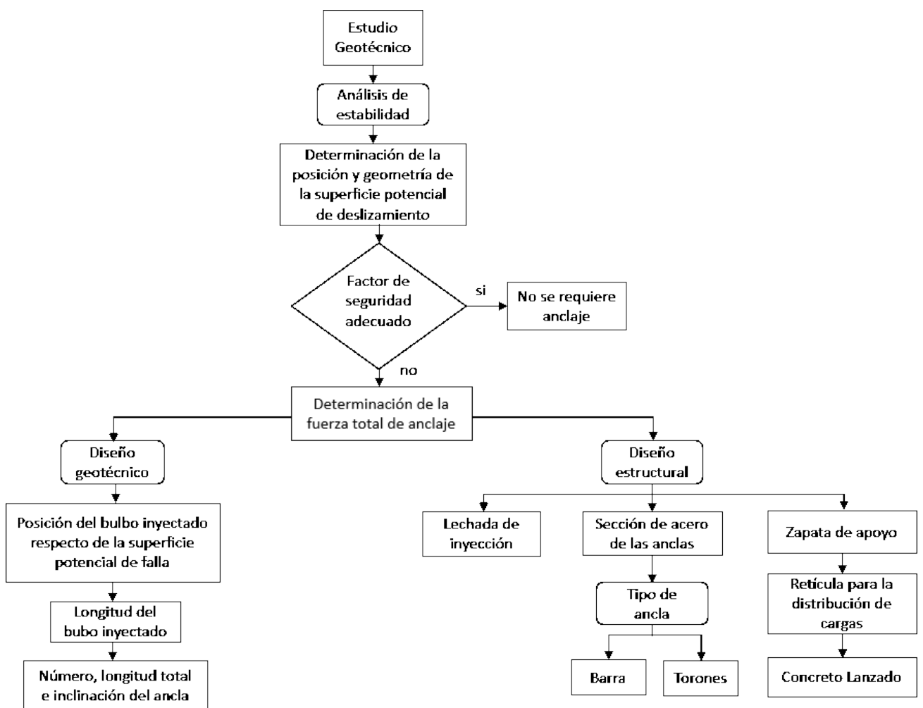
Figura 5. Secuencia de análisis y diseño para un sistema de anclaje. Fuente Ovando y Olguín (2002).
