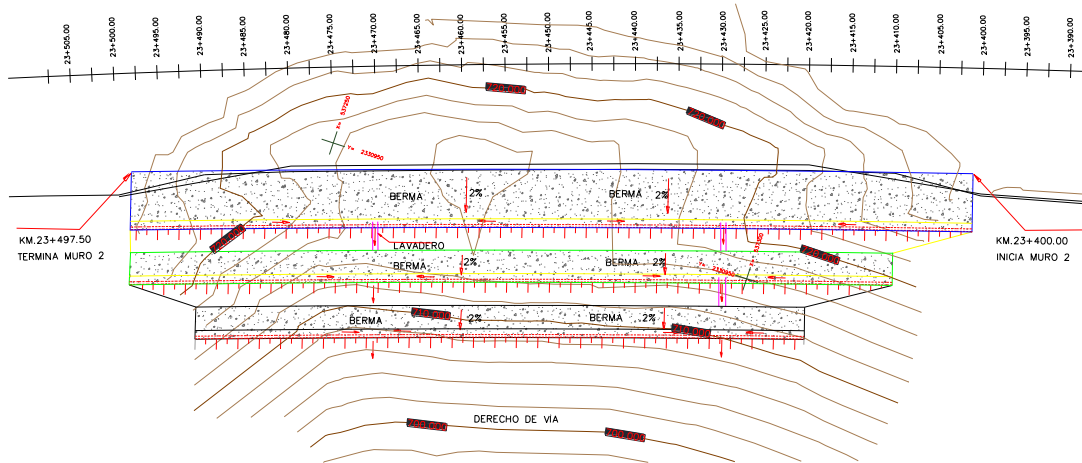
Figura 29. Topografía del sitio de proyecto, ubicación de bermas.
