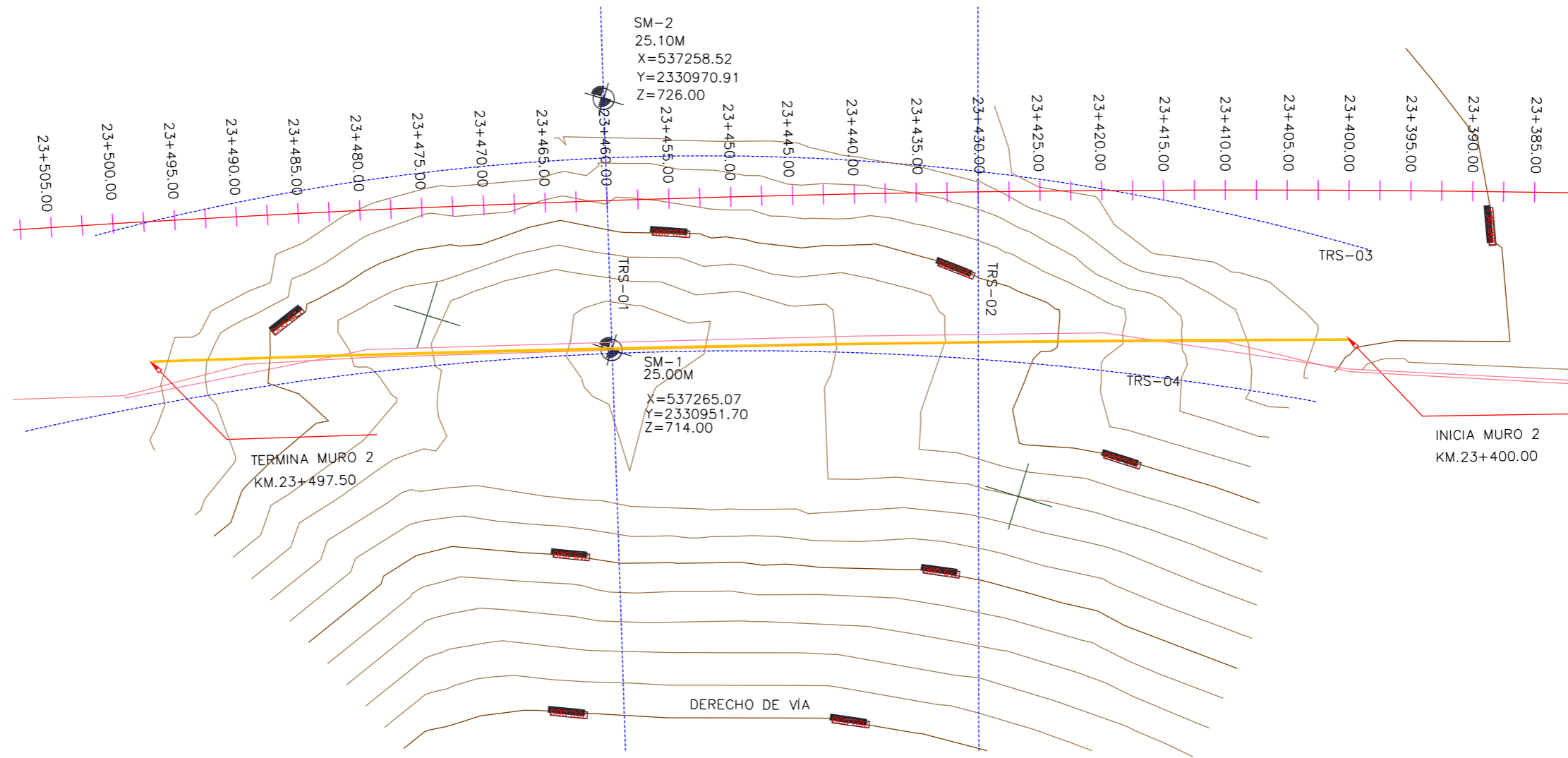
Ubicación de los sondeos mixtos (SM) y los tendidos de refracción sísmica (TRS)
