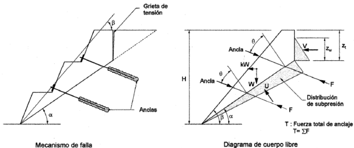
Figura 6. Geometría aplicada para el método de cuñas en un talud anclado. Fuente Ovando y Olguín (2002).
