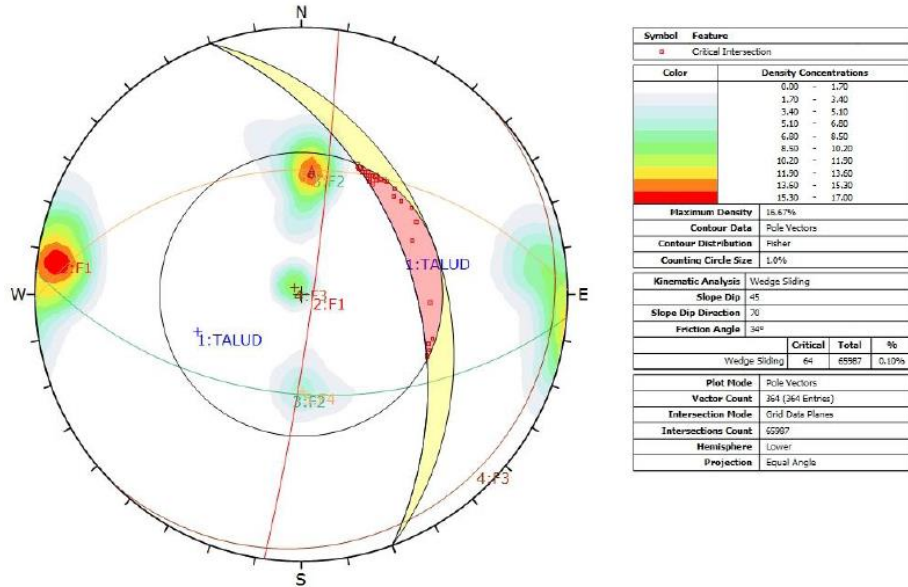
Figura 15. Análisis estereográfico de formación de cuñas sobre el muro.
