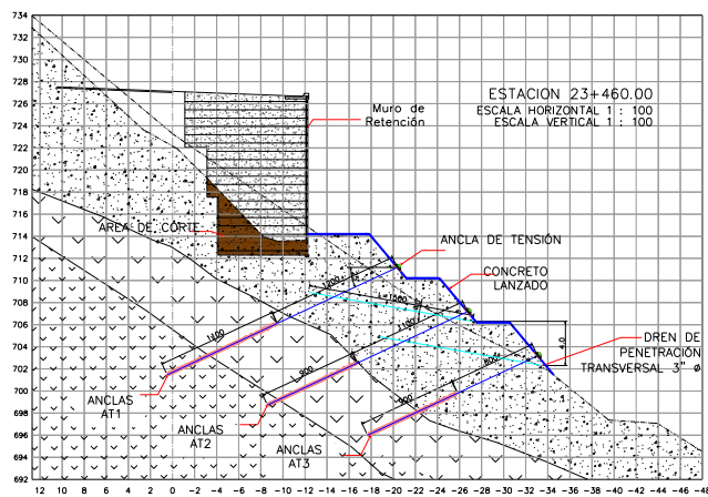
Figura 31. Distribución de las anclas y drenes, corte transversal.
