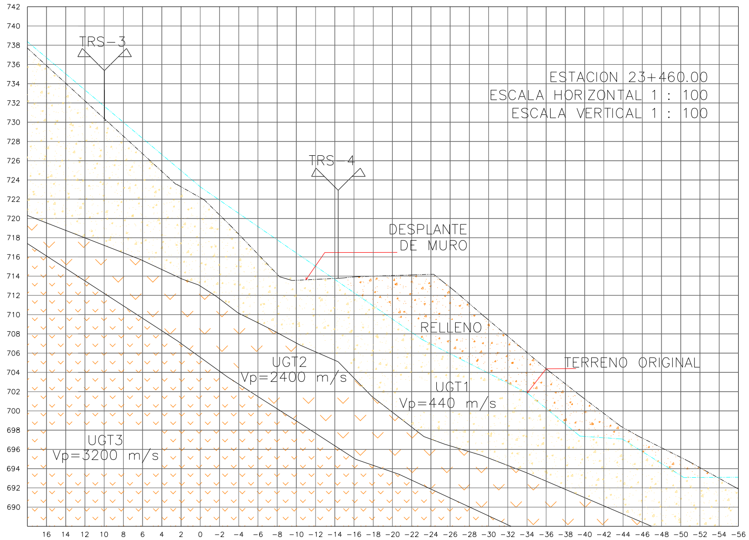
Ubicación de los tendidos de refracción sísmica transversales (TRS)
