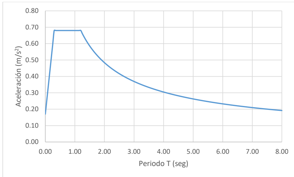
Figura 13. Espectro de diseño sísmico para estructuras tipo B
