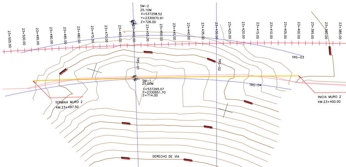
Figura 11. Ubicación de los sondeos y los tendidos de refracción sísmica, en planta.
