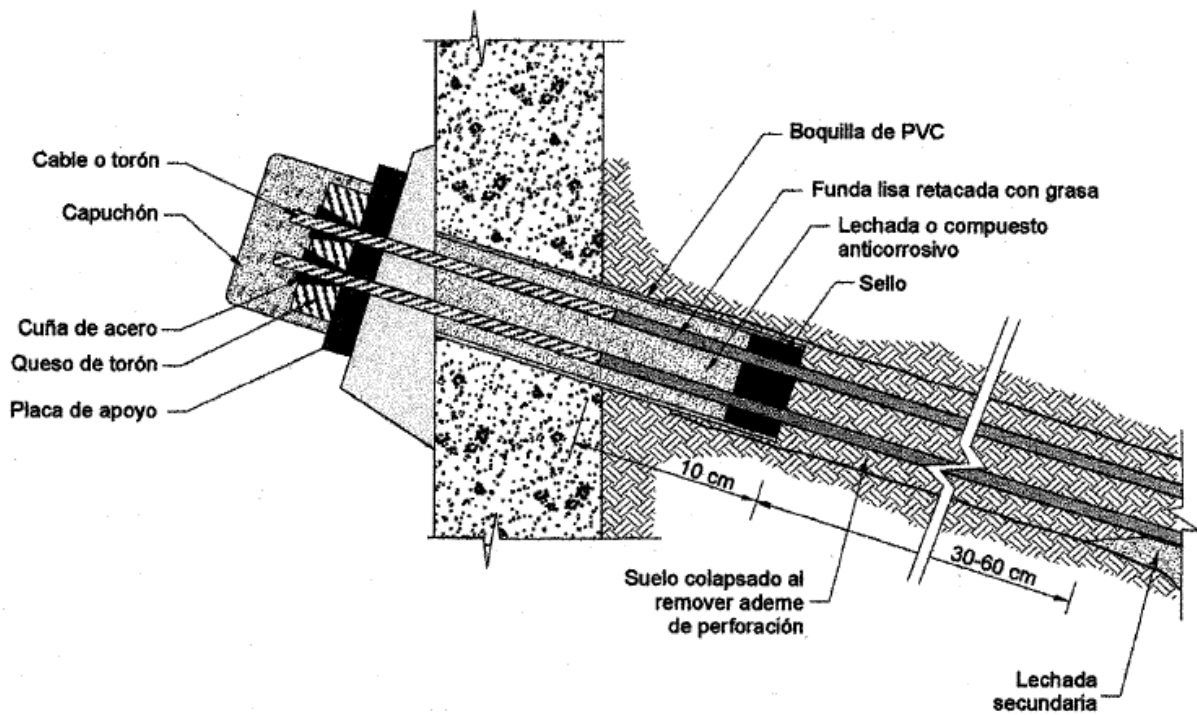
Figura 8. Elementos de protección simple en un ancla. Fuente Ovando y Olgúin (2002).
