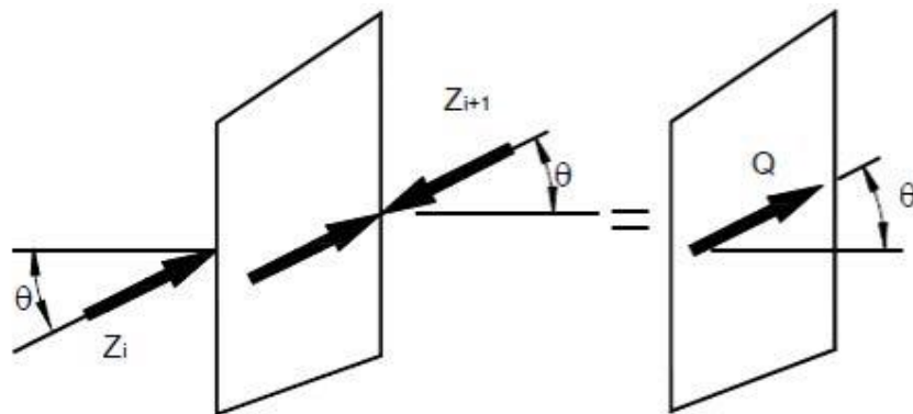
Figura 2. Paralelismo entre las fuerzas de las dovelas.
