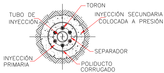
CORTE C-C
