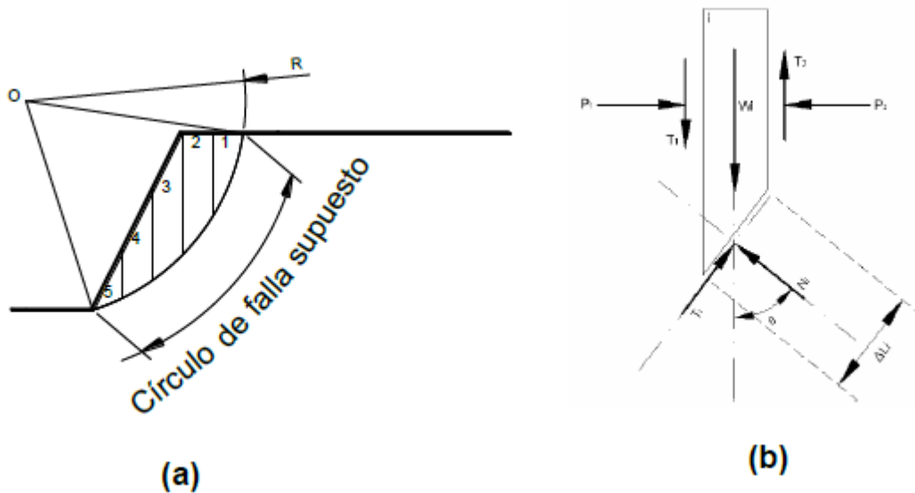
Figura 1. (a) Suposición de un círculo de falla. (b) equilibrio estático entre dovelas.
