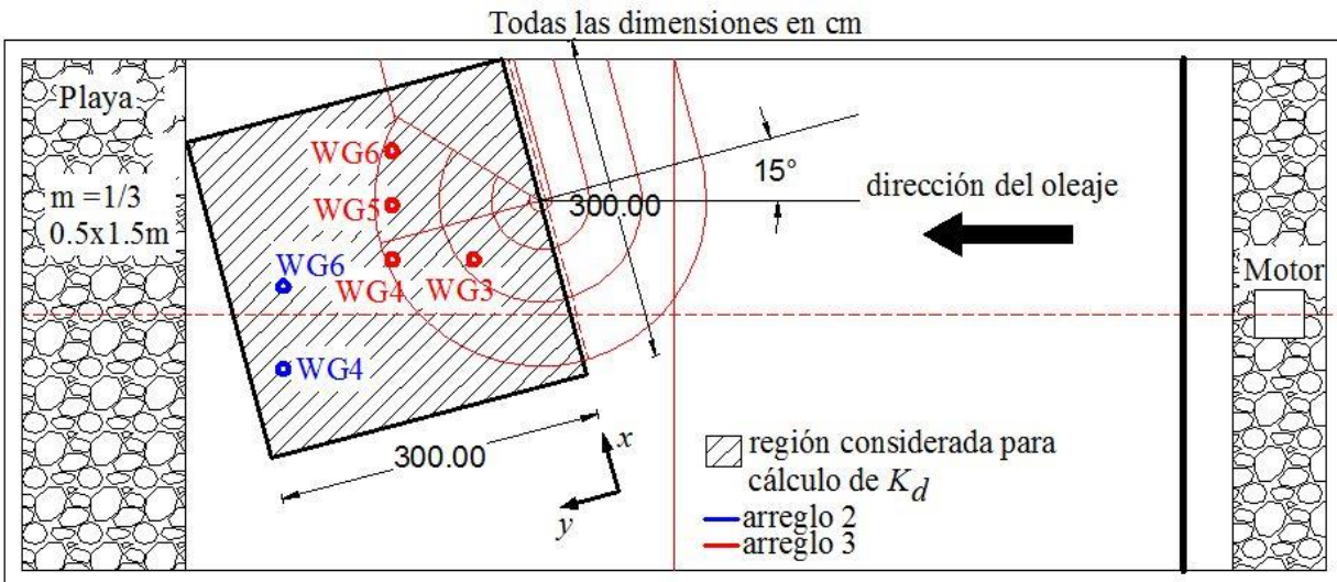
Figura 3.36 Definición de la zona de sombra para el caso de 15^\circ
