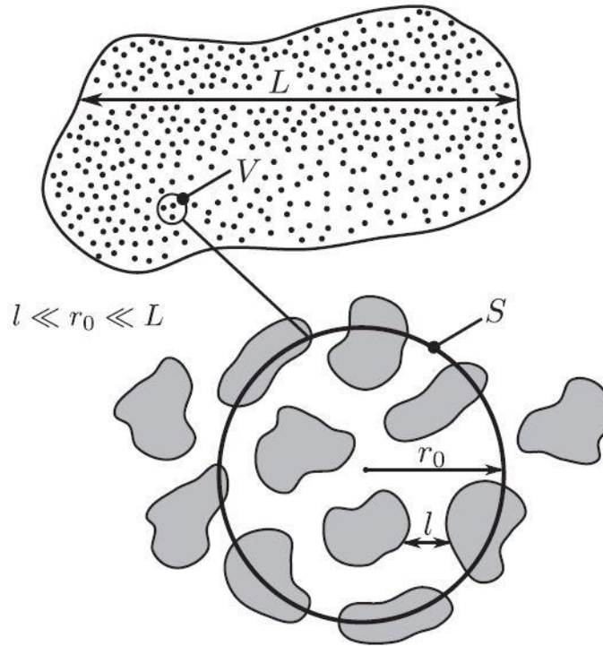
Figura 2.4 Definición del promedio en un volumen, áreas correspondientes y longitudes de escala (Imagen tomada de Jensen et al. (2014))
