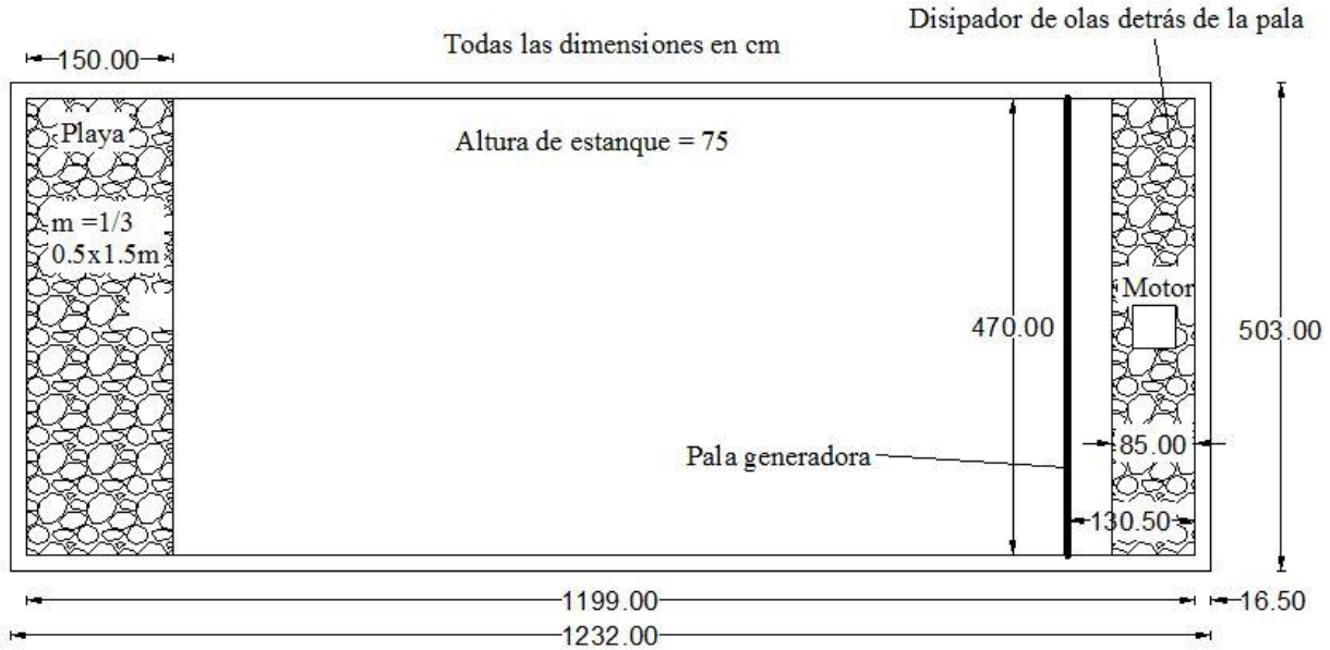
Figura 3.2 Dimensiones en planta del estanque de olas que posee el laboratorio de hidráulica de la Facultad de Ingeniería
