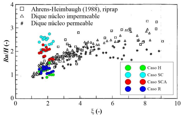
Figura 2.37 Comparación de los resultados numéricos del ascenso máximo con datos de Van der Meer y Stam (1992)
