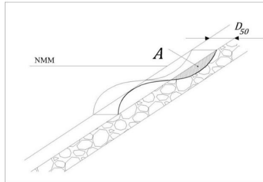
Figura 1.2 Definición de las variables para cuantificar el nivel de deformación de un DRPS, de acuerdo a Van der Meer (1988). En la figura NMM significa nivel medio del mar
