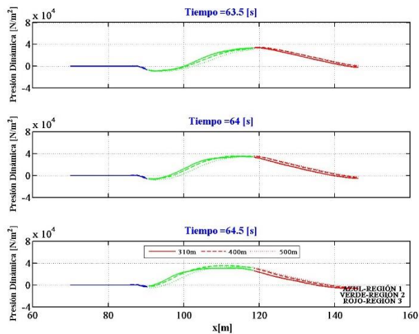
Figura 2.11 Comparación de la presión dinámica a lo largo del perfil en S para las tres longitudes propuestas
