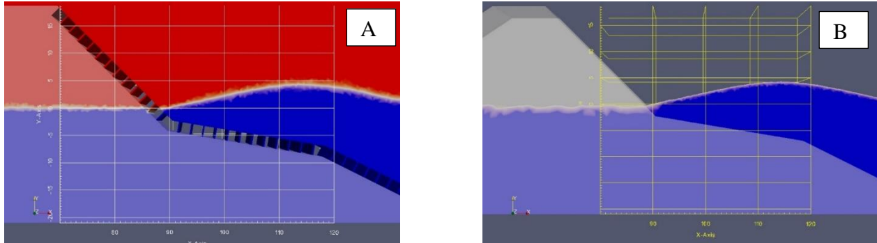
Figura 2.23 Contenido de agua ( \alpha_1 ). En el panel A el DRPS para cuando H = 7 m, T = 9 segundos, caso 2; en el panel B el DRPS cuando H = 7 m, T = 9 segundos, caso 1.
