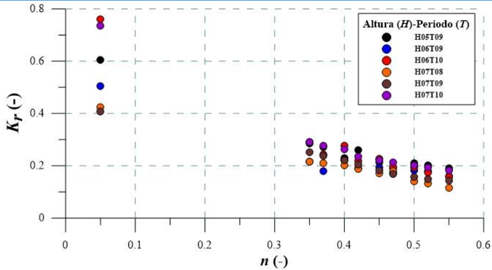
Figura 2.45 Resultados del coeficiente de reflexión K_r en función de la porosidad n
