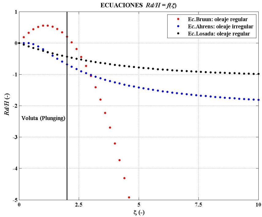
Figura 1.11 Comportamiento de las ecuaciones Rd/H = f(\xi)
