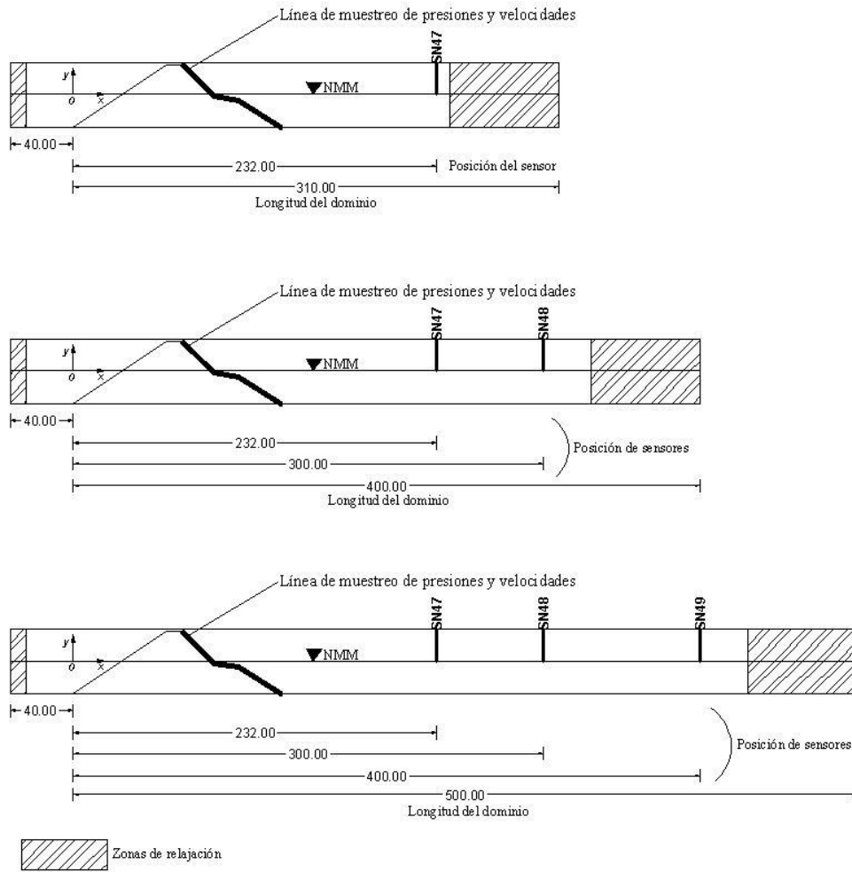
Figura 2.10 Longitudes de dominio propuestas y posición de sensores de nivel
