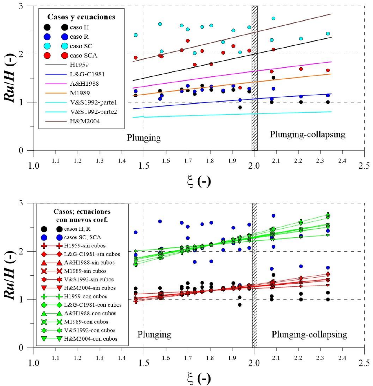
Figura 2.33 Comportamiento de 6 ecuaciones ajustadas a los resultados numéricos de Ru/H . En el panel superior, las ecuaciones sin los coeficientes c_f . En el panel inferior, las ecuaciones con los coeficientes c_f
