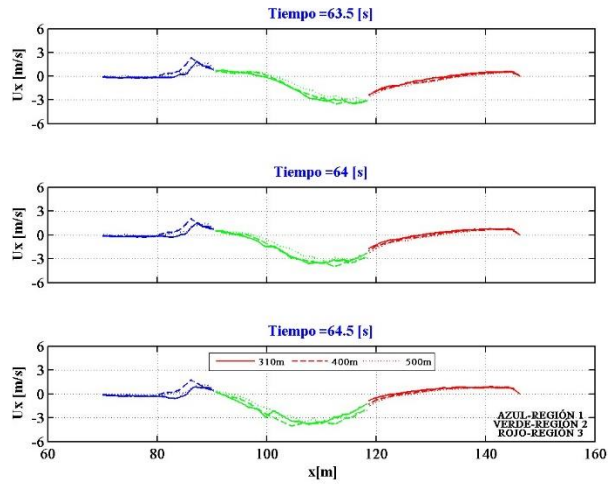
Figura 2.12 Comparación de la velocidad en dirección x a lo largo del perfil en S para las tres longitudes propuestas
