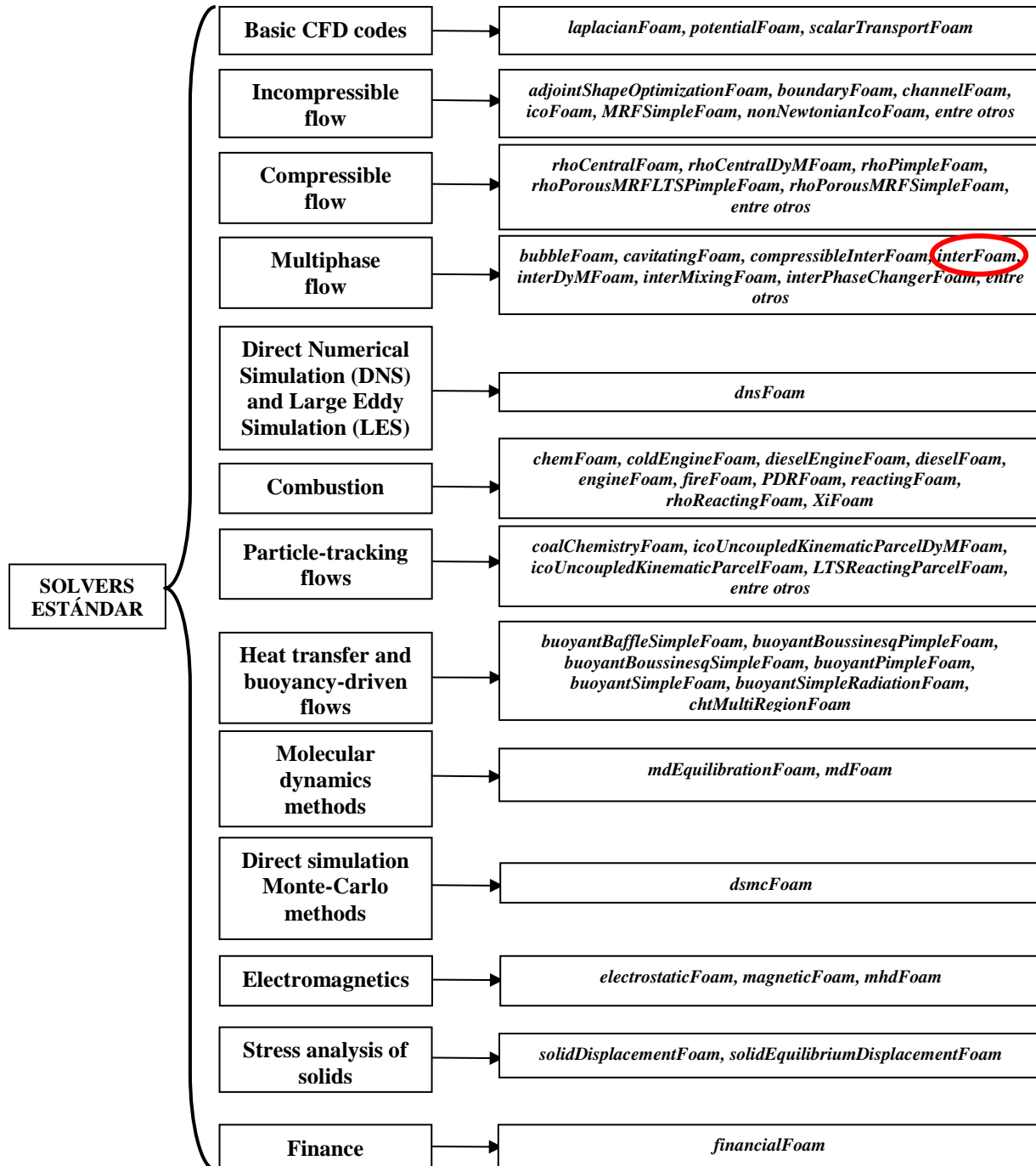
Figura 2.5 Solvers estándar integrados en la versión 2.2.2 de OpenFOAM
