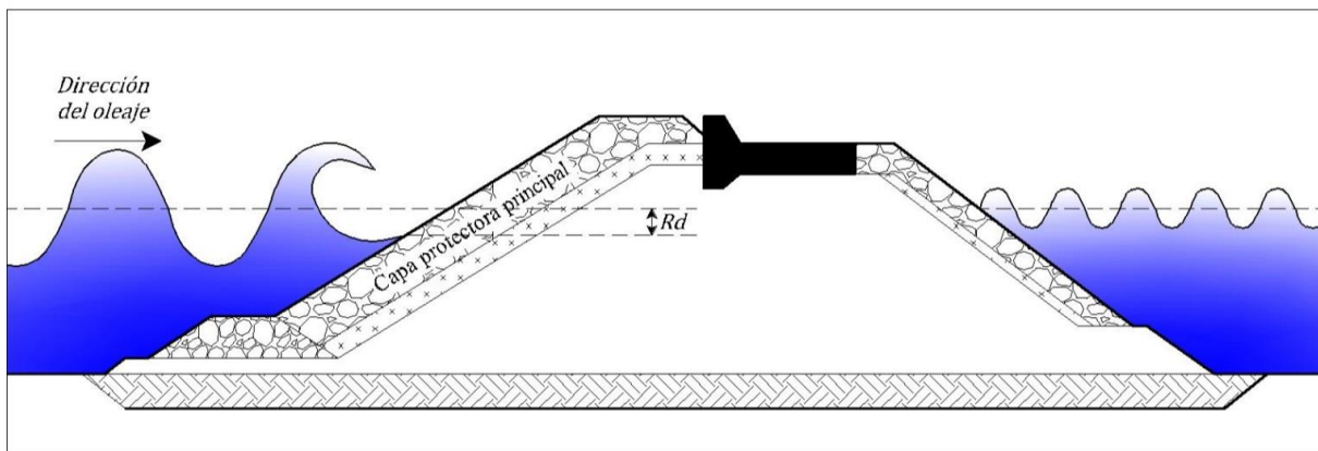
Figura 1.7 Definición del descenso máximo en un DRPS
