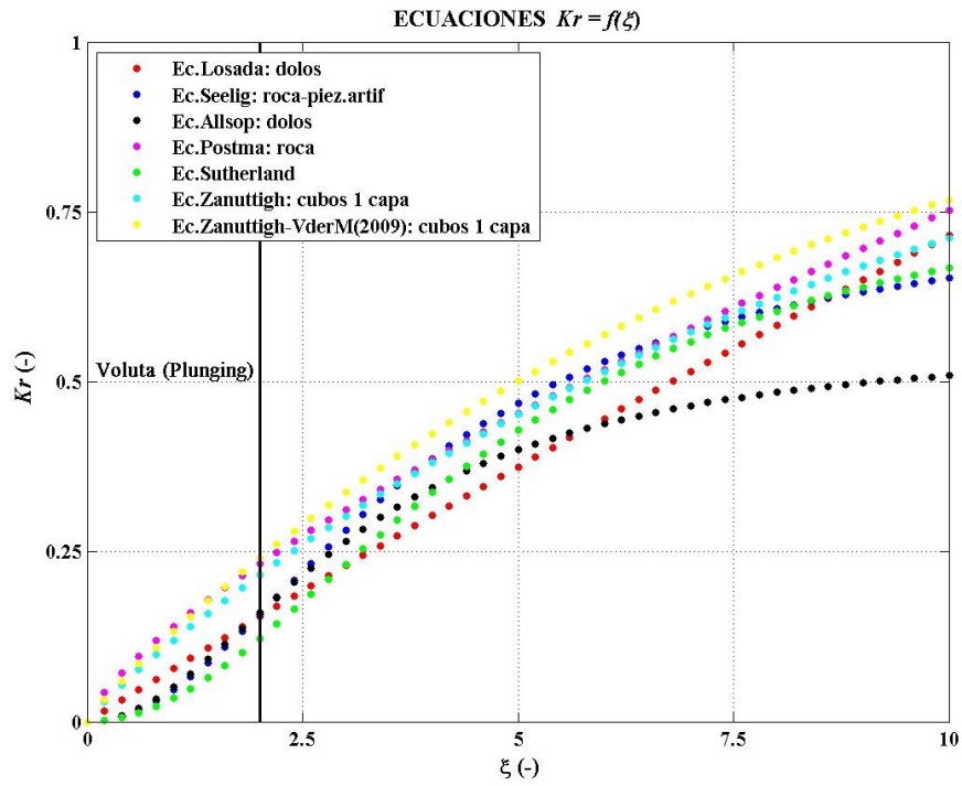
Figura 1.8 Comportamiento de las ecuaciones Kr = f(\xi)
