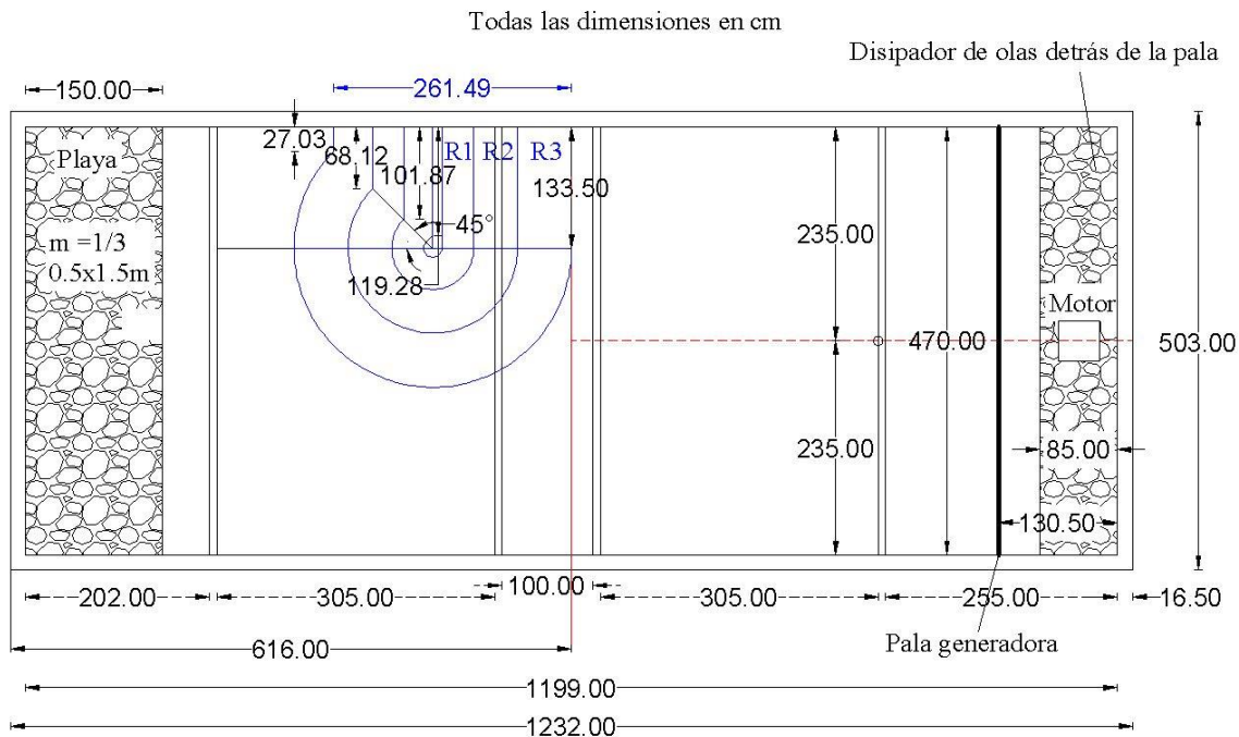
Figura 3.3 Distancias transversales del morro, considerando como eje transversal principal la línea roja sólida localizada a los 6.16 m
