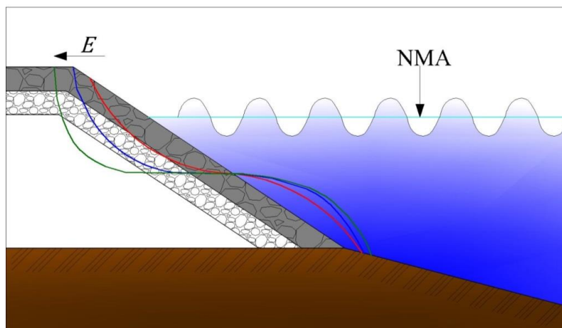
Figura 1.1 Progreso de la erosión (Burcharth y Frigaard, 1987). En la figura NMA y E significa Nivel Medio del Agua y Erosión, respectivamente
