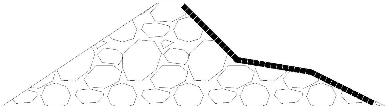
Figura 2.17 DRPS en S con cubos de 2 m de lado a lo largo del perfil en S
