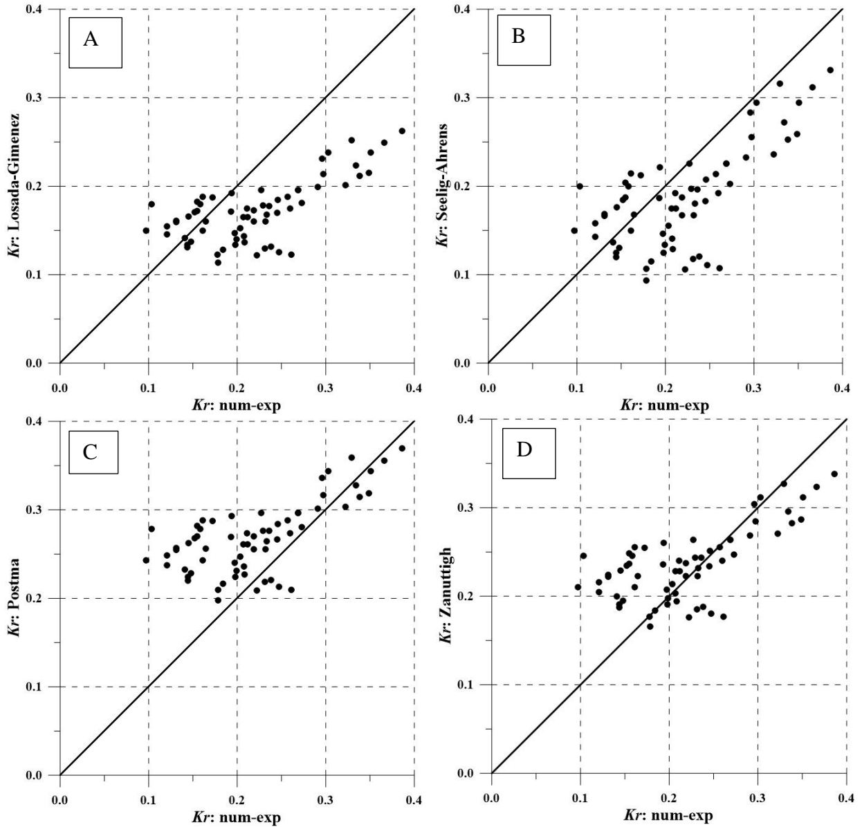
Figura 2.44 Comparación entre los resultados numérico (caso H)-experimentales (Quiñones) con los valores dados por las ecuaciones mostradas en la Tabla 2.16
