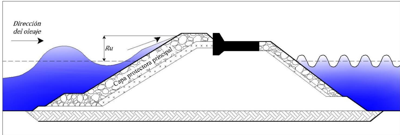
Figura 1.6 Definición del ascenso máximo ( Ru ) en un dique rompeolas
