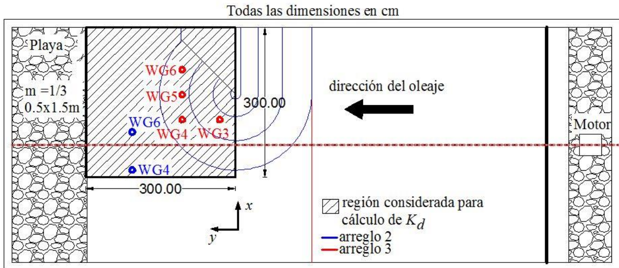
Figura 3.35 Definición de la zona de sombra para el caso de 0^\circ
