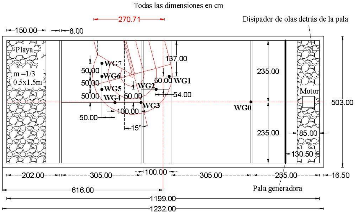
Figura 3.22 Tercer arreglo de sensores: 15 grados
