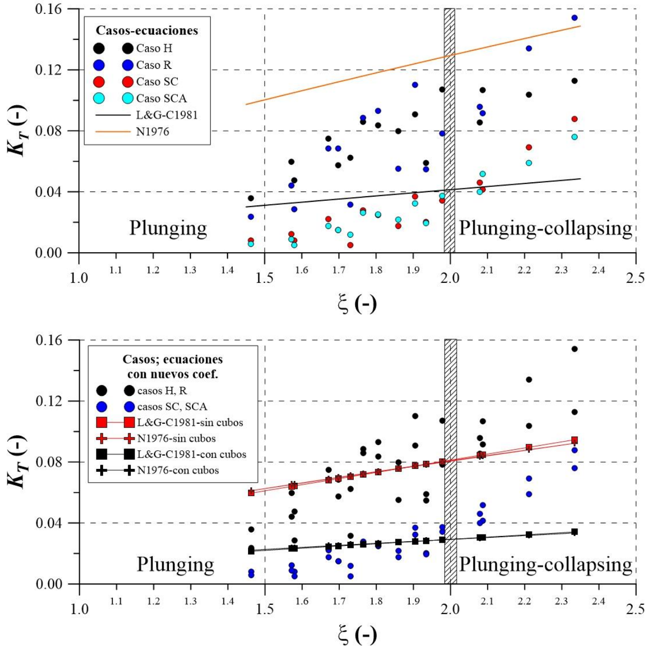
Figura 2.31 Comportamiento de 2 ecuaciones ajustadas a los resultados numéricos de K_T . En el panel superior, las ecuaciones sin los coeficientes cf . En el panel inferior, las ecuaciones con los coeficientes cf
