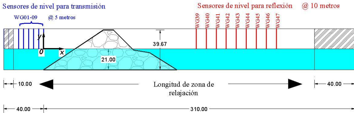
Figura 2.20 Posición de todos los sensores de nivel, para evaluar los coeficientes de reflexión y transmisión
