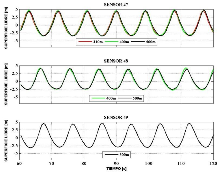
Figura 2.13 Comparación de los resultados de tres sensores comunes a las tres longitudes de cálculo propuestas
