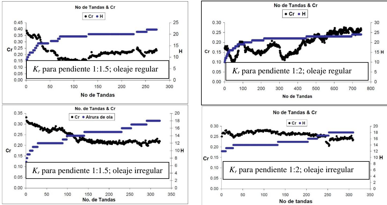
Figura 2.40 Evaluación experimental del coeficiente de reflexión realizado por Quiñones (2006) (Imágenes modificadas)
