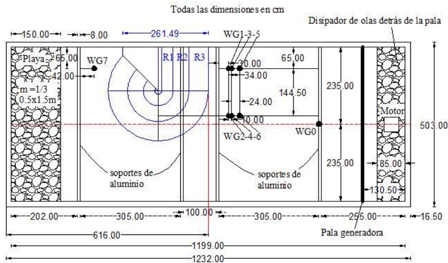
Figura 3.15 Primer arreglo de sensores: 0 grados
