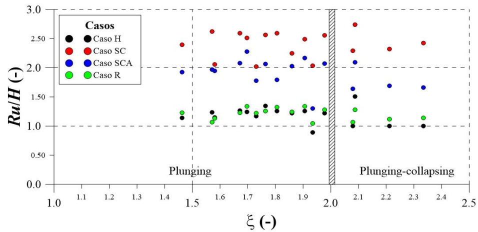
Figura 2.28 Resultados del ascenso máximo adimensional en función del número de Iribarren
