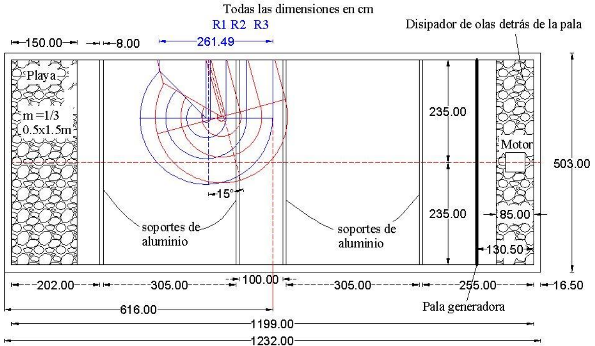
Figura 3.18 Esquema en planta del giro del morro. En color rojo, la estructura girada. En color azul, la estructura antes del giro
