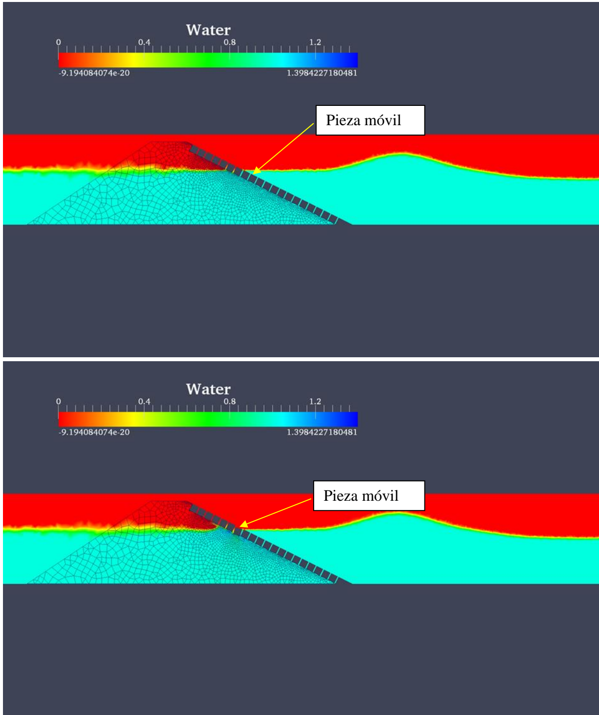
Figura 6.9 Movimiento inicial de una pieza utilizando el concepto de malla dinámica
