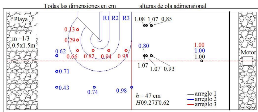
Figura 3.32 Resultados del estado de mar H = 9.27 cm, T = 0.62 s, h = 47 cm, giro = 0^\circ
