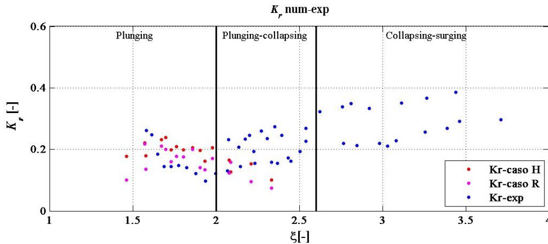
Figura 2.43 Comparación únicamente de los resultados numéricos de los casos H y R con los resultados experimentales de Quiñones
