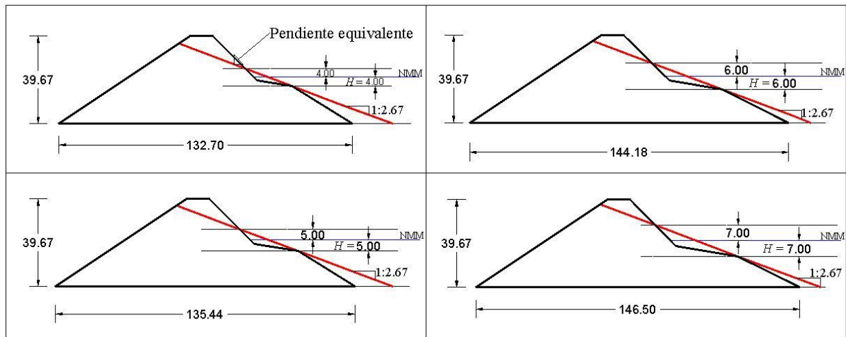
Figura 2.25 Definición de pendiente equivalente
