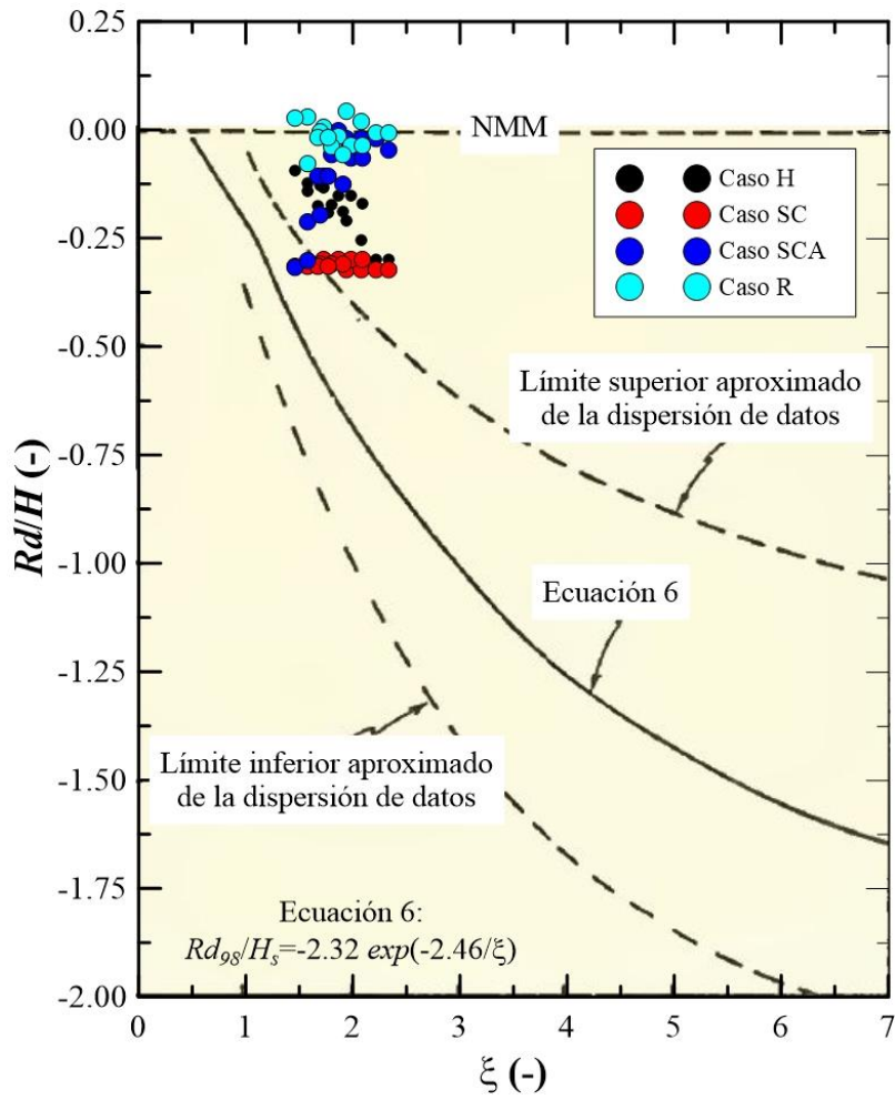
Figura 2.38 Comparación de los resultados numéricos del descenso máximo con datos de Ahrens (1981)
