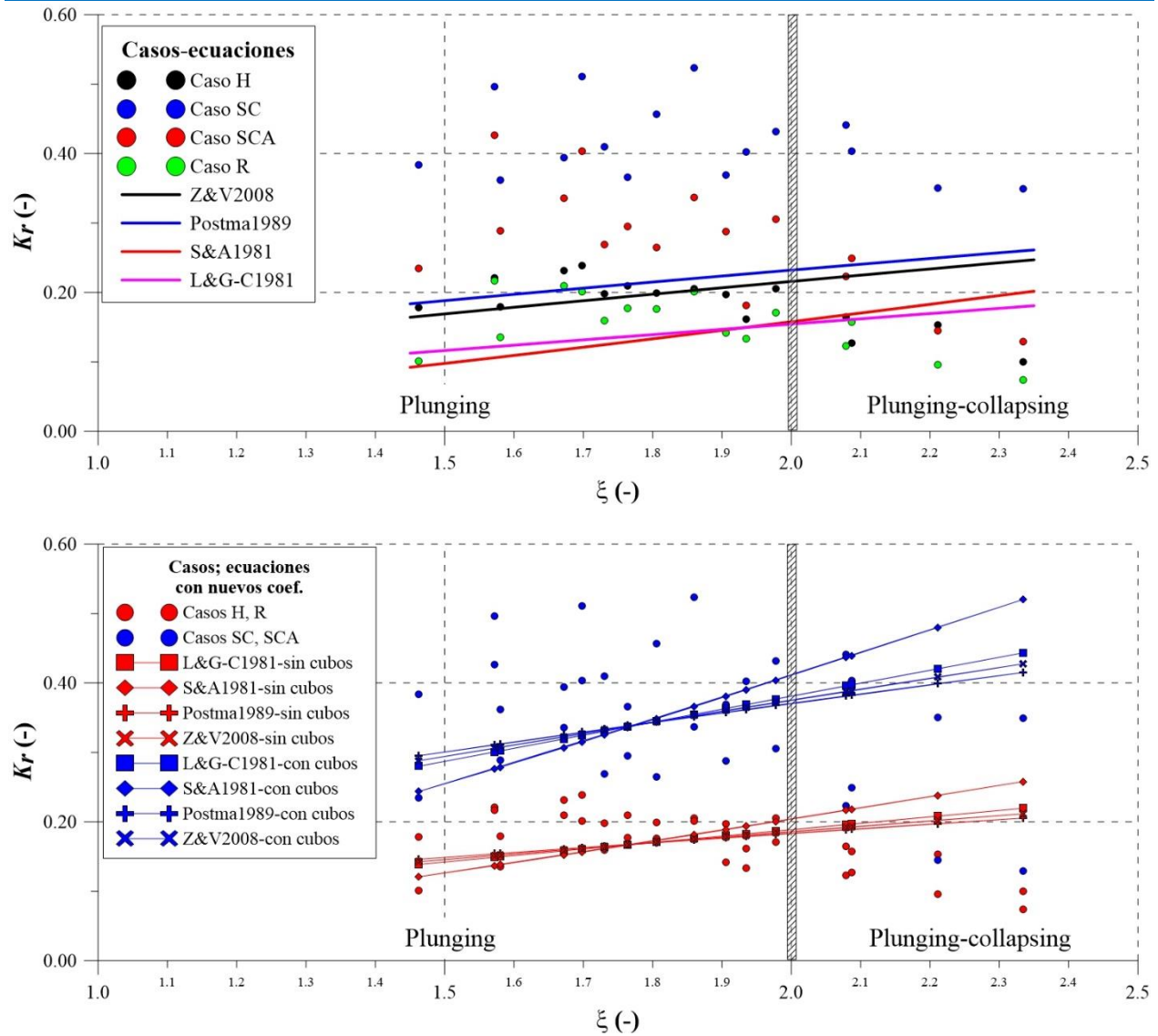
Figura 2.30 Comportamiento de 4 ecuaciones ajustadas a los resultados numéricos de K_r . En el panel superior, las ecuaciones sin los coeficientes cf . En el panel inferior, las ecuaciones con los coeficientes cf
