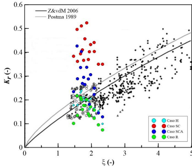
Figura 2.35 Comparación de los resultados numéricos del K_r con datos de Zanuttigh y Van der Meer (2008)
