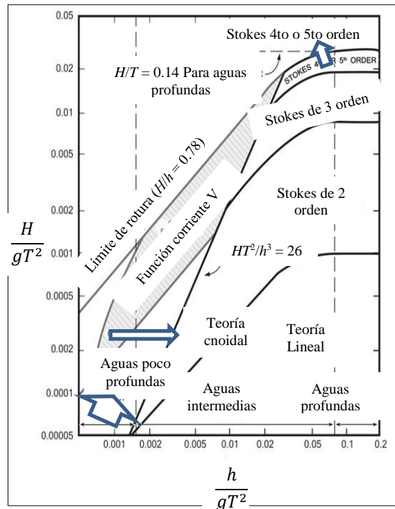
Figura 2.9 Diferentes teorías analíticas de oleaje y su rango de validez (Imagen modifica, tomada de la web)
