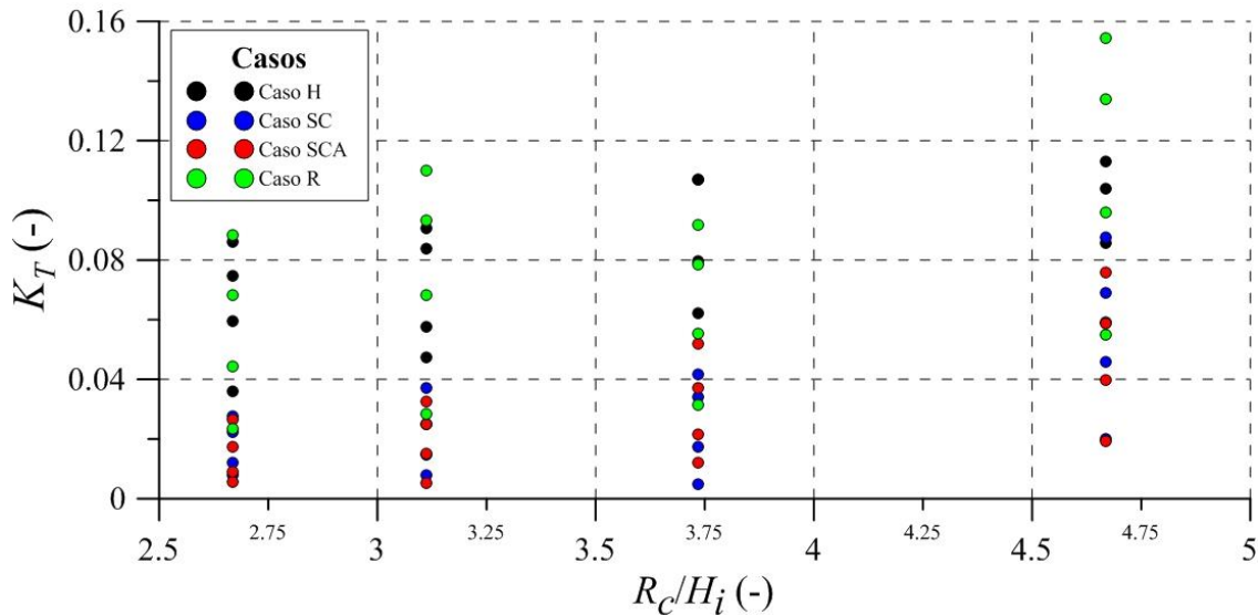
Figura 2.22 Coeficientes de transmisión medidos con ayuda del sensor #4 localizado a x = -25 m
