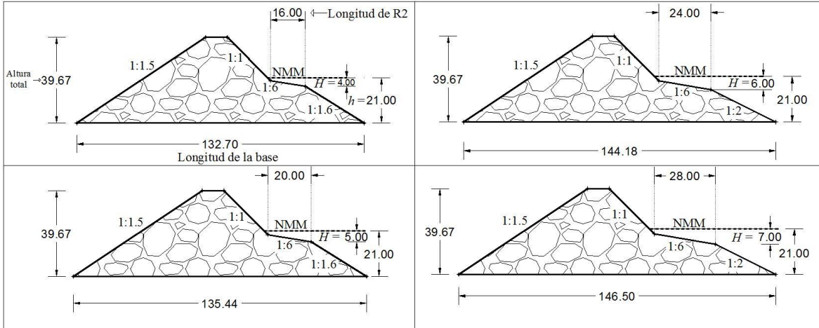
Figura 2.8 Secciones transversales teóricas propuestas para su análisis numérico
