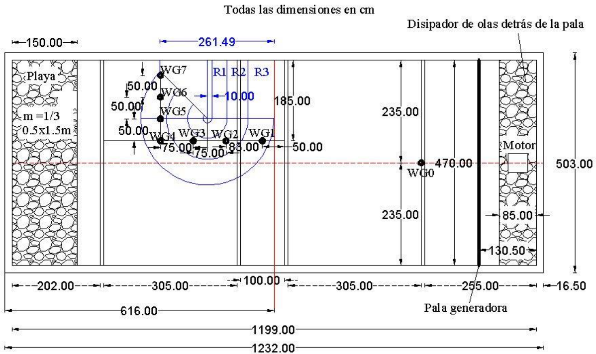
Figura 3.17 Tercer arreglo de sensores: 0 grados
