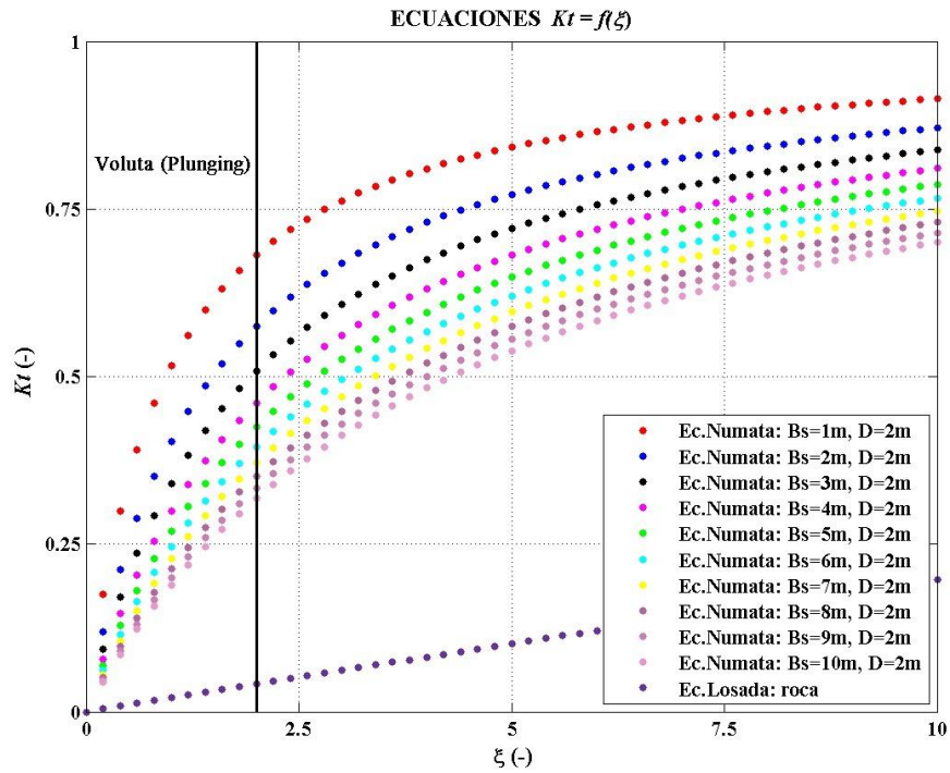
Figura 1.9 Comportamiento de las ecuaciones Kt = f(\xi)
