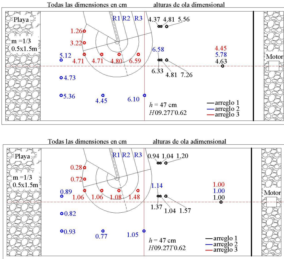
Figura 3.33 Resultados del estado de mar H = 9.27 cm, T = 0.62 s, h = 47 cm, giro = 15^\circ
