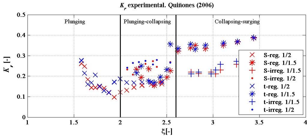
Figura 2.41 Coeficiente de reflexión experimental en función del número de Iribarren. En la leyenda, S se refiere al perfil en S, mientras que t se refiere al talud inicial del DRPS
