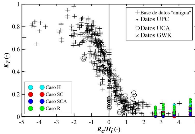
Figura 2.36 Comparación de los resultados numéricos del K_T con datos de Van der Meer et al. (2005)
