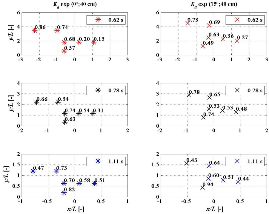
Figura 3.37 Valores promedio-experimentales de K_d considerando la profundidad de 40 cm
