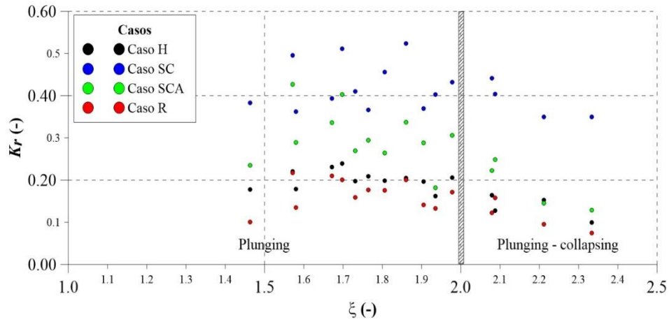
Figura 2.26 Resultados del coeficiente de reflexión en función del número de Iribarren
