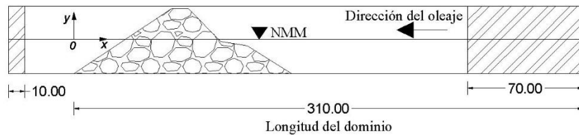
Figura 2.14 Longitud total final de cálculo. Además, se muestran en las regiones achuradas la longitud de las zonas de relajación
