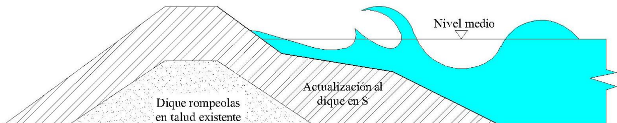
Figura 1.5 Actualización de un DRPS en talud a un DRPS-S (Del Valle et al. (2015))
