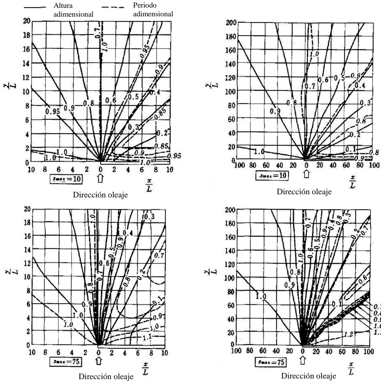
Figura 3.34 Diagramas de difracción de un rompeolas semi-infinito para oleaje normal e irregular (Imagen modificada de Goda, 2000)
