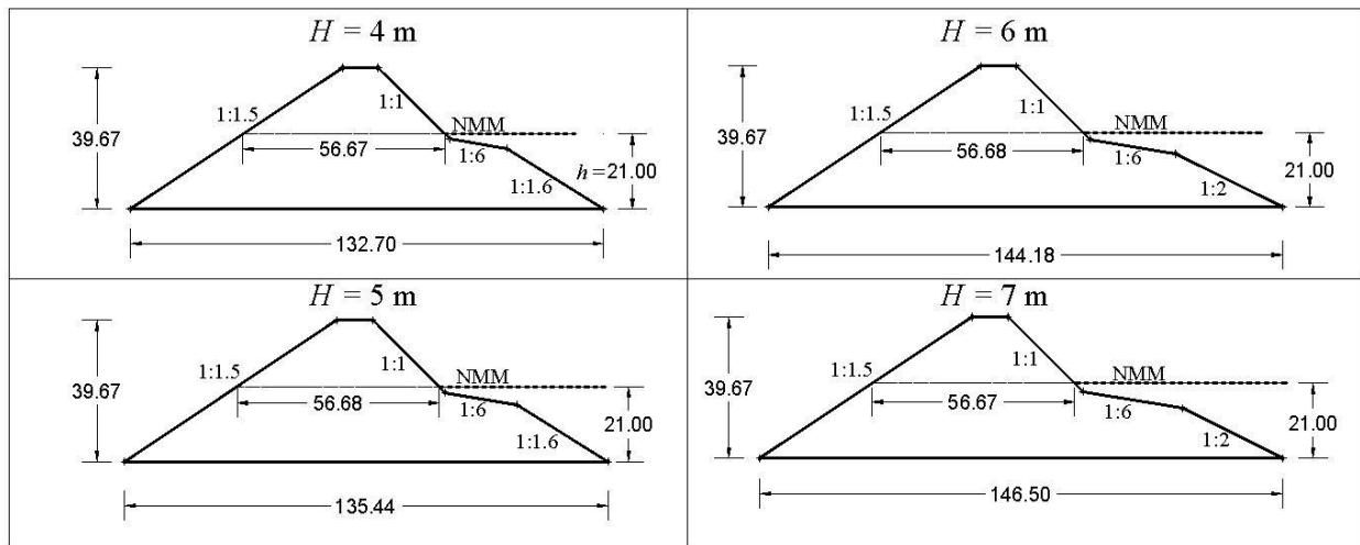
Figura 2.32 Valor del ancho del dique a la altura del NMA
