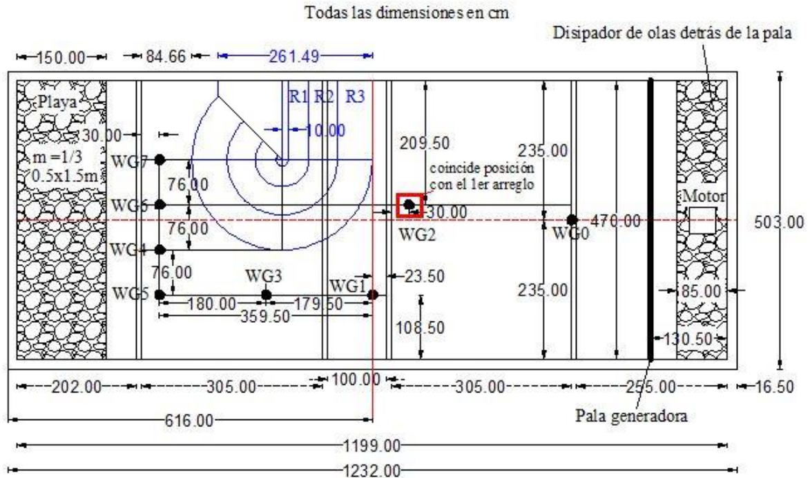
Figura 3.16 Segundo arreglo de sensores: 0 grados
