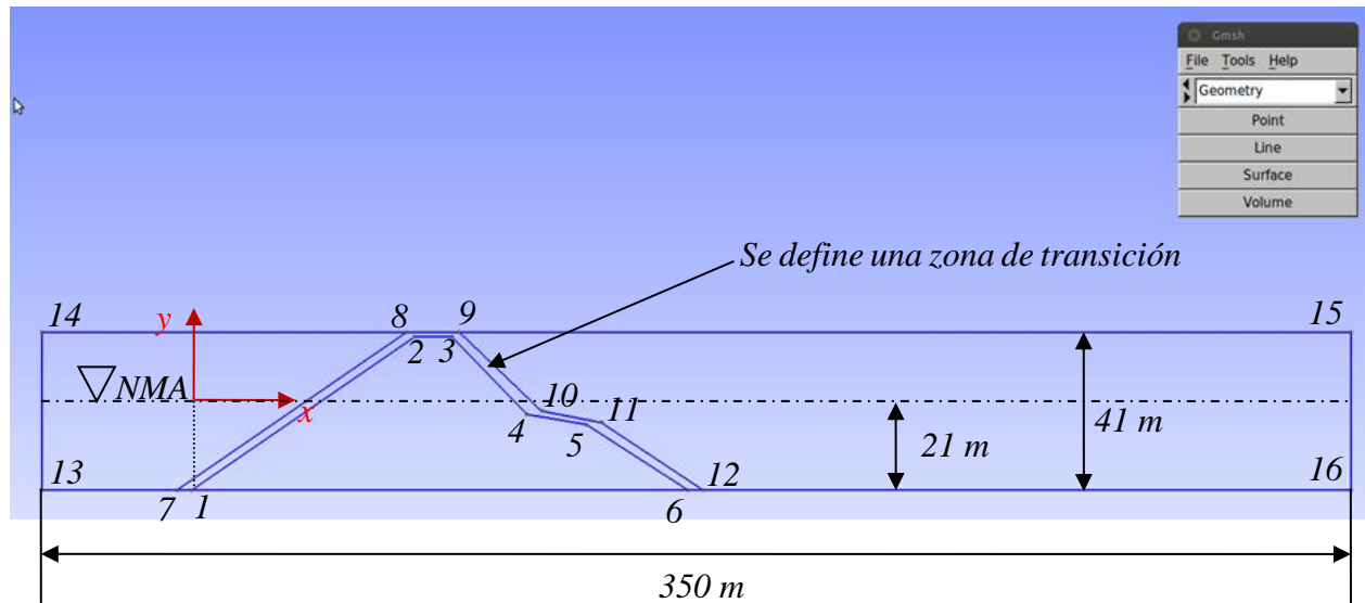
Figura 2.3 Características del dominio y de la geometría de la sección transversal de un DRPS-S
