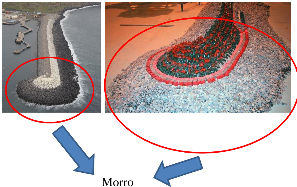
Figura 3.1 En el panel izquierdo, el morro en prototipo; en el panel derecho, un modelo físico de laboratorio
