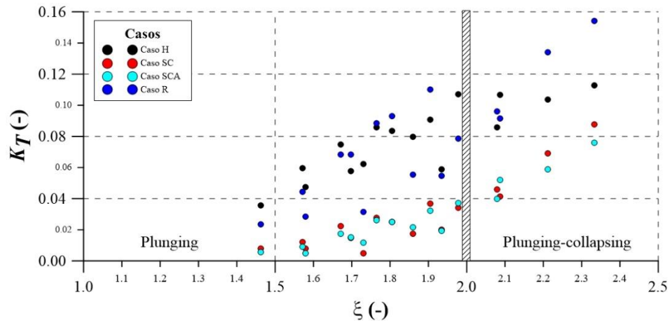
Figura 2.27 Resultados del coeficiente de transmisión en función del número de Iribarren
