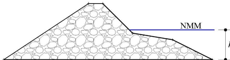
Figura 2.15 DRPS en S homogéneo
