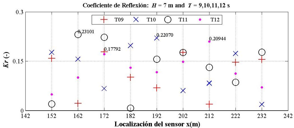
Figura 2.21 Máximos valores del K_r . Estos resultados pertenecen al caso homogéneo
