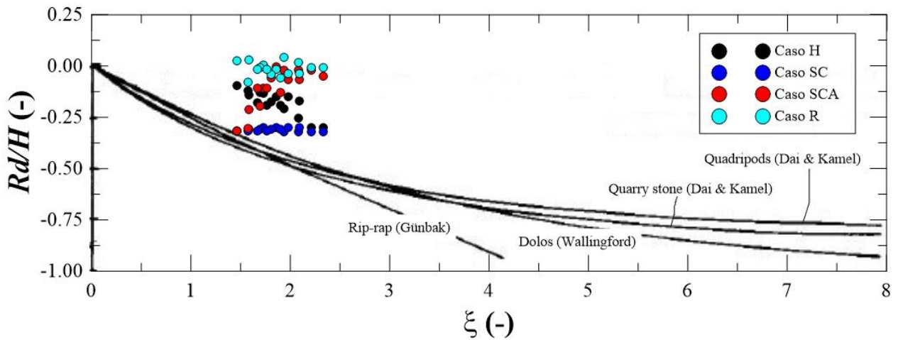
Figura 2.39 Comparación de los resultados numéricos del descenso máximo con datos de Losada y Gimenez-Curto (1981)
