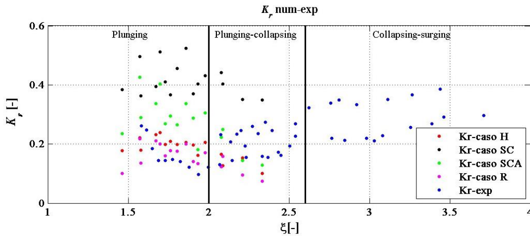
Figura 2.42 Comparación de los resultados numéricos del trabajo de Quiñones (2006) con los obtenidos en los 4 casos teóricos analizados en esta tesis
