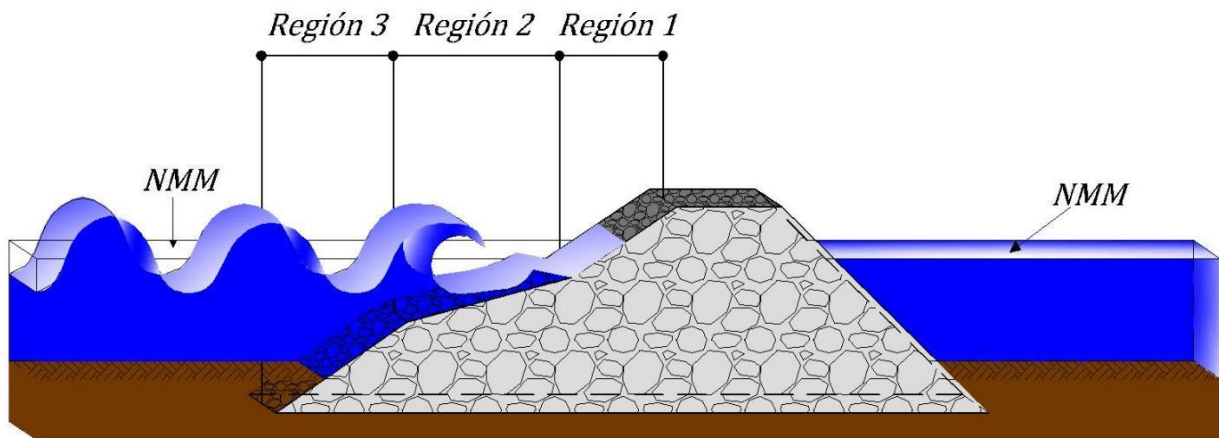
Figura 1.4 Definición de regiones en un DRPS-S. En la figura NMM significa nivel medio del mar
