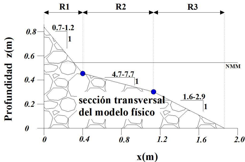
Figura 2.7 Intervalos de valores propuestos por Mendoza et al. (2010) para las tres regiones definidas en un DRPS-S
