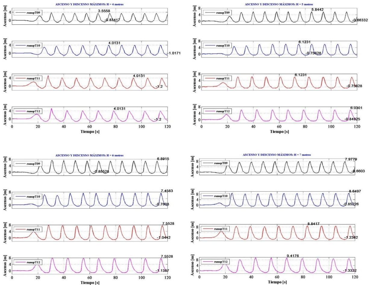
Figura 2.24 Comportamiento del ascenso y descenso del agua sobre el perfil en S del caso H
