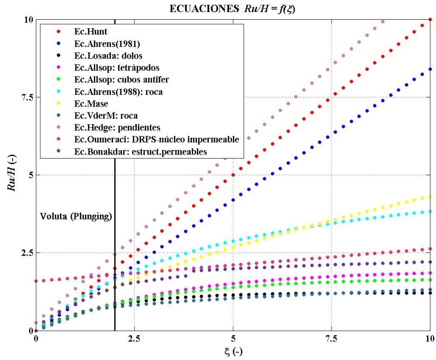
Figura 1.10 Comportamiento de las ecuaciones Ru/H = f(\xi)
