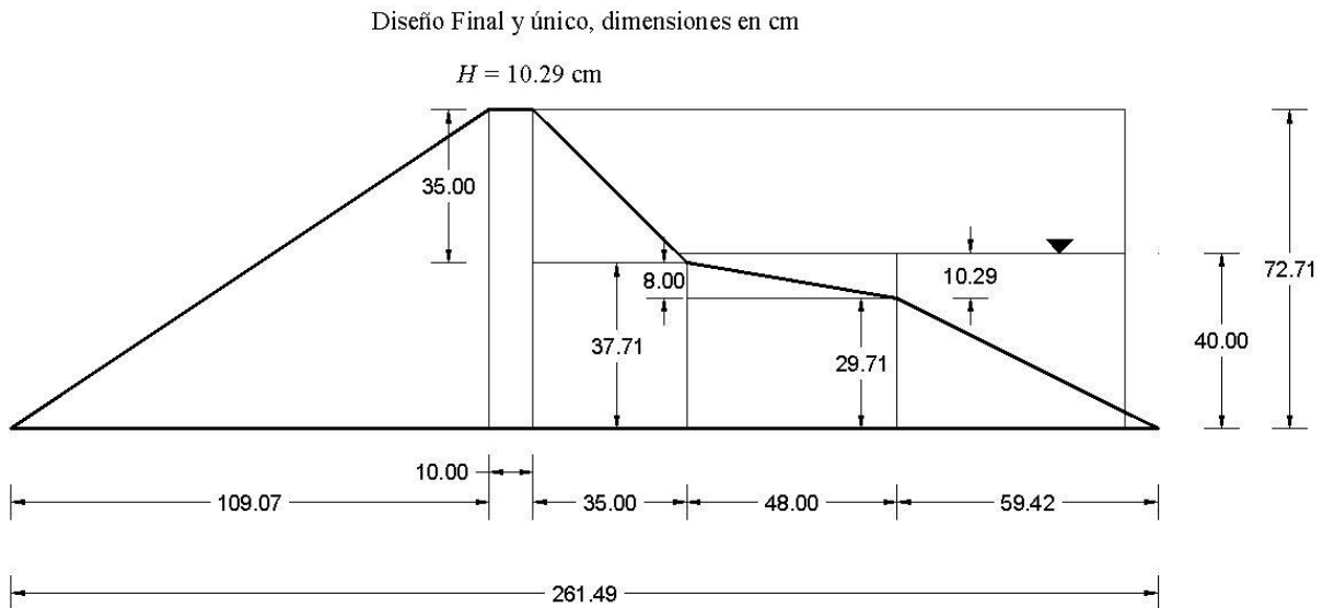
Figura 3.5 Dimensiones de la sección transversal del morro
