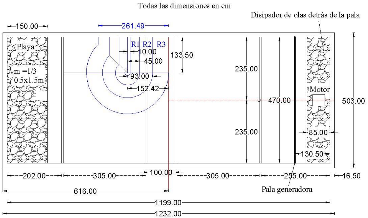
Figura 3.4 Distancias longitudinales del morro, considerando como eje longitudinal principal la línea rojo discontinua localizada a los 2.35 m
