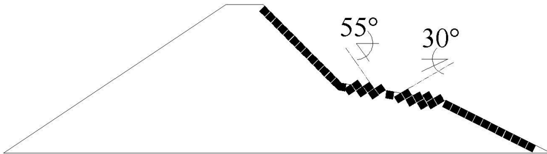
Figura 2.18 DRPS en S con cubos auto-organizados en región 2 del perfil en S
