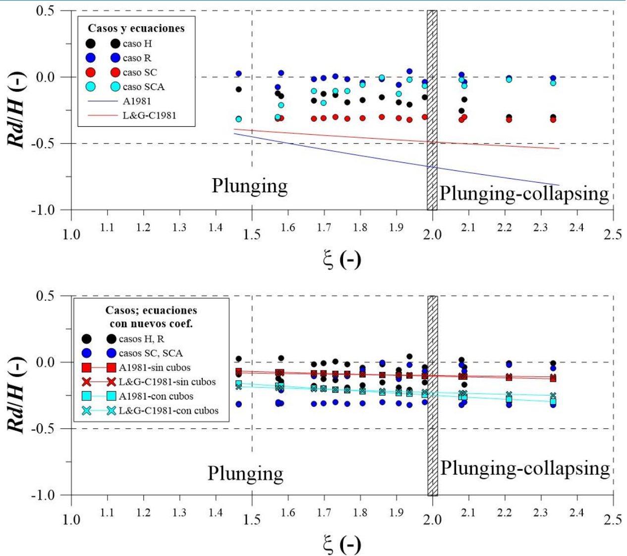
Figura 2.34 Comportamiento de 2 ecuaciones ajustadas a los resultados numéricos de Rd/H . En el panel superior, las ecuaciones sin los coeficientes cf . En el panel inferior, las ecuaciones con los coeficientes cf
