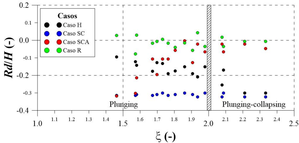
Figura 2.29 Resultados del descenso máximo adimensional en función del número de Iribarren
