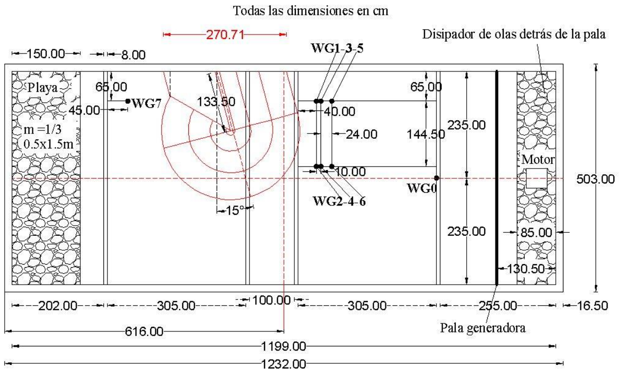
Figura 3.20 Primer arreglo de sensores: 15 grados
