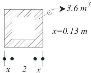
Figura 2.16 Separación de los cubos colocados a lo largo del perfil en S
