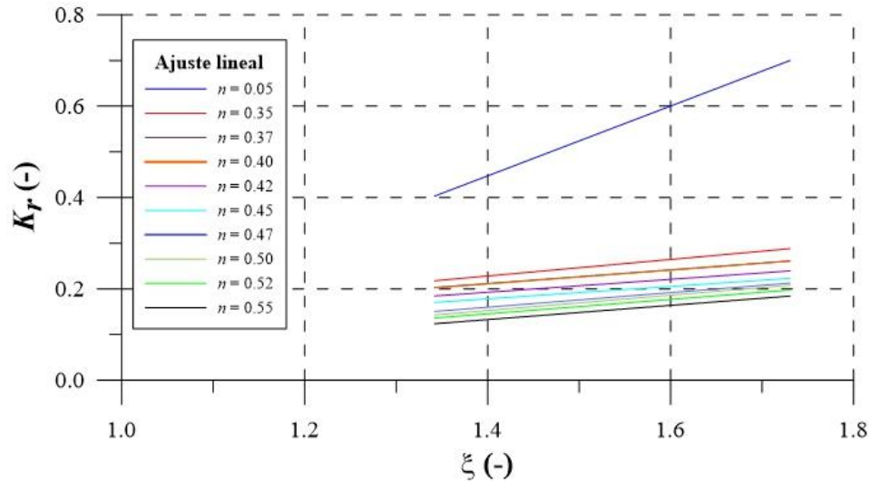
Figura 2.46 Curvas de ajuste K_r = f(\xi)
