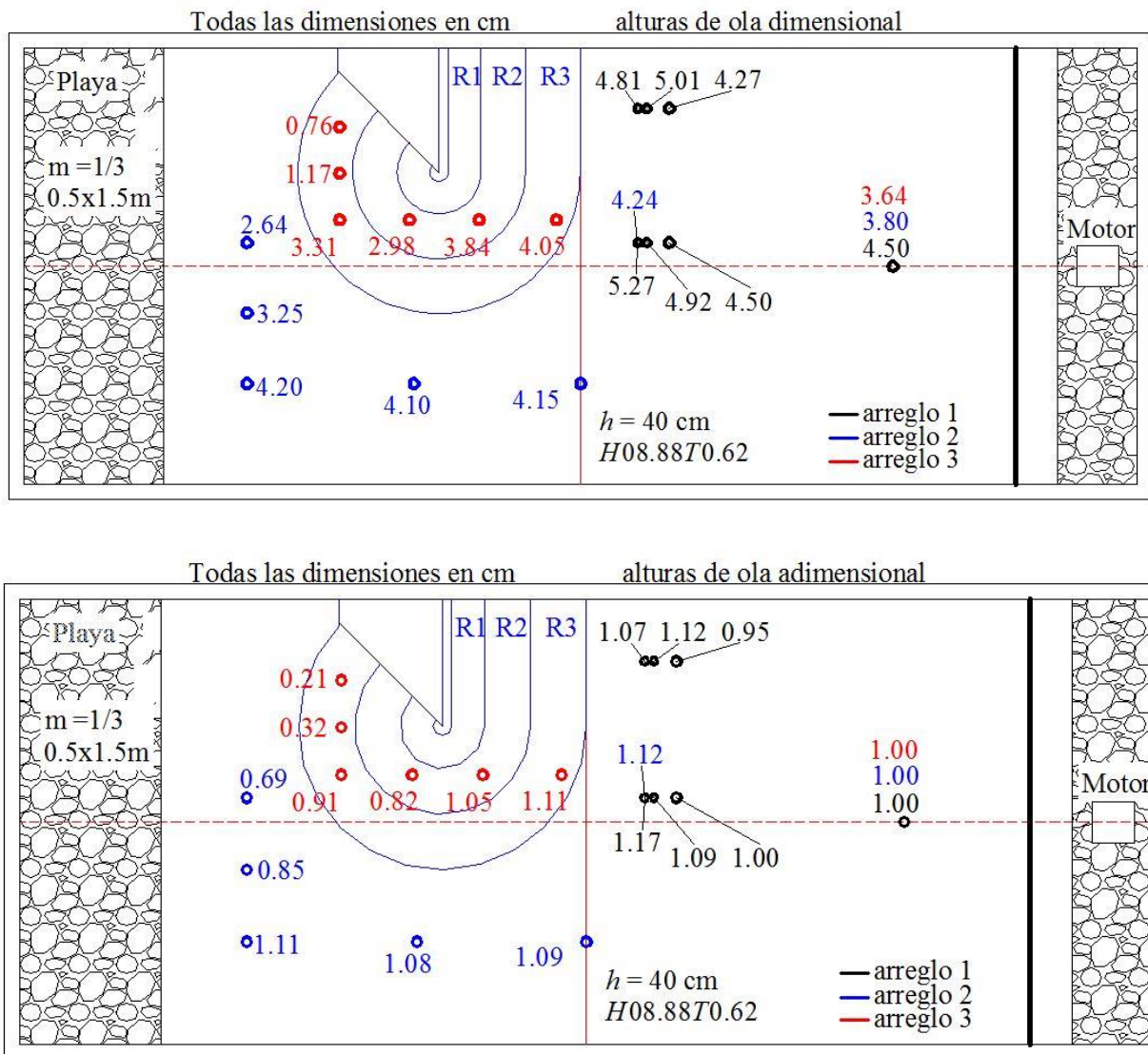
Figura 3.30 Resultados del estado de mar H = 8.88 cm, T = 0.62 s, h = 40 cm, giro = 0^\circ
