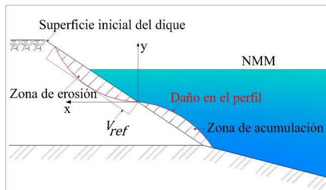
Figura 1.3 Esquema del daño del perfil expuesto a la acción del oleaje (Ergin et al. (1989))
