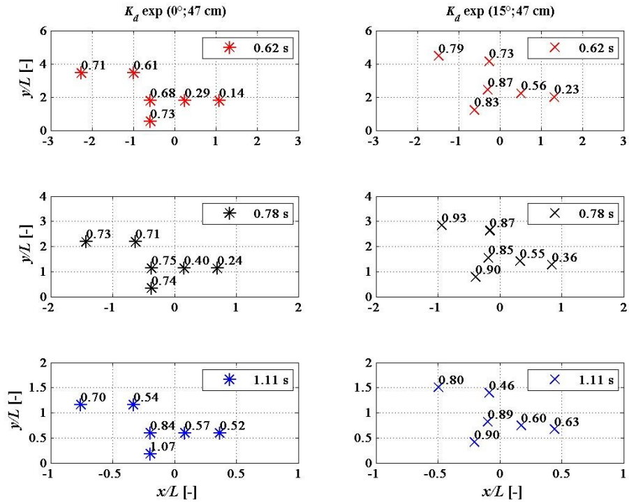
Figura 3.38 Valores promedio-experimentales de K_d considerando la profundidad de 47 cm
