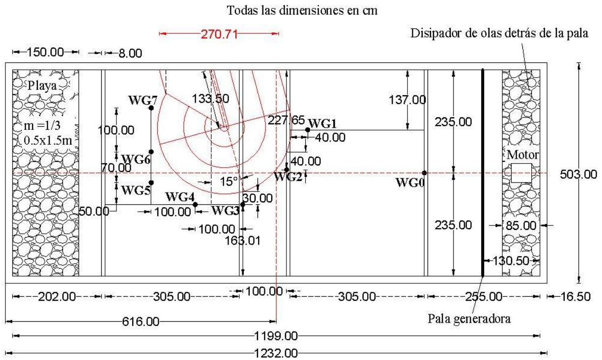
Figura 3.21 Segundo arreglo de sensores: 15 grados
