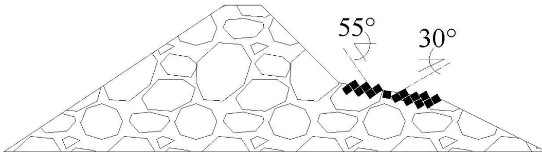
Figura 2.19 DRPS en S con cubos auto-organizados solo en la región 2 del perfil en S
