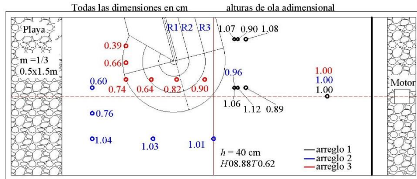
Figura 3.31 Resultados del estado de mar H = 8.88 cm, T = 0.62 s, h = 40 cm, giro = 15^\circ
