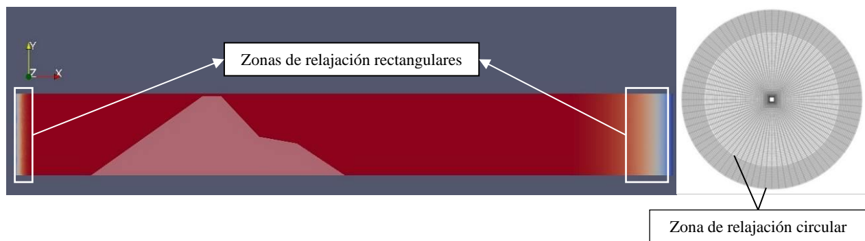
Figura 2.6 Formas geométricas que por defecto están definidas en la librería waves2foam
