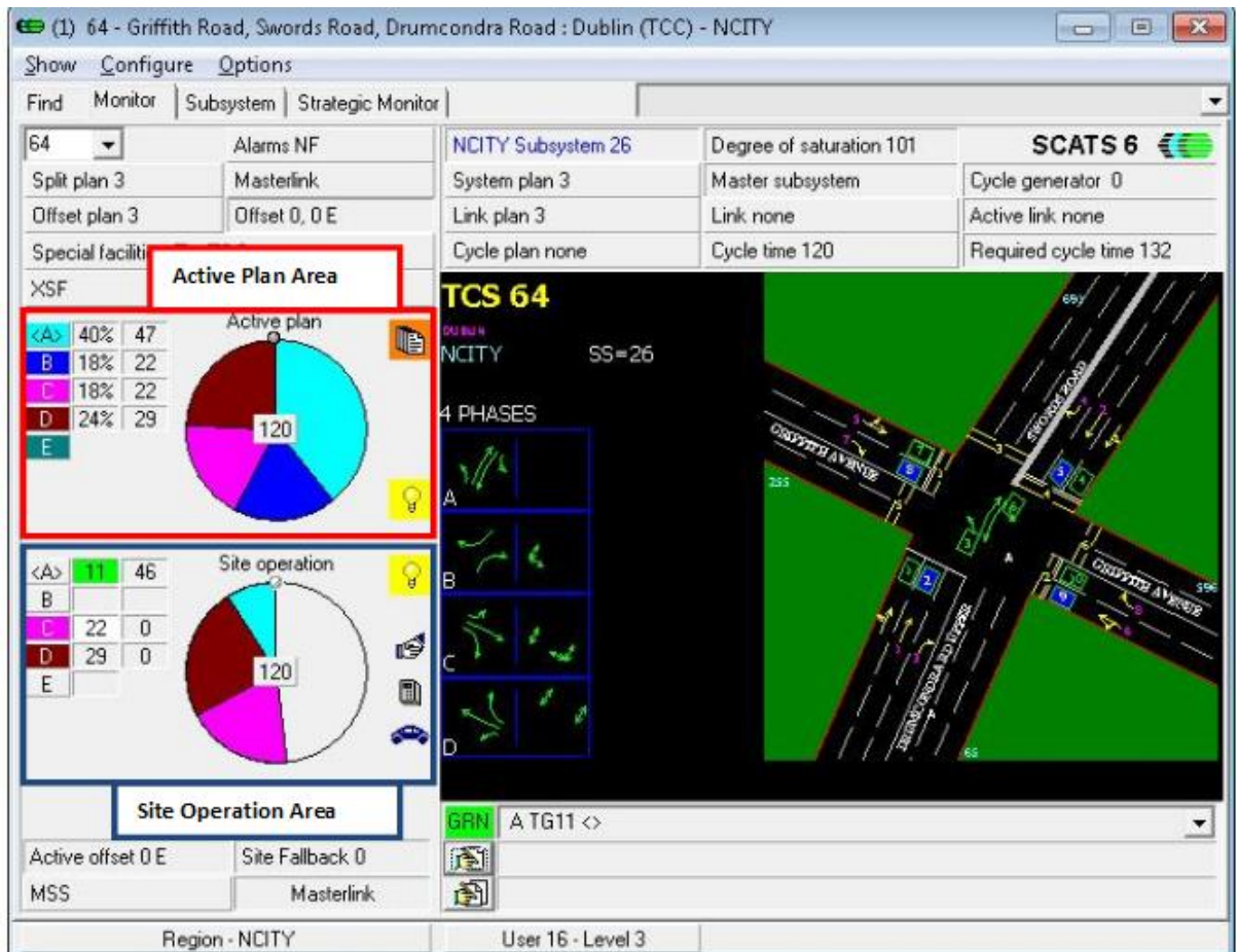
Figura 3.26. Interfaz del usuario en SCATS
