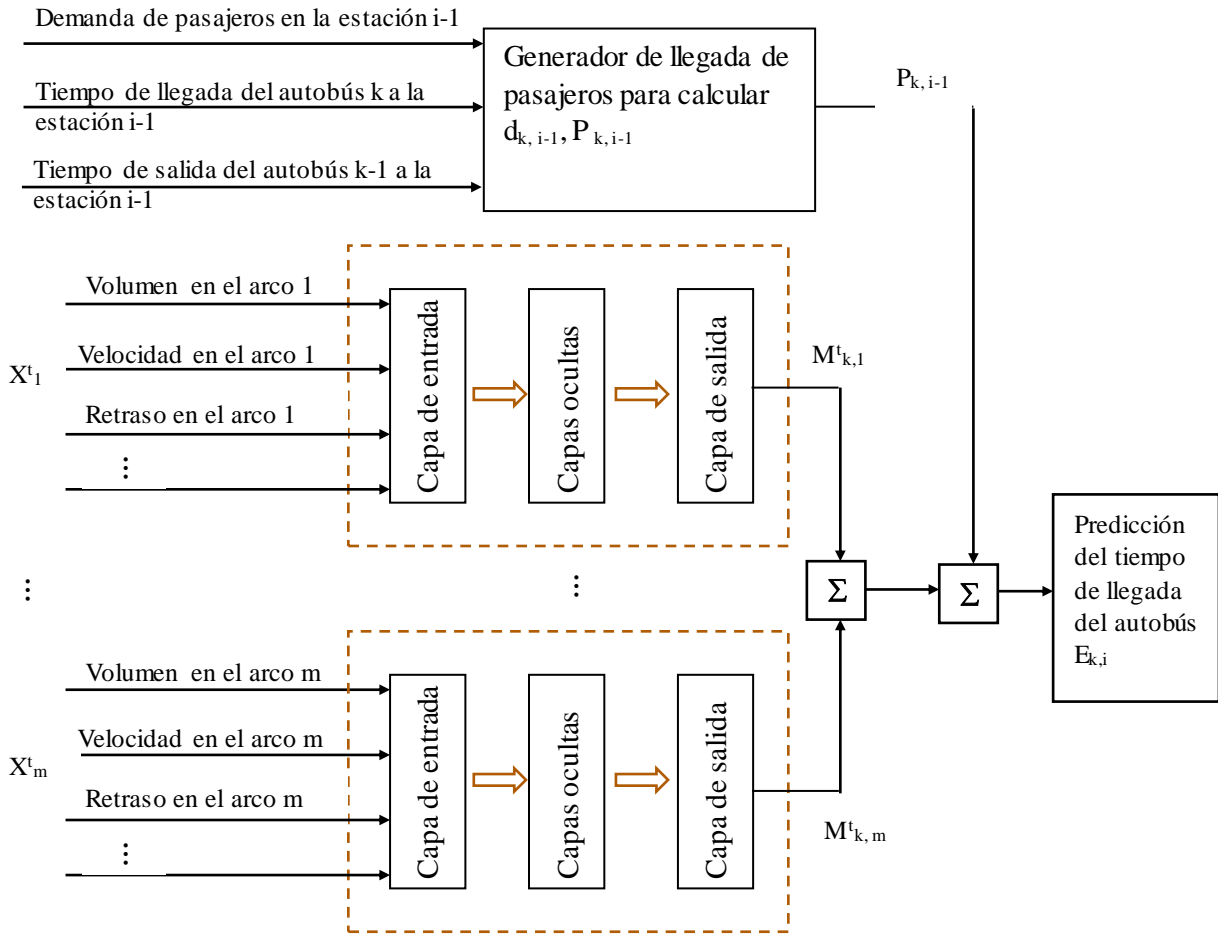
Figura B.2. Modelo de redes neuronales basado en arcos Fuente: (Chien, Ding y Wei, 2002)
