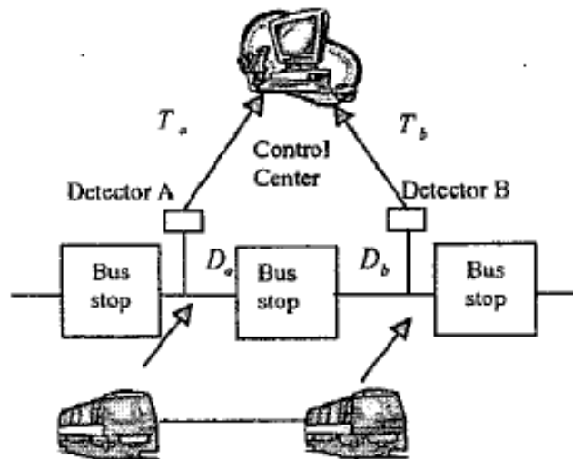
Figura 3.38. Dispositivos RSU para localización de vehículos Fuente: (Wang et al., 2002)
