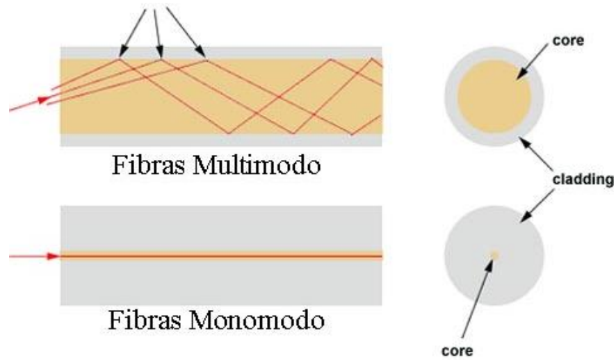
Figura 3.68. Fibra óptica multimodo y monomodo Fuente: (Rodríguez, 2012)
