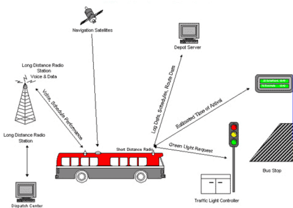
Figura 3.41. Sistema de prioridad semafórica y localización de vehículos Fuente: (ADLink, 2015)
