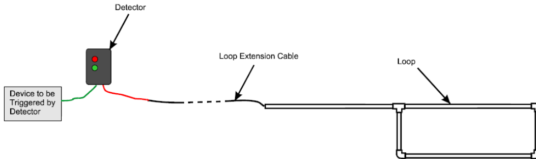
Figura 3.17. Bucles de inducción Fuente: (Marsh Products, 2000)
