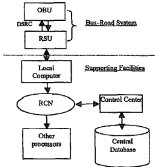
Figura 3.37. Esquema general del funcionamiento del sistema DSRC Fuente: (Wang et al., 2002)
