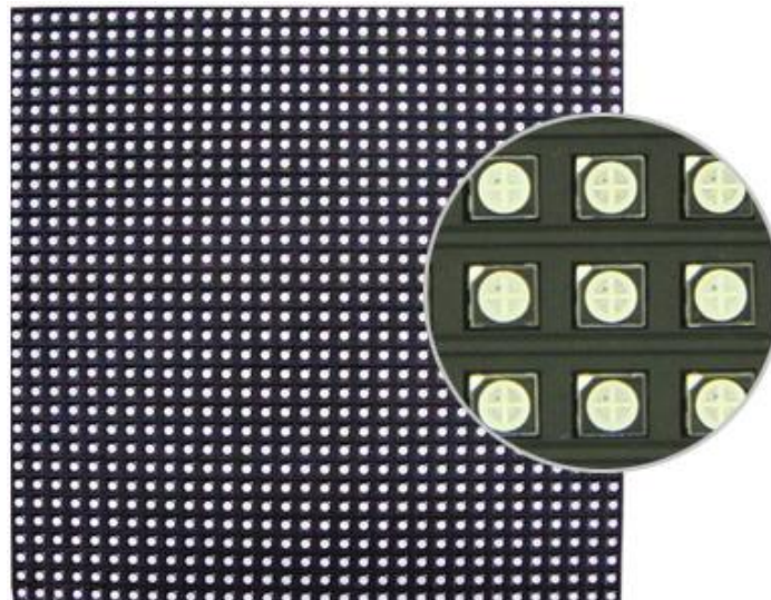
Figura 3.56. LED tipo SMD Fuente: (HTL Display, 2014)
