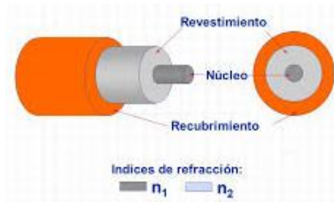
Figura 3.34. Estructura de la fibra óptica Fuente: (Blandón, 2014)
