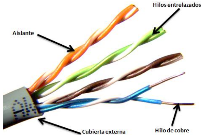
Figura 3.31. Cable de pares Fuente: (Blog Tecnología, 2015)
