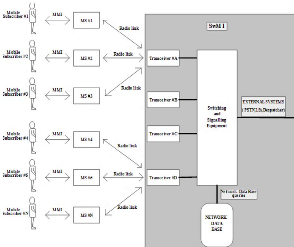
Figura 3.36. Estructura de la red Tetra Fuente : (European Telecommunications Standards Institute, 1997)
