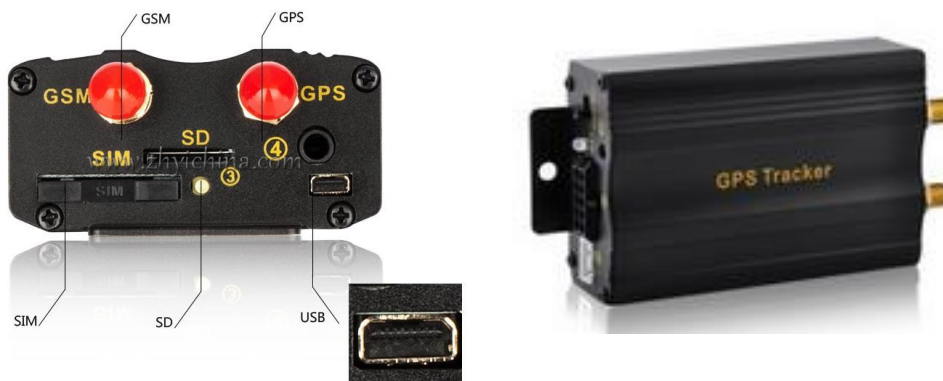
Figura 3.49. Dispositivo GPS conectado al sistema eléctrico del vehículo Fuente: (PosiTrace, 2016)
