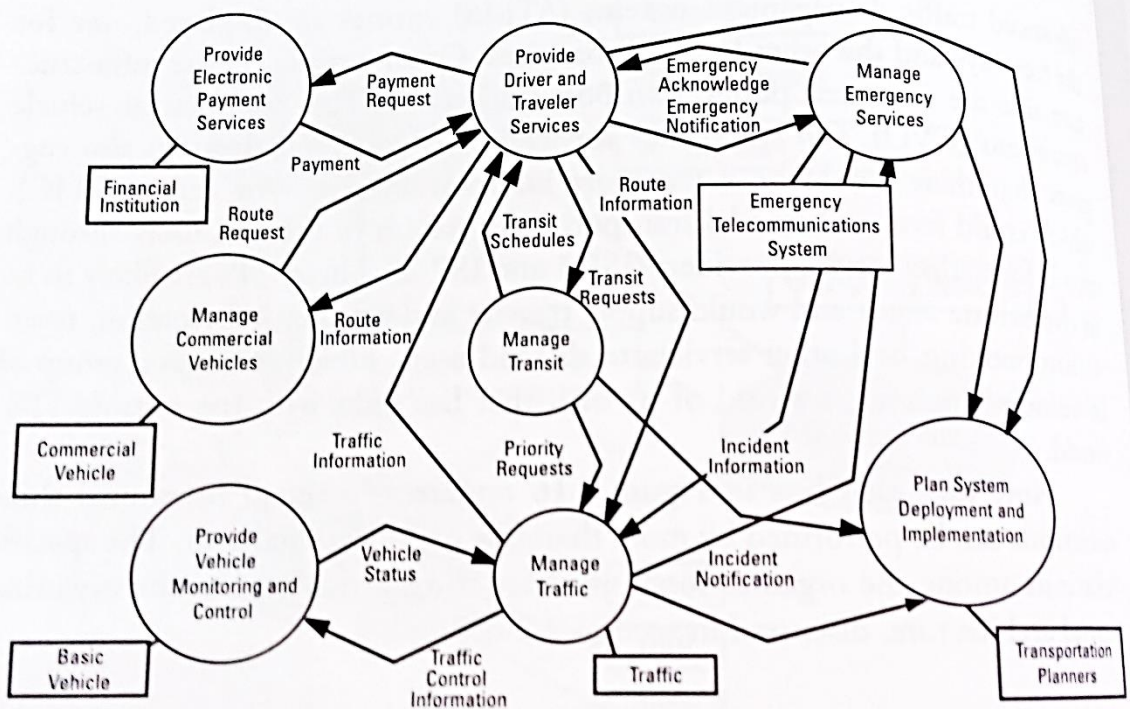
Figura 2.29. Arquitectura lógica Fuente: (World Road Association, 1999)
