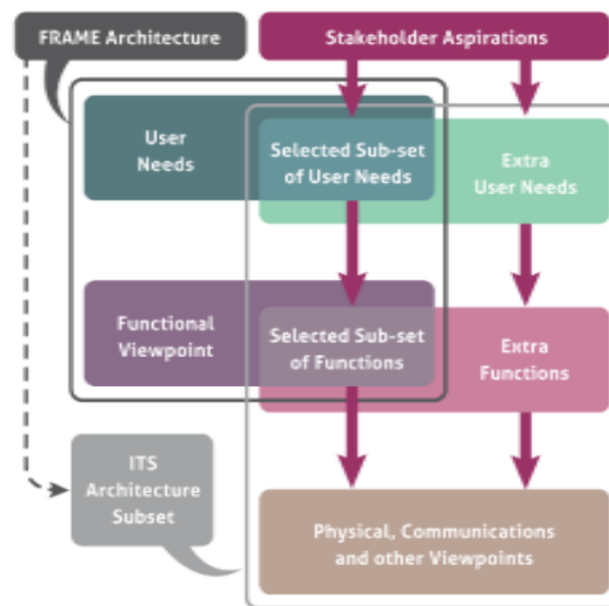
Figura 2.30. Arquitectura ITS Unión Europea Fuente: (Frame Architecture, 2016)
