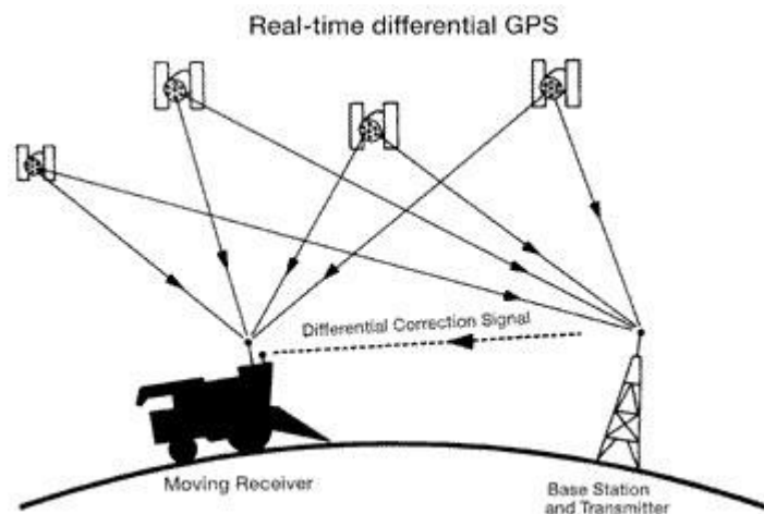
Figura 3.13. El DGPS o GPS Diferencial Fuente: (University of Missouri, 1998)
