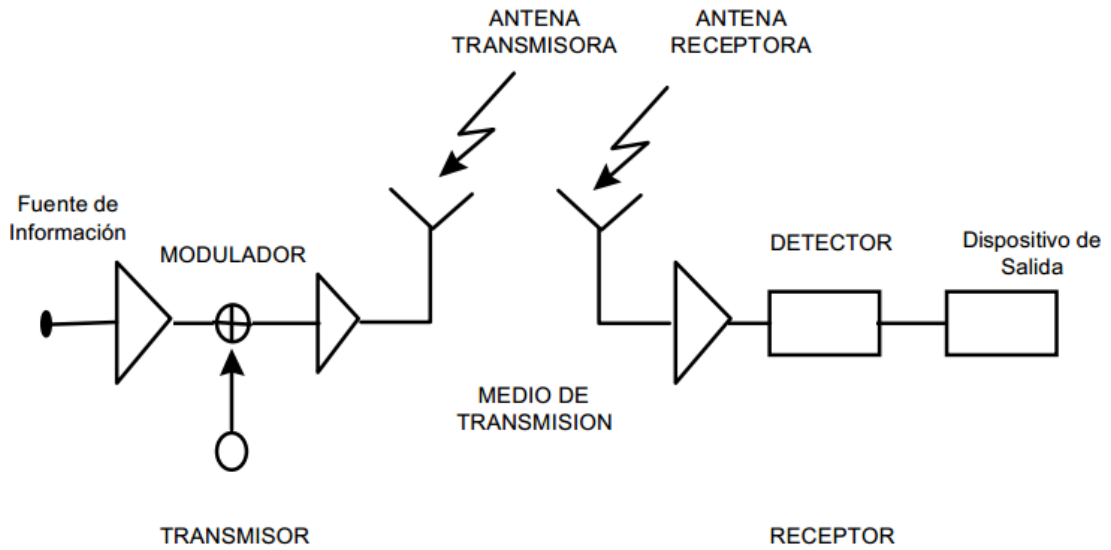
Figura 3.35. Funcionamiento de un sistema de radiocomunicación Fuente : (Jardón y Linares, 1995)
