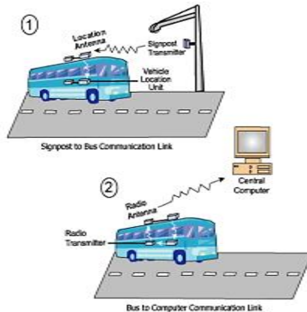
Figura 3.9. Localización de vehículos por signpost Fuente: (ITS Decision, s.f.)
