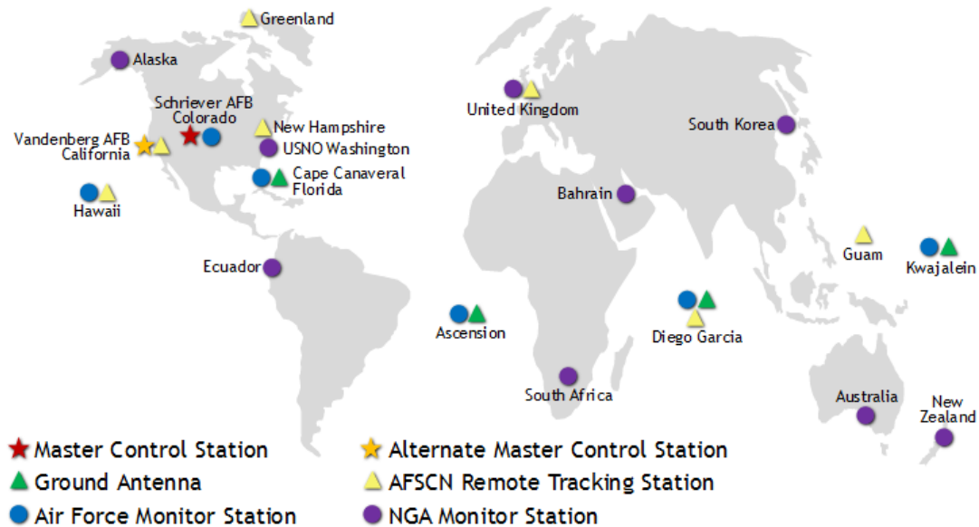
Figura 3.10. Segmento de control GPS Fuente: (GPS.gov, 2016)
