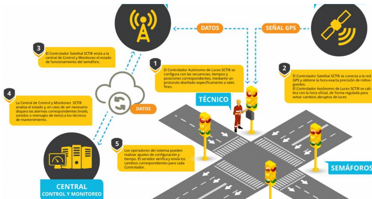
Figura 4.12. Sistema de control de tránsito Fuente: (SCT Vial, 2017)
