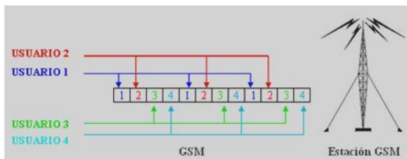
Figura 3.39. Tecnología GSM Fuente: (Albarracín, 2015)
