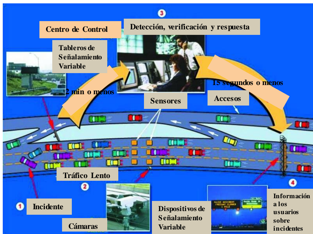
Figura 2.2. Funcionamiento de un SAGeT Fuente: (Southwest Research Institute, 2016)
