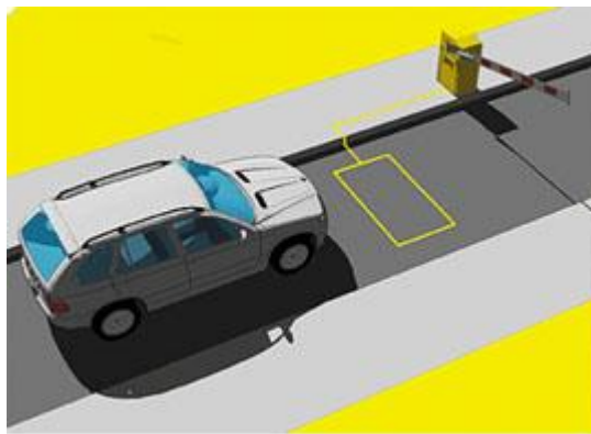
Figura 3.18. Cables instalados sobre la superficie de rodamiento Fuente: (Empretel, 2016)
