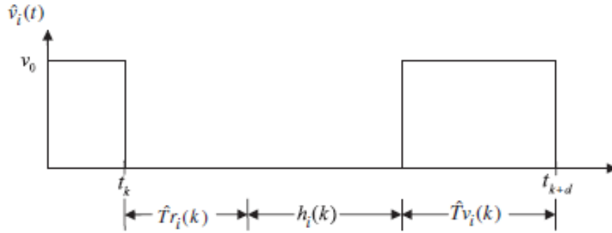
Figura 3.24. Función de velocidad del autobús i Fuente: (Sáez et al., 2012)
