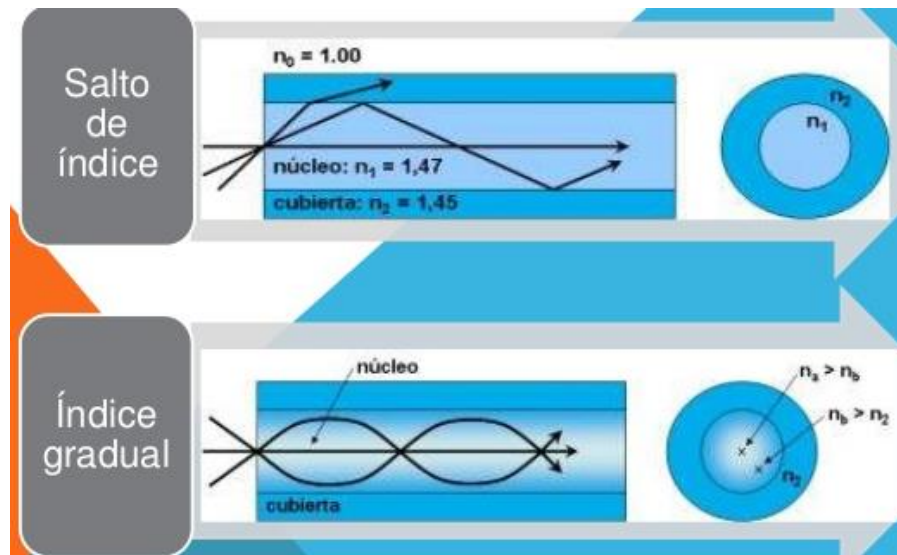
Figura 3.69. Tipos de fibra óptica multimodal Fuente: (Cabascango, Lomas y Ramos, 2014)
