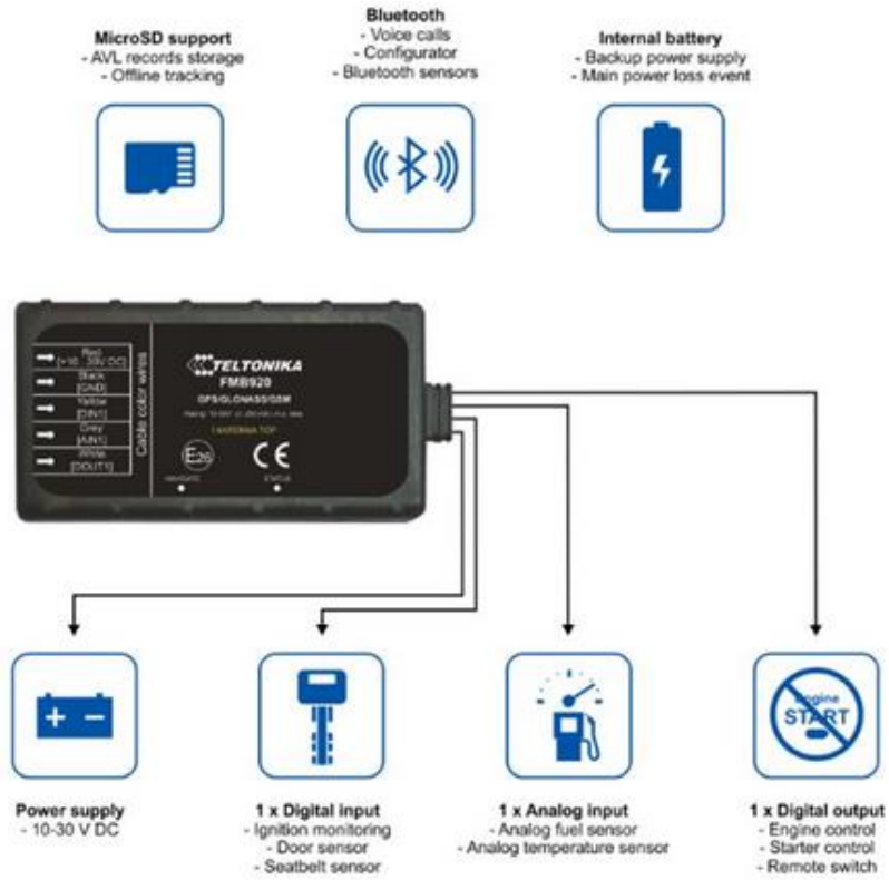
Figura 3.51. Dispositivos GPS con antena interna Fuente: (Teltonika, 2017)
