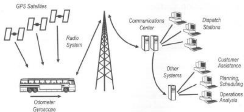
Figura 3.40. Localización automática de vehículos utilizando GPS
