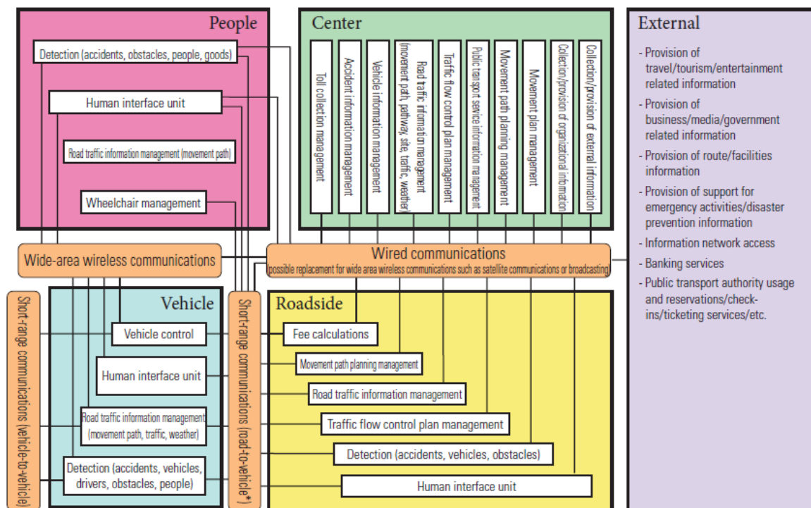
Figura 2.31. Arquitectura ITS Japón Fuente: (Hasegawa, 2013)
