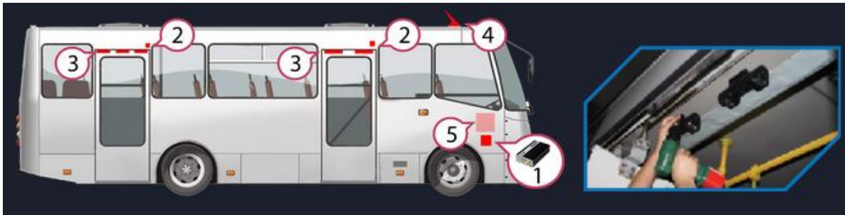
Figura 3.6. Sensores para conteo de pasajeros Fuente: (Starfinder Bus, 2013)
