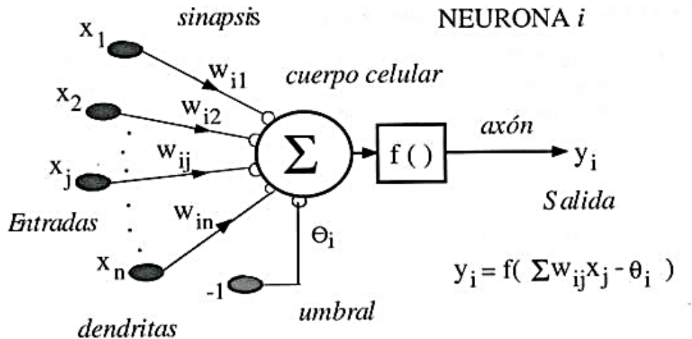
Figura A.2. Modelo de una neurona estándar Fuente: (Aguilar, 1999)
