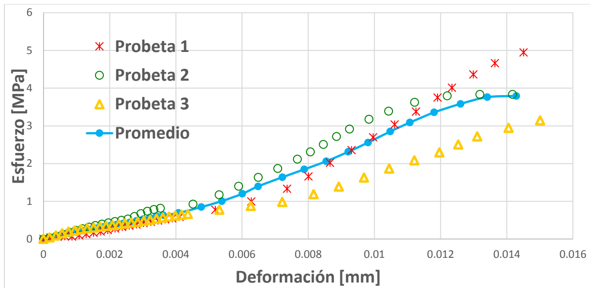
Figura 4.27 Gráfica de esfuerzo-deformación de la mezcla R-5
