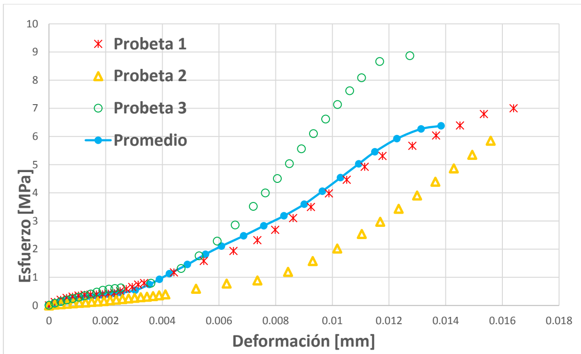
Figura 4.21 Gráfica de esfuerzo-deformación de la mezcla B
