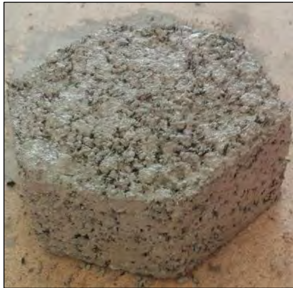
Figura 4.32 Adoquín hecho con mezcla B-2
