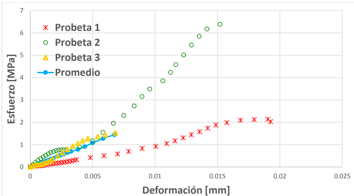
Figura 4.22 Gráfica de esfuerzo-deformación de la mezcla B-2
