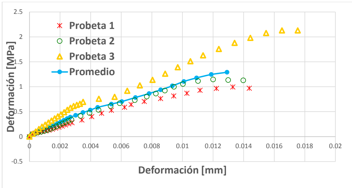
Figura 4.24 Gráfica de esfuerzo-deformación de la mezcla B-10
