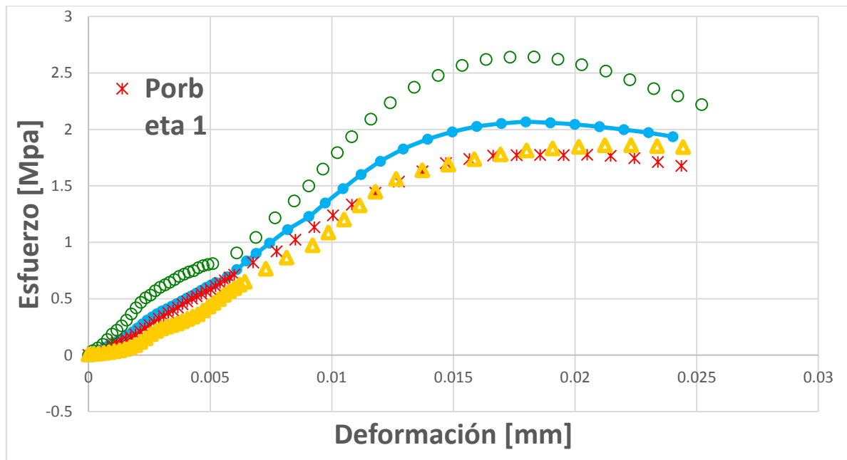
Figura 4.28 Gráfica de esfuerzo-deformación de la mezcla R-10
