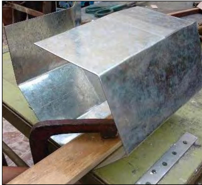
Figura 4.6 Doblado de lámina galvanizada
