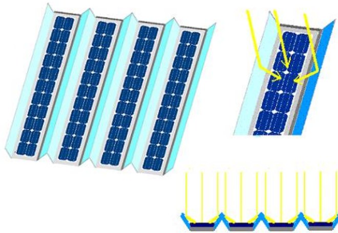
Fig. 2.6 Panel con sistema de concentración.
