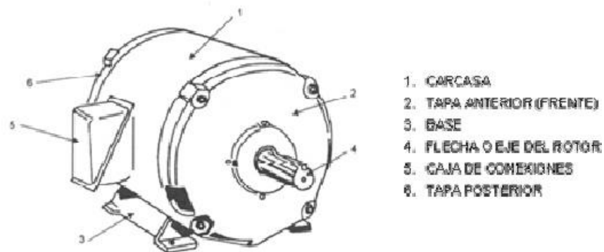
Fig. 1.3 Partes de un motor eléctrico.
