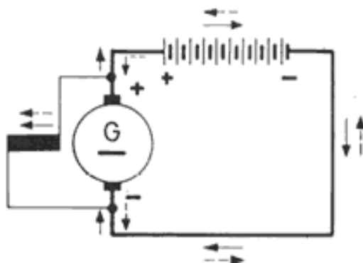
Fig. 1.11 Esquema motor Shunt.
