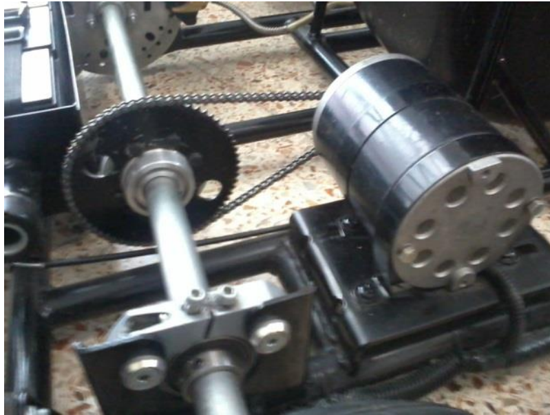
Fig. 4.7 Colocación de sprocket trasero.
