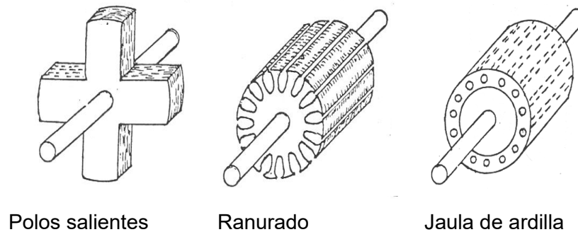
Fig. 1.5 Tipos de rotores.
