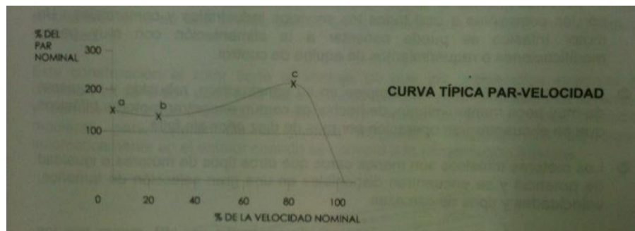
Fig. 1.7 Gráfica curva par- velocidad.
