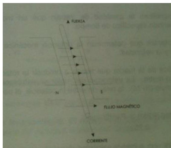
Fig. 1.1 Campo magnético.
