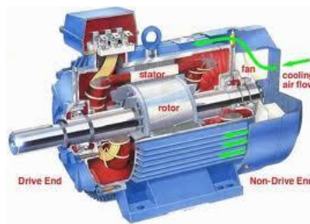
Fig. 1.10 Motor C.D.
