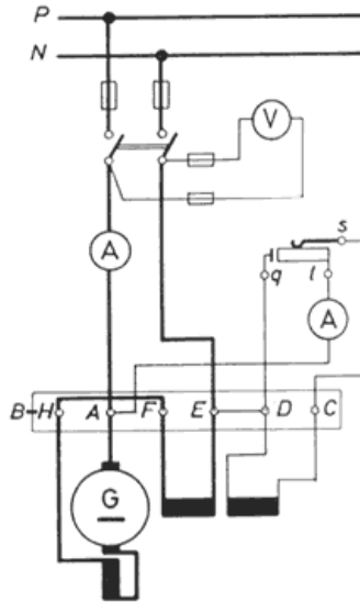
Fig. 1.12 Esquema motor compound.
