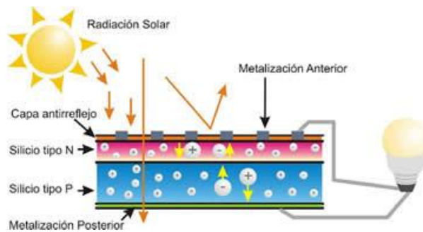
Fig. 2.1 Obtención de la energía eléctrica.
