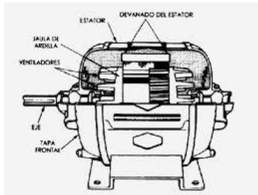
Fig. 1.9 Motor jaula de ardilla.
