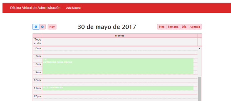
Figura 4.19: Vista Día.
