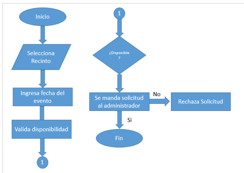
Figura D.6: Reservar Recintos
