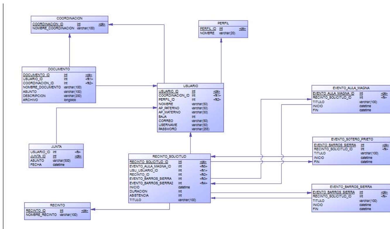
Figura 3.3: Diseño Físico
