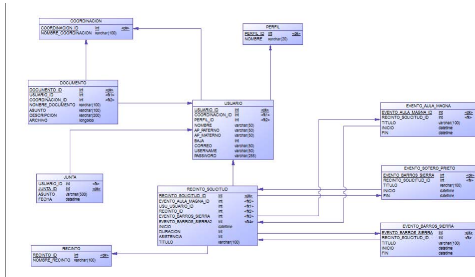
Figura C.1: Modelo entidad-relación
