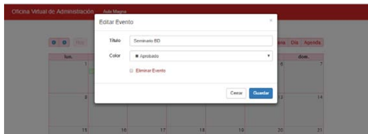
Figura 4.16: Editar Evento.
