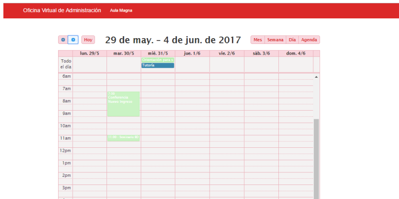
Figura 4.18: Vista Semana.
