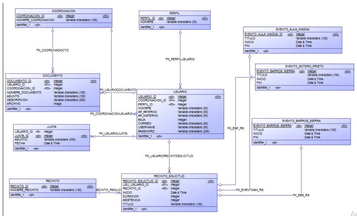
Figura 3.2: Diseño Lógico
