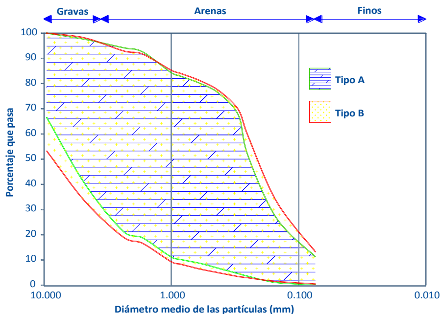
Figura 4.8. Curvas granulométría de los sedimentos
