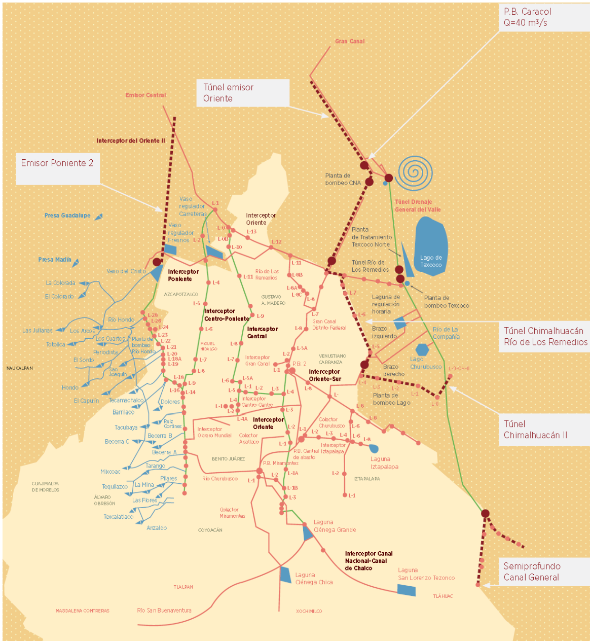
Figura 1.1. Sistema de alcantarillado de la Ciudad de México
