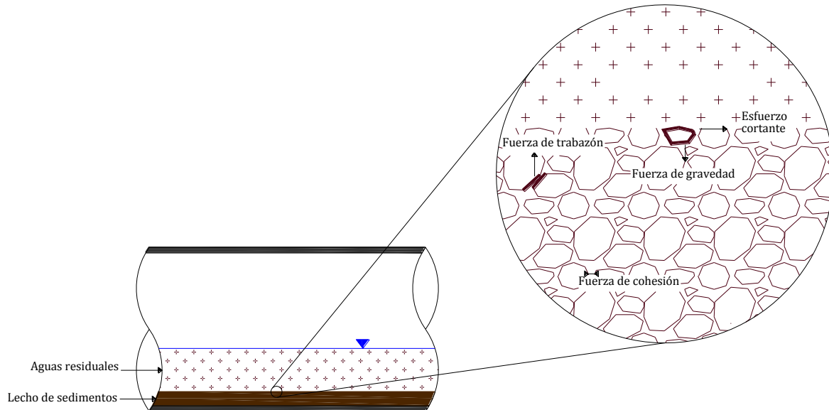
Figura 2.5. Fuerzas hidrodinámicas que se ejercen sobre las partículas
