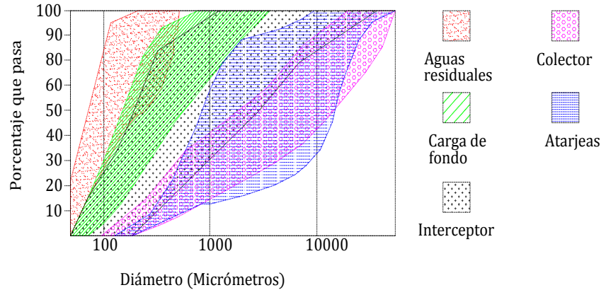
Figura 2.7. Granulometría de los sedimentos de atarjeas, colectores e interceptores
