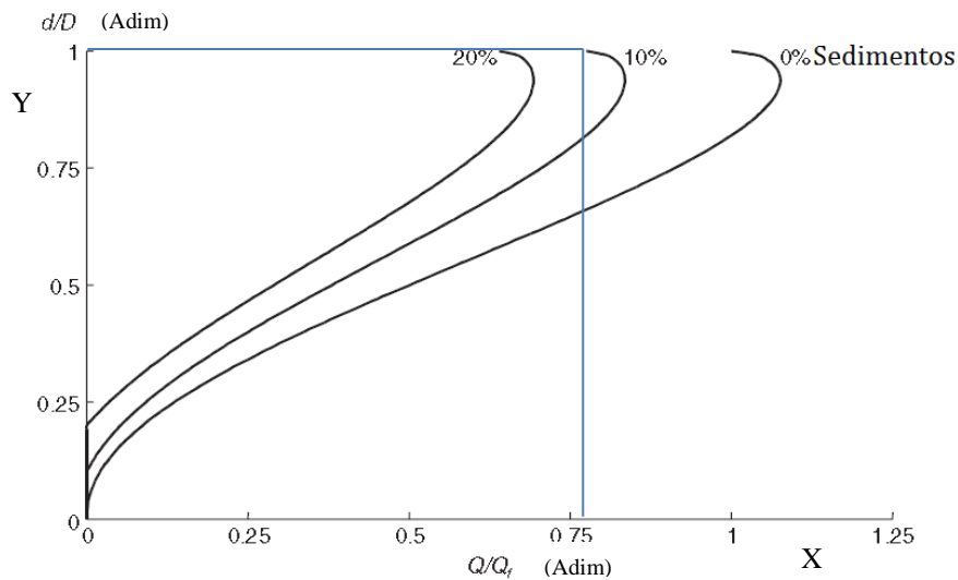
Figura 2.4. Efecto del lecho de sedimentos en la capacidad de flujo de las alcantarillas
