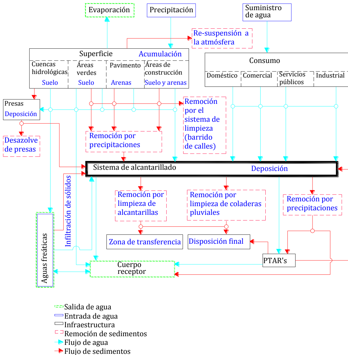
Figura 2.2. Principales entradas y salidas de los sedimentos en los sistemas de alcantarillado urbano
