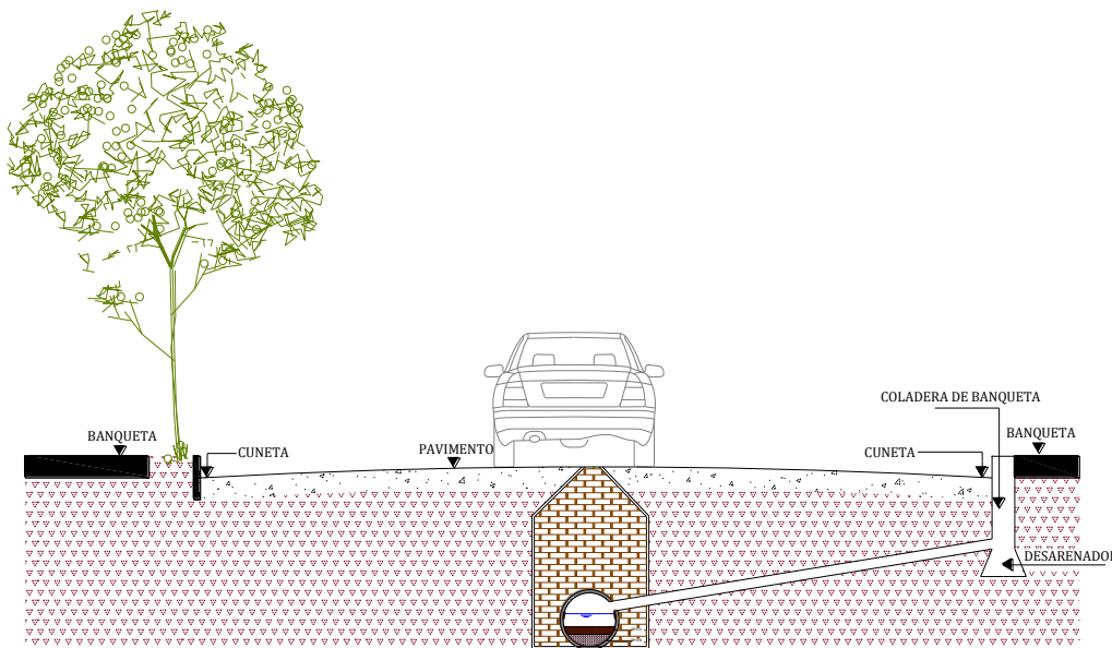
Figura 2.1. Entrada de sólidos a atarjeas
