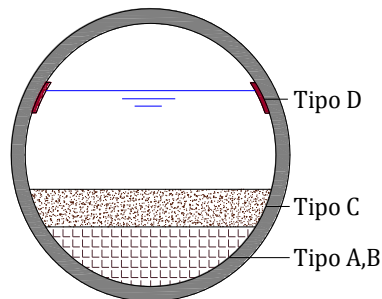
Figura 2.6. Sedimentos típicos en una alcantarilla
