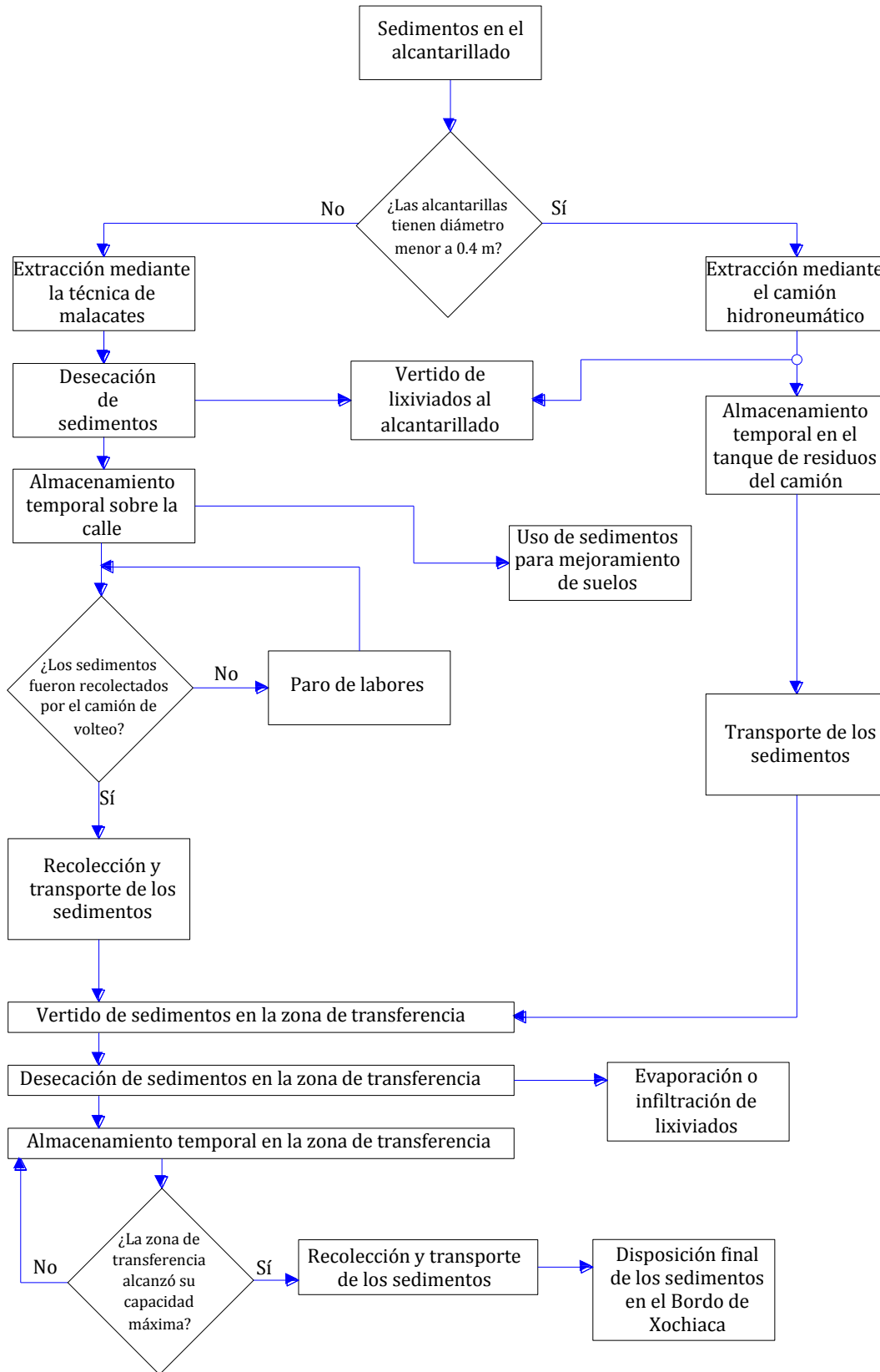
Figura 4.1. Diagrama de las actividades durante el manejo sedimentos en la Ciudad de México
