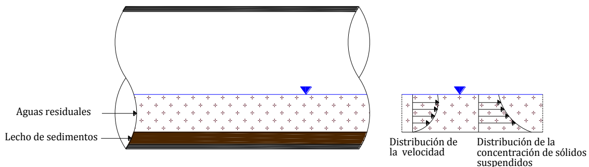
Figura 2.8. Velocidades y distribución de sedimentos suspendidos en tiempo seco
