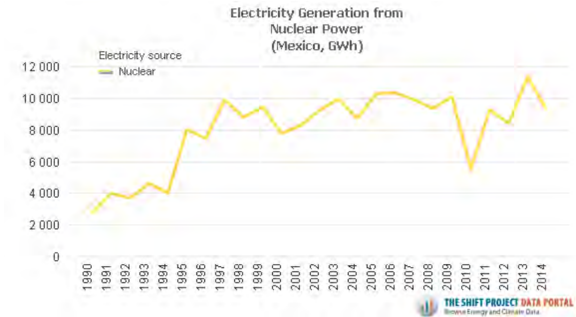
Figura 6. Generación de Electricidad por Energía Nuclear en México desde 1990 hasta 2014 (GWh) 18 .
