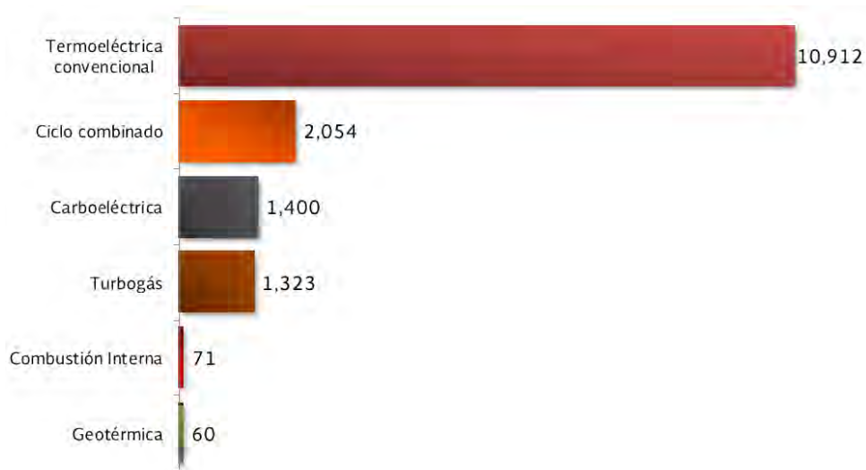
Figura 21. Retiro de Capacidad por tecnología de 2016 a 2030 (MW). 40
