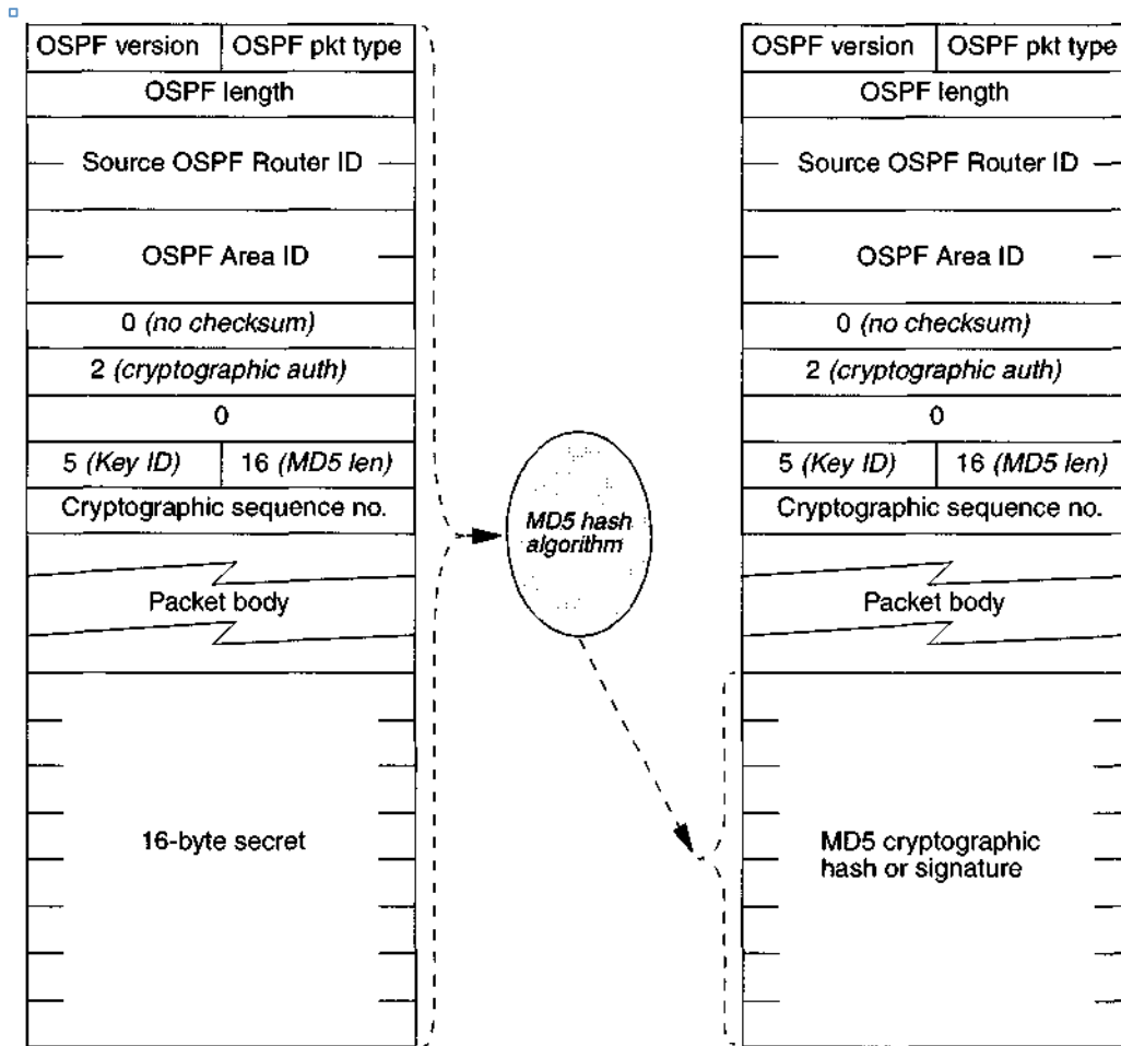
Imagen 2.2 Generación de mensaje OSPF Cryptographic Auth
