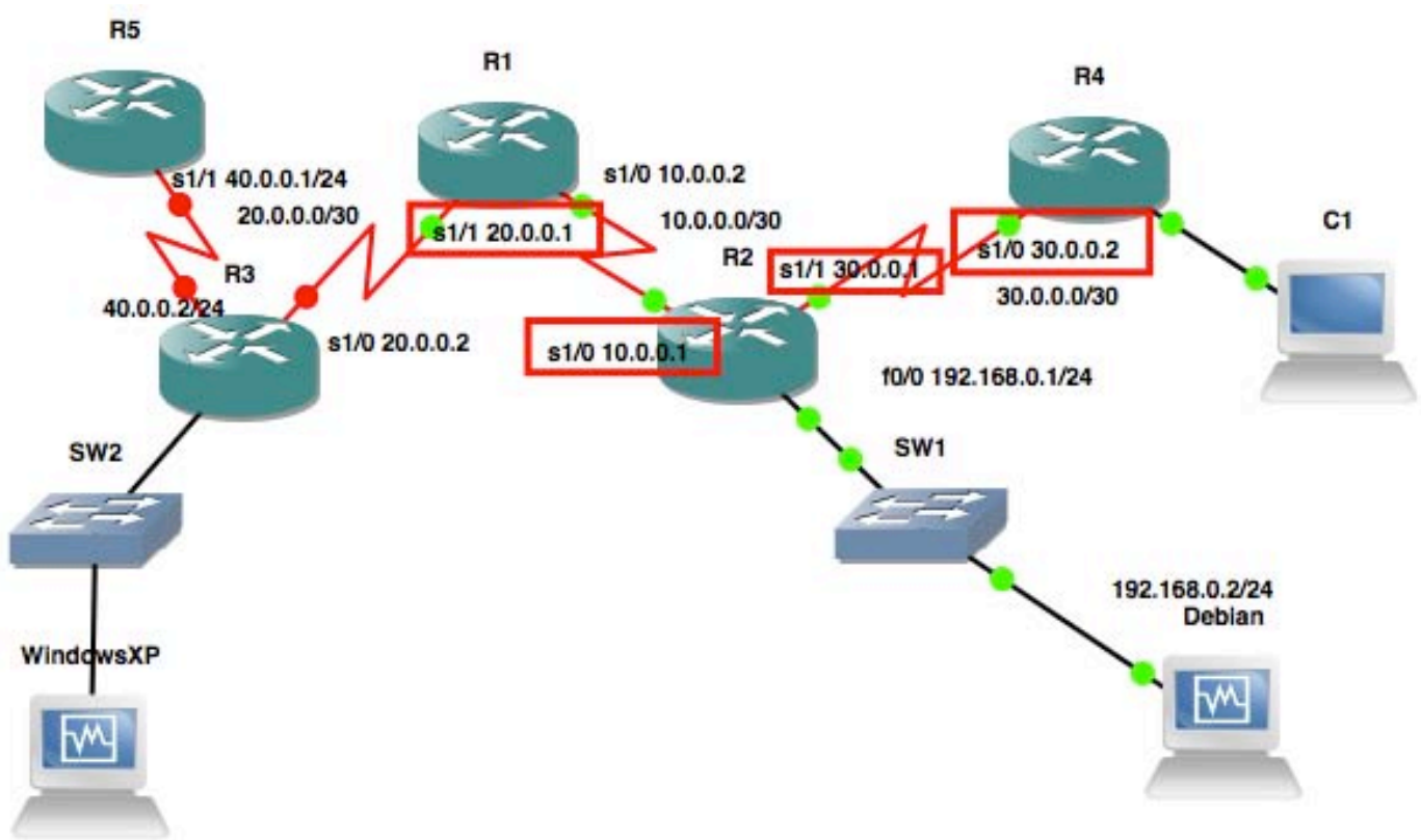
Figura 3.13 (Rutas vecindad de la víctima)
