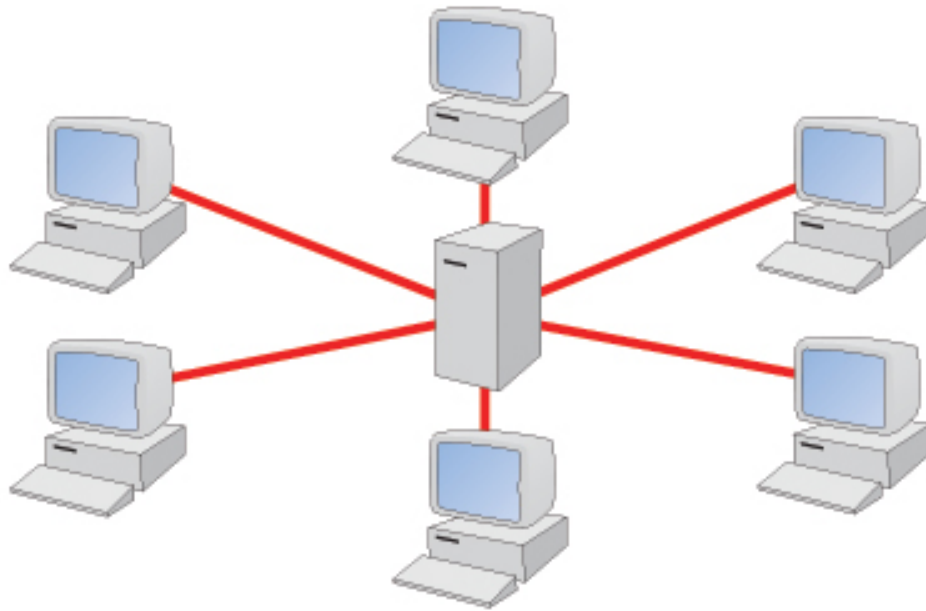
Imagen 1.3 Topología Estrella
