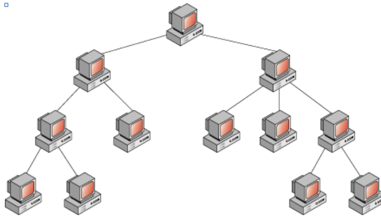
Imagen 1.4 Topología Jerárquica
