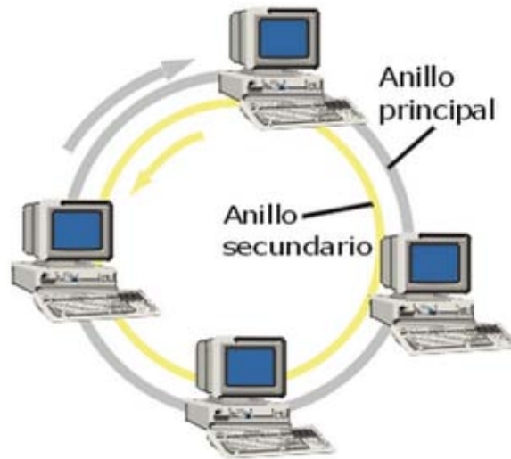
Imagen 1.2 Topología Anillo
