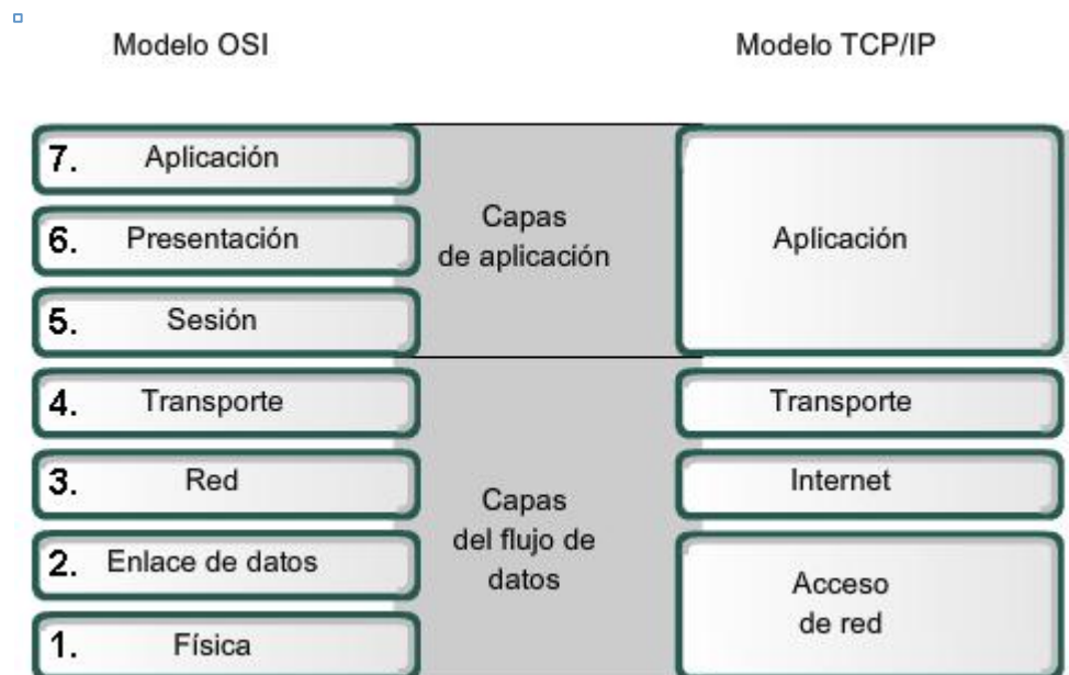
1.6 Modelo_OSI_y_modelo_TCP-IP-2
