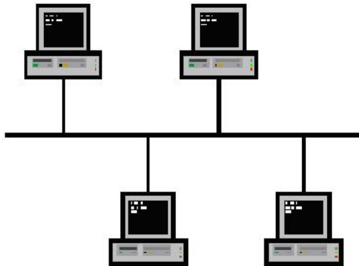
Imagen 1.1 Topología Bus
