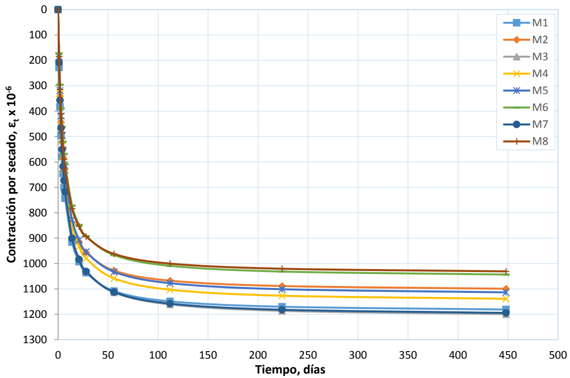
Figura 4.21 Variación de la contracción por secado con el tiempo
