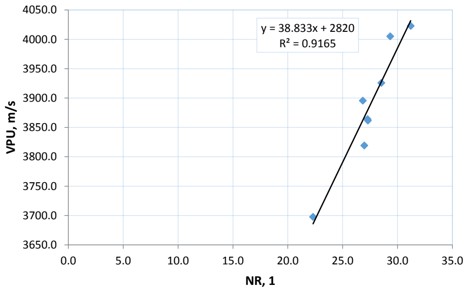
Figura 5.13 Tendencia entre el número de rebote y la VPU a 28 días de edad
