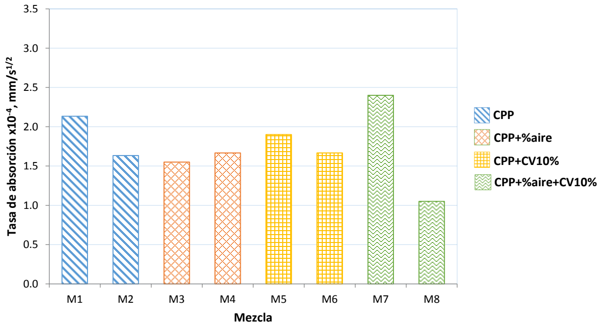
Figura 4.20 Tasa de absorción secundaria a 91 días de edad
