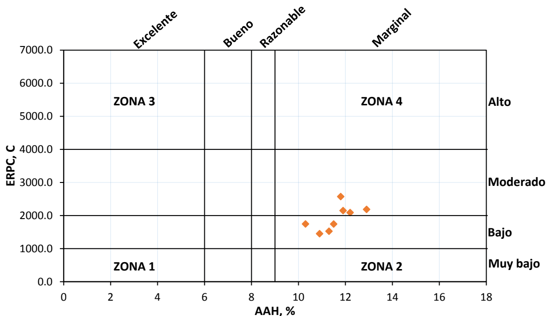
Figura 5.22 Relación entre AAH y ERPC a 91 días de edad
