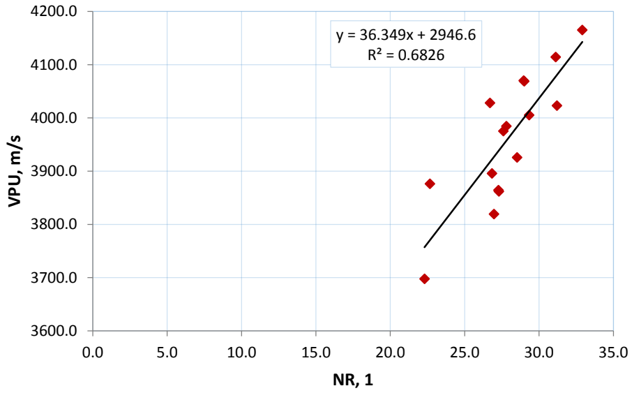
Figura 5.17 Tendencia entre el número de rebote y la VPU a 28 y 91 días de edad
