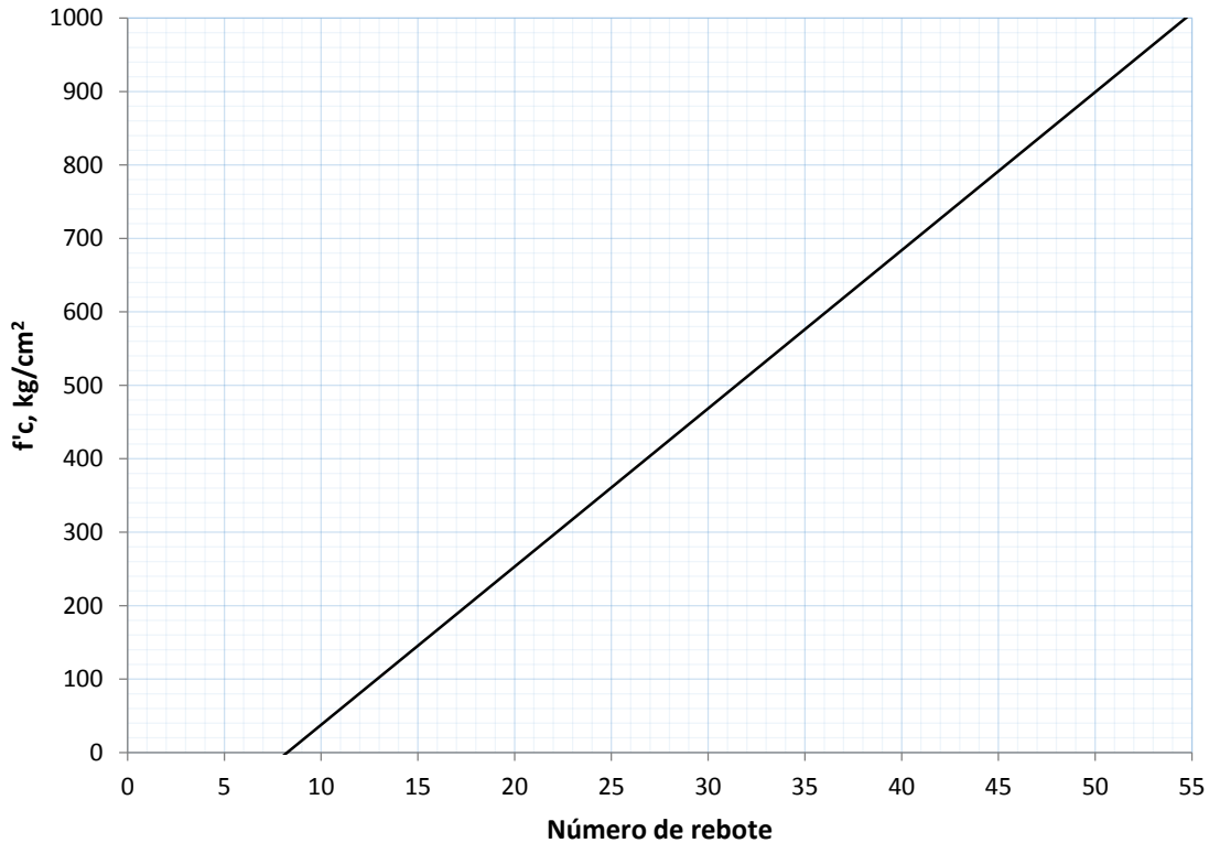
Figura 5.4 Relación entre el número de rebote y la resistencia a compresión simple a 91 días de edad
