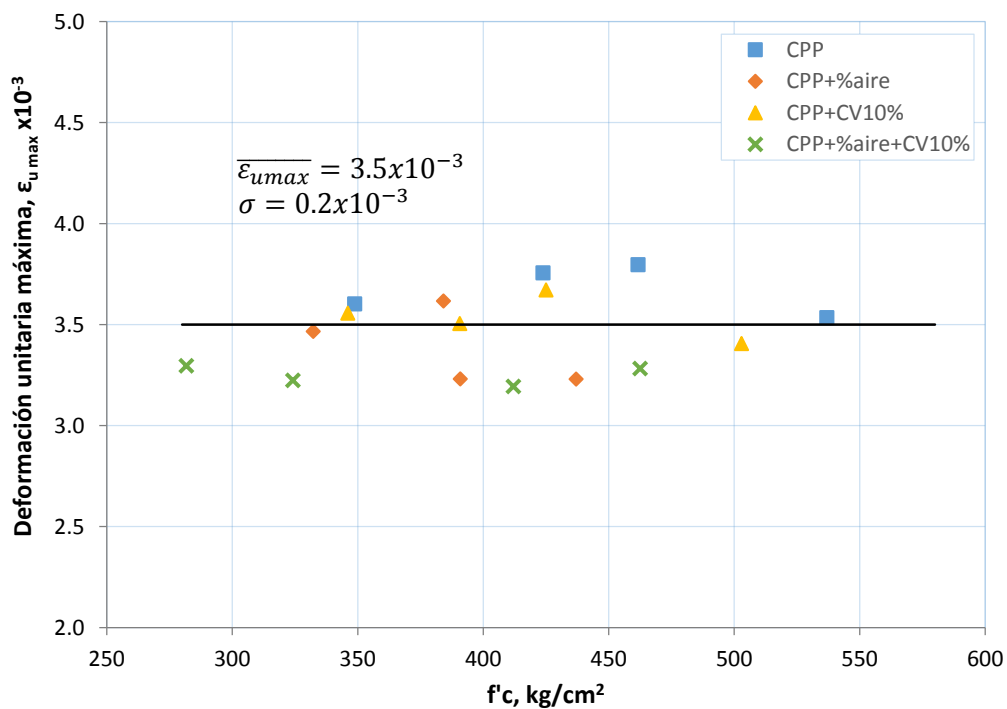
Figura 4.8 Relación entre deformación unitaria máxima y resistencia a compresión simple
