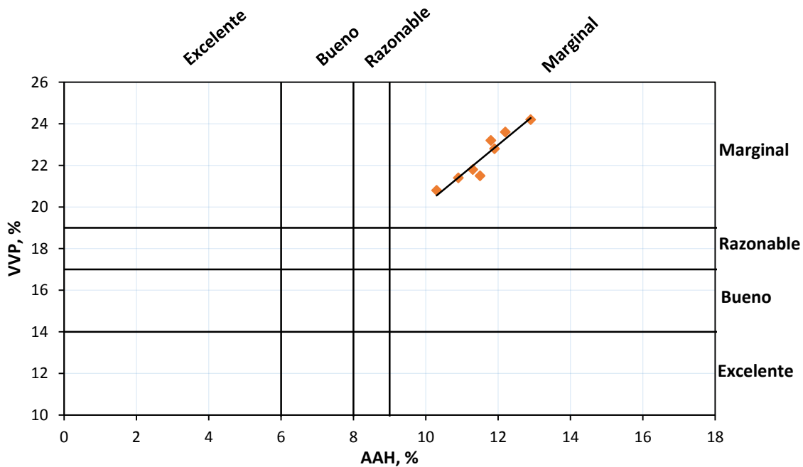
Figura 5.20 Relación entre AAH y VVP a 91 días de edad
