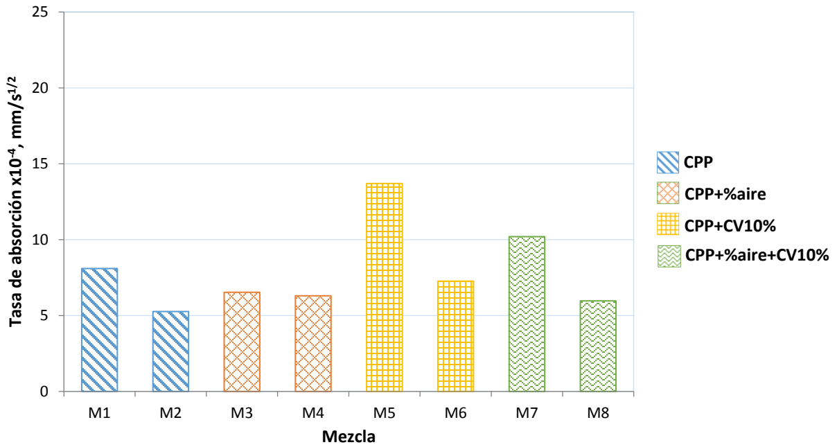
Figura 4.19 Tasa de absorción inicial a 91 días de edad
