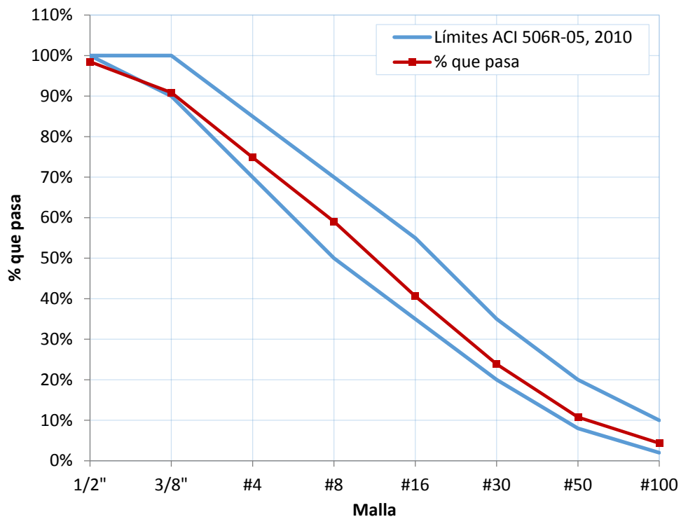
Figura 2.1 Granulometría combinada de los agregados utilizados (relación grava/arena de 25/75).
