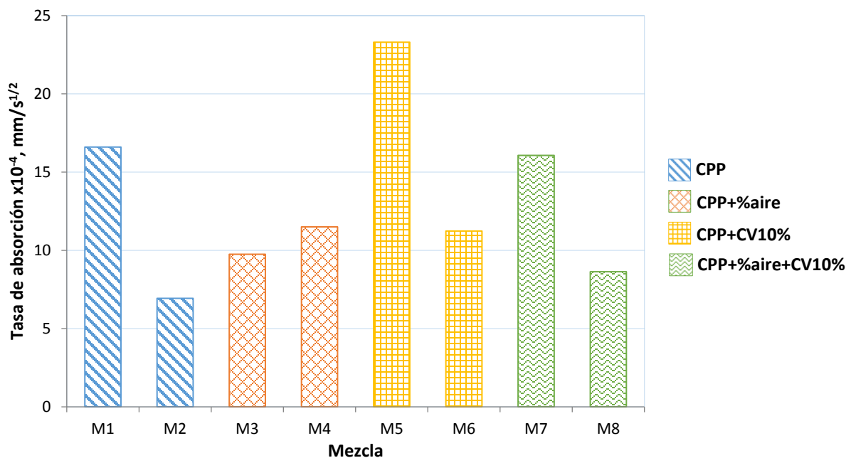
Figura 4.17 Tasa de absorción inicial a 28 días de edad.
