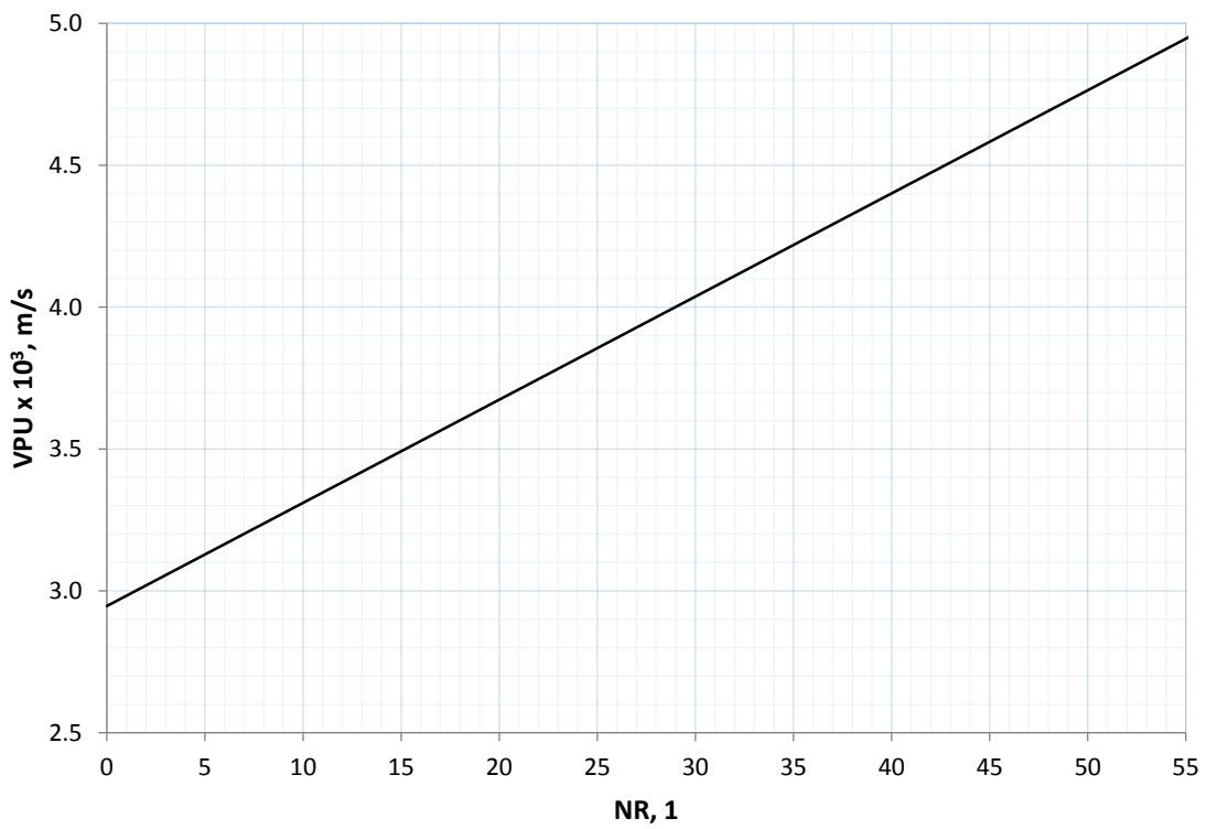
Figura 5.18 Relación entre el número de rebote y la VPU a 28 y 91 días de edad
