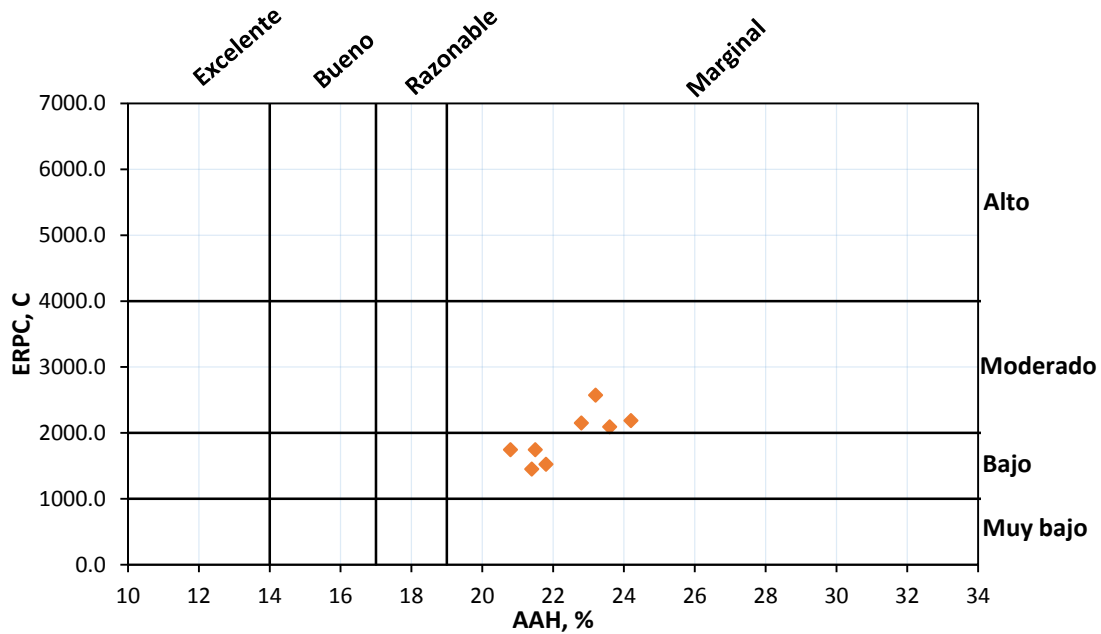
Figura 5.24 Relación entre VVP y el ERPC a 91 días de edad
