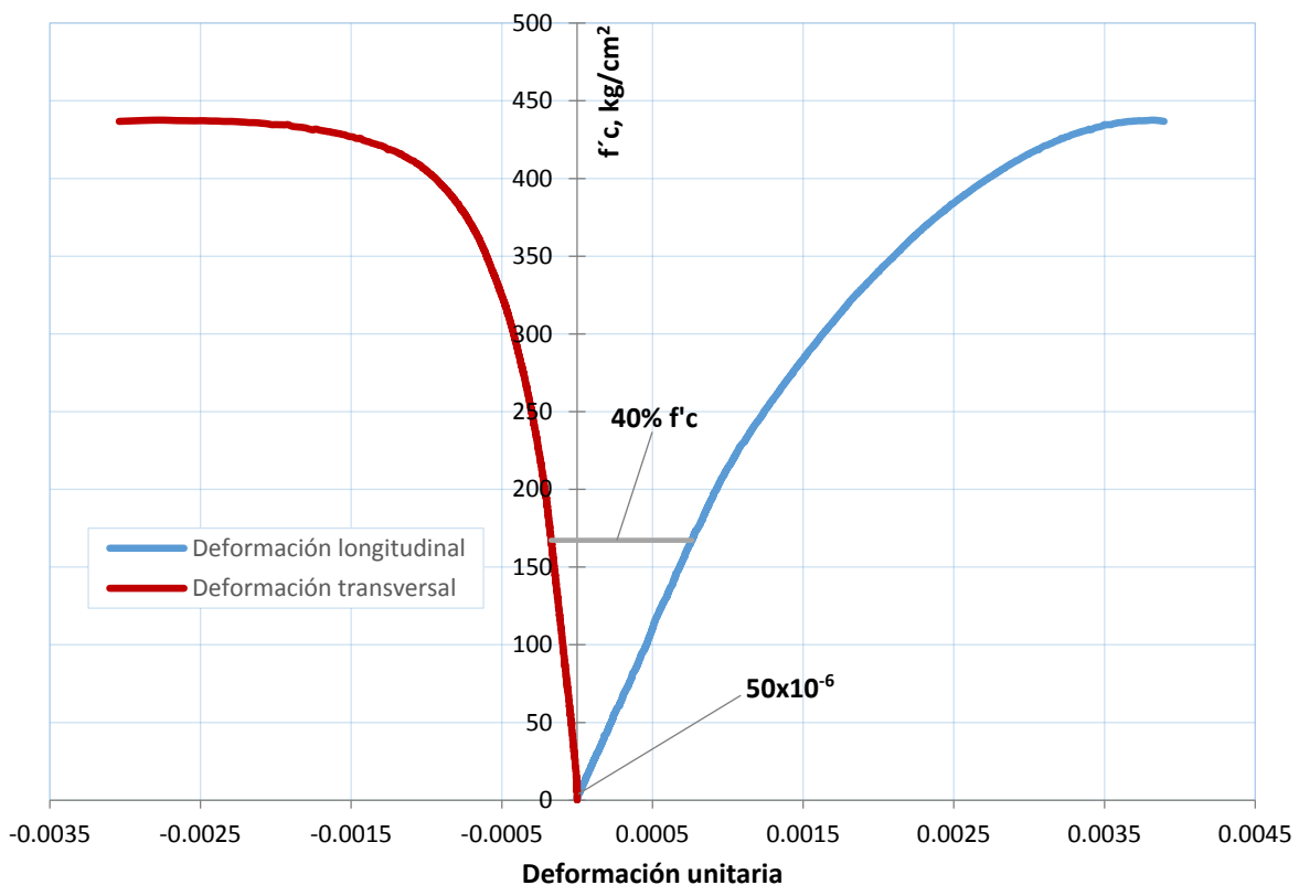
Figura 3.9 Curva esfuerzo – deformación unitaria de un espécimen fabricado con concreto lanzado con un consumo de cemento de 500 \text{ kg/m}^3 .
