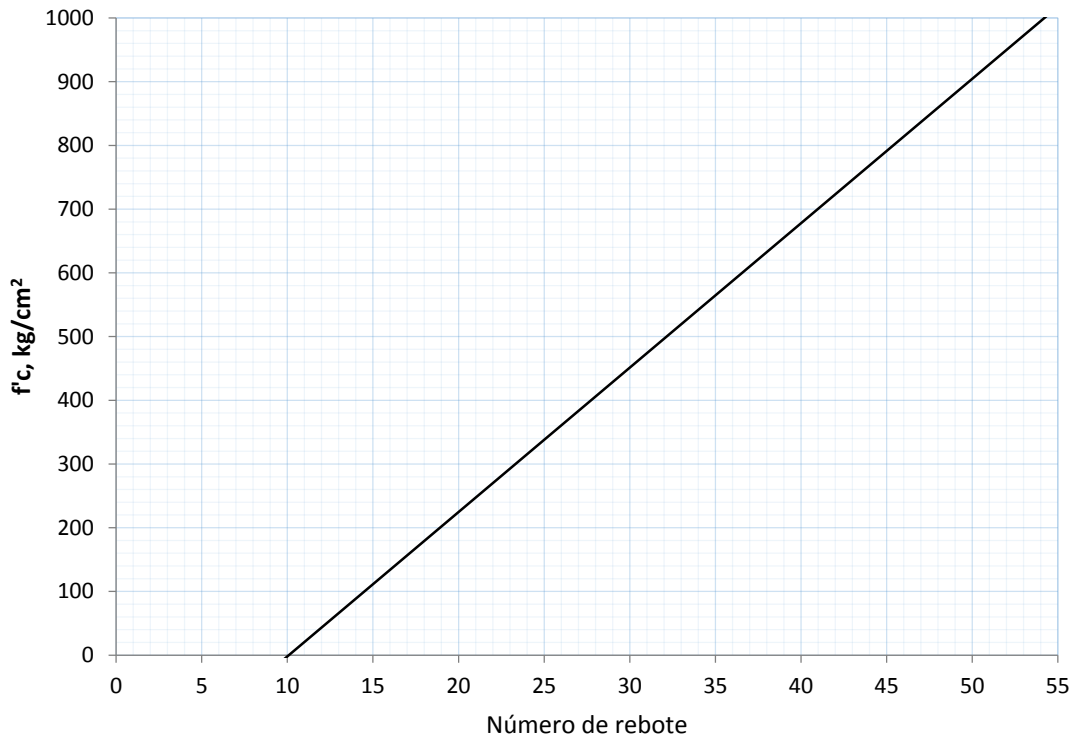
Figura 5.6 Relación entre el número de rebote y la resistencia a compresión simple a 28 y 91 días de edad
