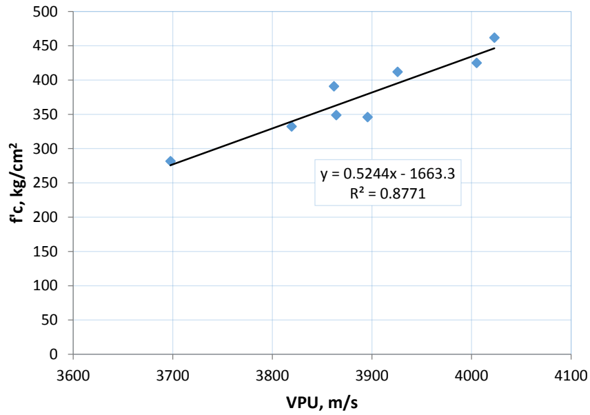
Figura 5.7 Tendencia entre la VPU y la resistencia a compresión simple a 28 días de edad
