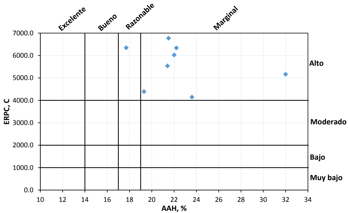
Figura 5.23 Relación entre VVP y el ERPC a 28 días de edad
