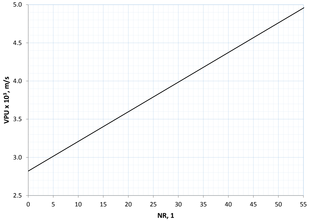
Figura 5.14 Relación entre el número de rebote y la VPU a 28 días de edad
