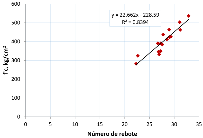
Figura 5.5 Tendencia entre el número de rebote y la resistencia a compresión simple a 28 y 91 días de edad
