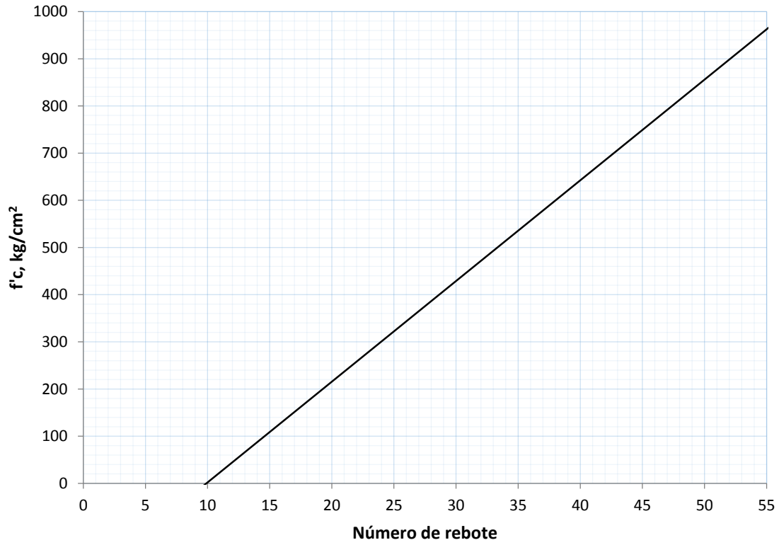
Figura 5.2 Relación entre el número de rebote y la resistencia a compresión simple a 28 días de edad
