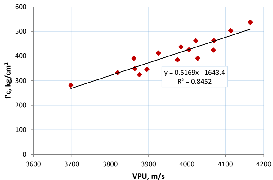
Figura 5.11 Tendencia entre la VPU y la resistencia a compresión simple a 28 y 91 días de edad
