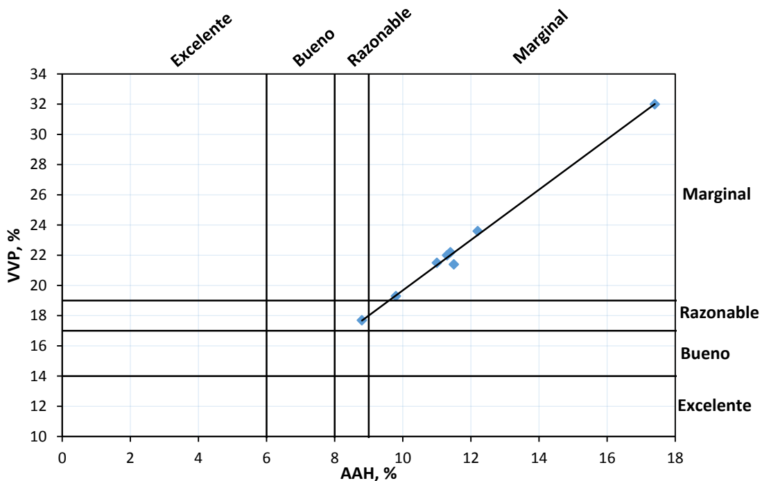
Figura 5.19 Relación entre AAH y VVP a 28 días de edad.
