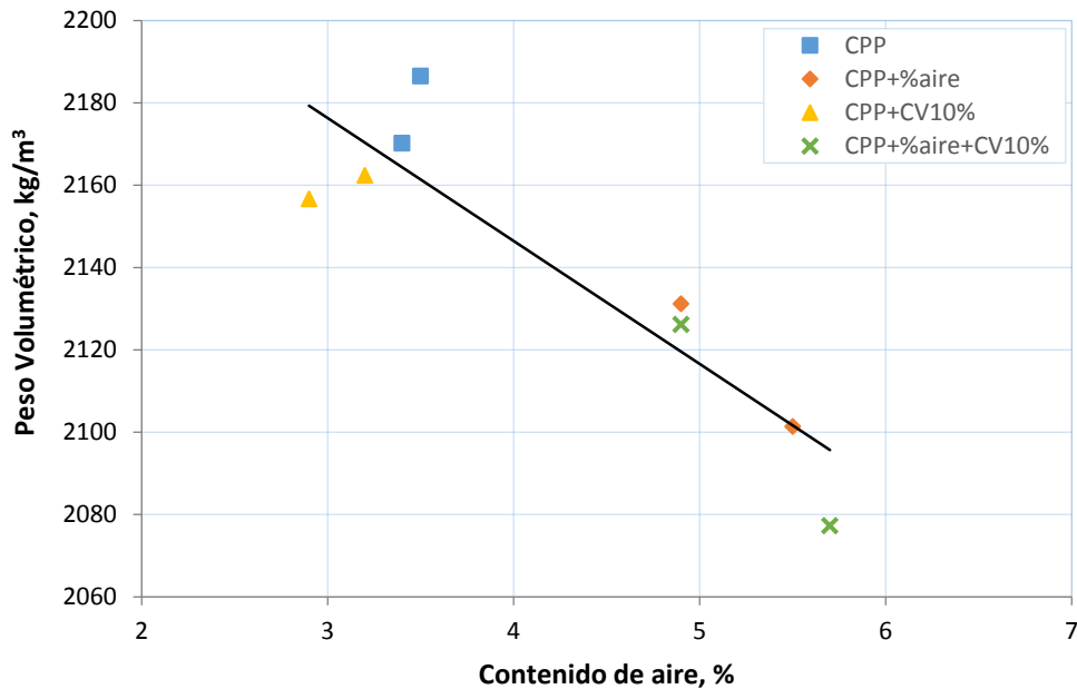
Figura 4.1 Variación del peso volumétrico con el contenido de aire.
