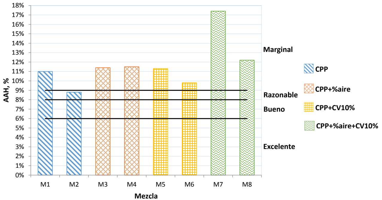
Figura 4.13 AAH a 28 días de edad.
