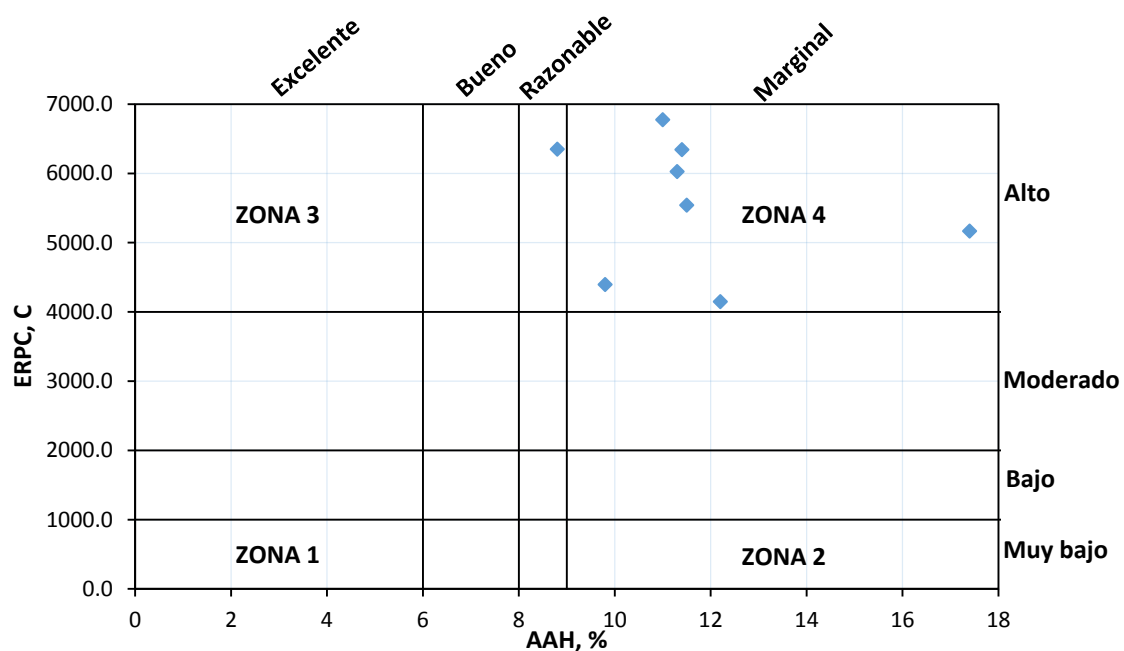
Figura 5.21 Relación entre AAH y ERPC a 28 días de edad
