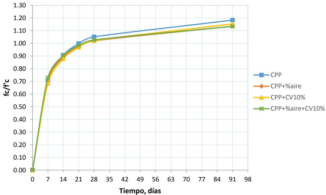
Figura 4.6 Variación promedio de la resistencia a compresión simple relativa respecto a la edad
