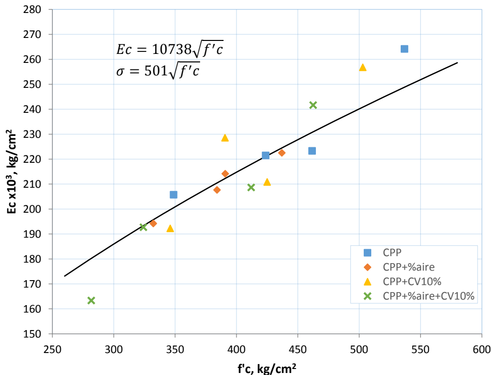
Figura 4.7 Relación entre módulo de elasticidad y resistencia a compresión simple.
