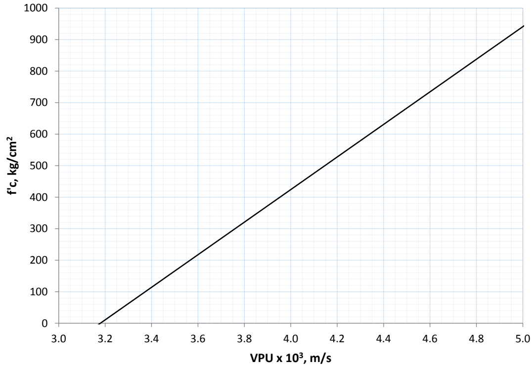
Figura 5.12 Relación entre VPU y resistencia a compresión simple a 28 y 91 días de edad
