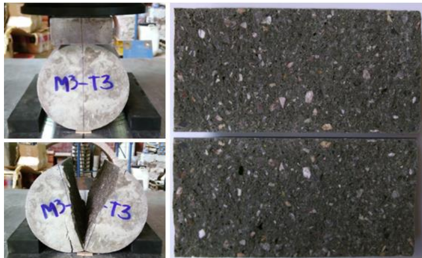
Figura 3.10 Configuración y forma de falla del espécimen en el ensaye de resistencia a tensión por compresión diametral. El espécimen que se muestra corresponde a la mezcla “M3”, con un consumo de cemento de 400 kg/m 3 y aire incluido (4.9%).
