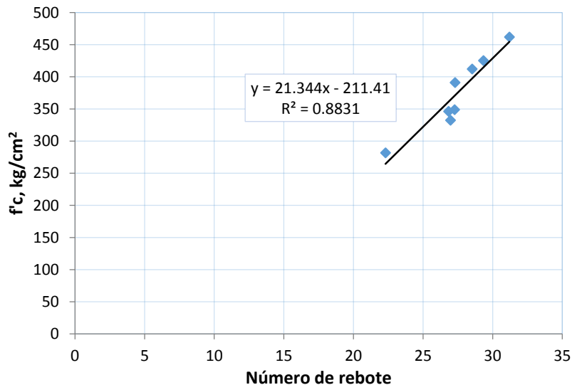
Figura 5.1 Tendencia entre número de rebote y resistencia a compresión simple a 28 días de edad
