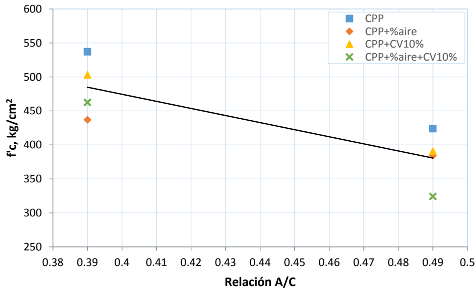
Figura 4.4 Variación de la resistencia a compresión a 91 días de edad con la relación a/c
