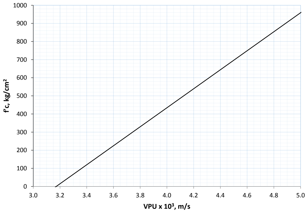
Figura 5.8 Relación entre la VPU y resistencia a compresión simple a 28 días de edad
