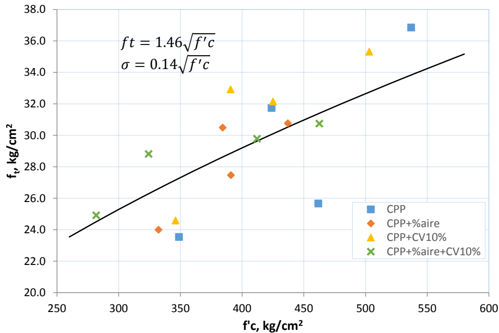
Figura 4.10 Relación entre la resistencia a tensión por compresión diametral y la resistencia a compresión simple
