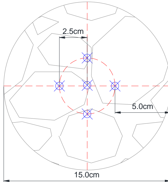
Figura 3.3 Distribución de puntos de aplicación del esclerómetro en la superficie de aplicación (extremos del cilindro).
