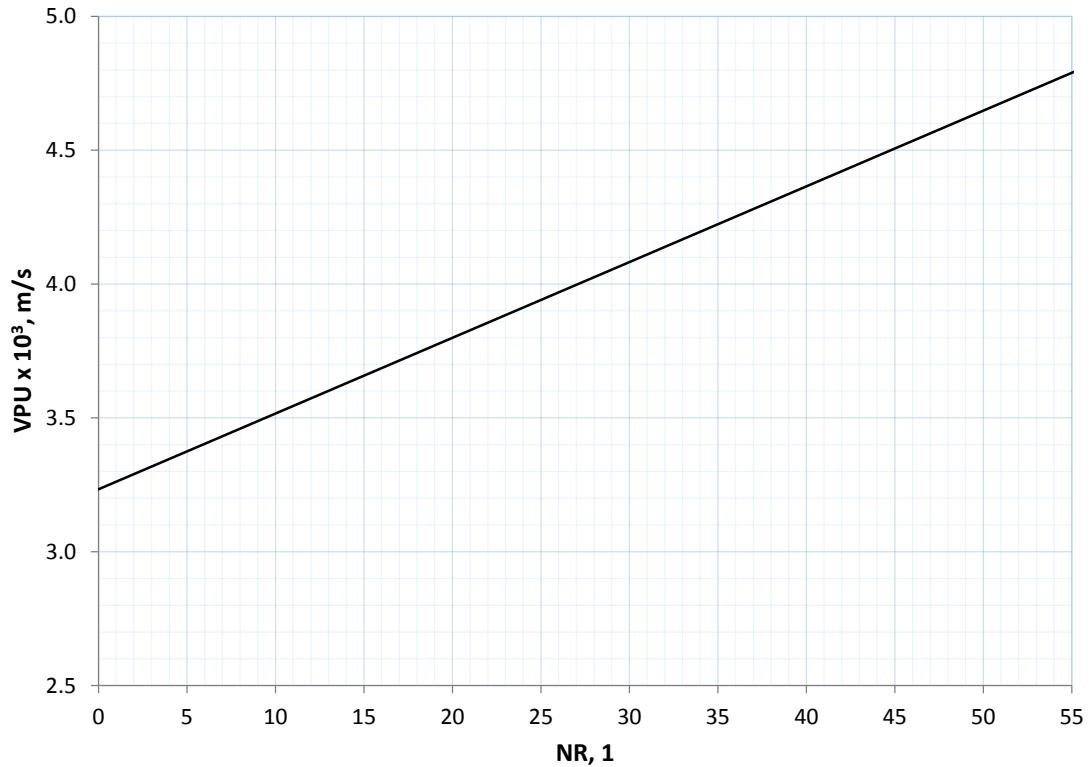
Figura 5.16 Relación entre el número de rebote y la VPU a 91 días de edad
