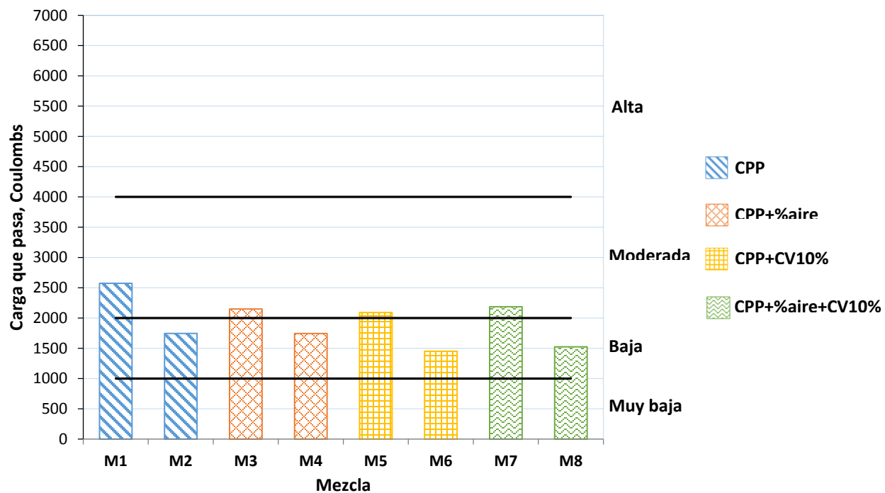
Figura 4.12 Penetrabilidad del ion cloruro a 91 días de edad
