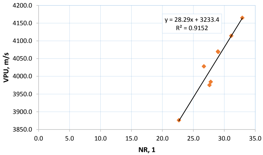
Figura 5.15 Tendencia entre el número de rebote y la VPU a 91 días de edad
