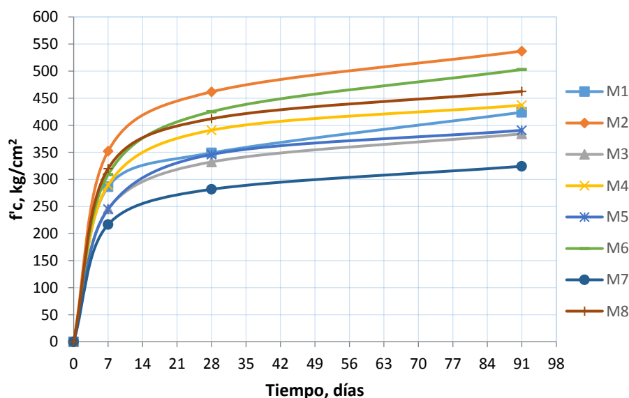
Figura 4.2 Evolución de la resistencia a compresión simple con la edad.
