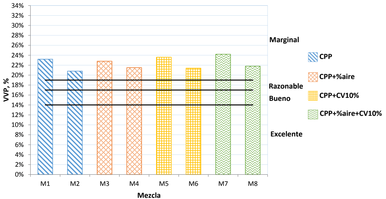
Figura 4.16 VVP a 91 días de edad
