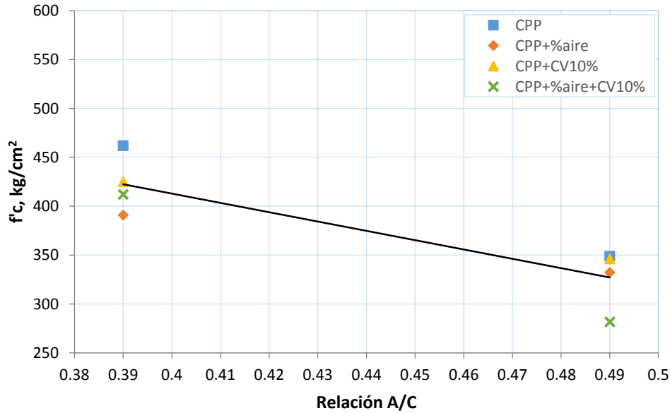
Figura 4.3 Variación de la resistencia a compresión a 28 días de edad con la relación a/c.
