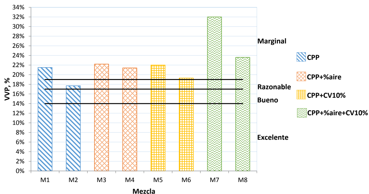
Figura 4.14 VVP a 28 días de edad
