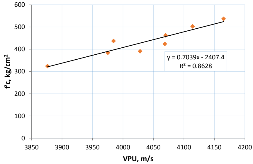
Figura 5.9 Tendencia entre VPU y resistencia a compresión simple a 91 días de edad
