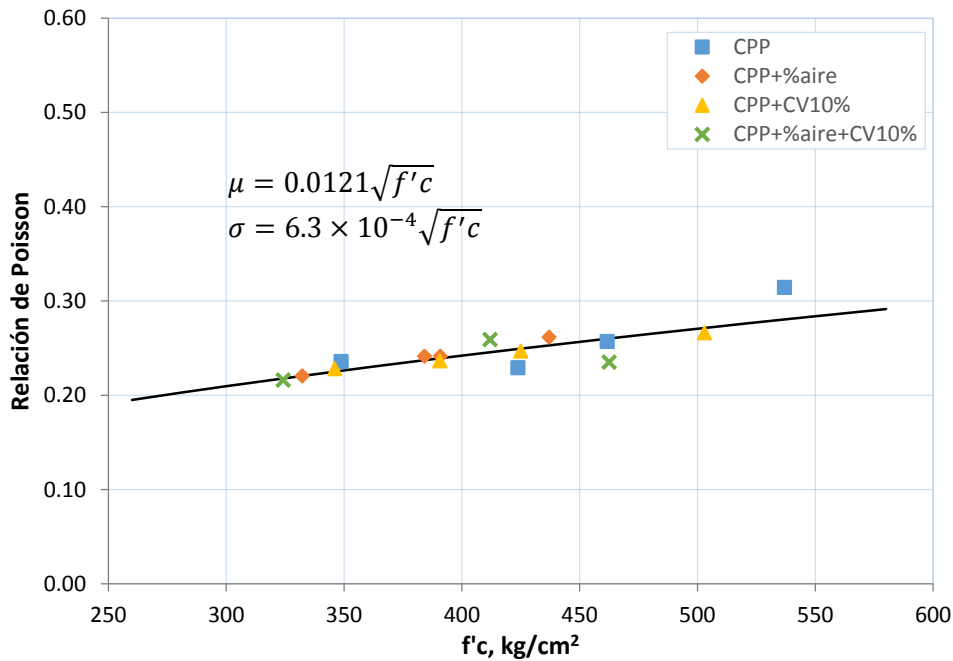
Figura 4.9 Variación de la relación de Poisson con la resistencia a compresión simple
