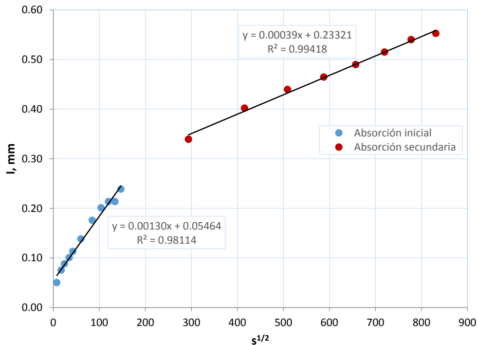
Figura 3.15 Ejemplo de cálculo de la velocidad de absorción primaria y secundaria de un espécimen de la mezcla “M6”, con un consumo de 400 kg/m 3 de cemento y una sustitución parcial con ceniza volante de 10%.
