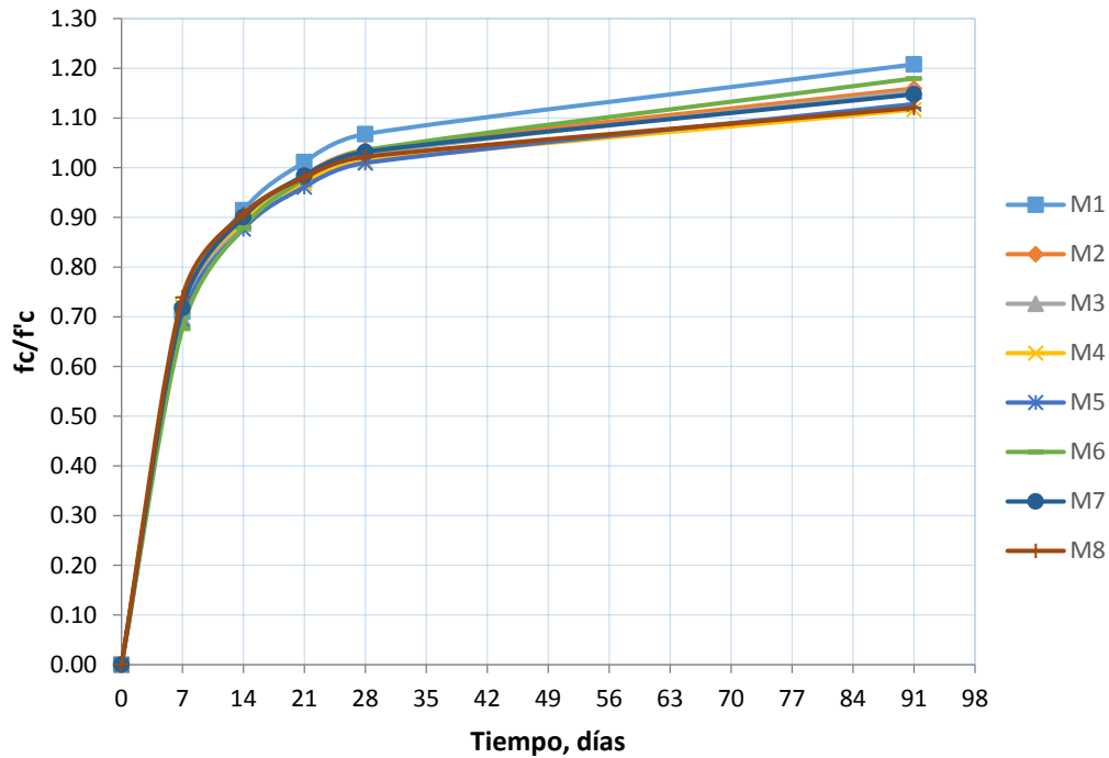
Figura 4.5 Variación de la resistencia a compresión simple relativa respecto a la edad
