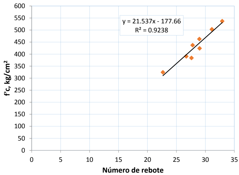
Figura 5.3 Tendencia entre número de rebote y resistencia a compresión simple a 91 días de edad
