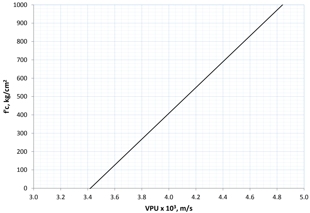
Figura 5.10 Relación entre VPU y resistencia a compresión simple a 91 días de edad
