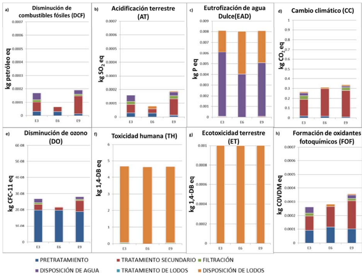
Figura 7.1 Comparación de impactos ambientales por unidad de proceso de los escenarios de los sistemas anaerobios (E3, E6 y E9) con base en la unidad funcional definida para este estudio, 1\text{m}^3 de agua residual tratada.
