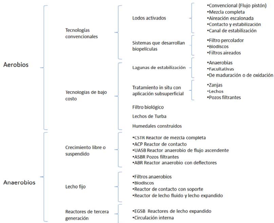
Figura 2.1 Clasificación de procesos de tratamiento biológico de agua residual. Adaptado de Metcalf & Eddy (2004).
