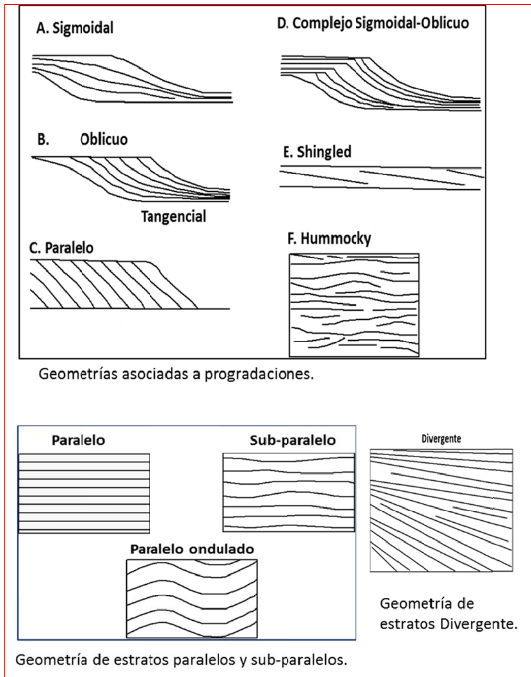
Figura IV.19. Geometría de los reflejos sísmicos.
