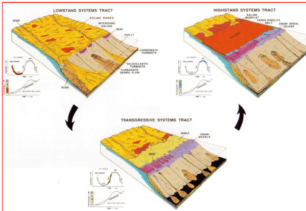
Figura III.10. Modelos sedimentarios del Lowstand, Transgresivo y Highstand para una plataforma evaporitica-siliciclastica de clima árido, Handford y Loucks, 1993.
