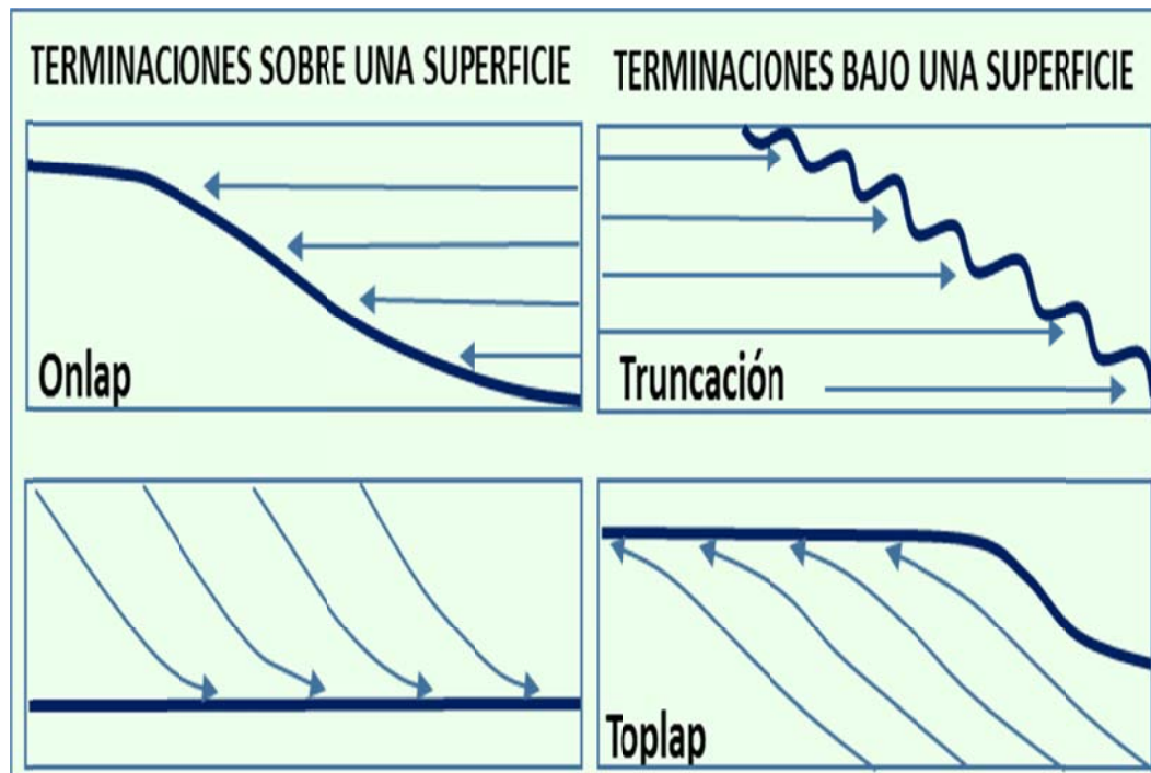
Figura IV.18. Terminación de los reflectores sísmicos.
