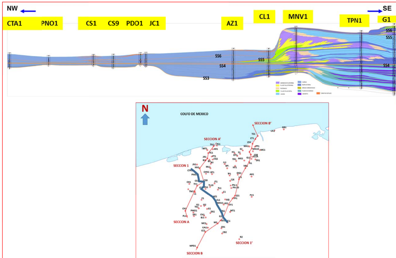
Figura IV.30. Sección estratigráfica 1-1' con interpretación de facies sedimentarias.
