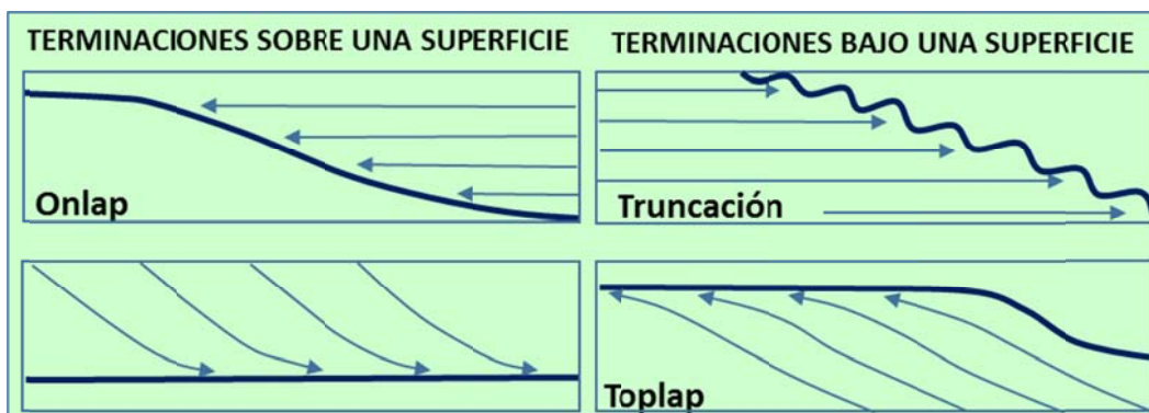
Figura III.2. Terminación de los estratos que pueden observarse arriba o debajo de una superficie estratigráfica en secciones sísmicas y en afloramientos. Mitchum y Vail, 1977.
