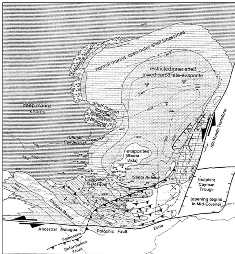
Figura II.10. Paleogeografía del Paleoceno-Eoceno Johnson et al. 1999.
