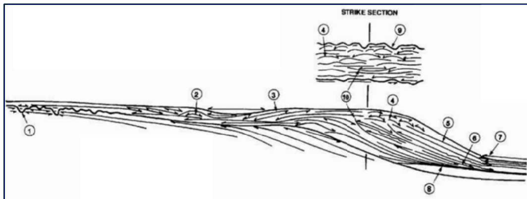
Figura III.6. Representación idealizada de los tipos comunes de los patrones de deposición de gran escala a través de las plataformas carbonatadas, muchas de las cuales son sísmicamente resoluble. Refiérase al texto para su discusión. (1) truncamiento relacionados con el Karst y relleno de onlap; (2) los montículos de la plataforma que tiene downlap en sus bases y se onlapan / downlapan en sus márgenes; (3) clinoformas de carbonato progradante a lo largo de los márgenes de sotavento de bordes de la plataforma; (4) hummocky inclinados de montículos lenticulares (biohermas a lo largo de los bordes la plataforma y en las zonas del talud; (5) talud depositacional hasta y excediendo el ángulo de reposo; (6) clinoformas con terminación downlap en el pie de talud; (7) alternancia downlap – onlap; (8) clinoformas que pueden simplemente converger por adelgazamiento; (9) Valles de incisión sobre la plataforma como límite de secuencia o sin secuencia(10).
