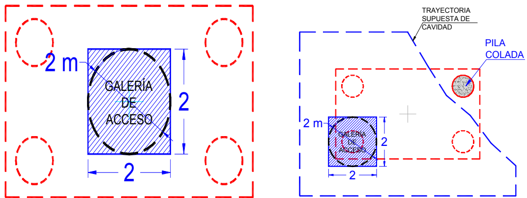
Figura 71. Galería de Acceso. Pilas en Zona Minada
