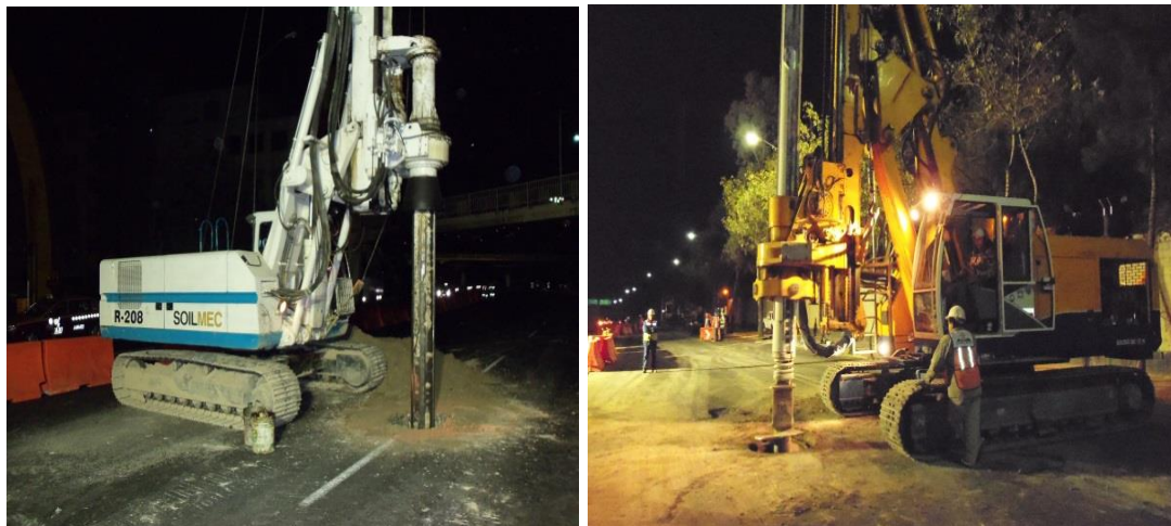
Figura 9. Perforación de pilas AUN y AUS.
