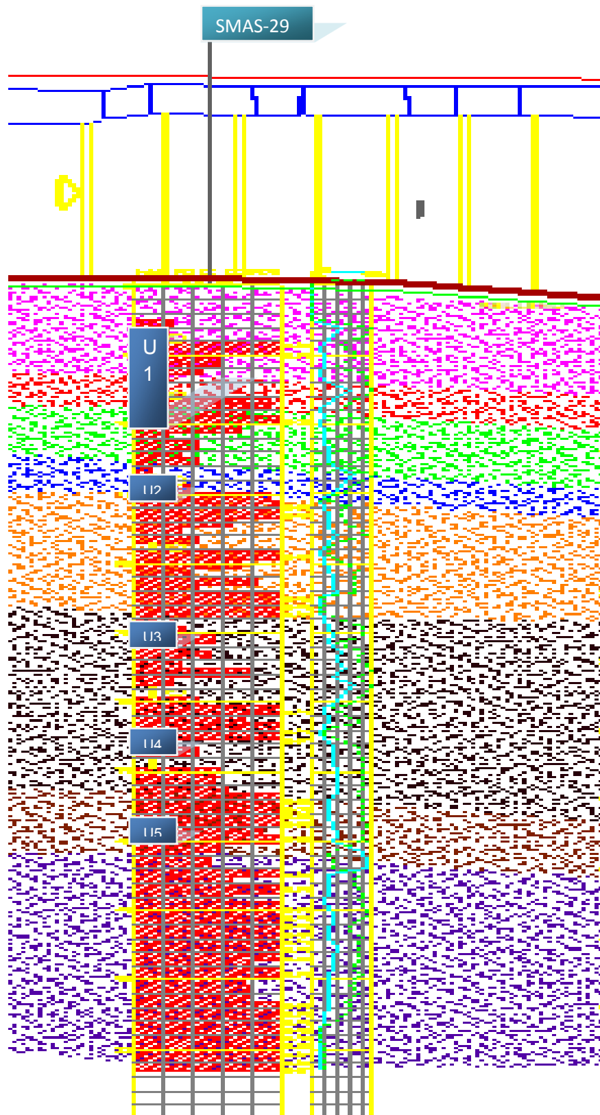
Figura 54. Zonificación geotécnica. Pilas Oblongas - Zona II
