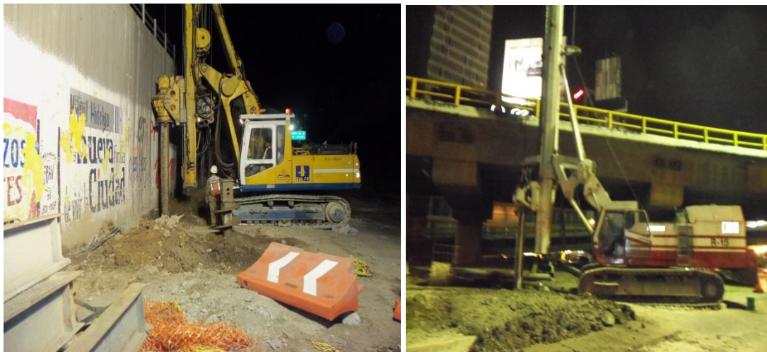
Figuras 37 y 38 .Equipos de perforación de rotación de barretón tipo kelly. Pilas en Arena
