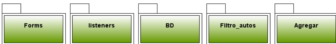
Figura 5.21. Interfaz gráfica
