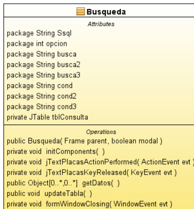
Figura 5.26. Clase búsqueda
