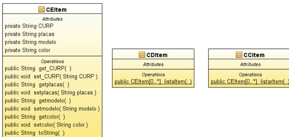
Figura 5.34. Filtro Auto
