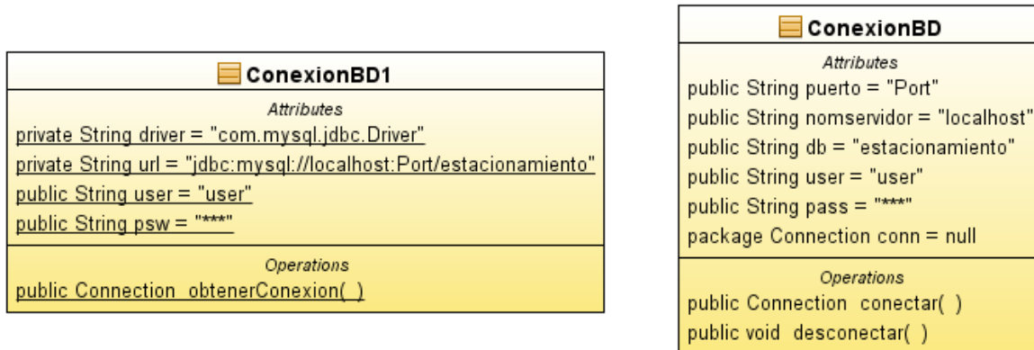
Figura 5.33. BD
