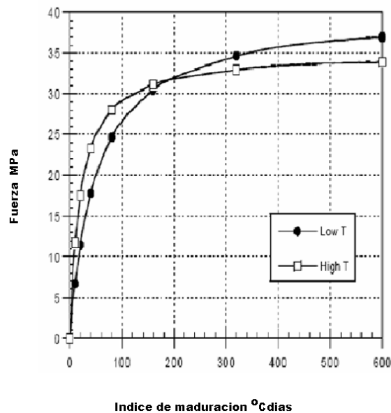
Figura. A.1 El efecto de cruce o crossover, debido a diferentes temperaturas de envejecimiento o maduración del concreto durante el desarrollo de la relación fuerza-madurez.
