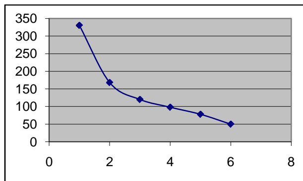
Figura. 4.20 En ésta grafica se aprecia el comportamiento de una mezcla de mortero; se tiene la intensidad de la señal contra las horas transcurridas bajo el haz de microondas.
