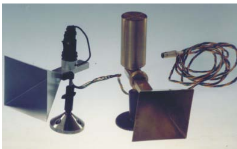
Figura. A.5.6 Fotografía de antenas piramidales con montura para oscilador
