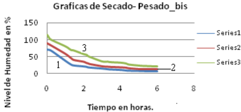
Figura 4.28. Grafica resultante del proceso pesado-secado-pesado aplicado a cada una de las muestras de concreto.
