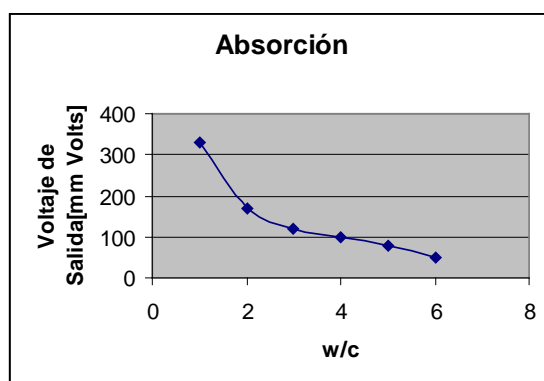
Figura. A.5.7 Dibujo de la respuesta que presenta la muestra cuando su nivel de humedad es modificado.
