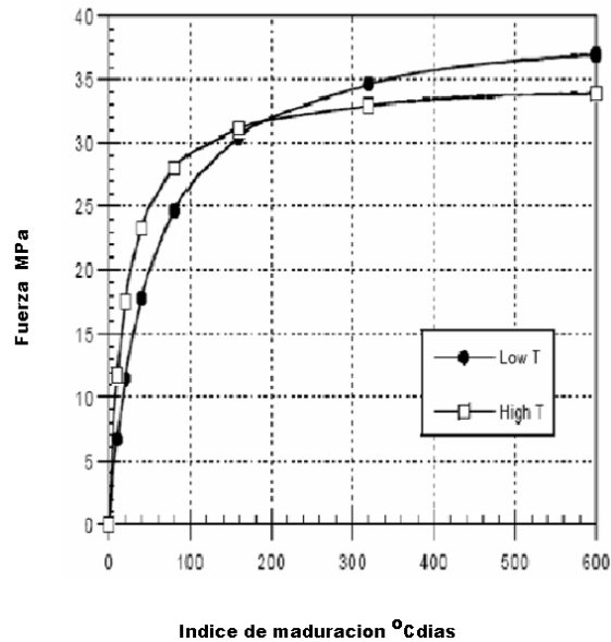
Figura.4.23 El efecto de cruce o crossover, debido a diferentes temperaturas de envejecimiento o maduración del concreto, durante el desarrollo de la relación fuerza-madurez.
