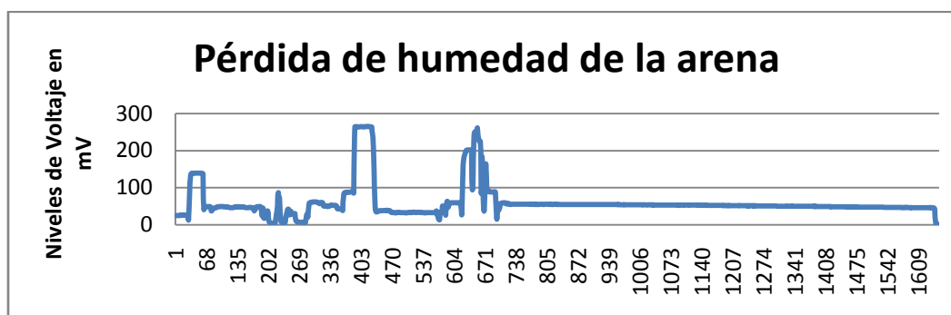
Figura. 4.19 En ésta figura se aprecia un histograma que presenta el nivel de humedad asociado con el voltaje. Es arena similar a la utilizada en las mezclas de prueba. Son niveles de voltaje contra muestras por segundo.
