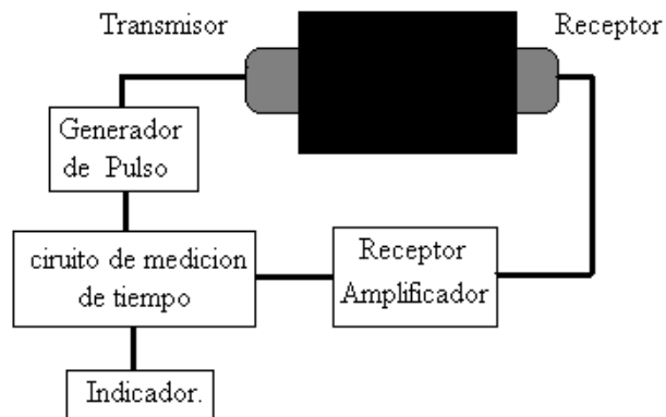
Figura 2.1 Dibujo de un arreglo básico de aplicación de pulso ultrasónico en un bloque de concreto.
