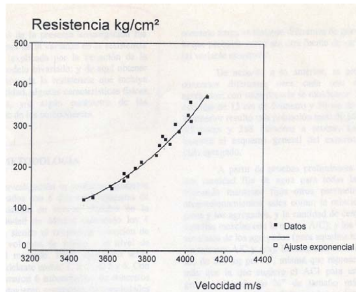
Figura 4.3. Datos y curva de ajuste velocidad-resistencia para un concreto preparado con materiales de una región conocida. (Castellanos)
