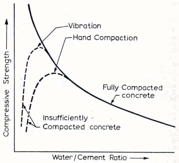
Figura 4.4 Relación entre fortaleza del concreto y la relación agua/cemento del concreto. (Neville 1963).
