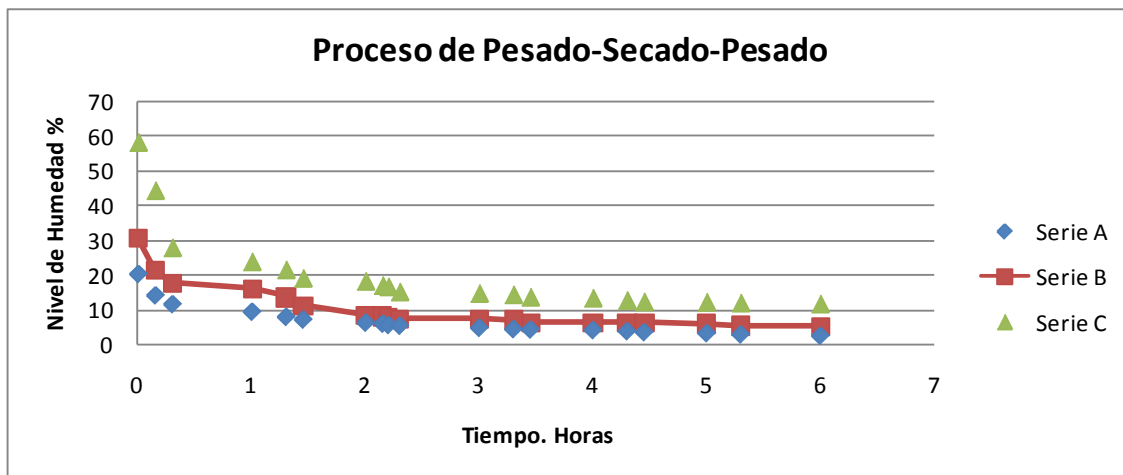
Figura 4.30. Grafica generada por los datos del proceso pesado-secado-pesado, realizado con las muestras de concreto fresco. Concreto preparado para tres posibles relaciones de agua/cemento.
