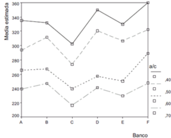
Figura 4.2. Resistencia media (Kg/cm 2 ) respecto de la relación agua/cemento y banco de procedencia. (Solis 2008)
