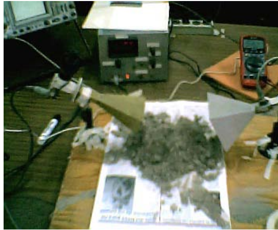
Figura. 4.14 Fotografía mostrando el equipo electrónico asociado a la generación de señales de microondas, los sensores y la interfaz del sistema datalogger
