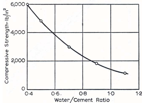
Figura 4.6 Relación entre resistencia (7 días) y la relación agua / cemento para concreto hecho con acelerante. (Neville 1963)
