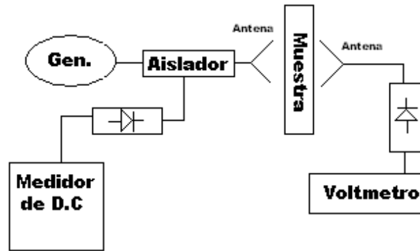
Figura. A.5.3 Diagrama de bloques de un sistema de microondas que está basado en la transmisión a través del material.
