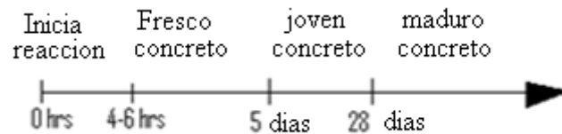
Figura 4.34. Dibujo que nos ilustra las etapas consideradas en el fraguado del concreto
