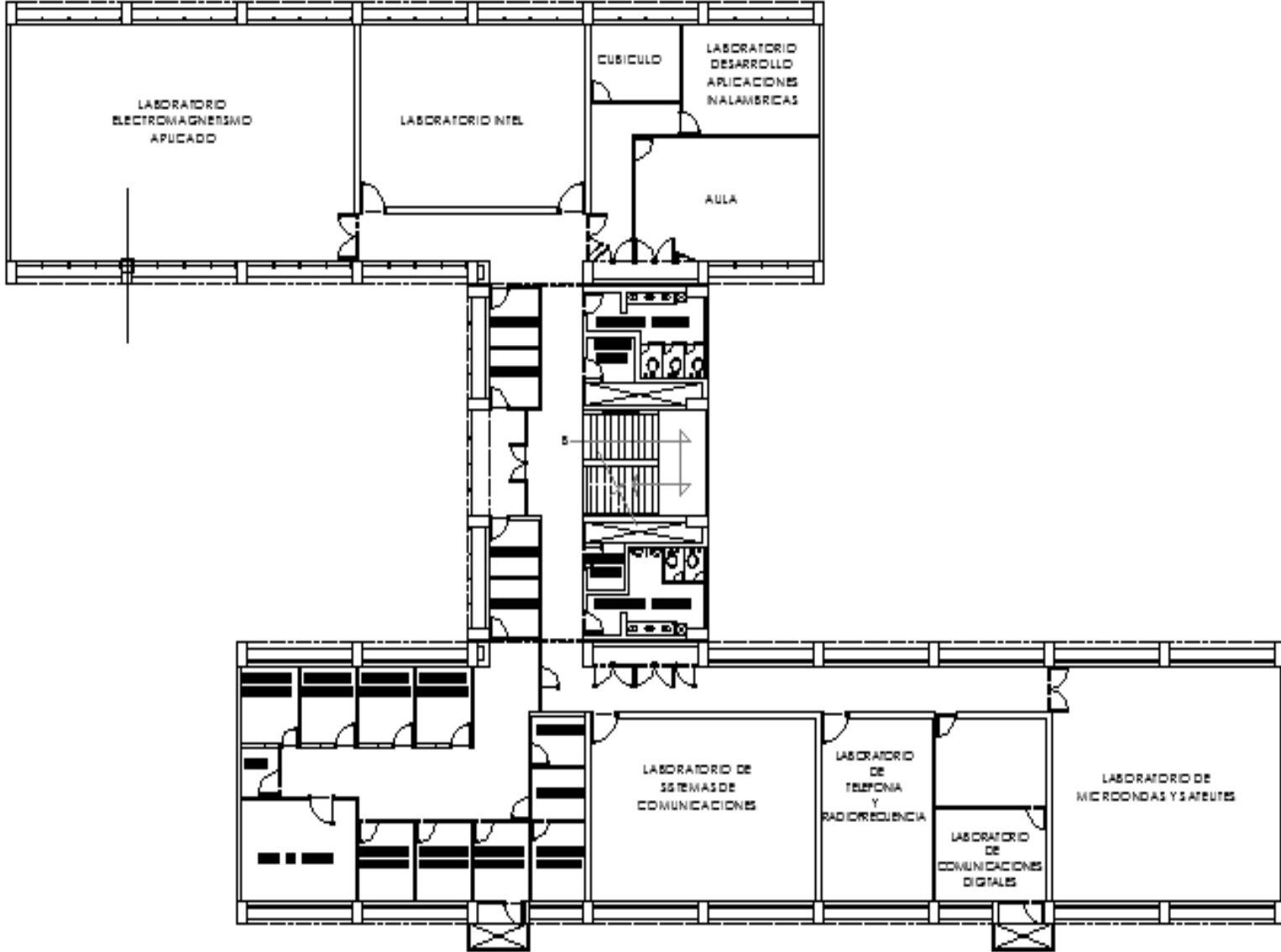
PLANTA 3er. NIVEL
