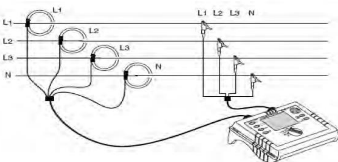
Fig. 8 Conexión de un analizador de redes
