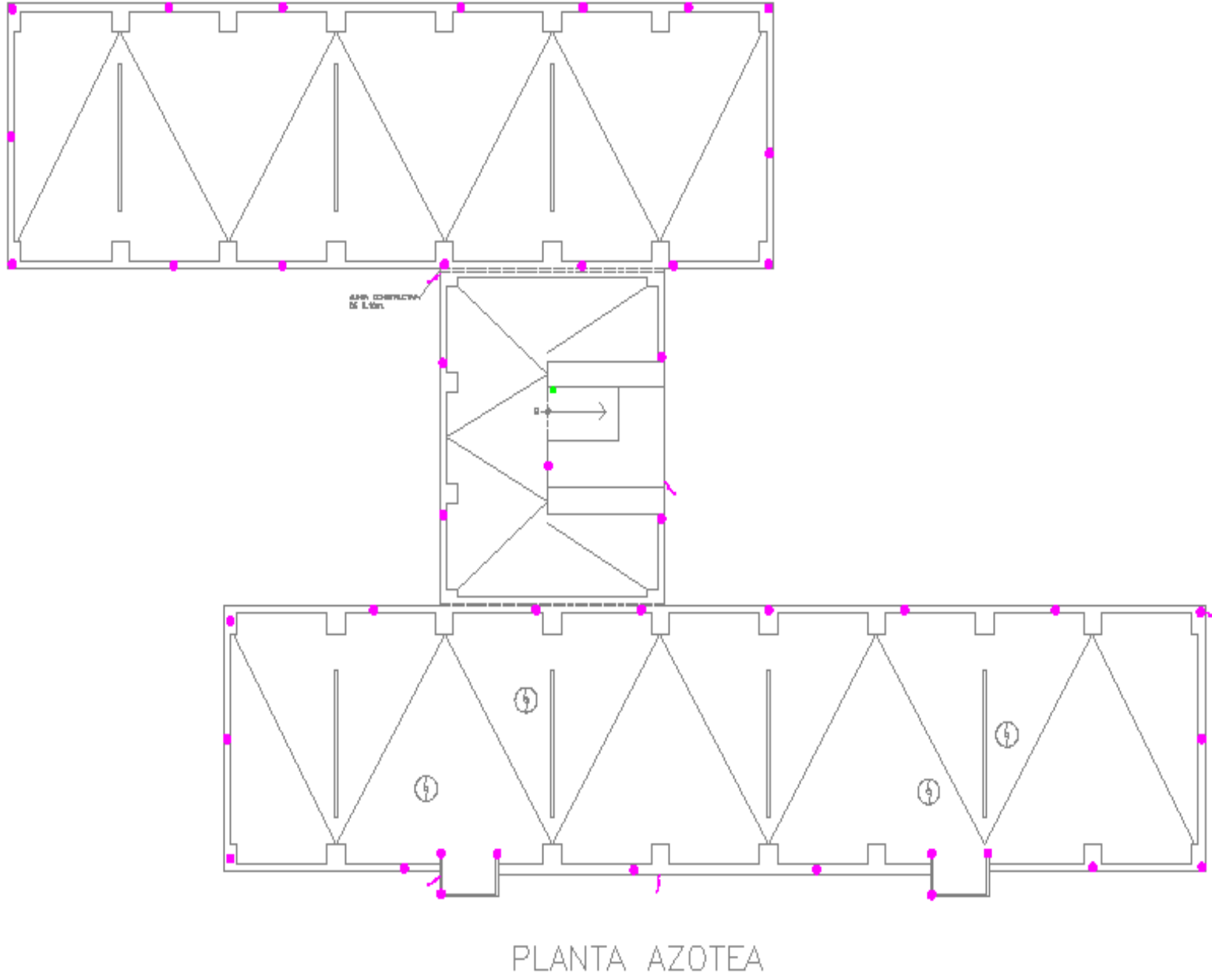
Fig. 13 Ubicación de puntas de pararrayos en la Azotea
