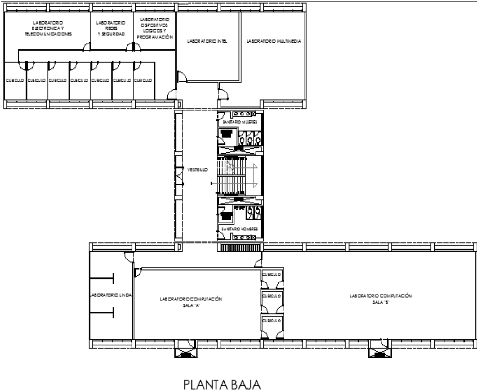
Fig. 3 Planta baja
