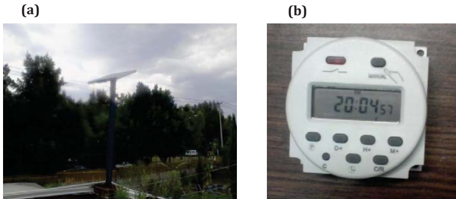
Figura 9. (a) Celda fotovoltaica ubicada en la azotea del edificio del gimnasio de la FES Zaragoza C - 2 (UNAM), (b) Temporizador digital.
