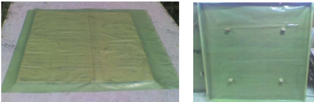
Figura 2. (a) Colocación de la primera capa de hule para impermeabilizar ambos paneles. (b) Bastidor con la segunda capa de hule y con soportes para el anclaje de la malla de contención.
