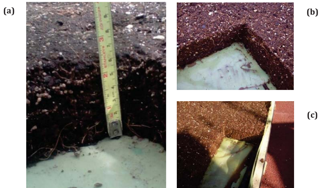
Figura 25. (a) Espesor del sustrato utilizado en ambos paneles. (b y c) Fotografías que muestran diferentes ángulos del espesor del sustrato ya montado en los paneles verticales.
