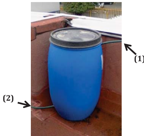
Figura 7. Vista lateral del tambo con manguera para el llenado del mismo (1) y manguera de salida, para el riego de ambos páneles verticales (2).
