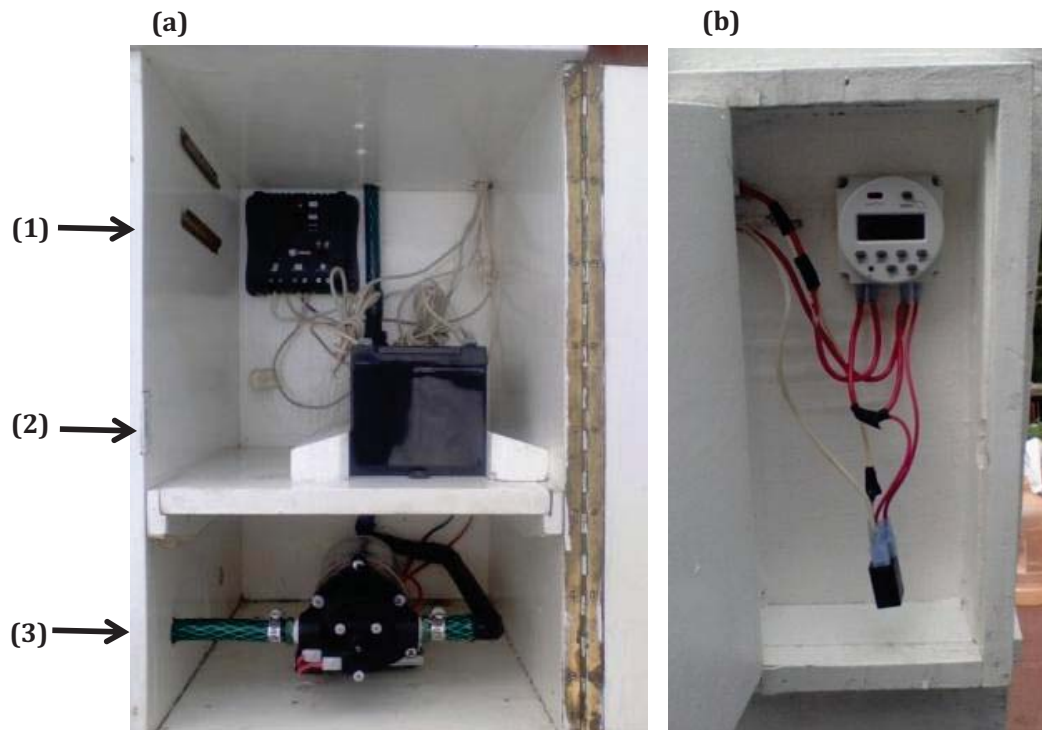
Figura 24. (a) Componentes eléctricos del sistema de riego dentro de su caja; 1.- Regulador de carga, 2 - Batería solar y 3 Bomba solar. (b) Temporizador digital dentro de su caja.
