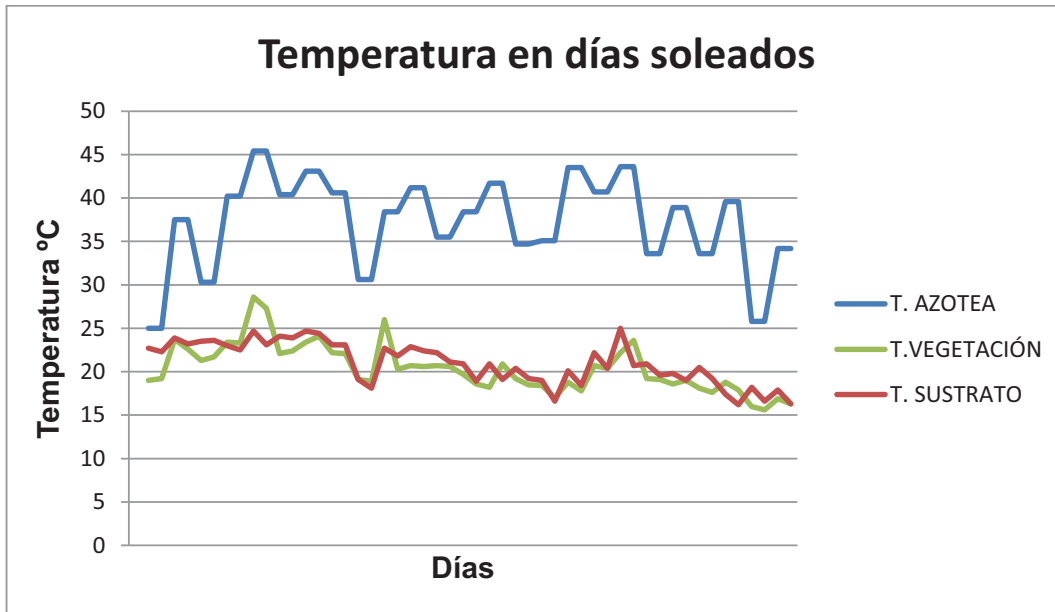
Figura 42. Oscilación de la temperatura en la azotea del gimnasio en días soleados
