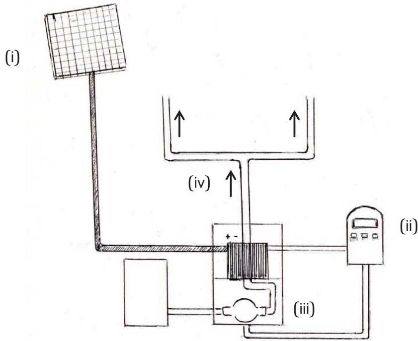
Figura 8. Diseño del sistema de energía fotovoltaica para la propulsión del agua de riego.
