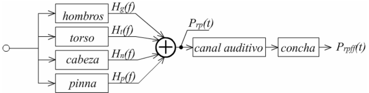
Figura 3.7. Modelo de oído mediante funciones de transferencia.
