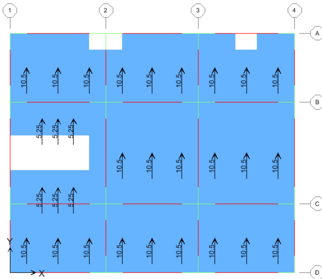
Figura 3.7 MEF Distribución de fuerzas de piso en firme con el programa ETABS.
