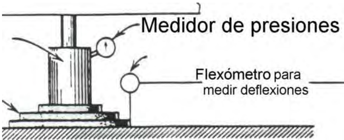
Fig.3.8.b.7 Prueba de placa en sub-base pavimento rígido.
