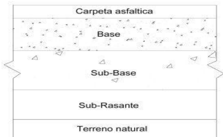
Fig.3.8.b.20 Sección de pavimento flexible.
