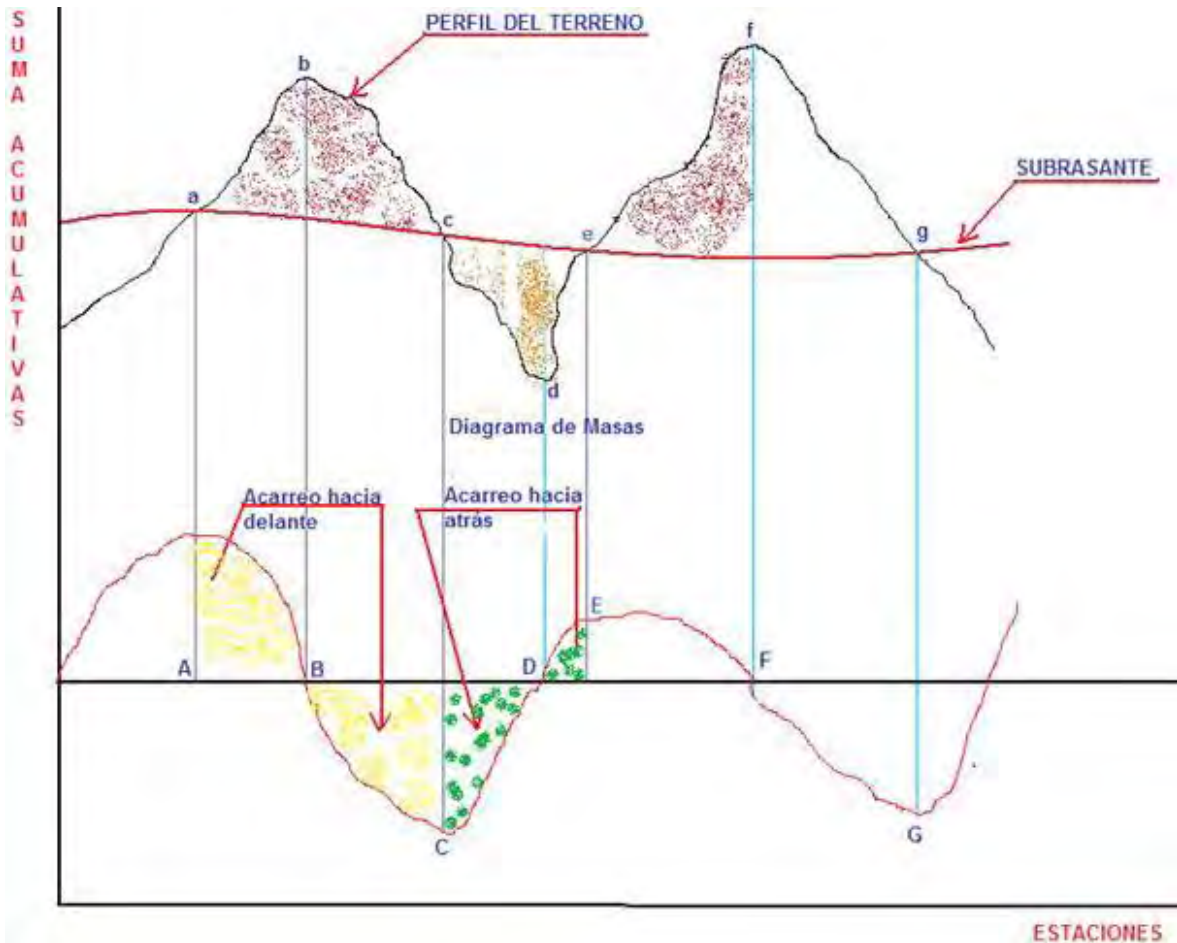
Fig. d.1 Curva Masa.
