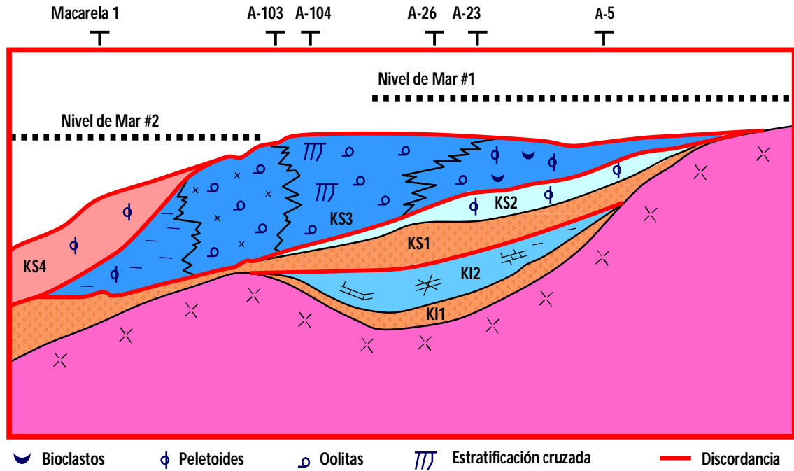
Figura 1.14 Distribución de parasecuencias en el campo Arenque (PEMEX).
