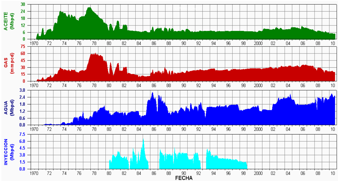
Figura 1.29 Historia de producción de Arenque y Lobina (PEP 2010).
