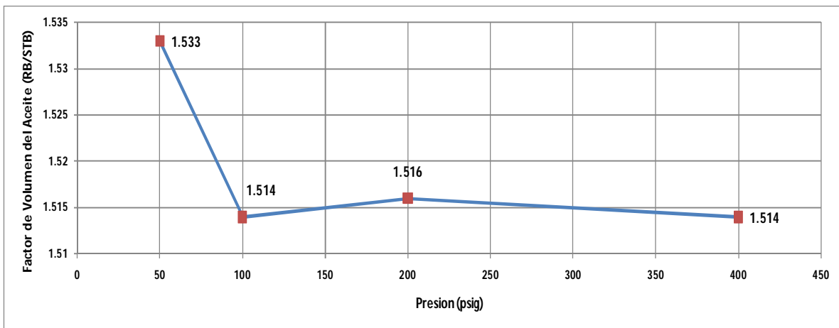
Figura 1.31 Presión óptima de separación @ 28°C, para el fluido del yacimiento Jsa bloque AI, campo Arenque (PEP 2010).
