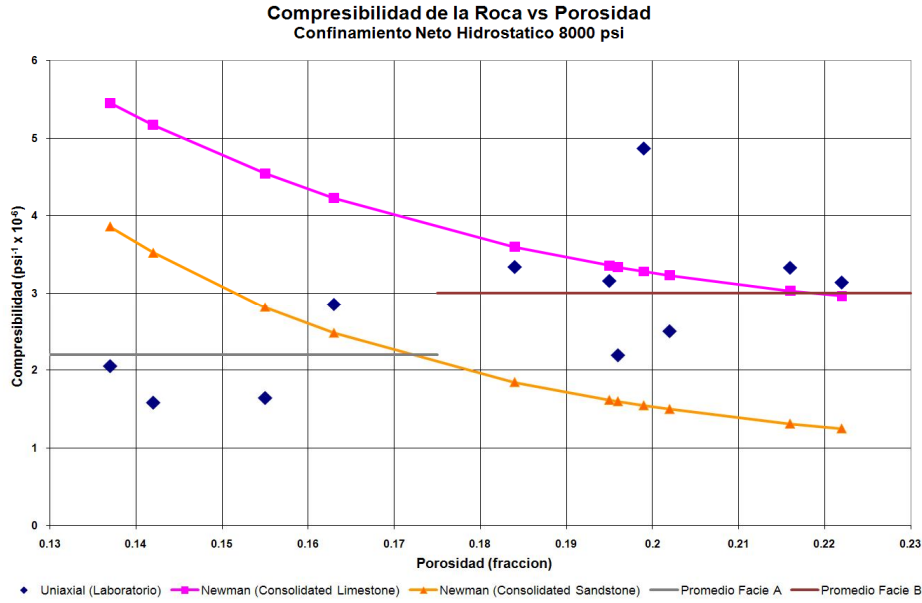
Figura 3.11 Compresibilidad de la roca del campo Arenque (PEP 2010).
