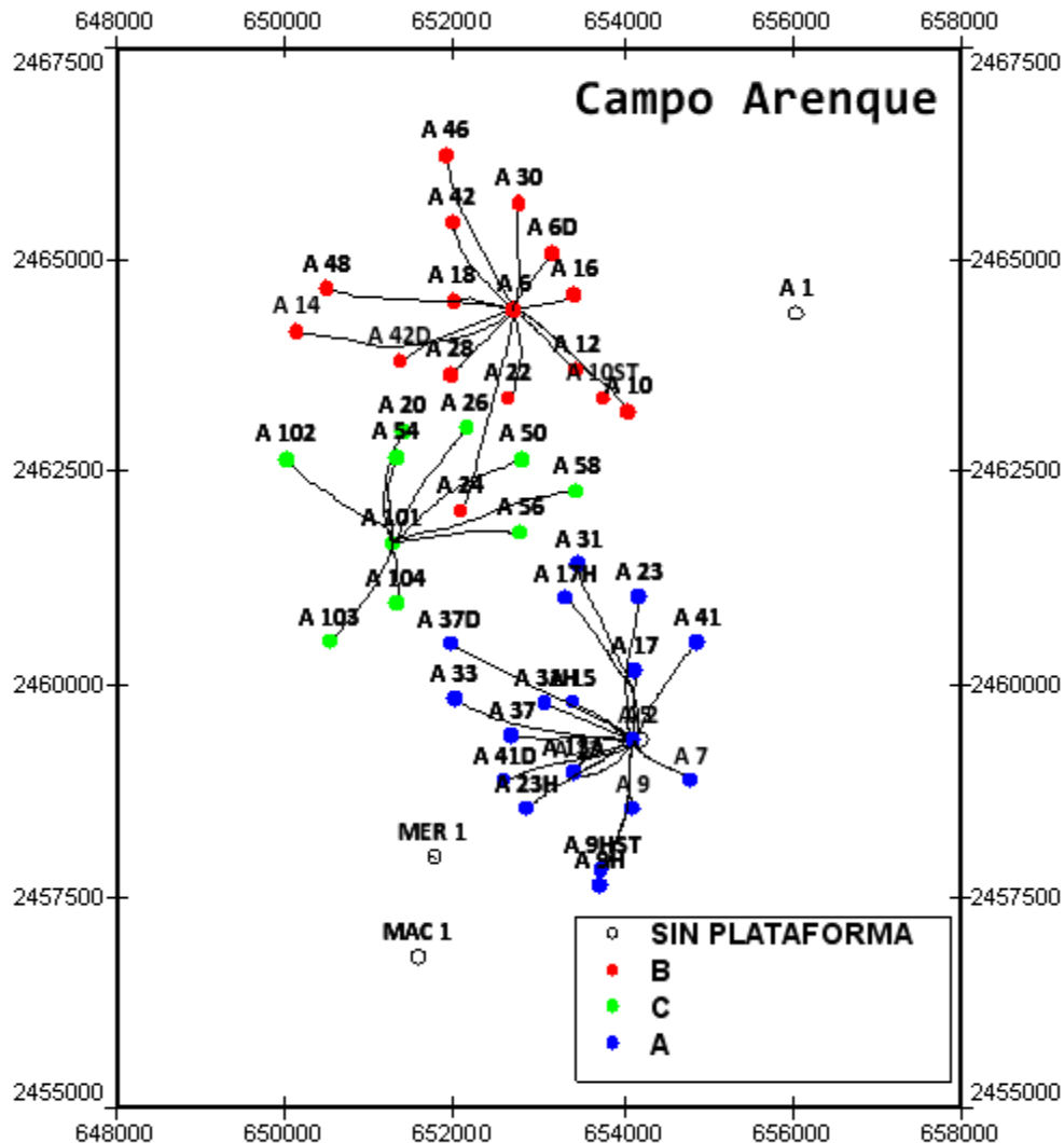
Figura 1.19 Distribución de pozos por plataforma (PEMEX).
