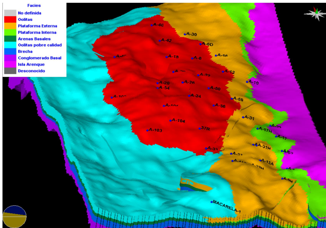
Figura 1.16 Distribución de facies en el Campo Arenque (PEMEX).
