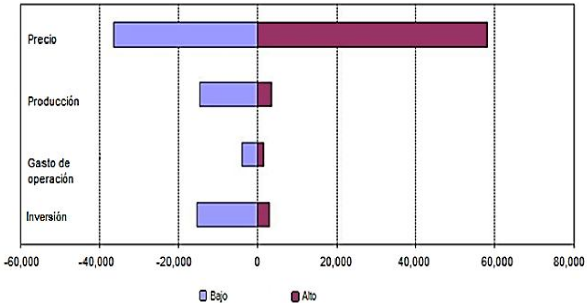
Figura 4.5 Diagrama de tornado de la opción 2
