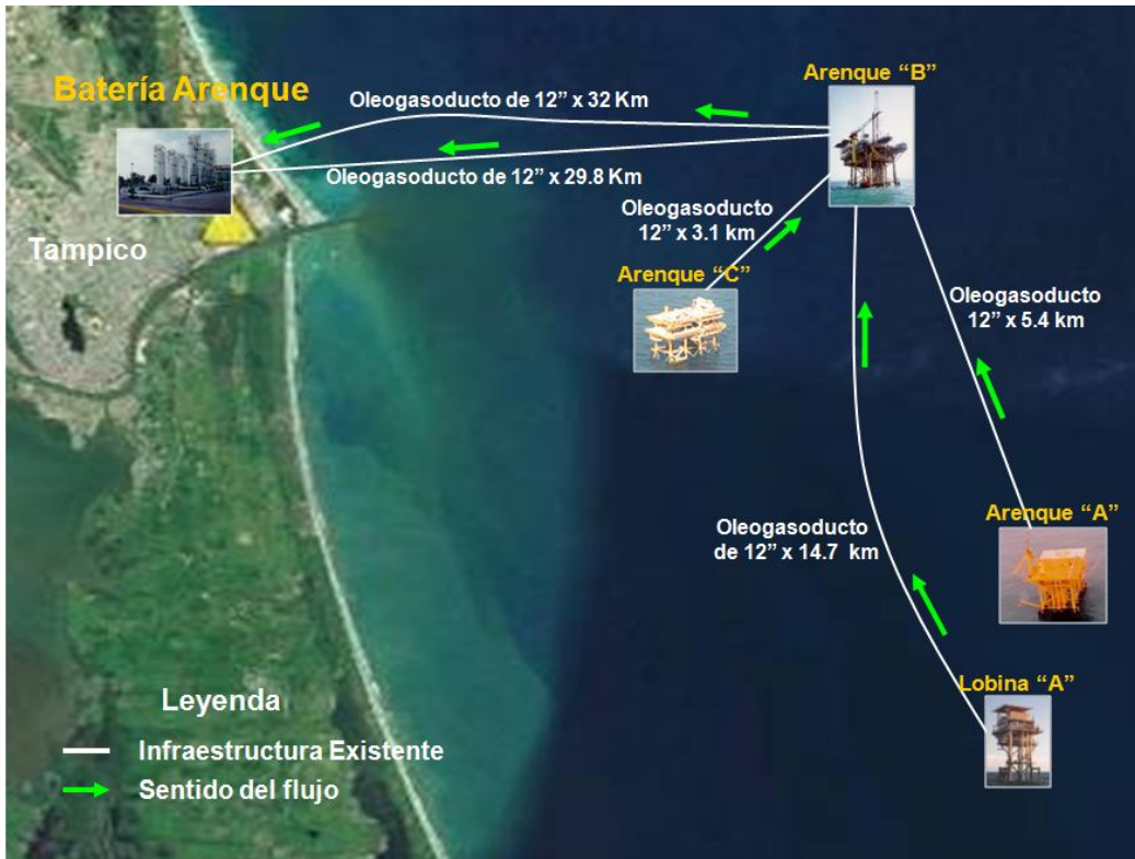
Figura 5.1 Manejo actual de la producción Arenque – Lobina. (PEP 2010).
