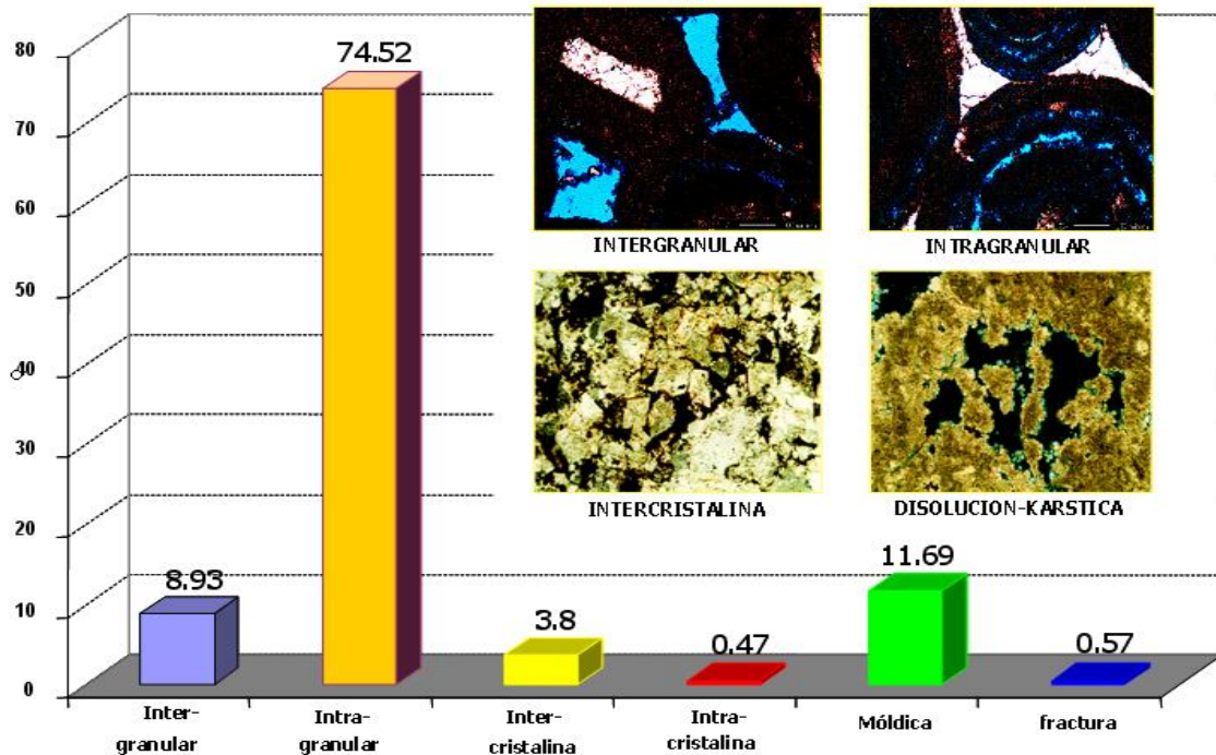
Figura 1.18 Se observa que la mayor porosidad es intragranular (PEMEX).
