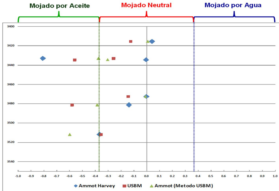
Figura 3.12 Mojabilidad de la roca (PEP 2010).
