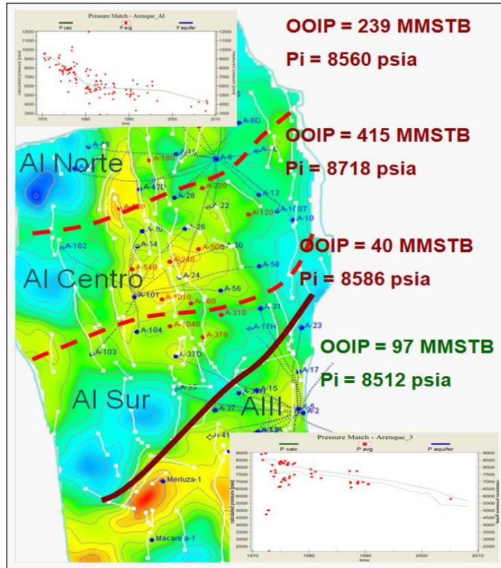
Figura 2.4 Volúmenes originales de aceite para cada una de las áreas del campo Arenque, (PEP).
