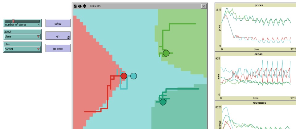
Figura 3.2: Simulación de un problema de localización empleando la ley de Hotelling usando NetLogo
