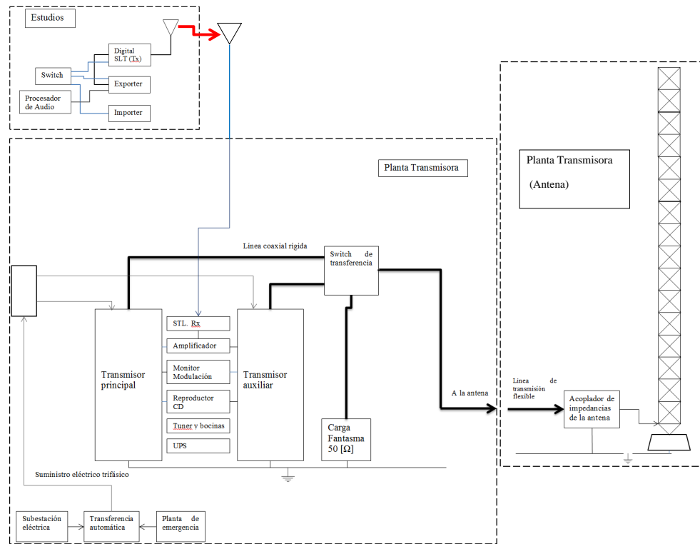
Figura 3.1: Diagrama general de la planta transmisora.
