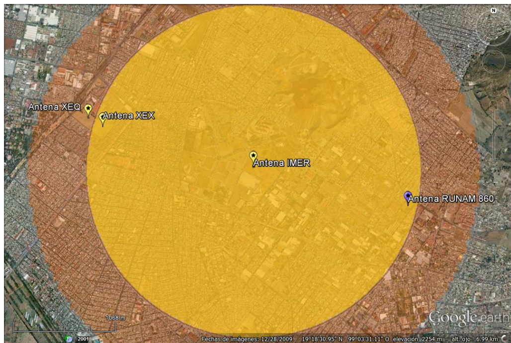
Figura 6.7: Contorno de 1[V/m] para las estaciones del IMER.
