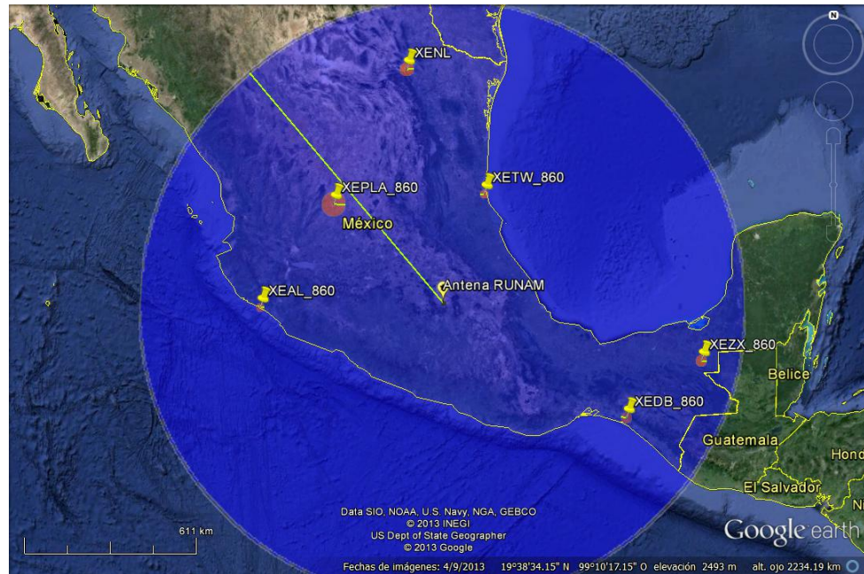
Figura 6.14: Contorno Interferente Cocanal Nocturno de Radio UNAM ( 10[kW] ) y Contornos Protegidos Cocanales Nocturnos de las demás estaciones.
