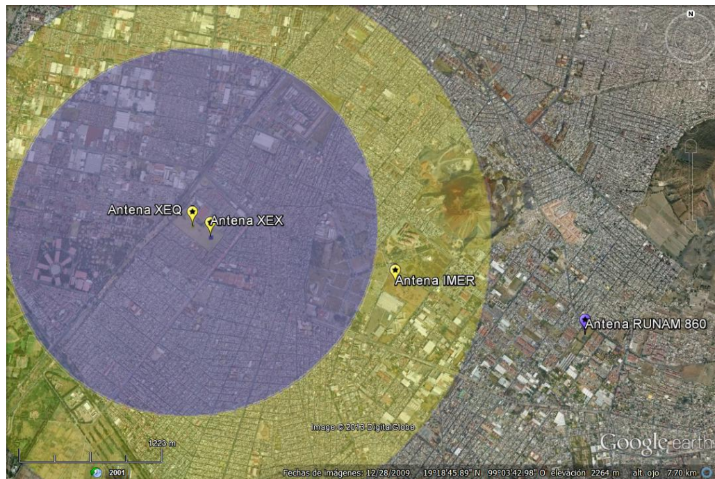
Figura 6.8: Contorno de 1[V/m] para las estaciones de la Cadena Radiodifusora Mexicana.
