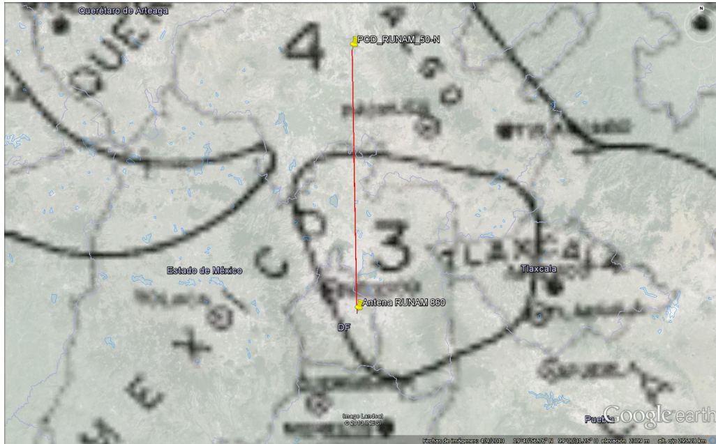
Figura B.3: Medición del alcance en dirección Norte del Contorno Protegido Cocanal Diurno de Radio UNAM (50[kW])
