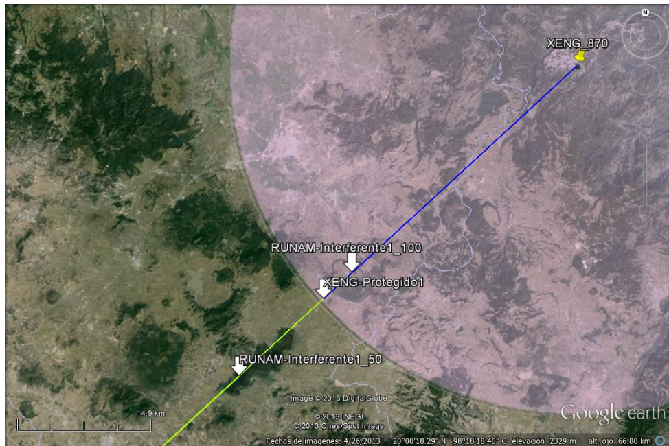
Figura 6.16: Análisis de interferencia de Radio UNAM con la estación XENG utilizando el método de Kirke.
