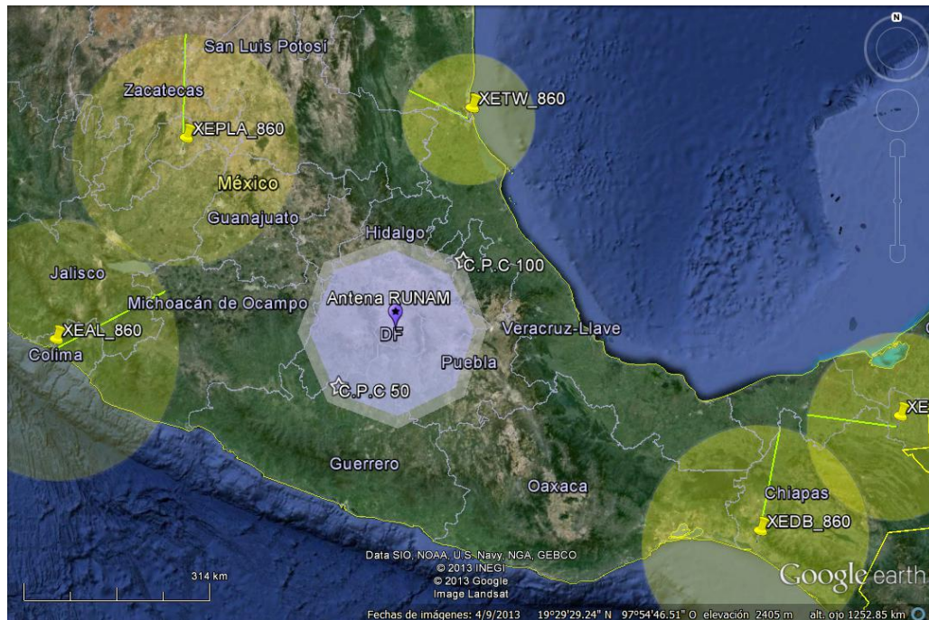
Figura 6.9: Contorno protegido cocanal diurno de Radio UNAM (50 [kW] y 100 [kW]) y contornos interferentes cocanales diurnos de otras estaciones a 860[kHz].
