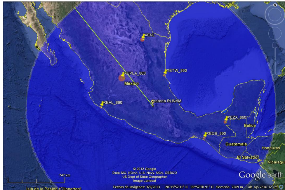
Figura 6.13: Contorno Interferente Cocanal Nocturno de Radio UNAM ( 50[kW] ) y Contornos Protegidos Cocanales Nocturnos de las demás estaciones.
