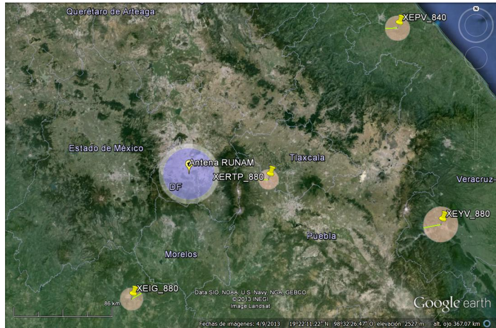
Figura 6.17: Contornos Protegidos e Interferentes del segundo canal adyacente de Radio UNAM y de las estaciones del segundo canal adyacente.
