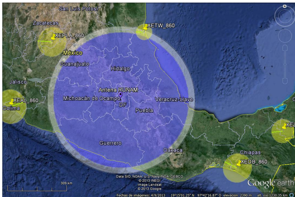
Figura 6.10: Contorno interferente cocanal diurno de Radio UNAM (50 [kW] y 100 [kW]) y contornos protegidos cocanales diurnos de otras estaciones a 860[kHz].
