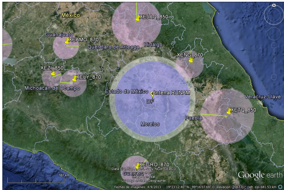
Figura 6.15: Contornos Protegido e Interferente de Radio UNAM ( 50[kW] y 100[kW] ) y de las estaciones del primer canal adyacente.
