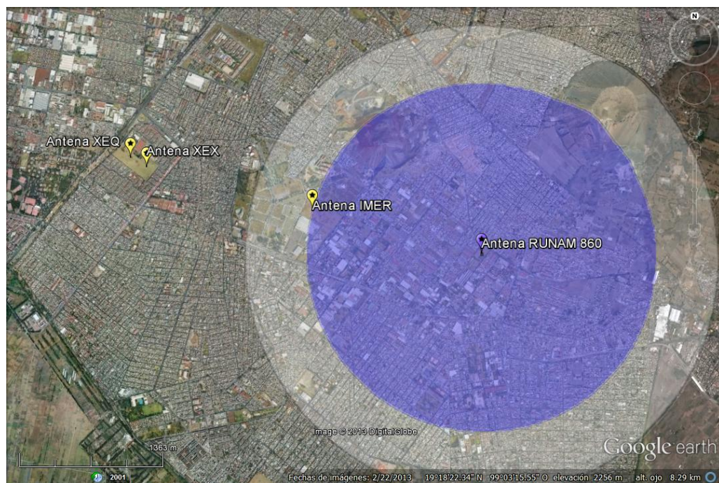
Figura 6.6: Contorno de 1[V/m] para Radio UNAM ( 50kW y 100[kW] ).
