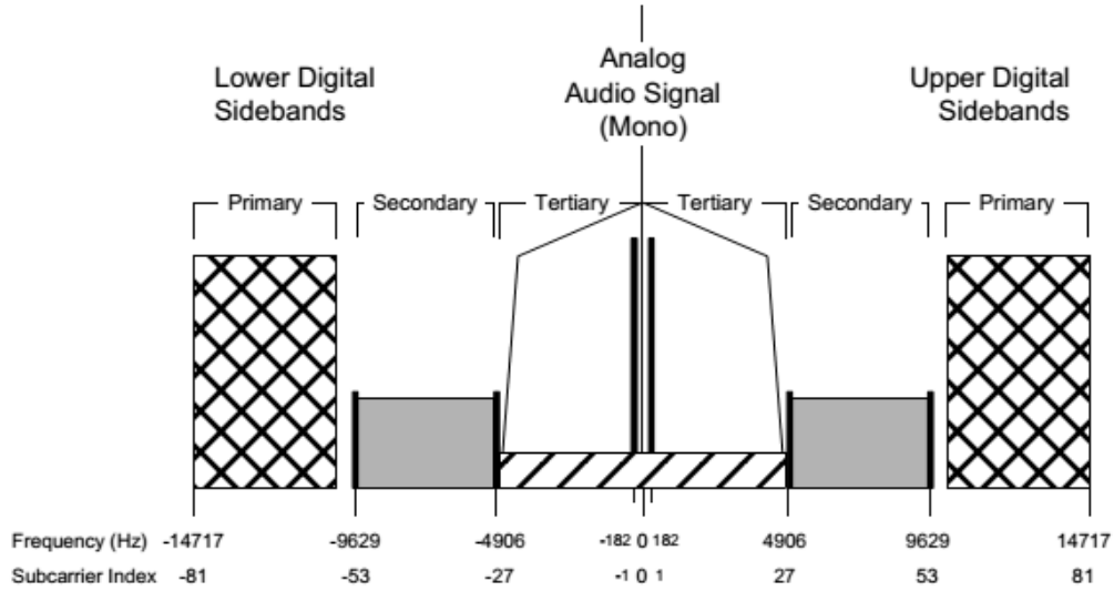
Figura 6.18: Espectro de la forma de onda híbrida de IBOC AM [21].
