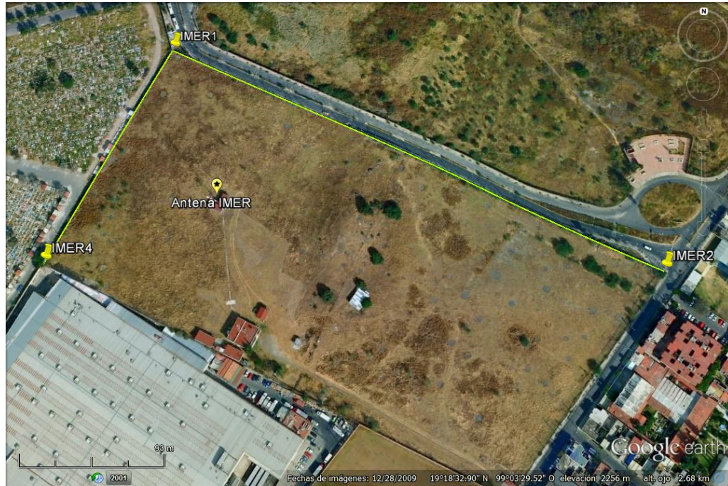
Figura 6.3: Terreno de la planta de transmisión del IMER.
