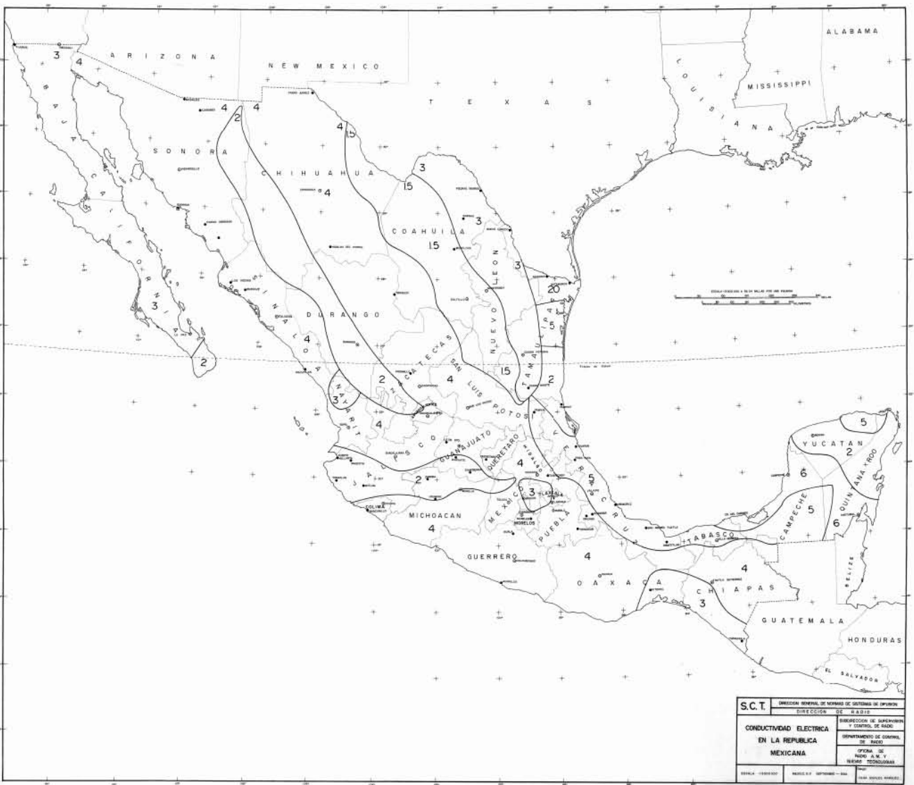
Figura E.1: Carta de Conductividad Eléctrica de la República Mexicana
