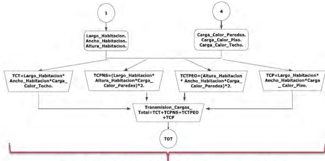
Cálculos de cargas por transmisión de las paredes, techo y piso de la nevera
