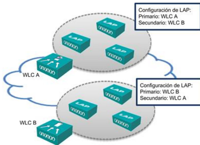
Figura 2.18 Arquitectura de redundancia N+N
