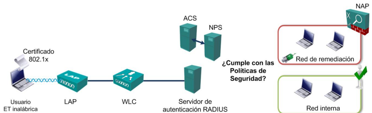
Figura 3.15 Integración de NAP en la arquitectura de red empresarial
