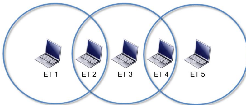
Figura 2.9 Problema de los nodos ocultos y expuestos
