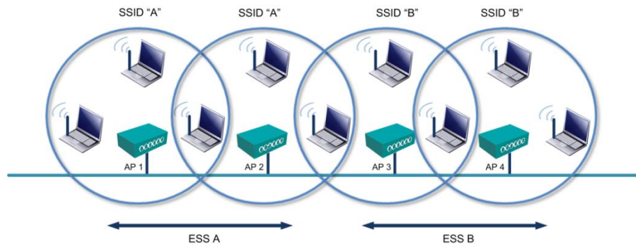
Figura 2.14 Múltiples ESS
