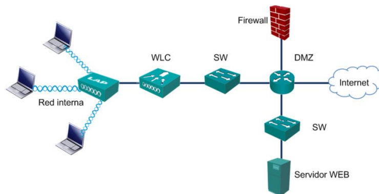
Figura 3.16 Configuración de Firewall único
