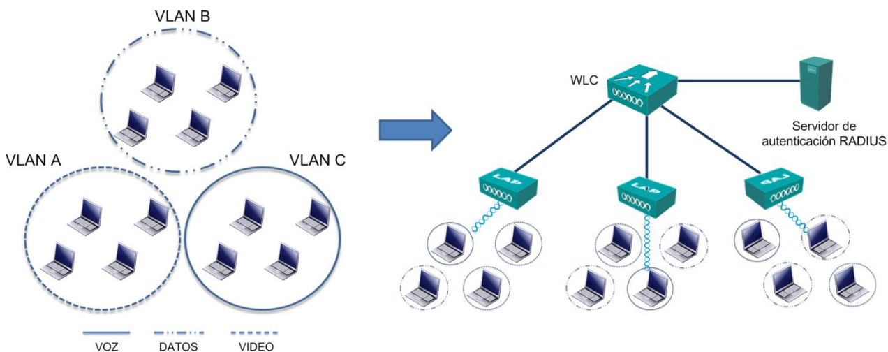
Figura 3.12 Arquitectura de configuración de VLANs
