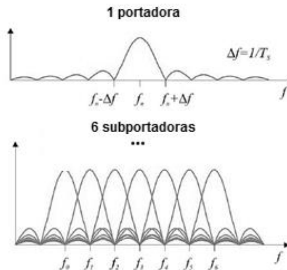
Figura 2.7 Técnica de transmisión OFDM
