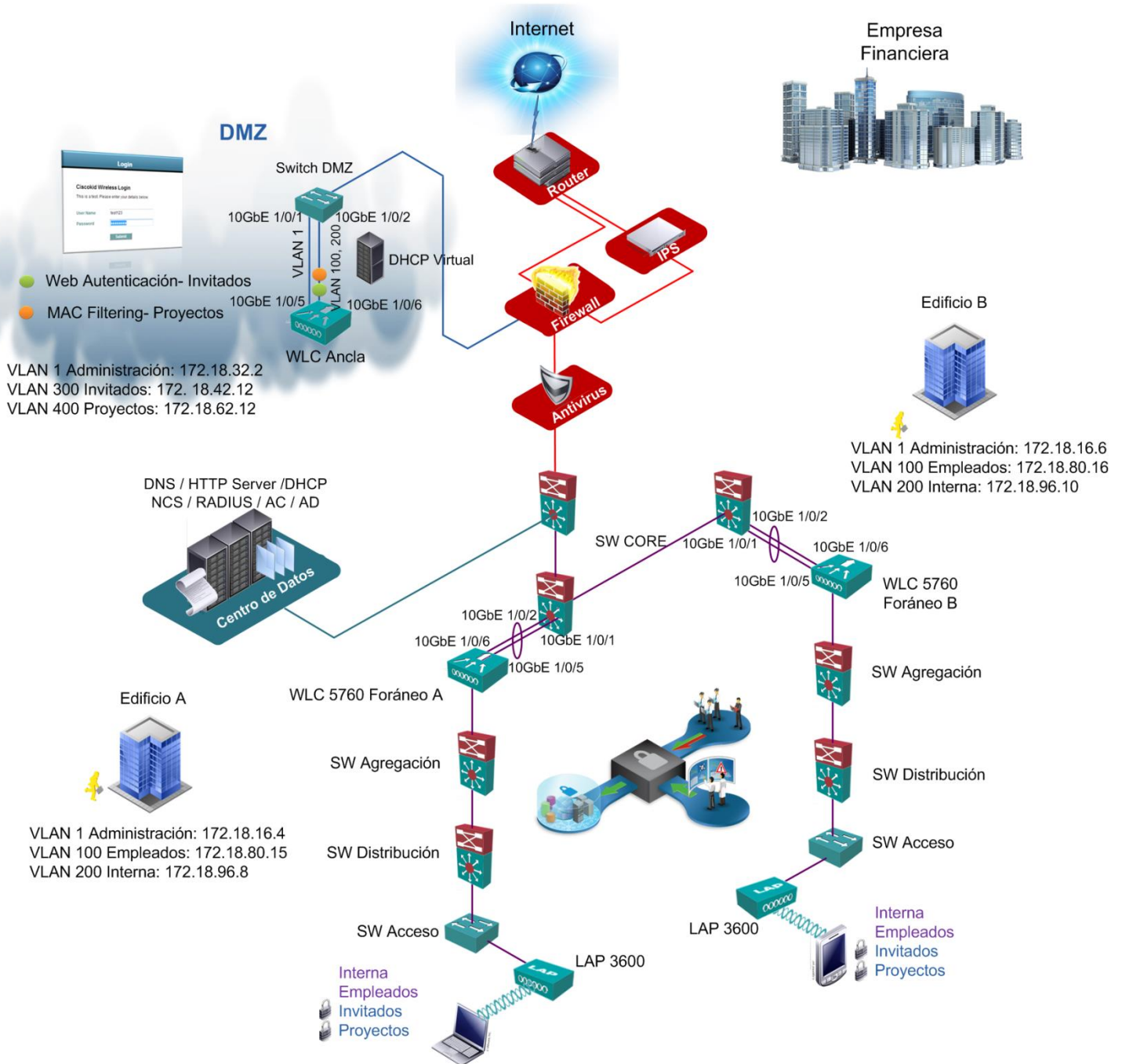
Figura 5.3 Prototipo de diseño de red WLAN IEEE 802.11
