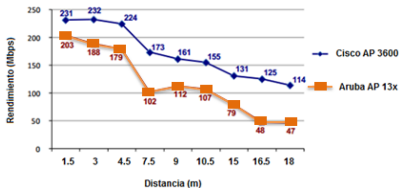
Figura 4.16 Rendimiento de los AP [51]
