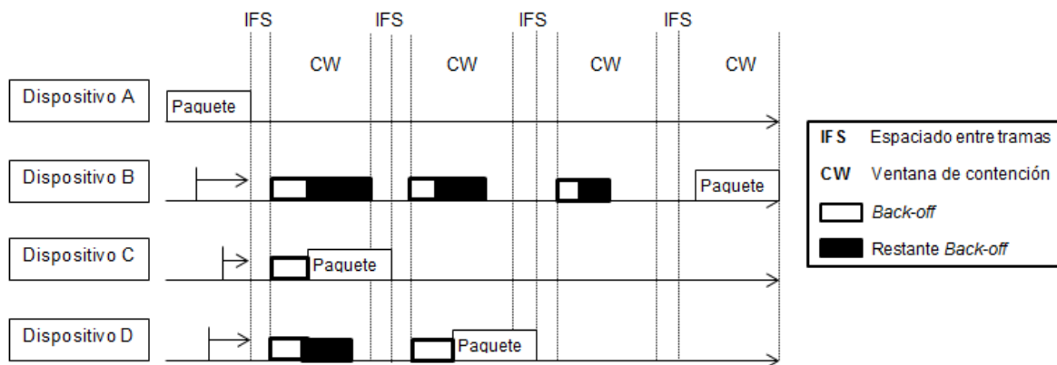
Figura 2.8 Acceso al medio en la capa MAC (CSMA/CA)
