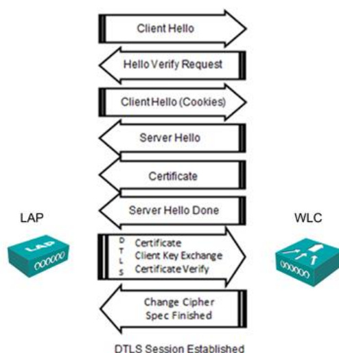
Figura 2.17 Establecimiento de CAPWAP y túnel DTLS
