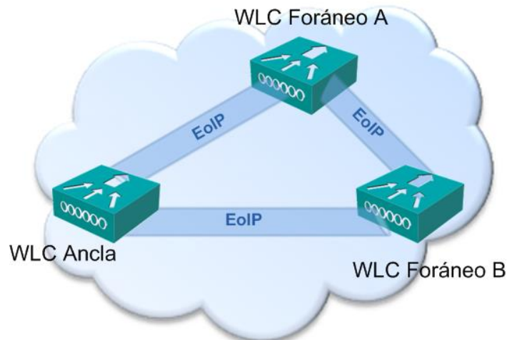
Figura 5.31 Grupo de Movilidad
