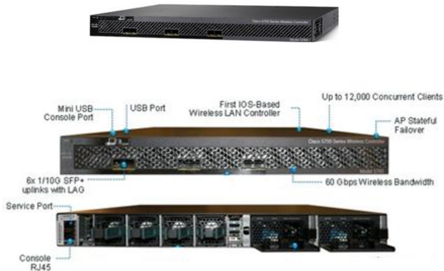
Figura 5.12 Estructura física del Cisco WLC 5760
