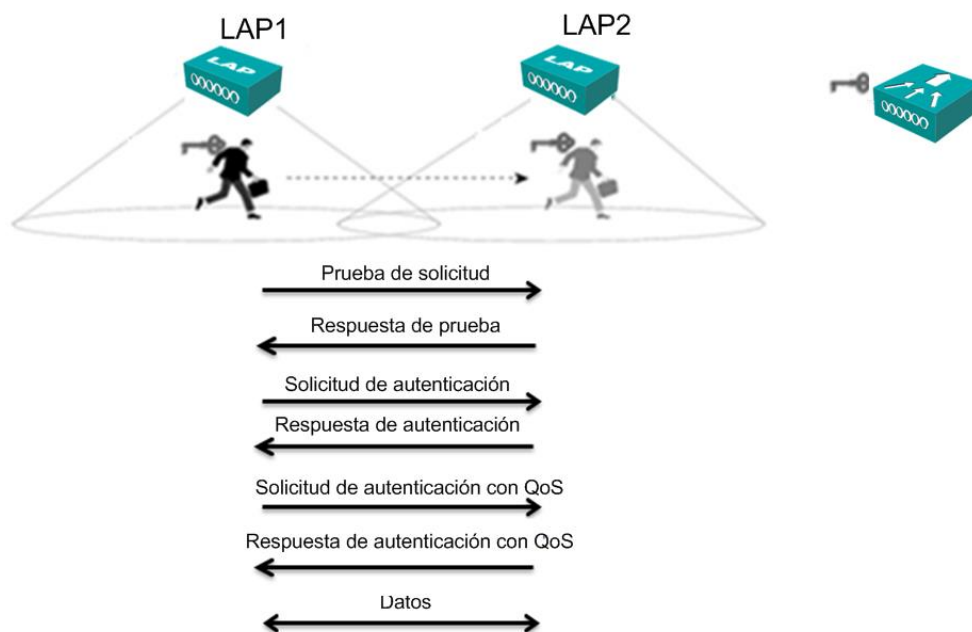
Figura 3.19 IEEE 802.11r-2008. Rápida movilidad
