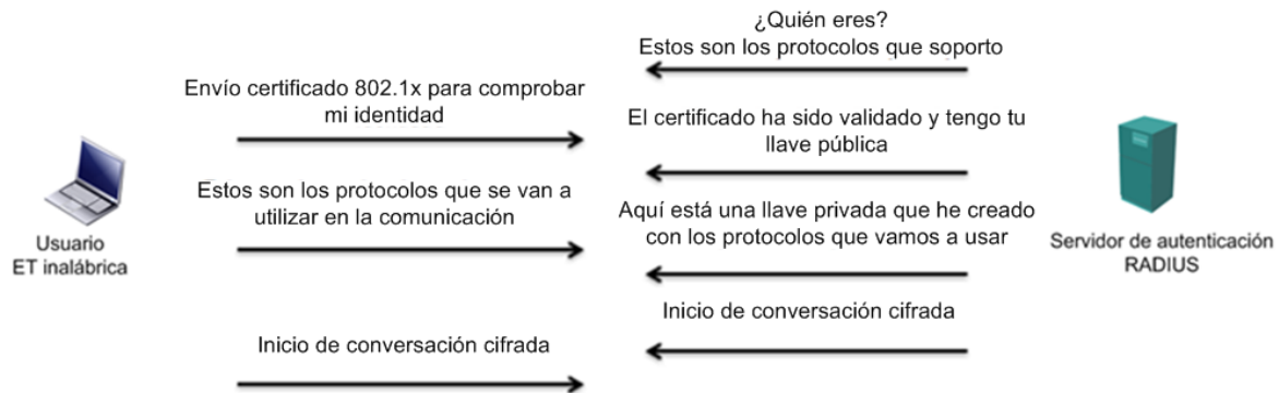
Figura 3.10 Esquema de funcionamiento del protocolo EAP-TLS
