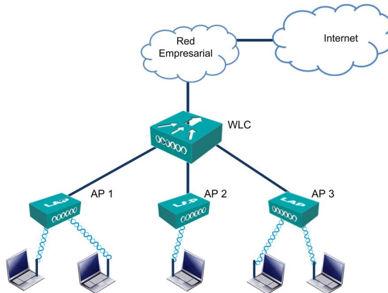
Figura 2.16 Sistema WLAN centralizado
