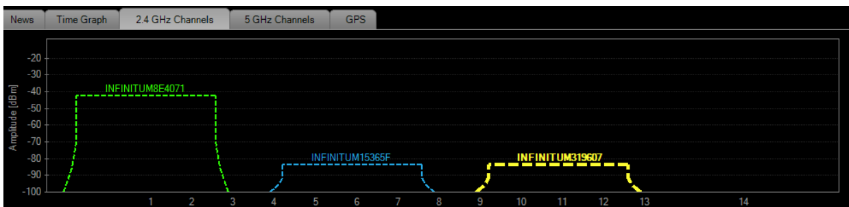
Figura 3.6 Distribución de canales para tres AP
