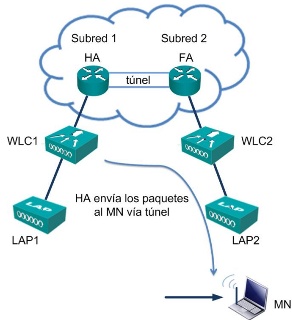
Figura 3.18 Movilidad en Capa 3
