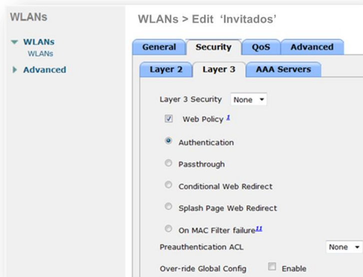
Figura 5.23 Configuración de seguridad en Capa 3
