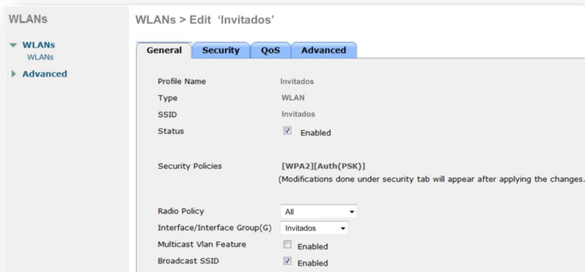
Figura 5.21 Configuración general de la red WLAN Invitados
