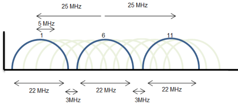
Figura 3.5 Canales en la banda de operación de 2.4 GHz
