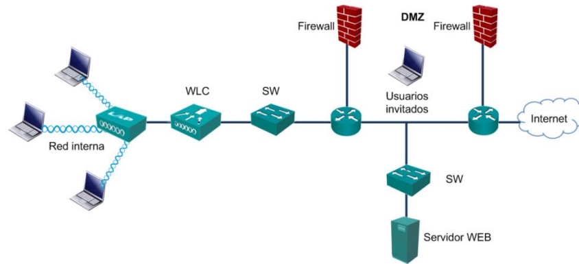
Figura 3.17 Configuración de dos firewall
