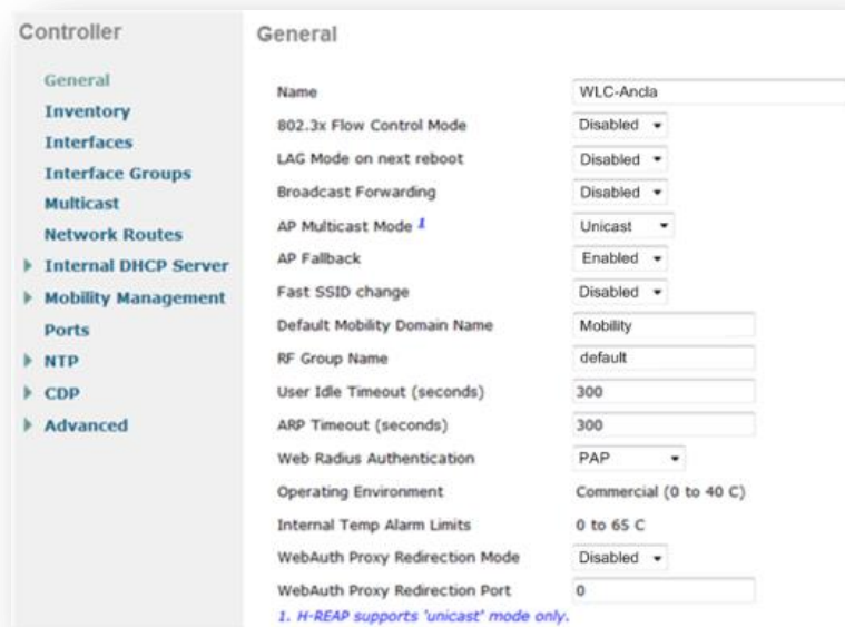
Figura 5.14 Configuración general del WLC Ancla
