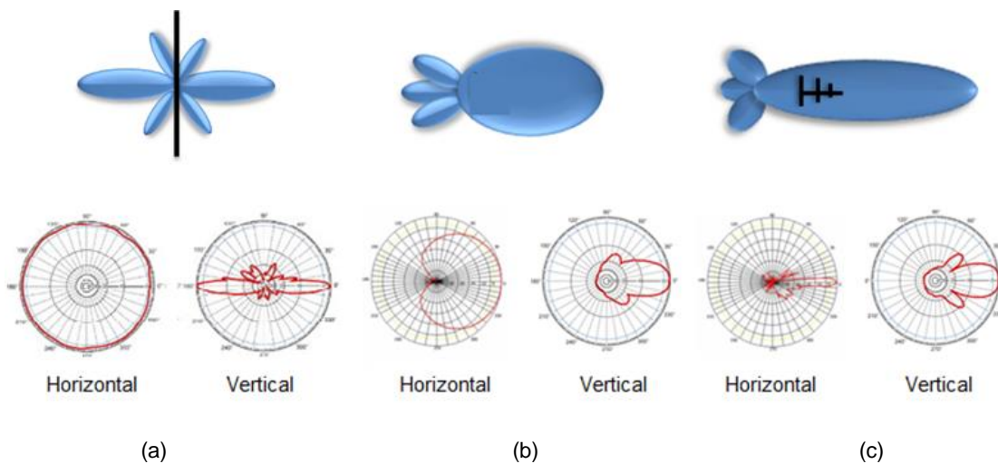
Figura 3.4 Tipos de antenas: (a) omnidireccional; (b) sectorial; (c) direccional
