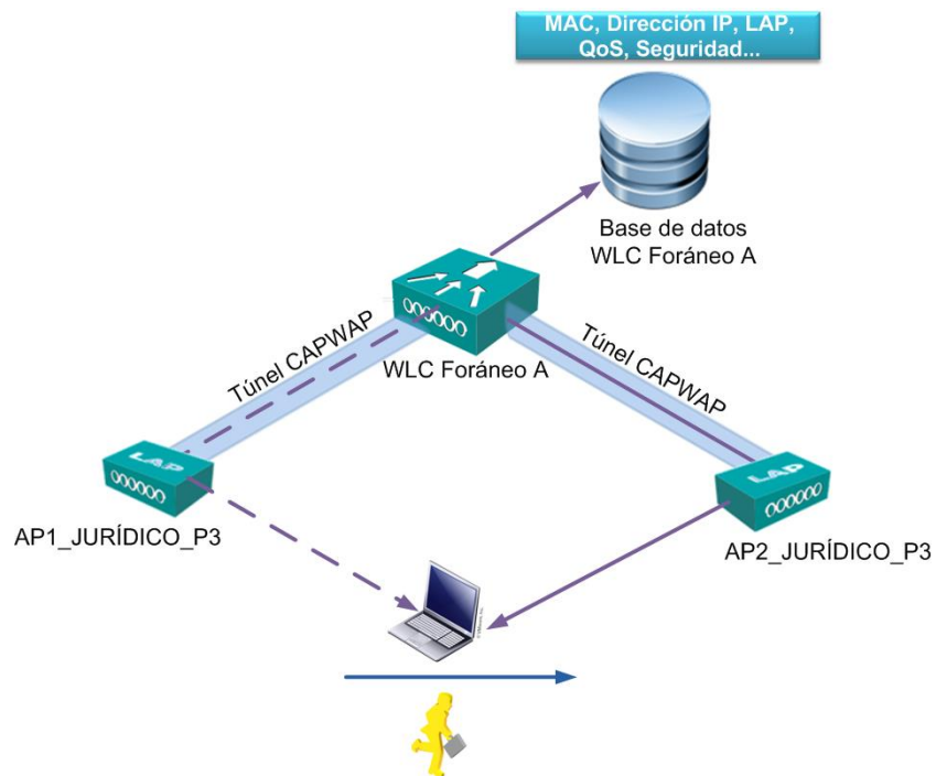
Figura 5.29 Movilidad entre dos LAP
