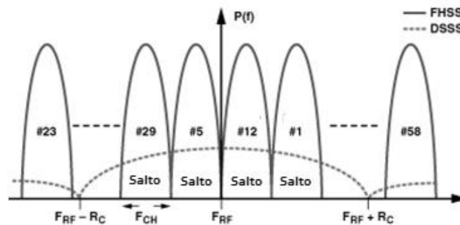
Figura 2.6 Técnicas de transmisión FHSS y DSSS
