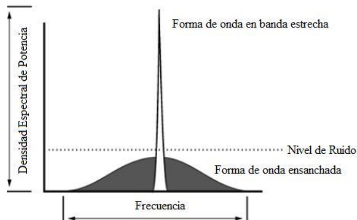
Figura 2.5 Espectro disperso
