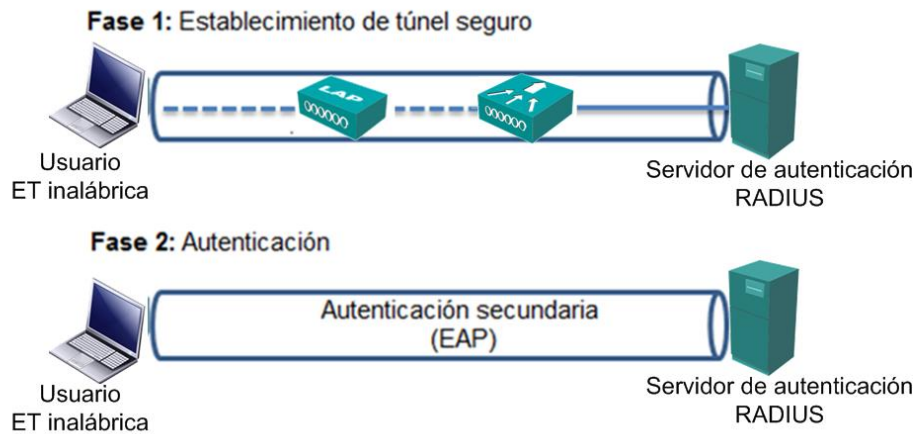
Figura 3.11 Autenticación EAP-TTLS
