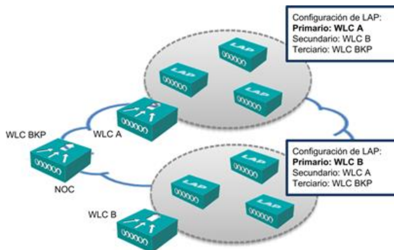
Figura 2.20 Arquitectura de redundancia N+N+1
