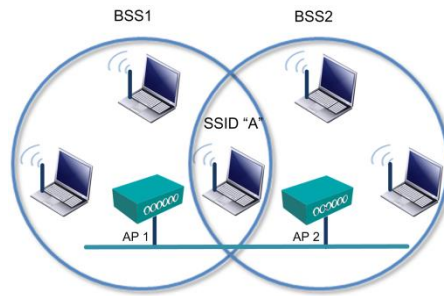
Figura 2.13 Conjunto de servicios extendidos
