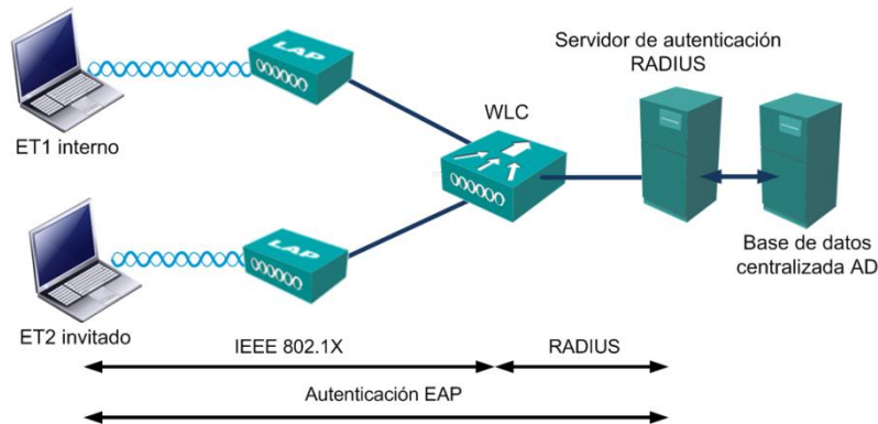
Figura 3.8 Arquitectura de autenticación IEEE 802.1x y EAP basada en RADIUS
