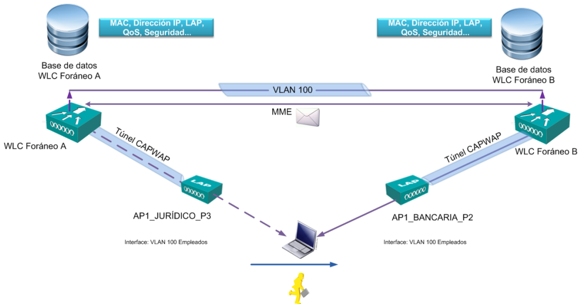
Figura 5.30 Movilidad intra-WLC
