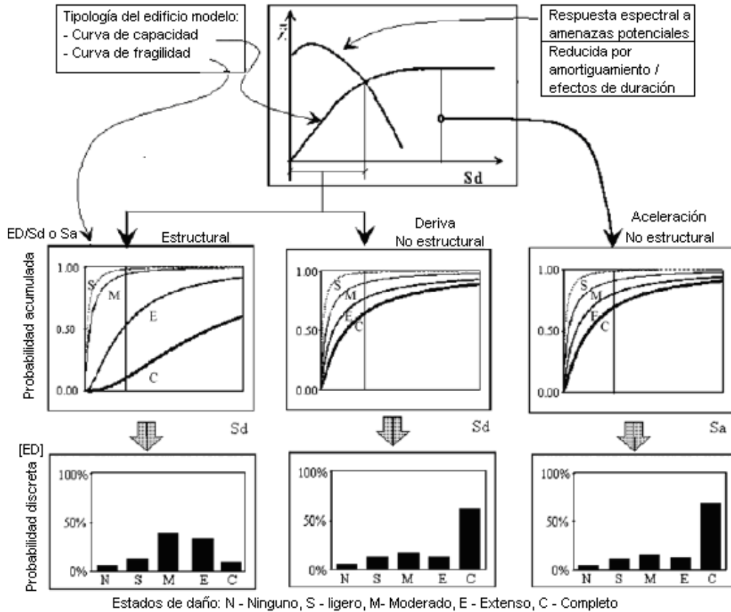
Figura 2.6 Ilustración de la estimación de daño esperado a partir de la vibración del suelo en HAZUS (FEMA, 1999, 2003)
