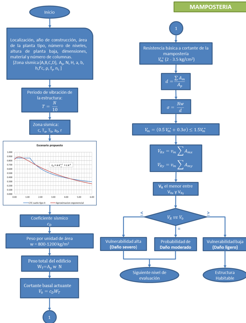
Figura 3.12 Procedimiento de evaluación intermedia para estructuras de mampostería
