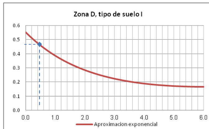
Figura 4.2 Demanda sísmica calculada para la evaluación
