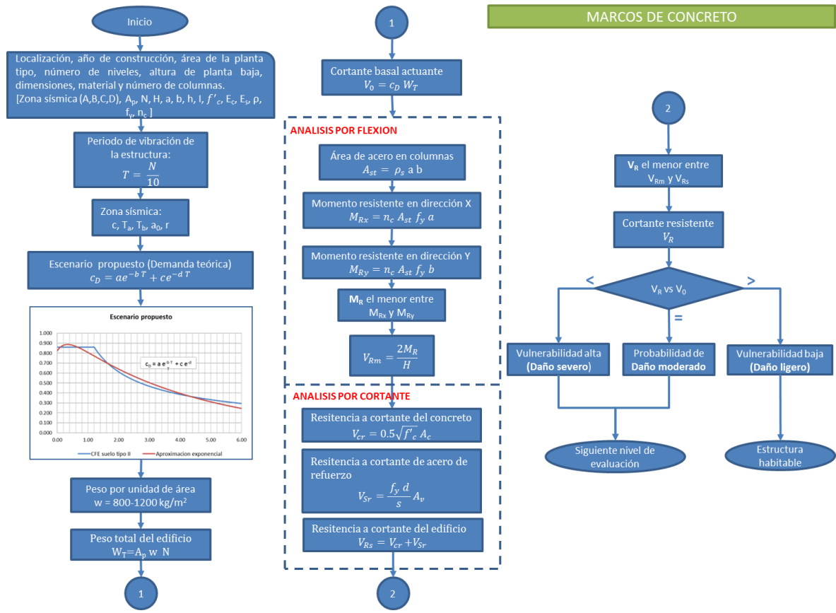
Figura 3.13 Estimación de la resistencia a través de las áreas de los elementos estructurales
