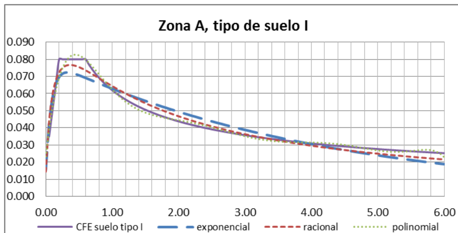
Figura A.1 Aproximaciones realizadas para ajustar los espectros de diseño de CFE
