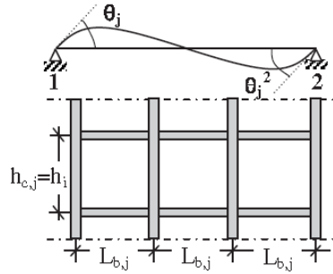
Figura 3.16 Definiciones de rotación y altura del elemento j
