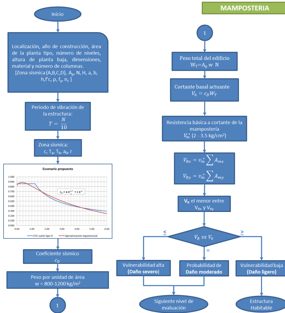
Figura 3.7 Procedimiento de evaluación intermedia para estructuras de mampostería
