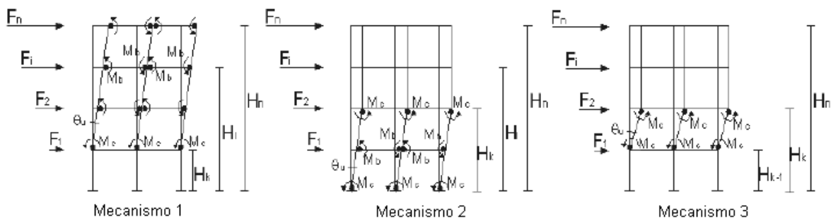
Figura 2.15 Mecanismos predefinidos de colapso
