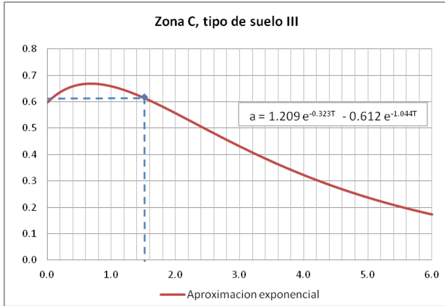
Figura 4.4 Demanda sísmica calculada para la evaluación
