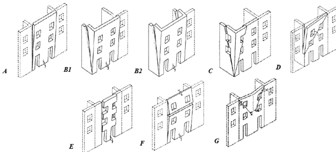
Figura 2.3 Mecanismos de falla fuera del plano (según D'Ayala y Speranza, 2002)
