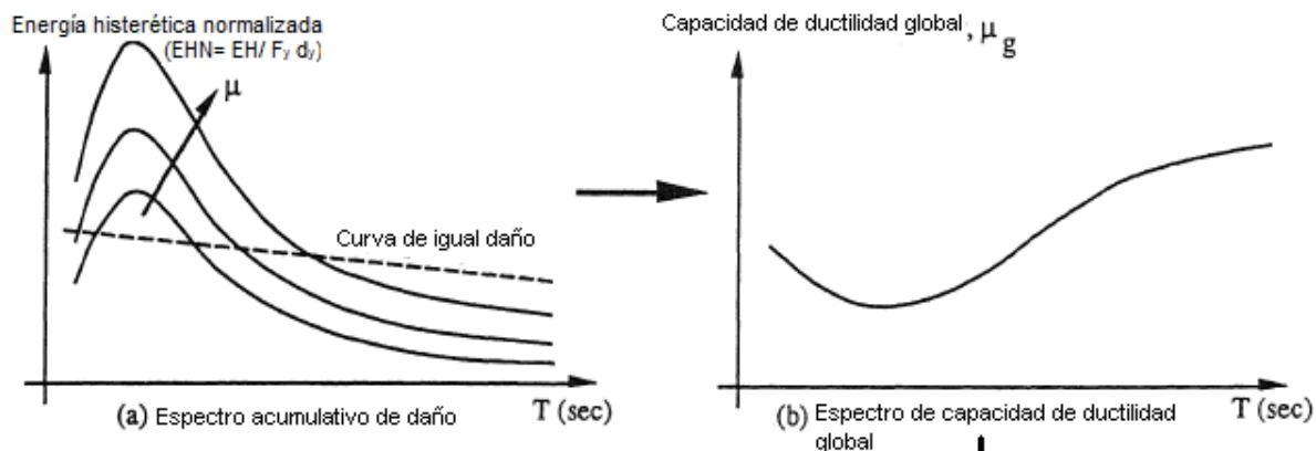
Figura 2.4 Implementación del procedimiento propuesto por Nassar-Osteraas de diseño sismico.
