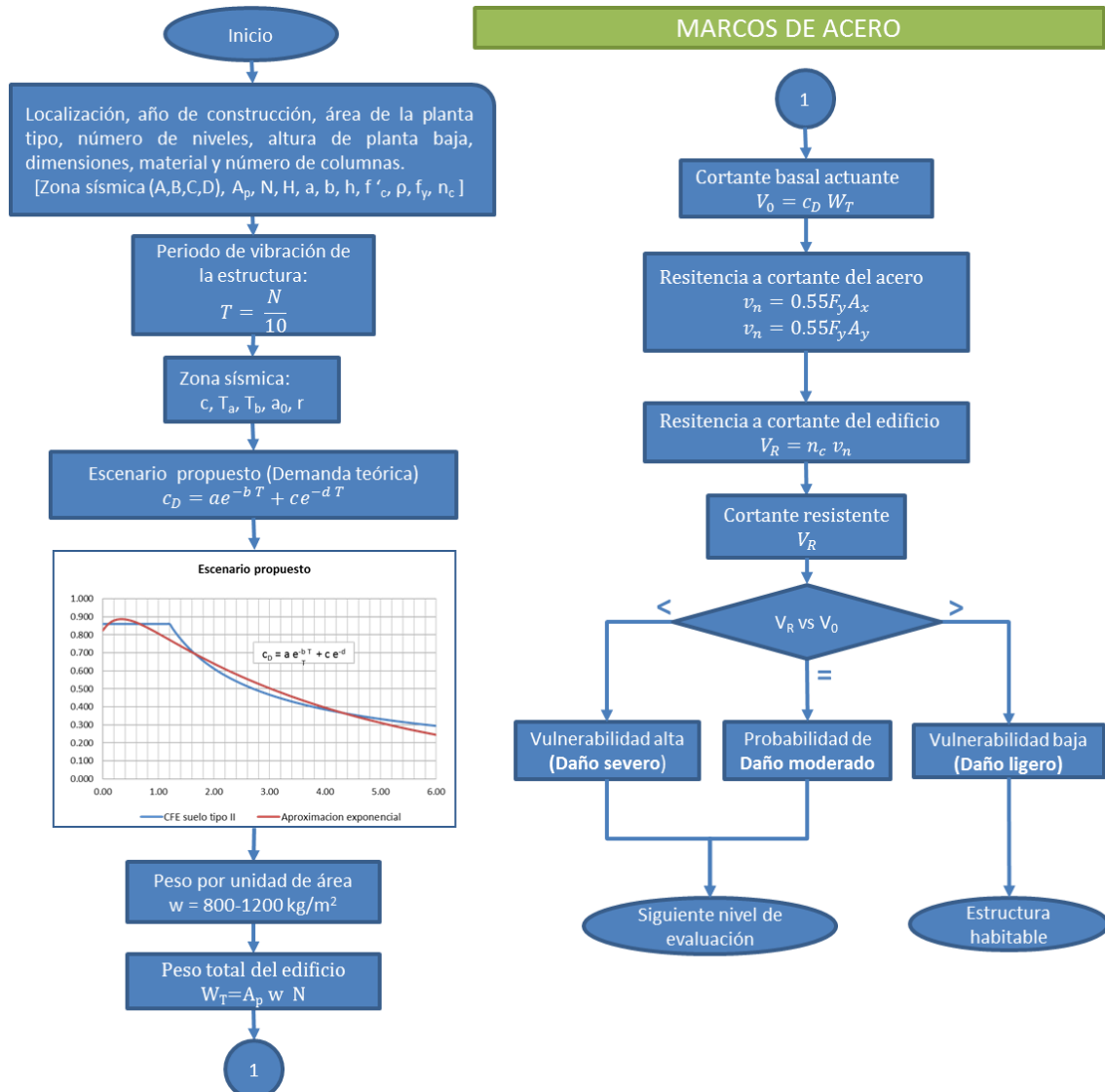
Figura 3.8 Estimación de la resistencia a través de las áreas de los elementos estructurales
