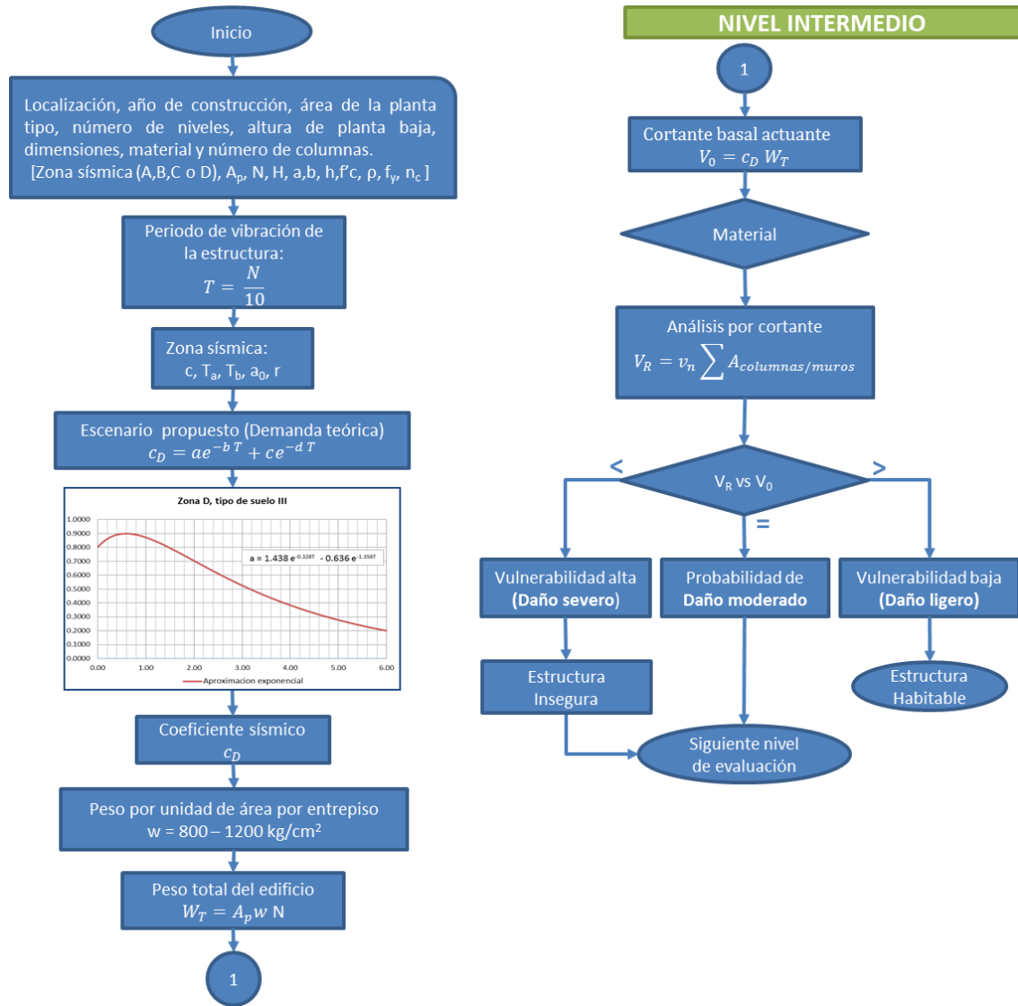
Figura 3.6 Evaluación intermedia de vulnerabilidad estructural
