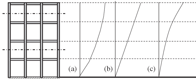
Figura 3.15 Perfil de desplazamiento de un edificio a base de marcos a) por cortante b) triangular c) por flexión
