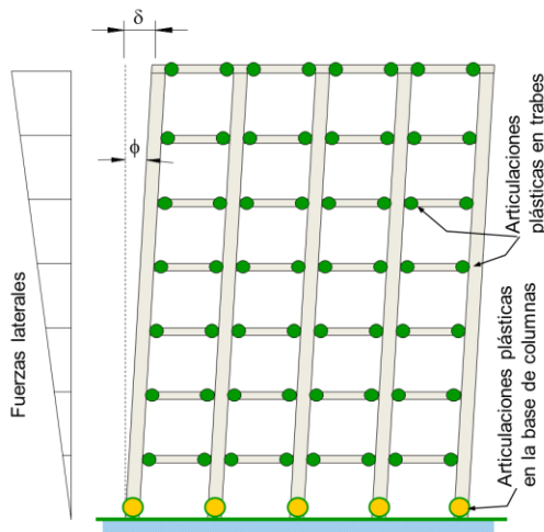
Figura 3.10 Mecanismo de cortante (acervo de imágenes del CENAPRED)
