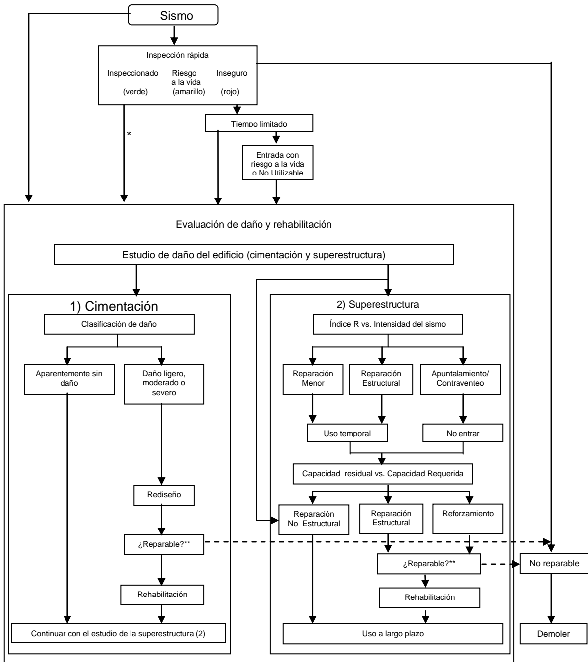
Figura 2.11 Diagrama de flujo de la evaluación y rehabilitación de daños supuesta en la guía.
