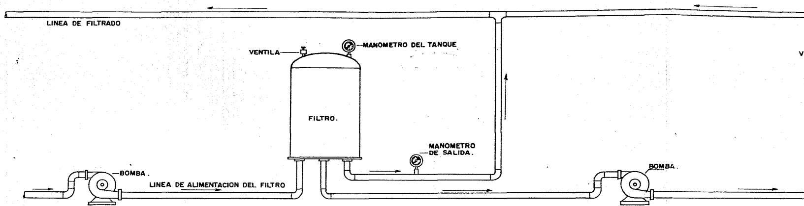
fig. 3 SISTEMA DE FILTRADO DE ALTA PRESION.
