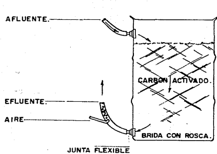
fig. 2 FILTRACION QUIMICA.
