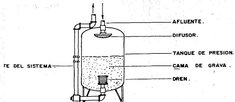
fig. 1 FILTRO RAPIDO DE ARENA.
