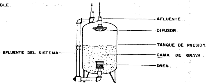
fig. 1 FILTRO RAPIDO DE ARENA.
