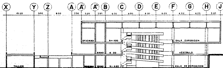
CORTE LONGITUDINAL
