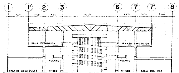
CORTE TRANSVERSAL
