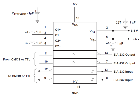
Figura 4.4: MAX232.
