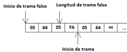
Figura 3.8: Inicio de trama debido a ruido.
