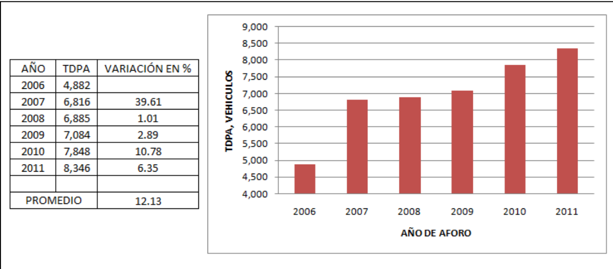
Figura 5.3. Variación del volumen de tránsito vial 2006 – 2011, carretera federal libre 120. Fuente: S.C.T.
