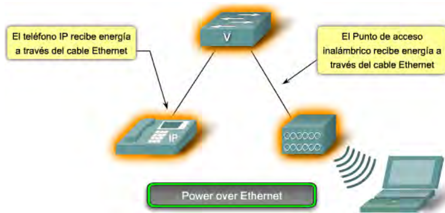
Figura 4.8 Switch con tecnología PoE
