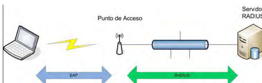
Figura 1.21 Autenticación EAP con RADIUS
