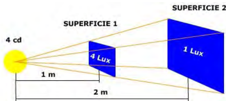
Figura A1.13 Ejemplo la ley de la inversa del cuadrado de la distancia
