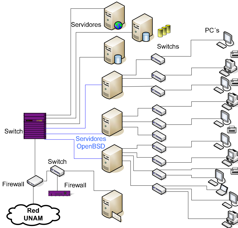
Figura 4.2. Esquema de red de la BC.
