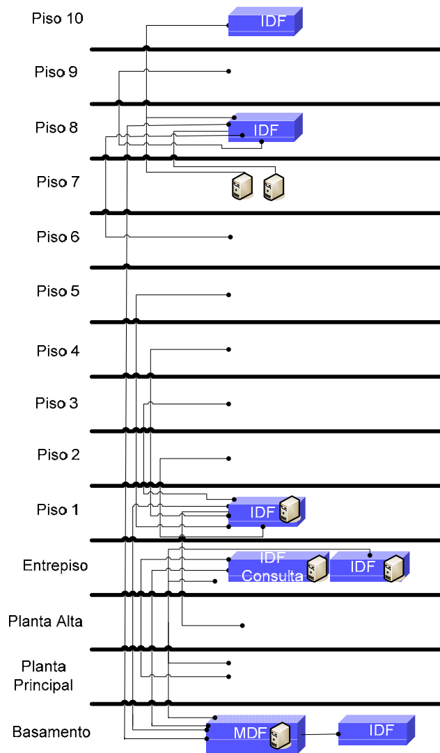
Figura 4.1. Red de la BC-RedDGB.
