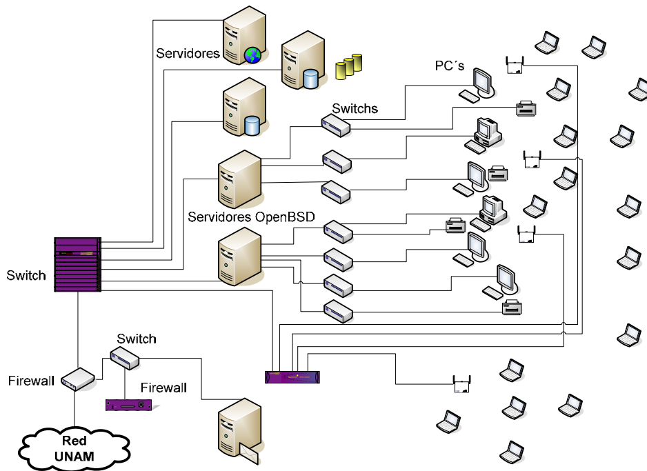
Figura 4.7. Instalación de red Inalámbrica con equipo Altitud 300-2 y Summit 300.
