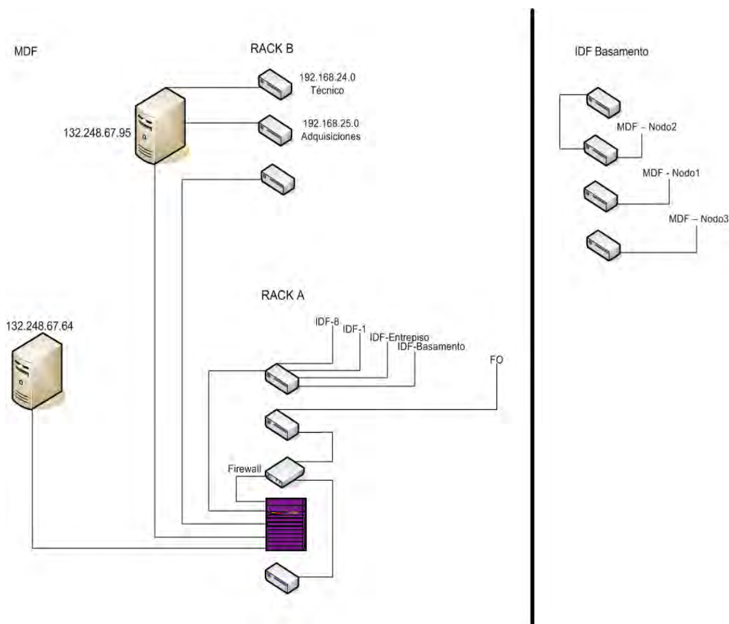
Figura 5.2. Esquema de IP en el MDF y en el IDF de Basamento.
