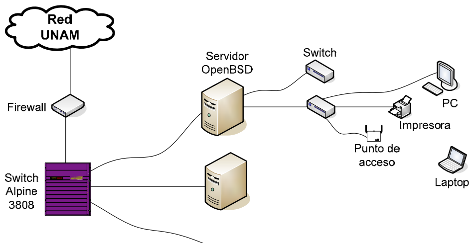
Figura 5.1. Equipos Activos de la red de la BC.
