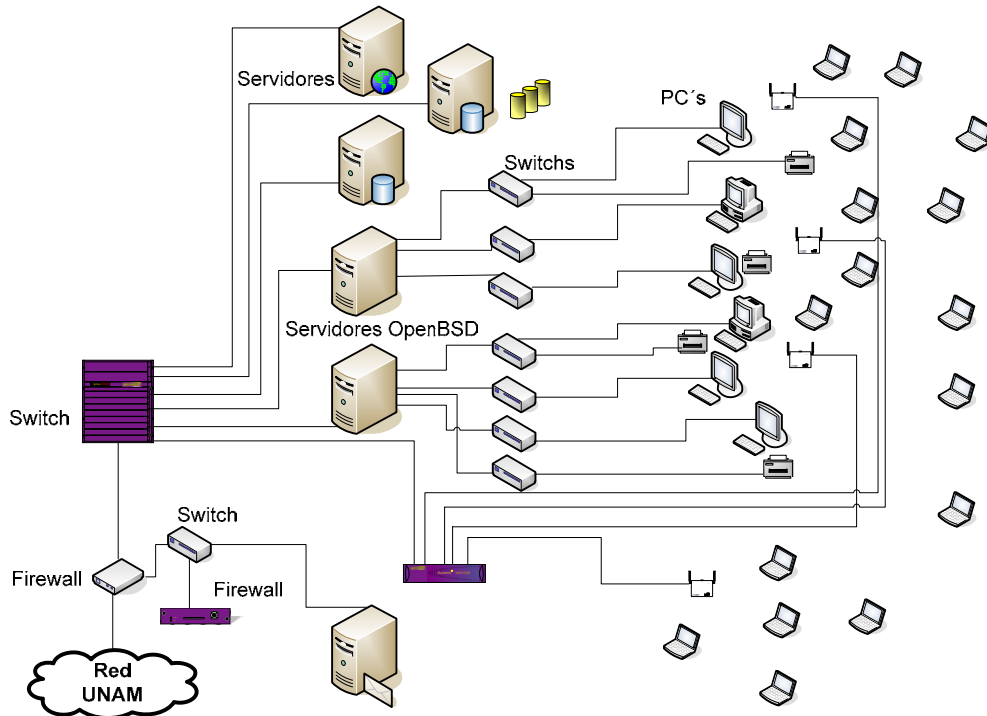
Figura 4.9. Instalación de red Inalámbrica con equipo 3com y Summit 300.
