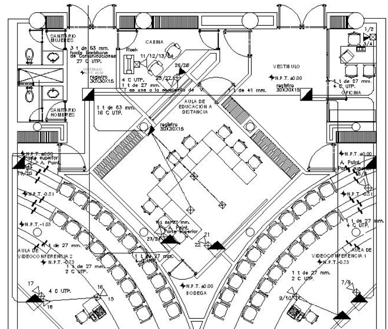
Plano 4.4. Sala de Videoconferencia.
