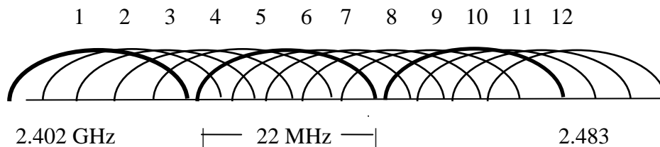
Figura 3.8. Diagrama de canales de frecuencias de trabajo.
