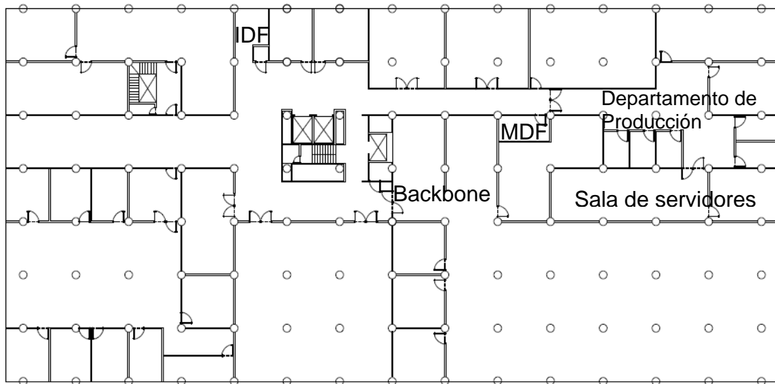
Figura 1.5. Plano de distribución de los cuartos de comunicación en Basamento.
