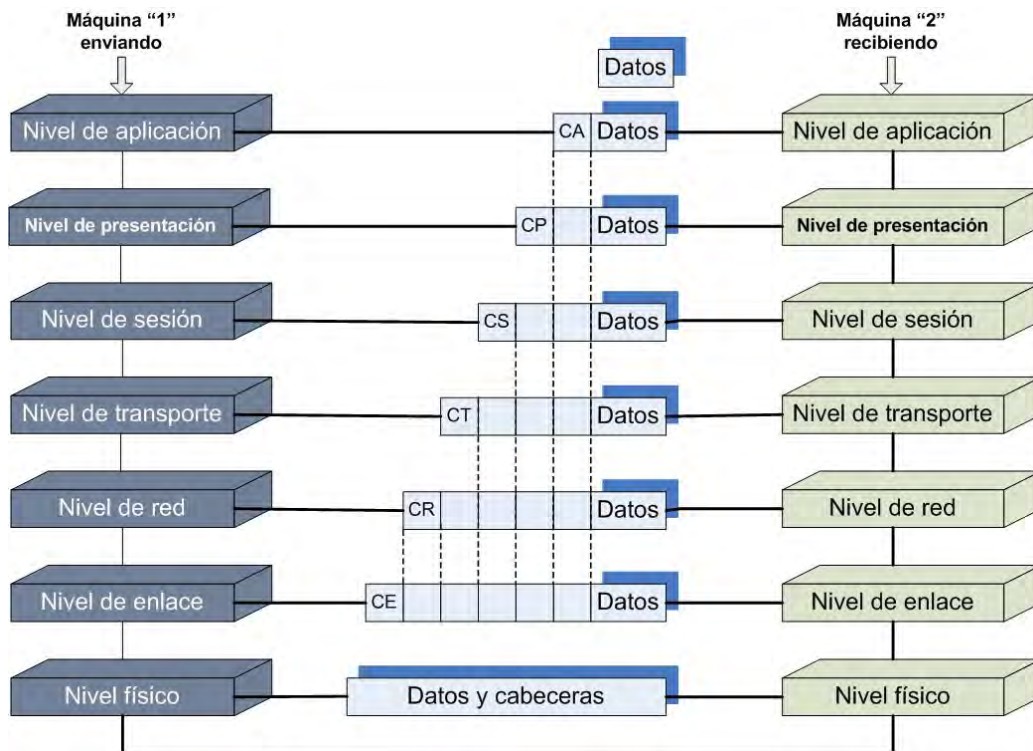
Figura 2.10. Modelo OSI.
