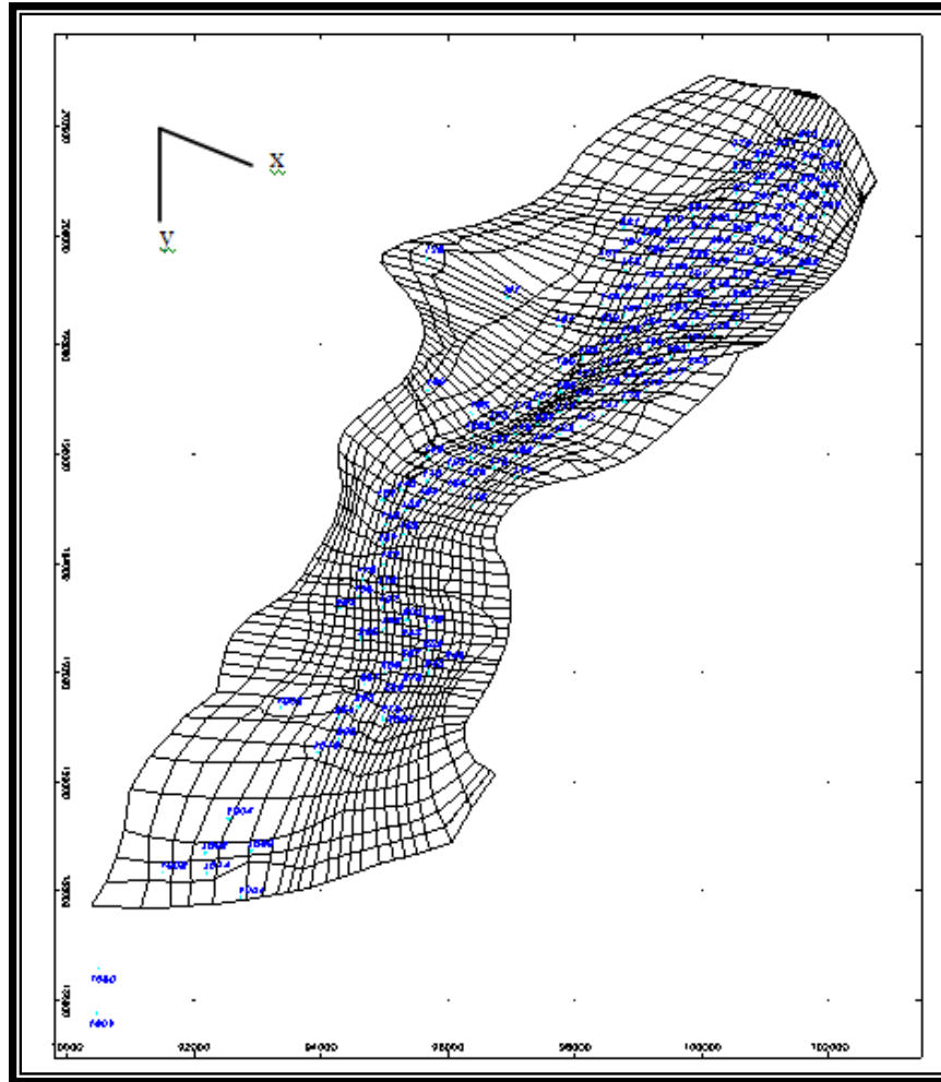
Figura II.12. Malla irregular de simulación (vista areal).
