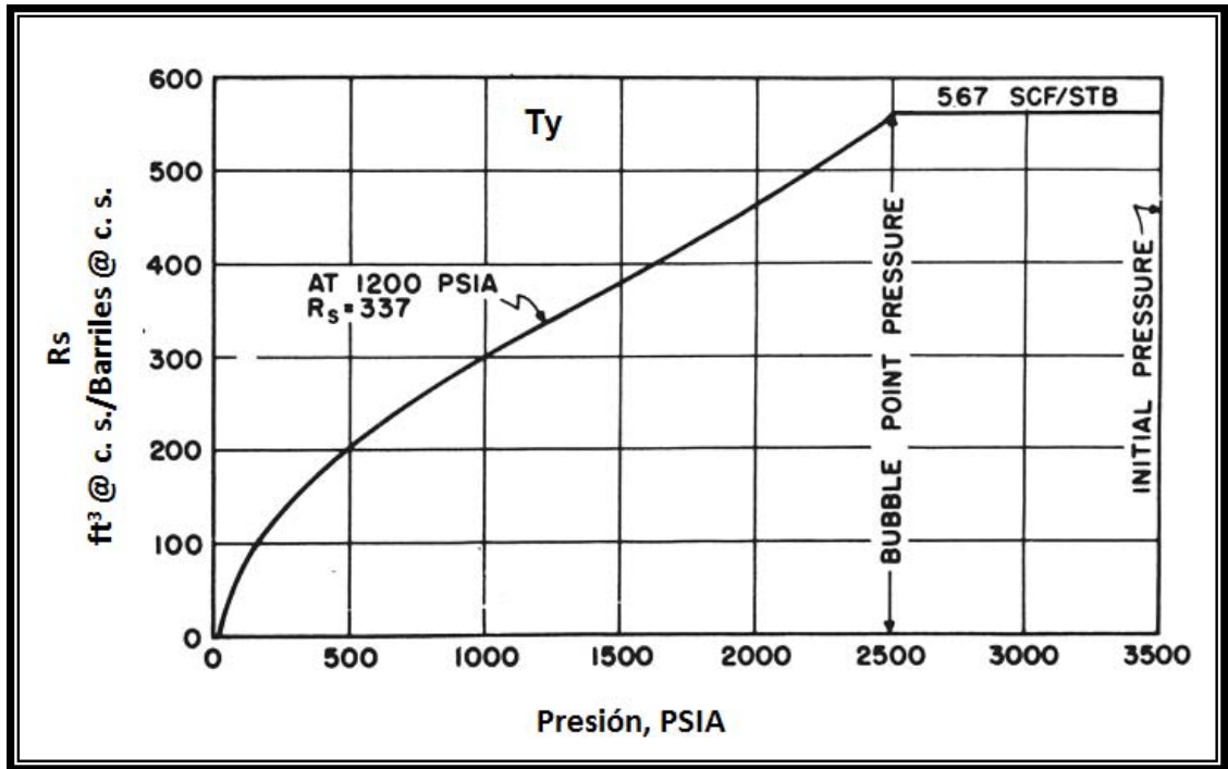
Figura II.18. Curva típica de R_s .
