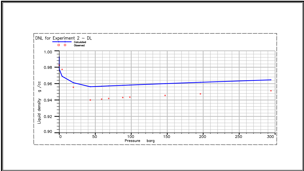
Figura IV.16. Densidad del aceite (11 componentes). Pozo Alfa-1.
