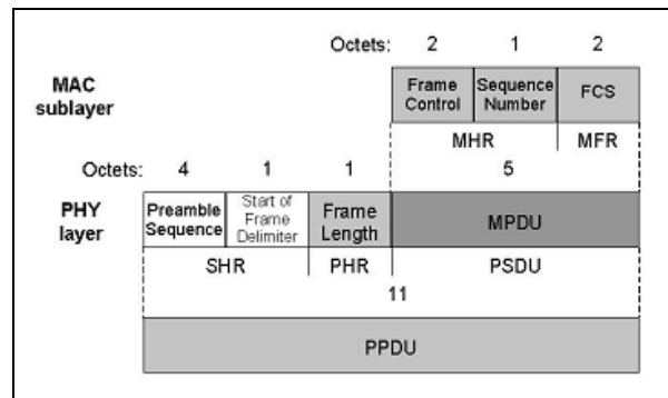
Figura 3.10 Estructura de la trama de reconocimiento (ACK)
