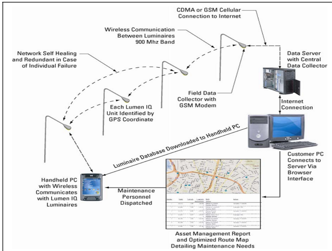
Figura 1.4 Modo de operación del sistema
