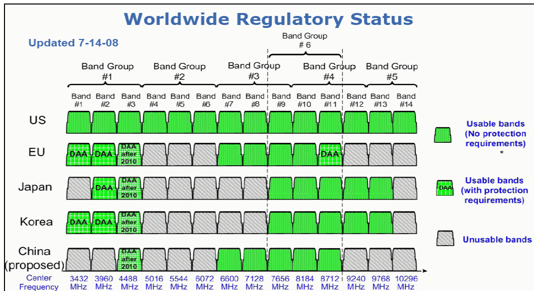
Figura 2.7 Bandas de frecuencia asignadas para UWB
