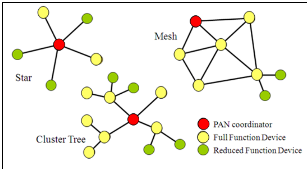
Figura 3.4 Topologías Zigbee
