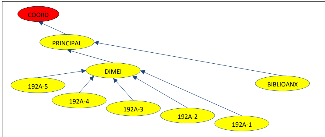
Figura 5.24 Estructura de red para la formación 6
