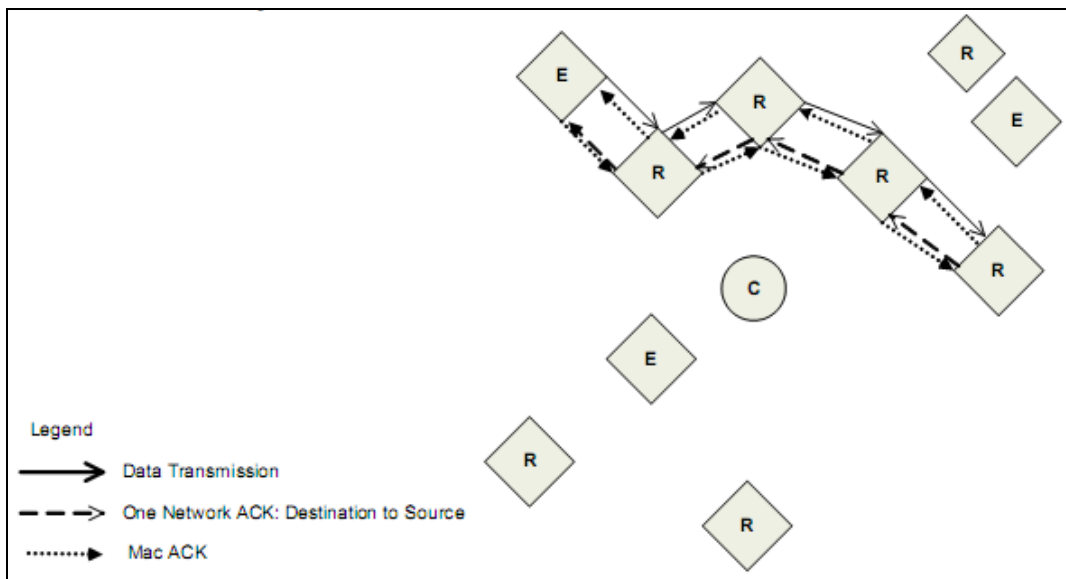
Figura 3.21 Proceso de transmisión de datos en entre nodos Zigbee.
