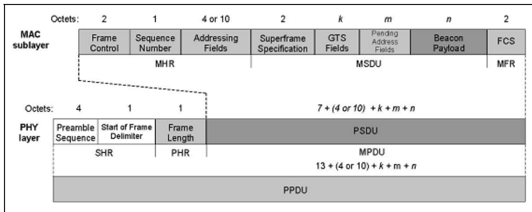
Figura 3.12 Estructura de la trama Beacon
