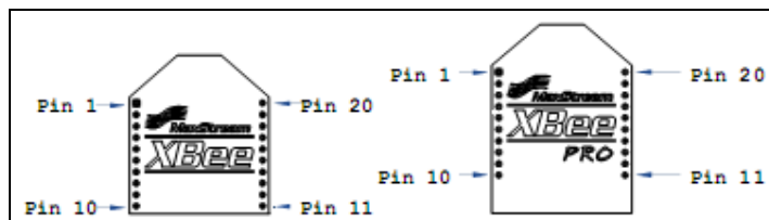
Figura 4.3 Disposición de pines en los radios XBee
