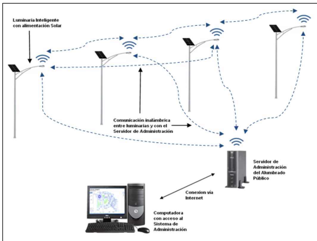
Figura 1.5 Visión General del Sistema de Alumbrado Público Inteligente
