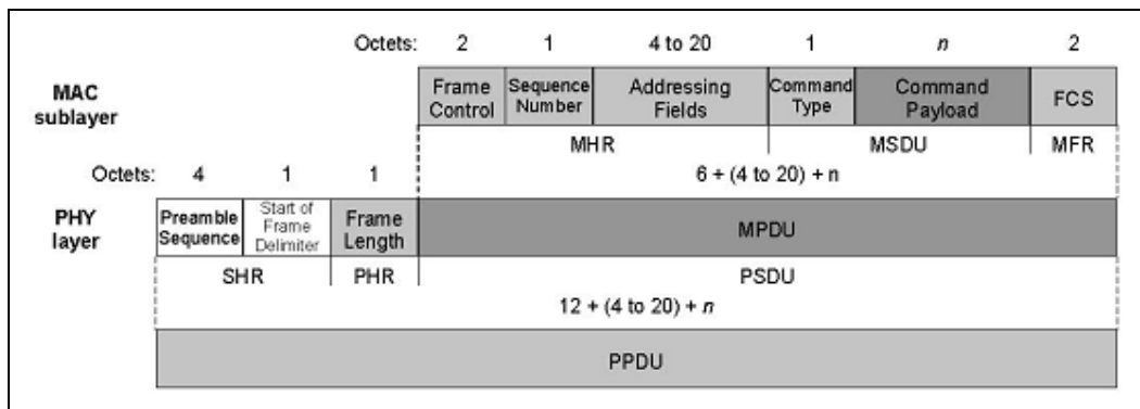
Figura 3.11 Estructura de la trama de comandos MAC
