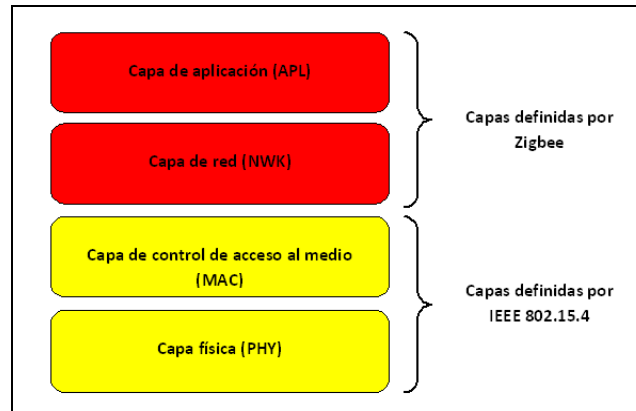
Figura 3.1 Modelo de las capas de Zigbee
