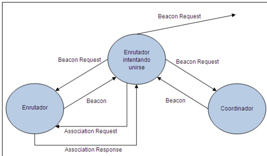
Figura 3.15 Proceso de unión en una PAN
