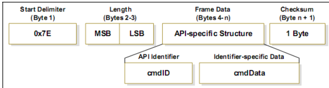
Figura 4.15 Trama de datos UART y estructura específica API
