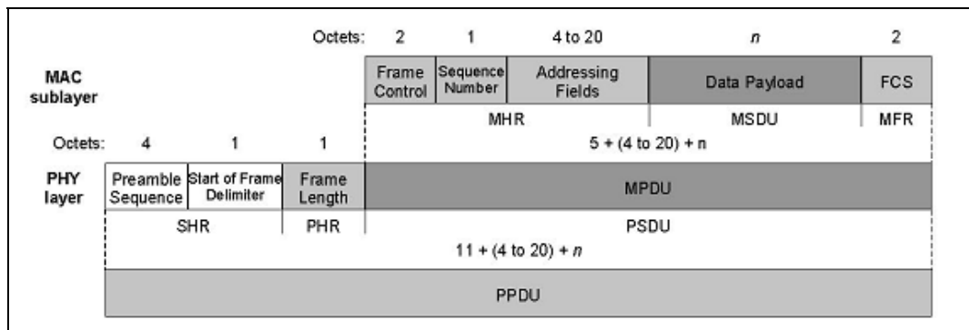
Figura 3.9 Estructura de la trama de datos
