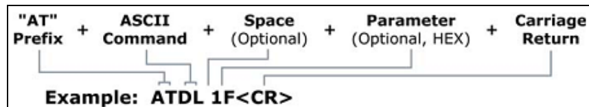
Figura 4.10 Sintaxis para enviar un comando AT
