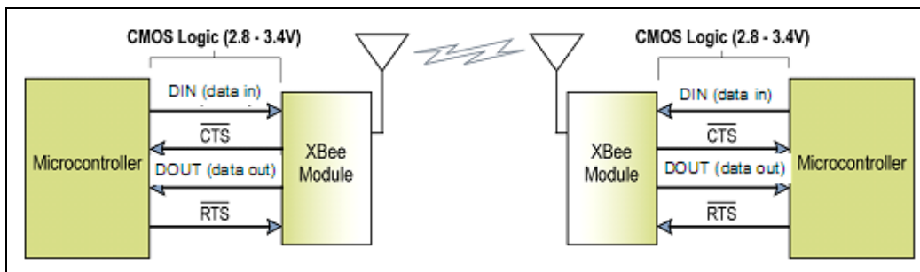
Figura 4.5 Diagrama de flujo de datos en dispositivos con interface UART
