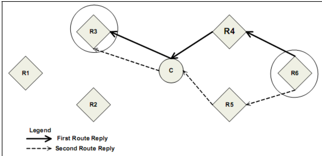
Figura 3.19 Ejemplo de Route Reply Command, R6 puede enviar más de un Route Reply si este identifica una mejor ruta
