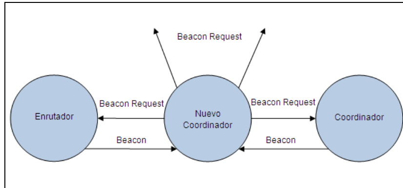
Figura 3.14 Operación del escaneo activo.
