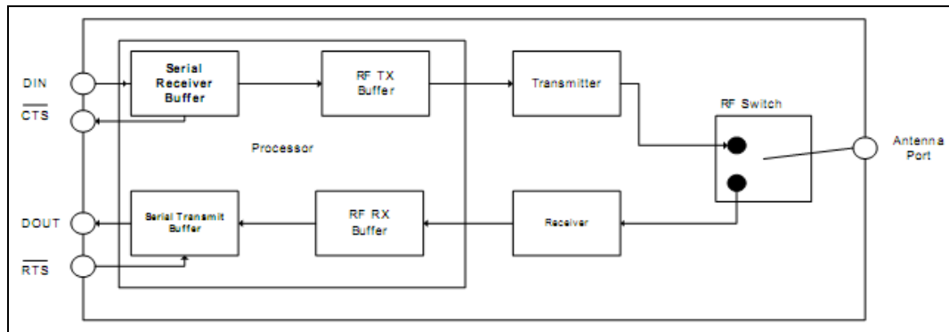
Figura 4.7 Diagrama interno de flujo de datos
