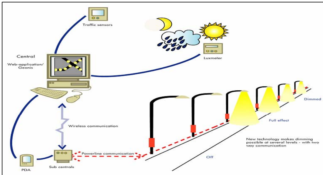
Figura 1.3 Sistema de Alumbrado Inteligente, Oslo Noruega
