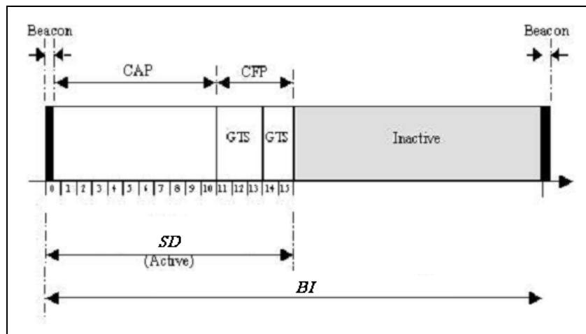
Figura 3.13 Ejemplo de supertrama
