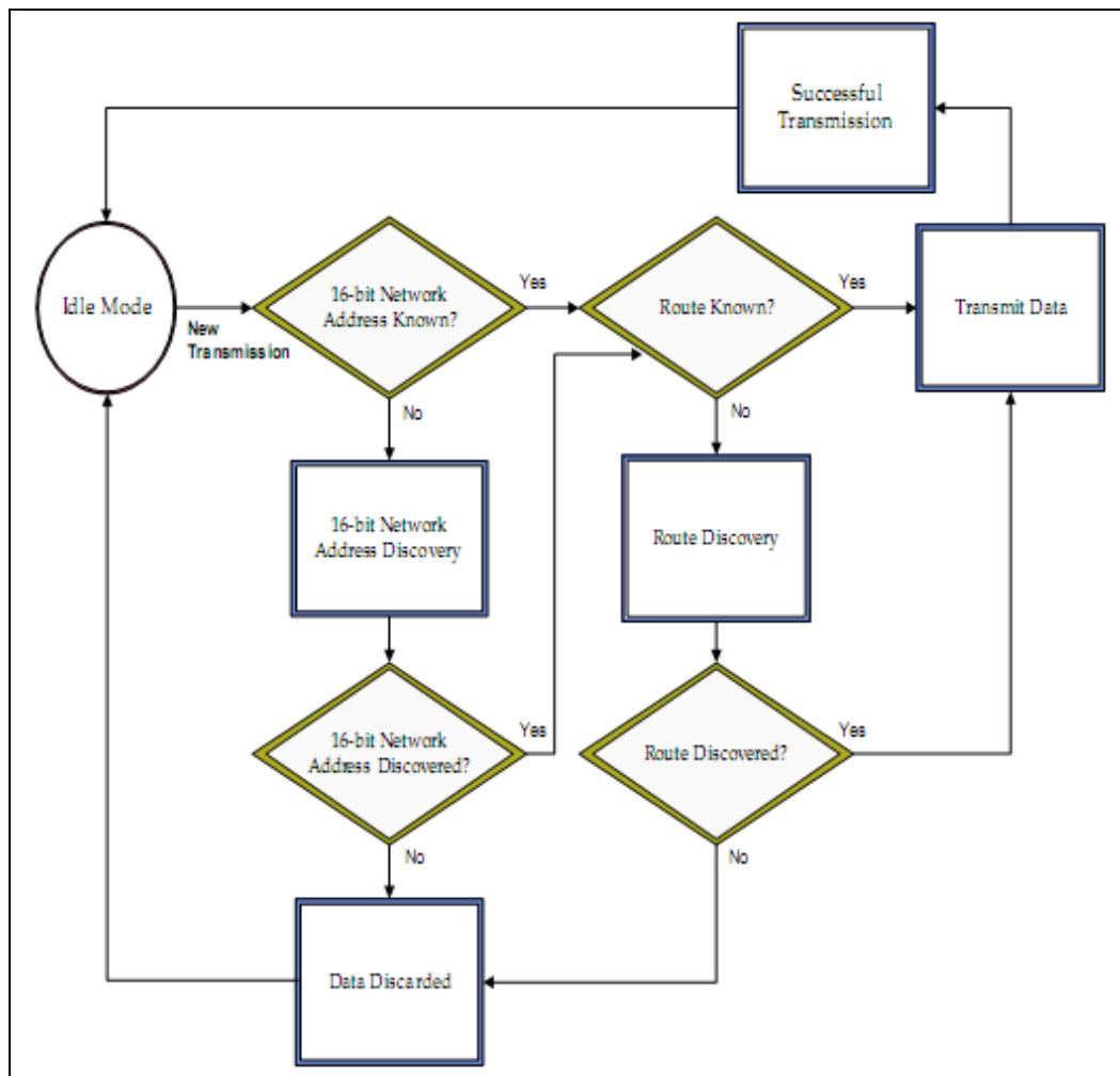
Figura 4.9 Modo de secuencia de transmisión
