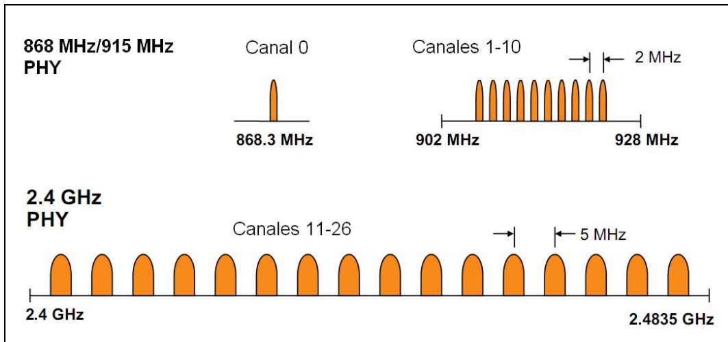
Figura 3.6 Canales IEEE 802.15.4
