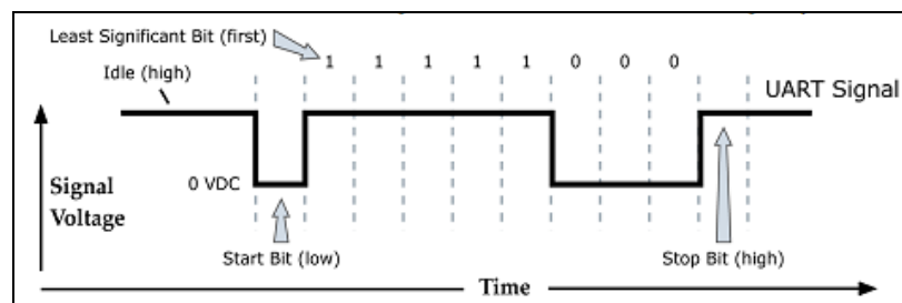
Figura 4.6 Paquete de datos UART 0x1F (valor decimal "31").
