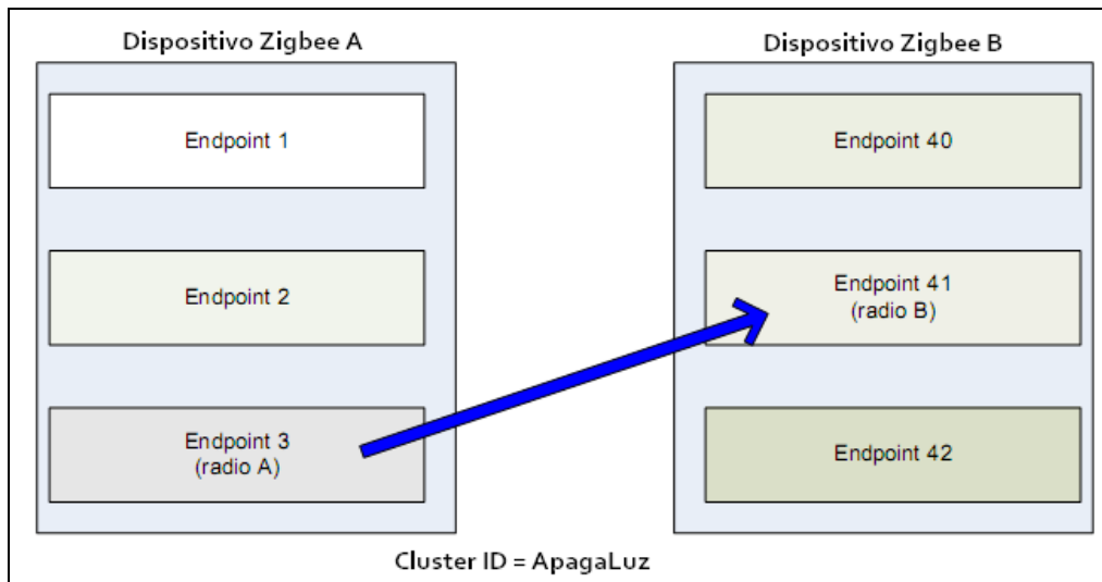
Figura 3.16 Ejemplo de direccionamiento de aplicación Zigbee
