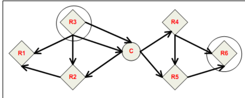
Figura 3.18 Ejemplo de broadcast de Route Request Command, búsqueda de ruta de R3 a R6
