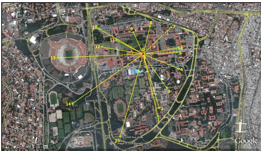
Figura 5.4 Ubicación visual de los radios XBee-Pro dentro del campus
