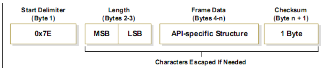
Figura 4.14 Estructura de trama de datos UART con AP = 2.
