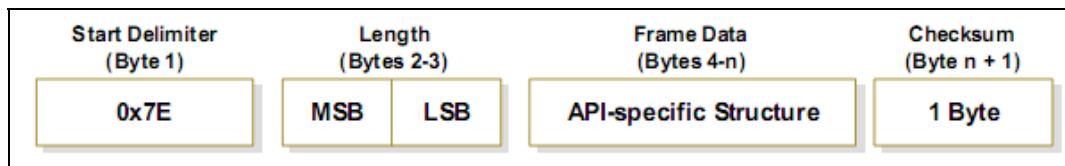
Figura 4.13 Estructura de trama de datos UART con AP = 1. MSB = More Significant Byte, LSB = Less Significant Byte.
