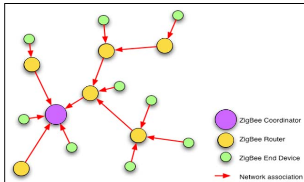
Figura 2.10 Estructura en la red Zigbee
