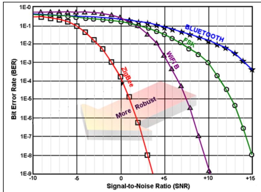
Figura 3.3 Comportamiento de BER respecto a SNR
