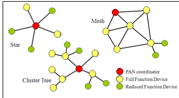
Figura 2.9 Topologías de red en Zigbee
