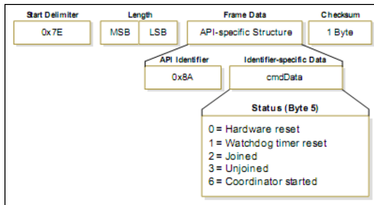
Figura 4.17 Trama Modem Status
