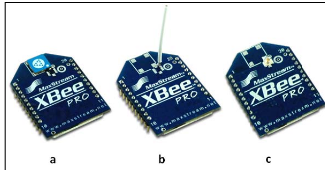
Figura 5.2 Tipos de antena en radios XBee/XBee-Pro, a) antena de chip, b) antena de látigo y c) conector U.FL
