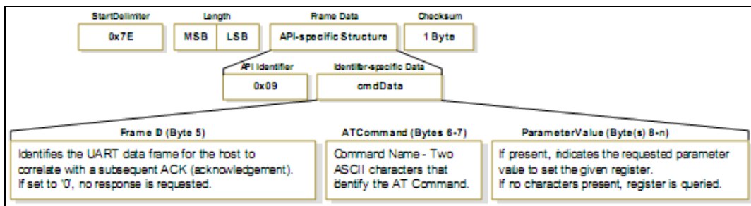
Figura 4.19 Trama AT Command con valor en cola. La trama es igual que la AT Command a excepción del identificador API.
