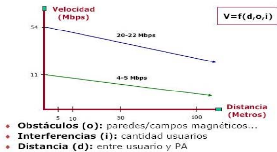
figura 3.1 comportamiento de la velocidad de transmisión con respecto a ciertos fenómenos involucrados
