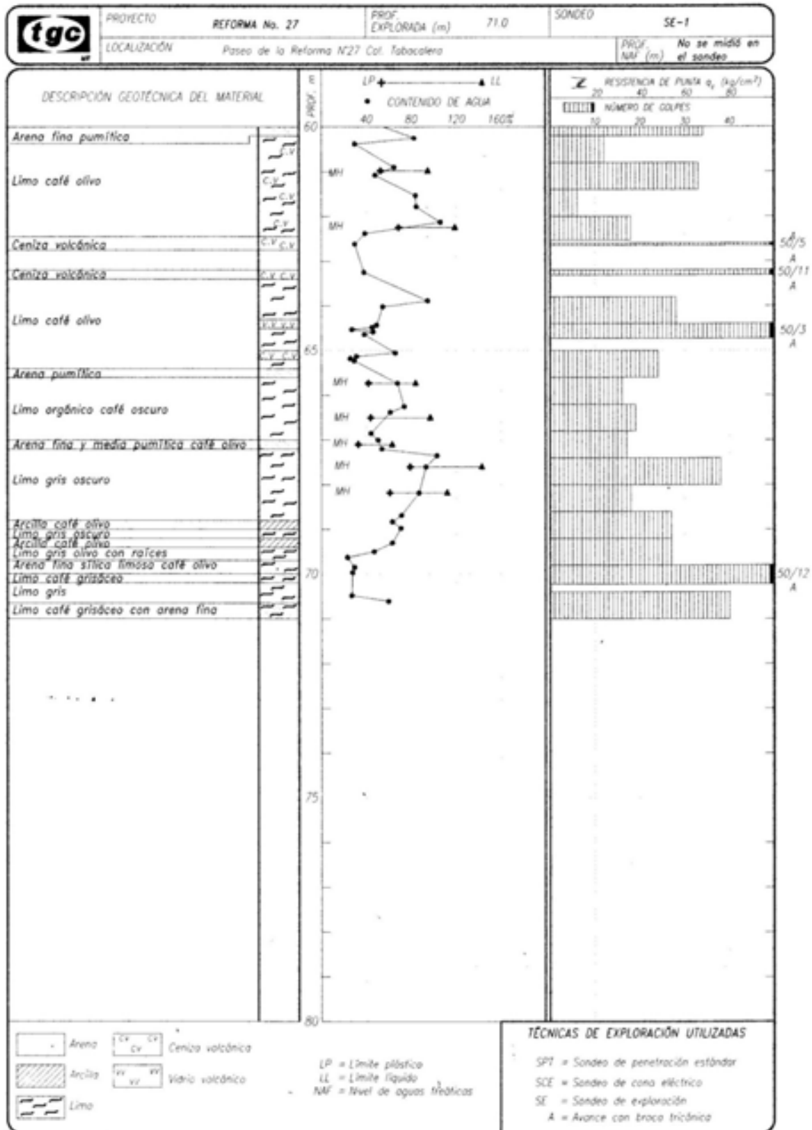
Fig. 2-2d Registro de exploración geotécnica (SPT).
