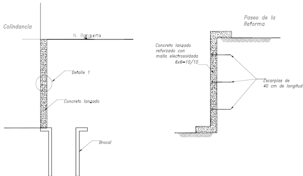
Fig. Protección de colindancias.
