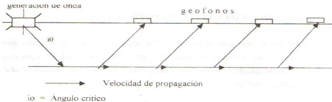
Fig. Esquema del método geofísico de refracción.
