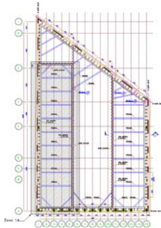
Fig. 16 b Procedimiento constructivo Etapa 1a.
