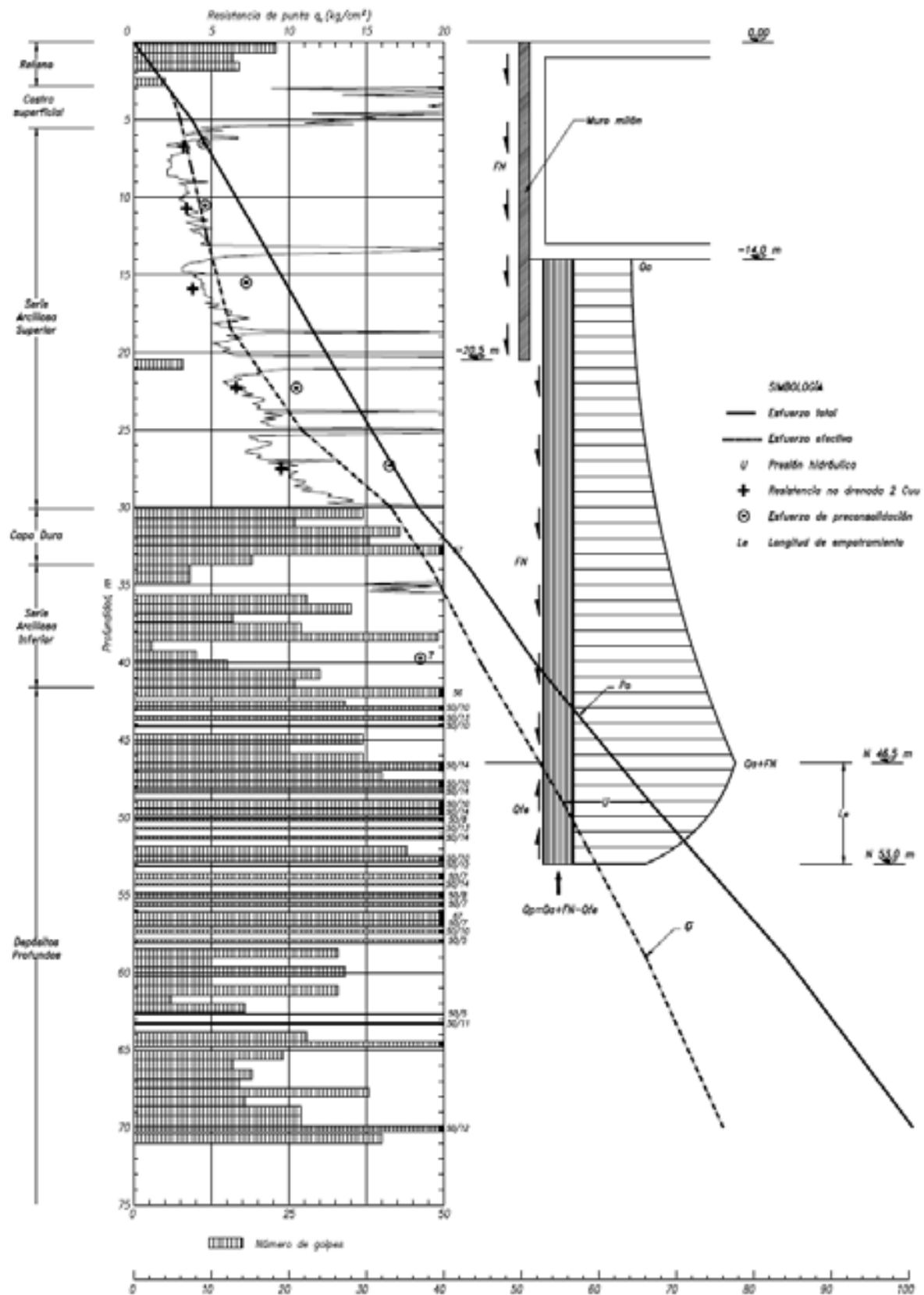
Fig. 10 SE -1 Condiciones geotécnicas de diseño.
