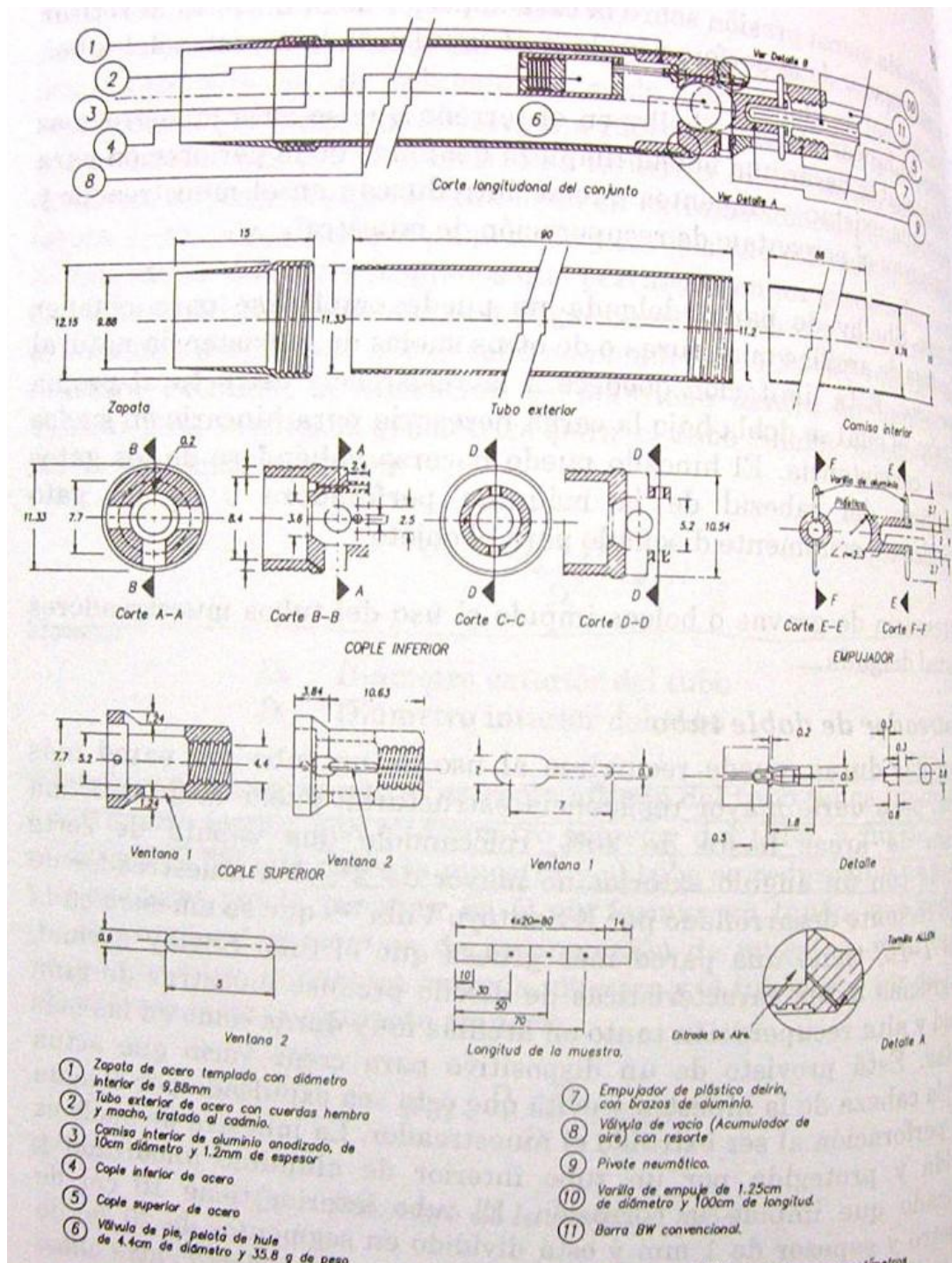
Fig. Muestreador de doble tubo.
