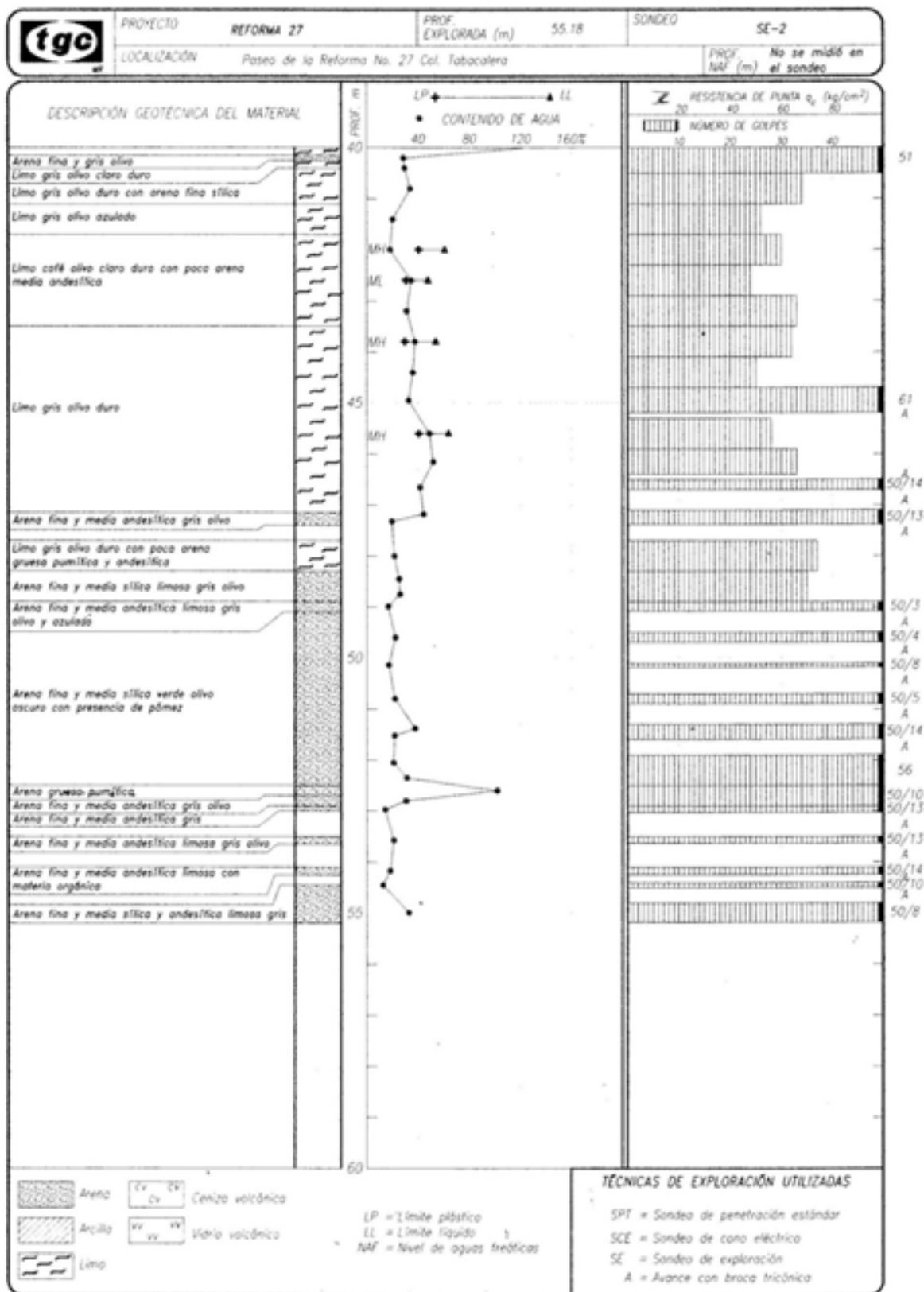
Fig. 2-4c Registro de exploración geotécnica (SPT).
