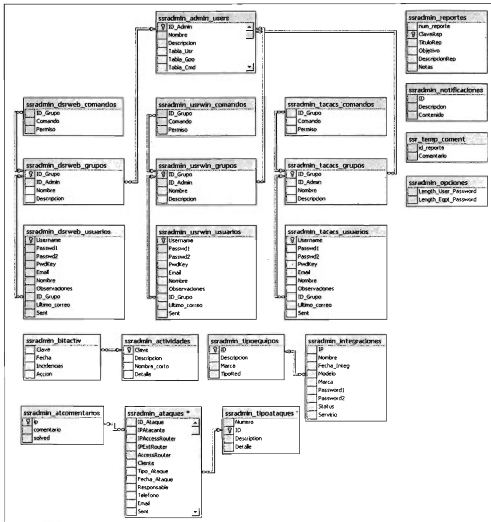
Figura 4.1.4.1 Diagrama Entidad-Relación
