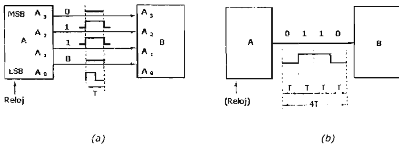
Figura 2.1 Transmisión de datos: (a) paralelo, (b) serie.
