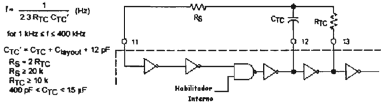
Figura 3.12 Oscilador RC.
