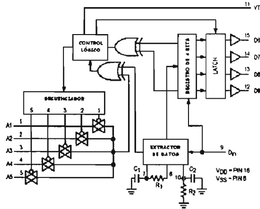
Figura 3.15 Diagrama de bloques del decodificador MC145027
