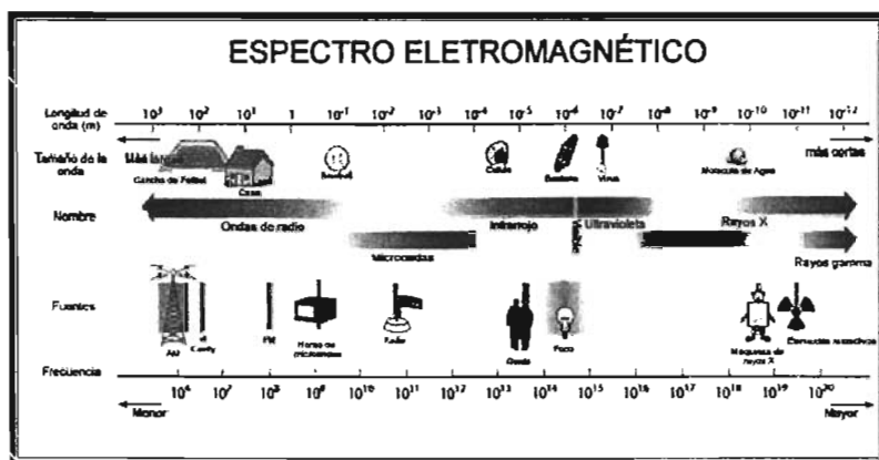
Figura 3.6 Espectro Electromagnético.
