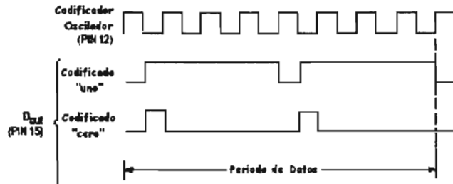
Figura 3.11 Codificación de estados.
