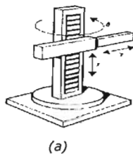
Fig. 1.3 Esquema de movimientos de coordenadas cilíndricas. (b) Robot con configuración de coordenadas cilíndricas.
