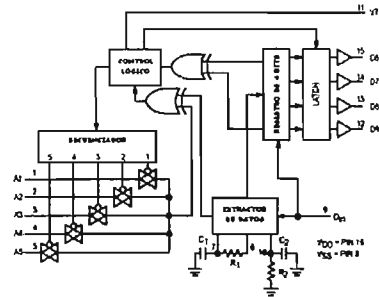
Diagrama de Bloques del Decodificador
