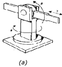
Fig. 1.2 (a) Esquema de movimientos de coordenadas polares. (b) Robot con configuración de coordenadas polares.
