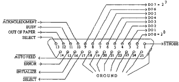
Fig. 2.2 Conector hembra DB-25S.
