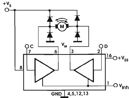
Fig. 4.9 Diagrama esquemático de un CI L293B
