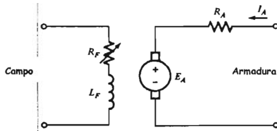
Fig. 4.2 Circuito equivalente de un motor de CD.
