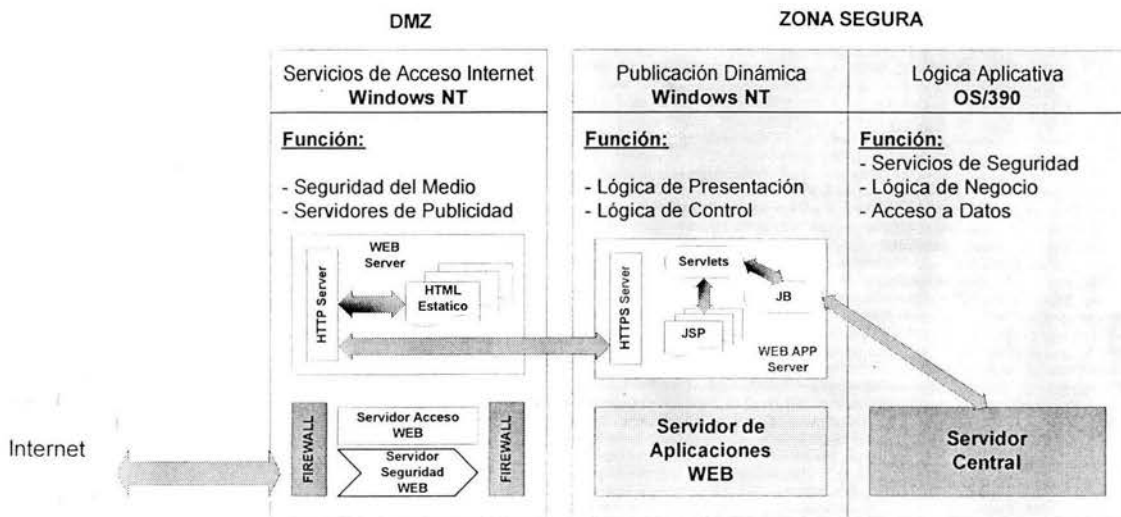
Figura 4.4 Esquema de operación del acceso a Internet
