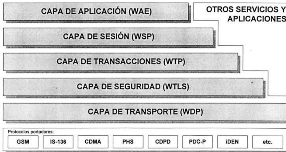
Figura 2.3 Arquitectura de WAP
