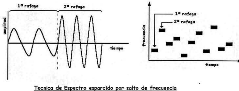
Figura 1.2. Técnica de espectro por salto de frecuencia
