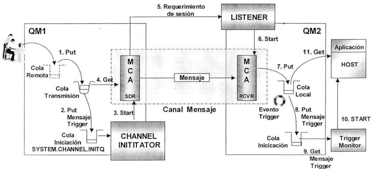
Figura 4.8 Componentes de MQ Series®
