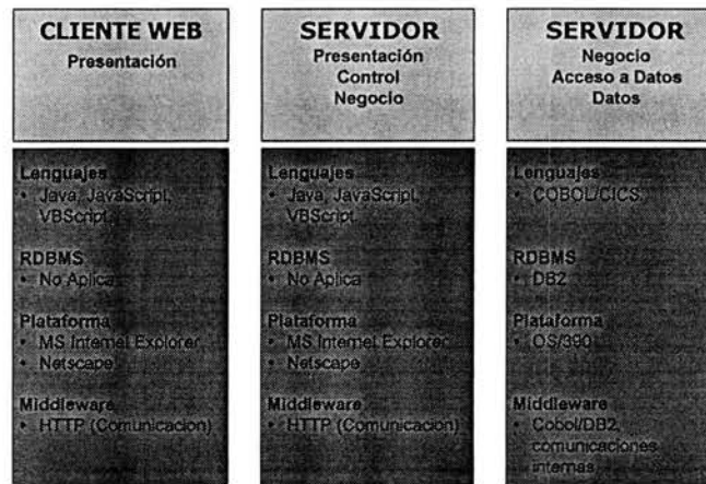
Figura 4.2 Modelo de 3 Capas Web
