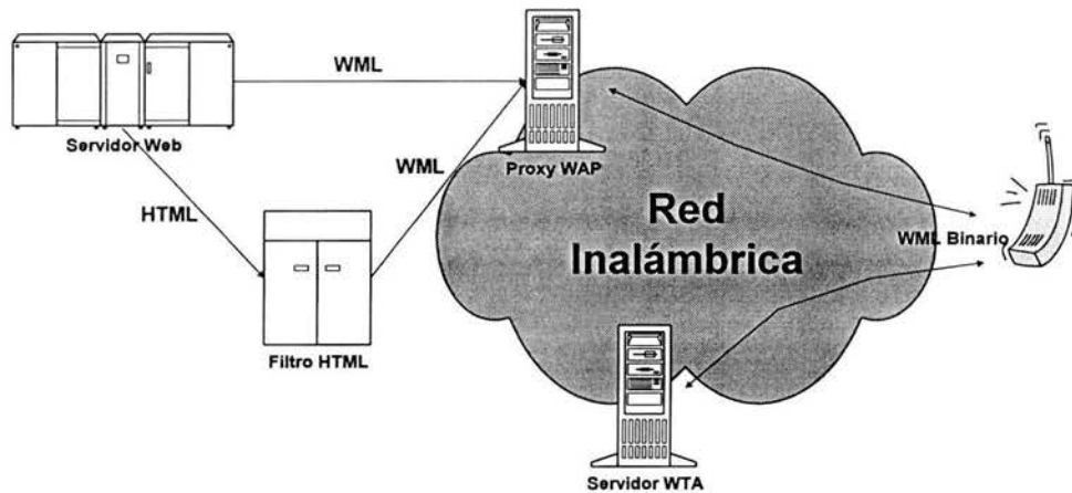
Figura 2.2 Ejemplo de una red WAP
